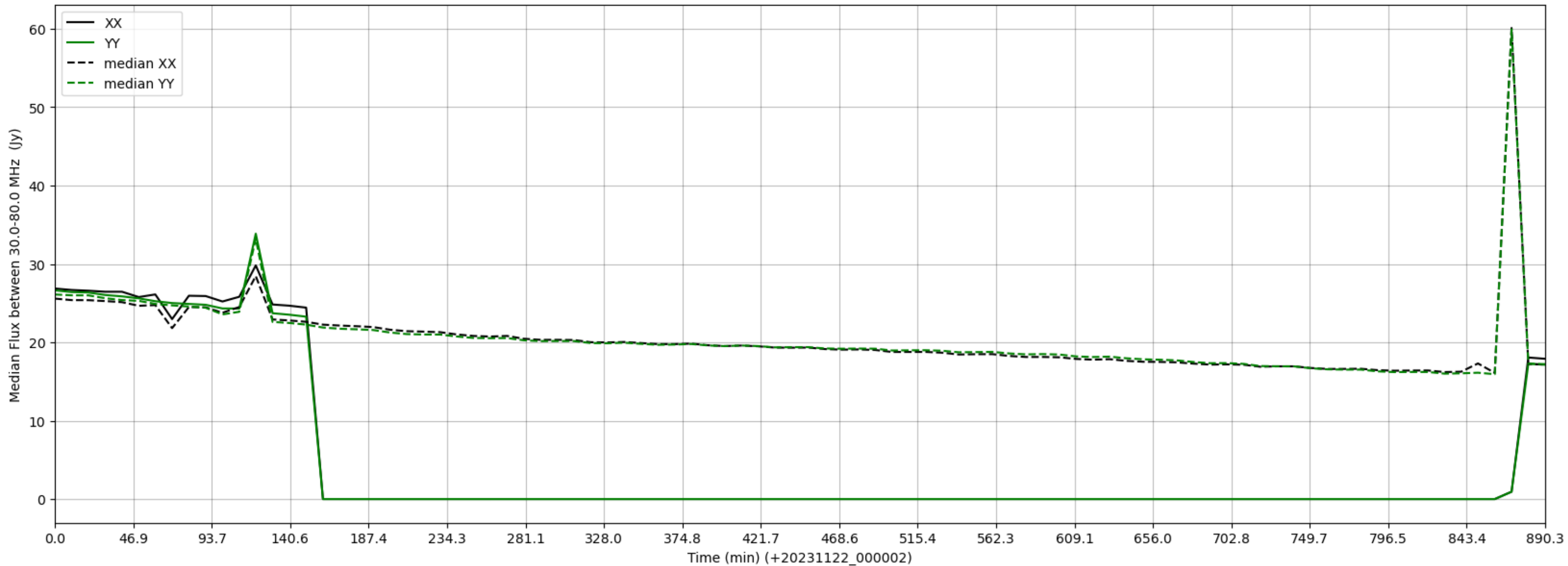
LWA031 - Correlator# 131 - XX FLAGS:LowFlux - YY FLAGS:LowFlux
