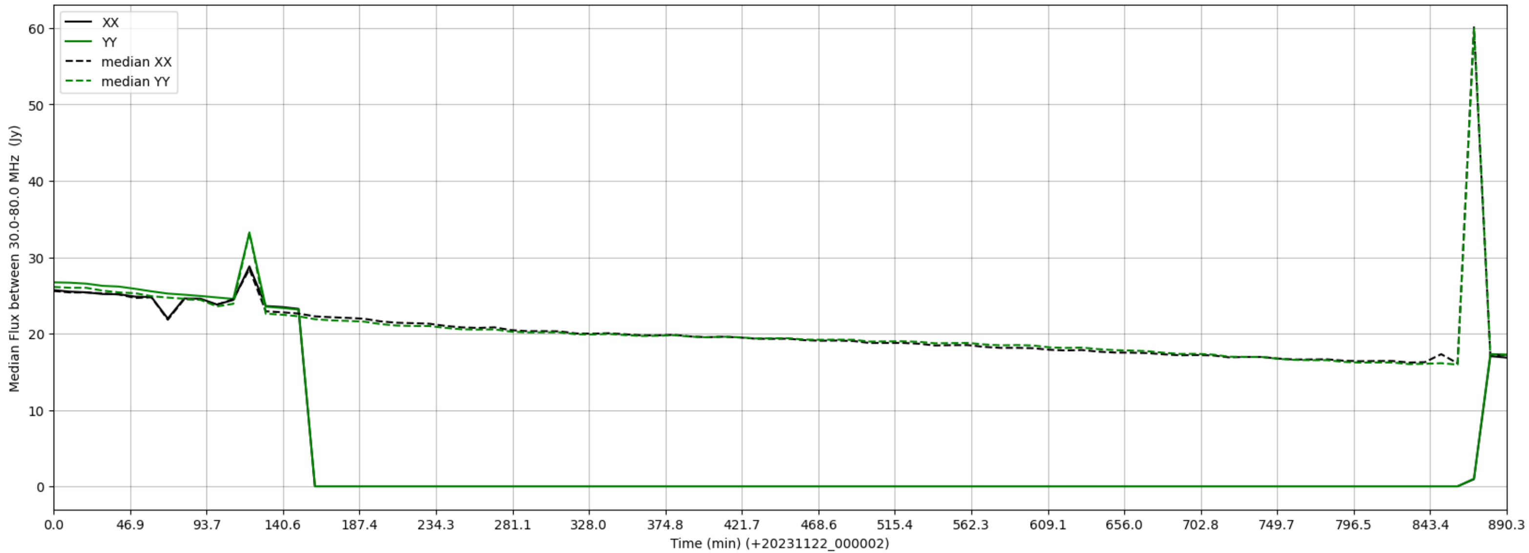
LWA028 - Correlator# 129 - XX FLAGS:LowFlux - YY FLAGS:LowFlux
