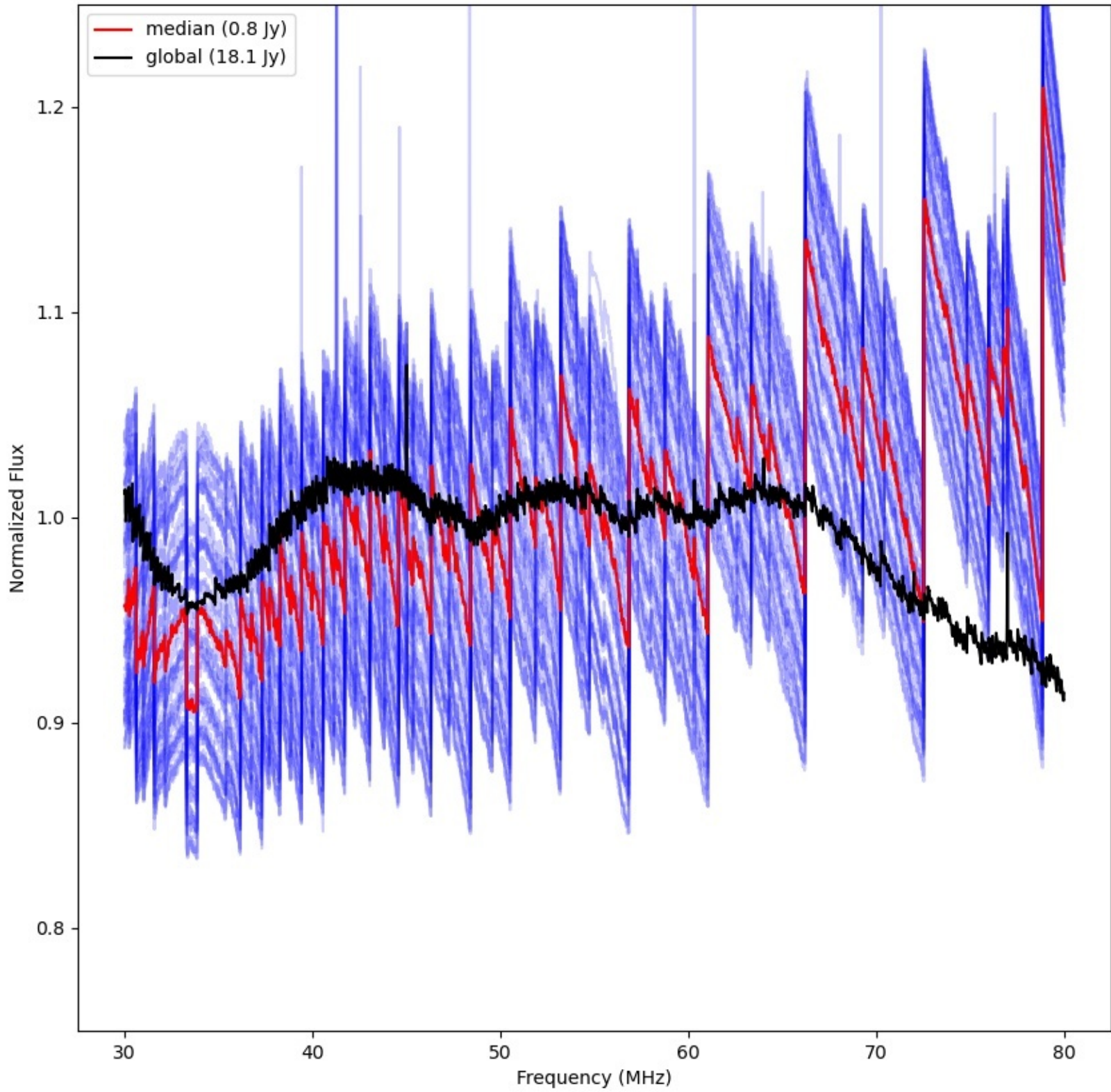
LWA203 - Correlator# 295 - XX - FLAGS:LowFlux
