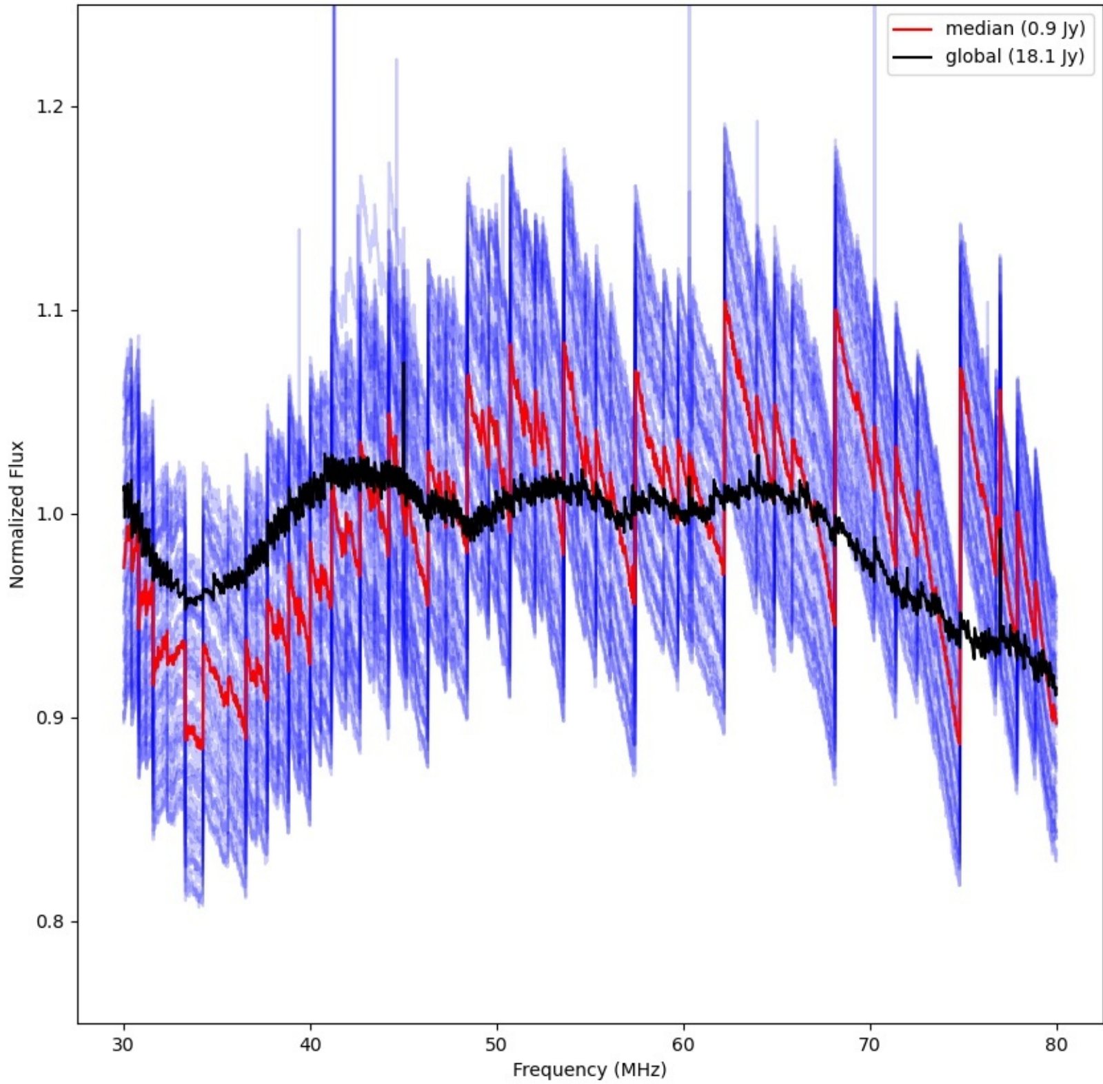
LWA207 - Correlator# 299 - XX - FLAGS:LowFlux
