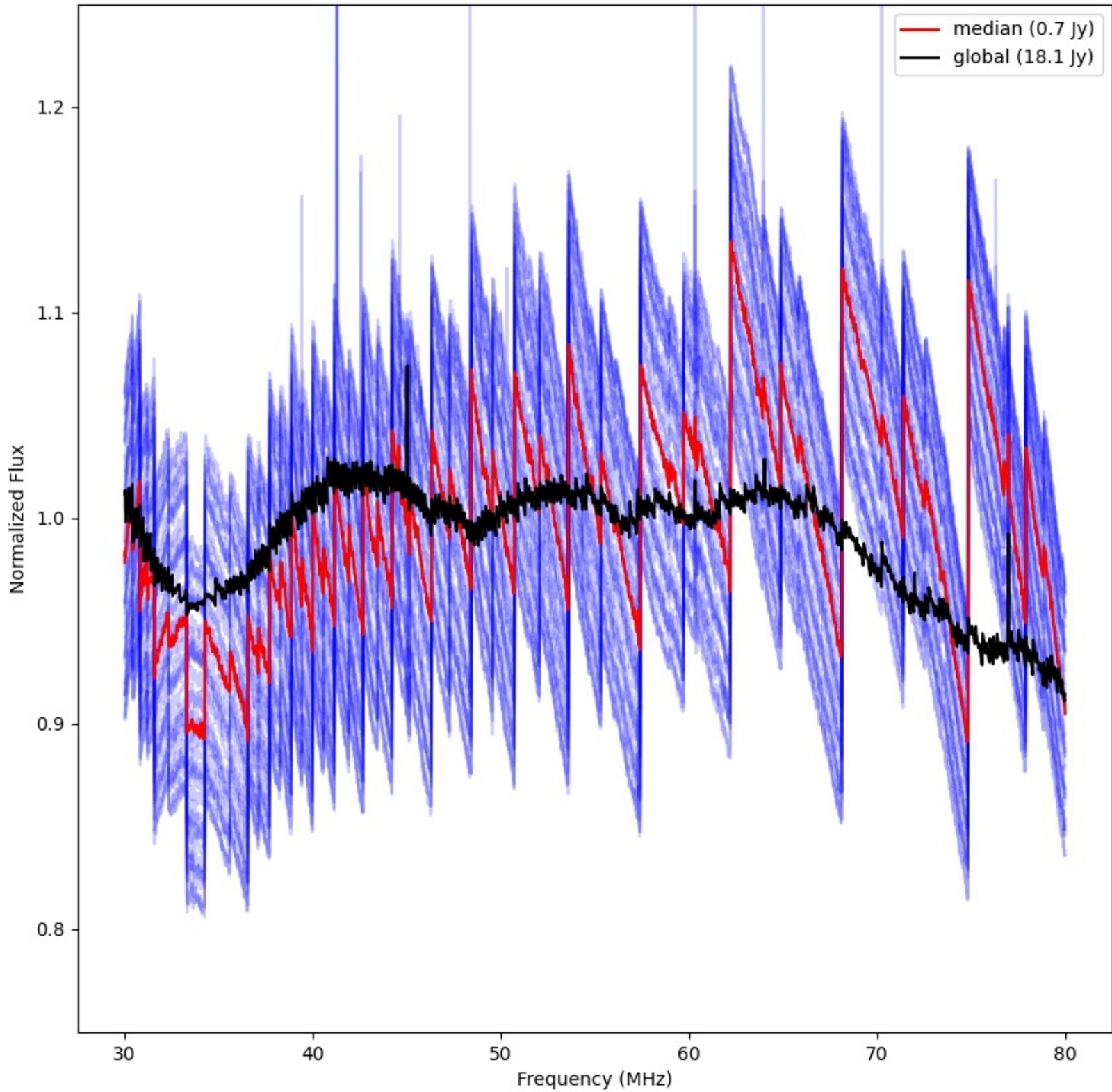
LWA206 - Correlator# 296 - XX - FLAGS:LowFlux
