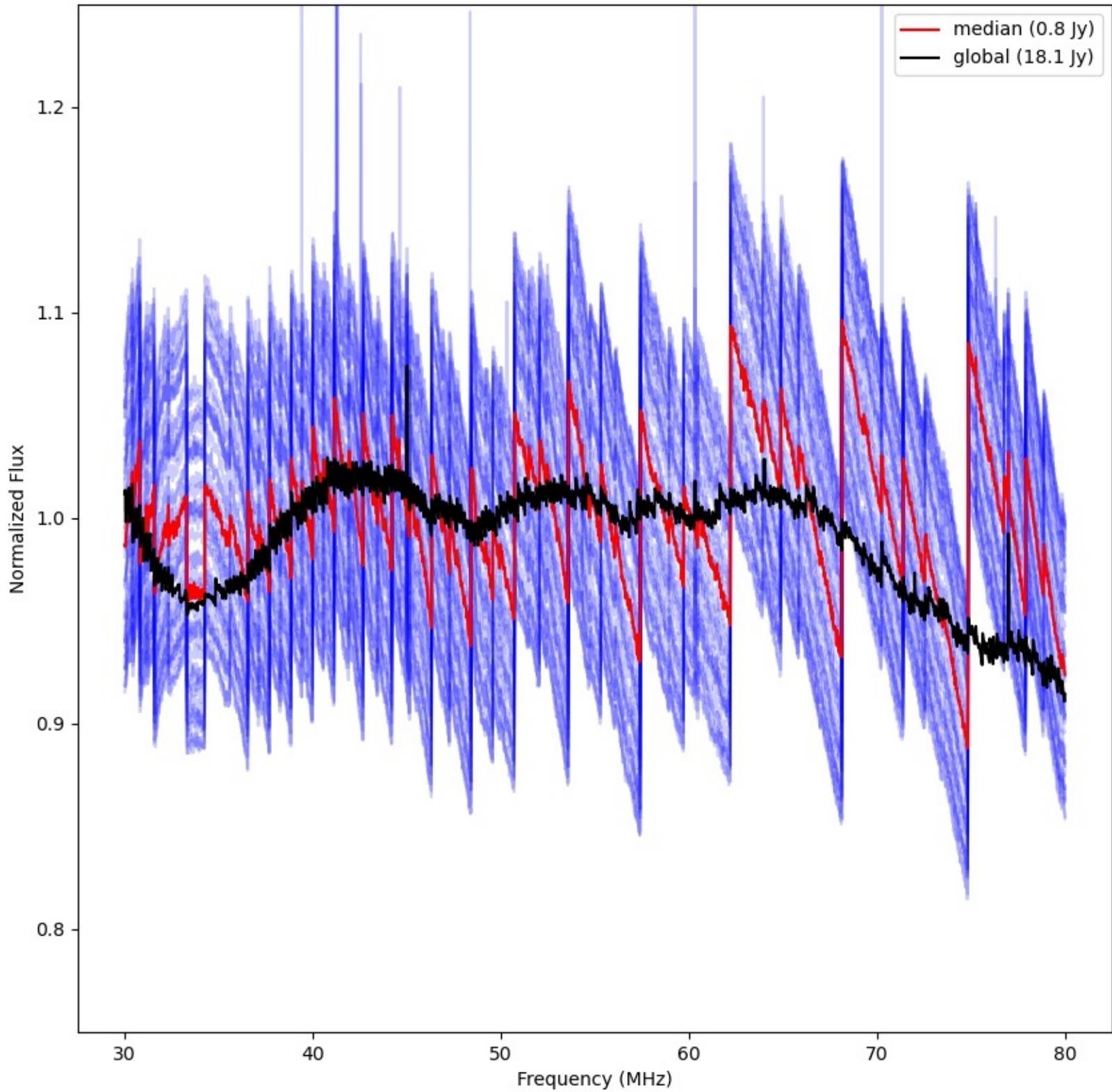
LWA205 - Correlator# 297 - XX - FLAGS:LowFlux
