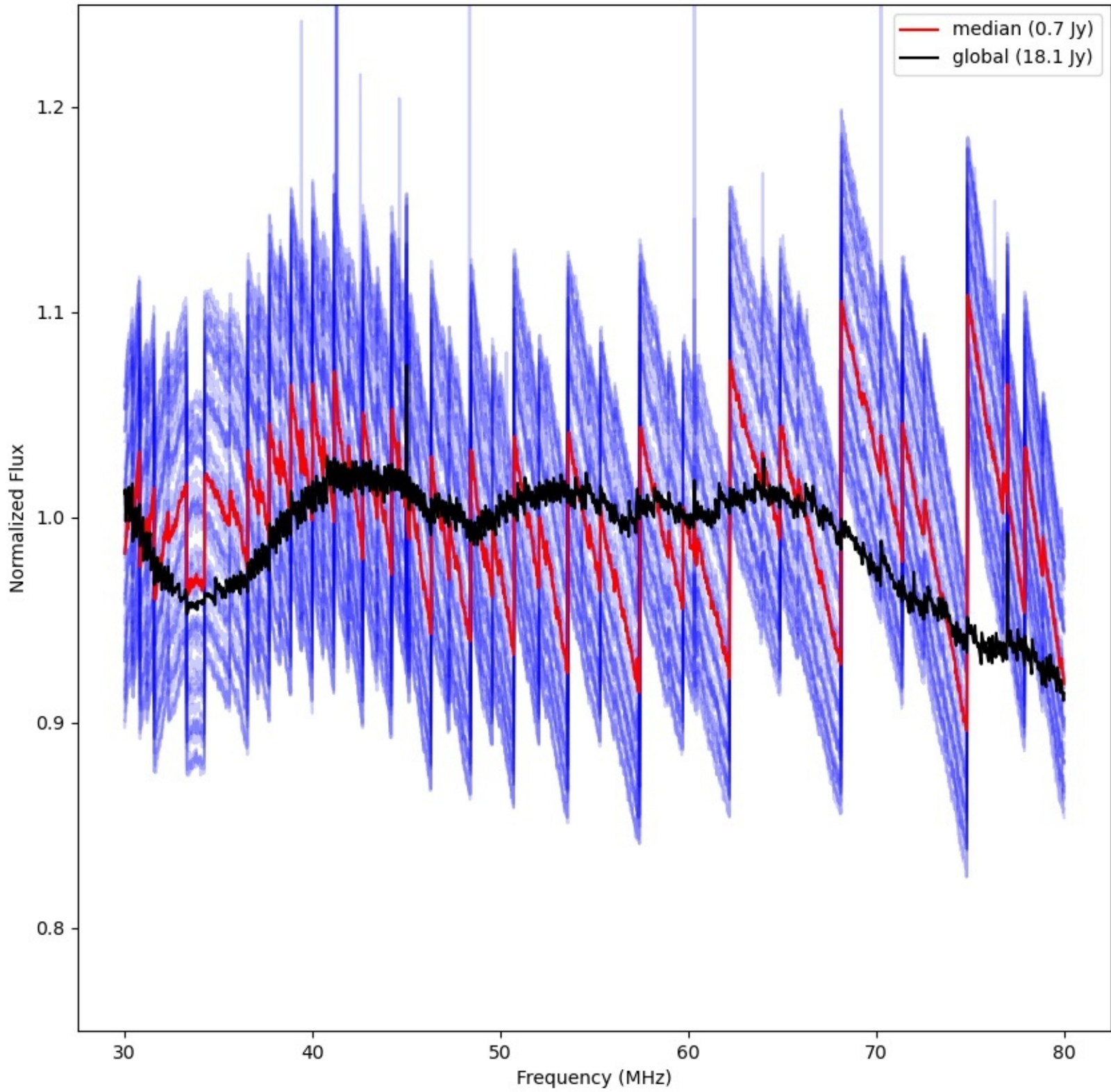
LWA173 - Correlator# 290 - XX - FLAGS:LowFlux
