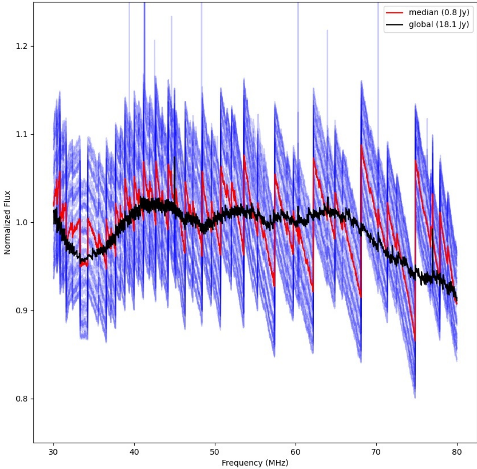
LWA204 - Correlator# 294 - XX - FLAGS:LowFlux
