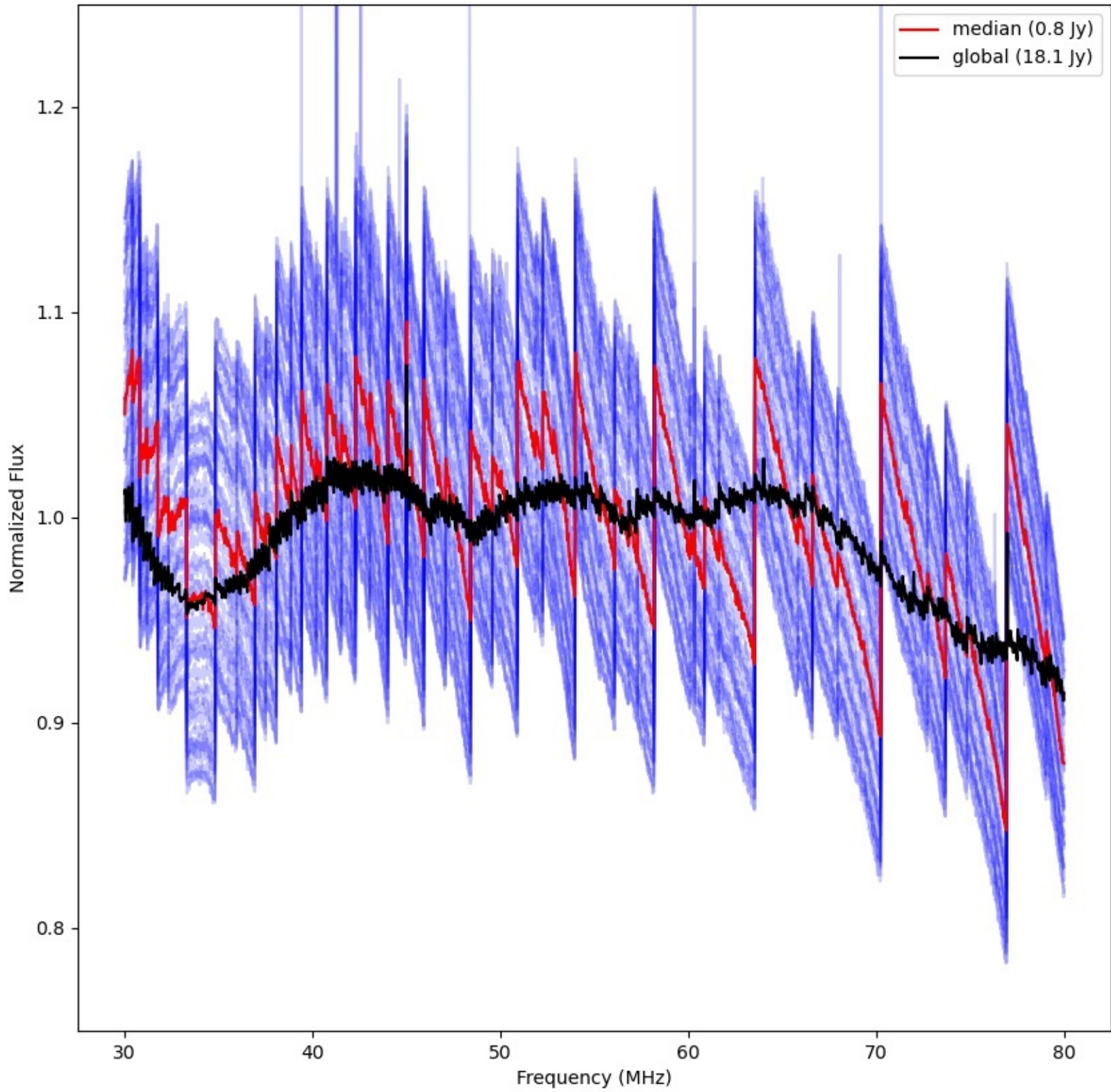
LWA175 - Correlator# 293 - XX - FLAGS:LowFlux
