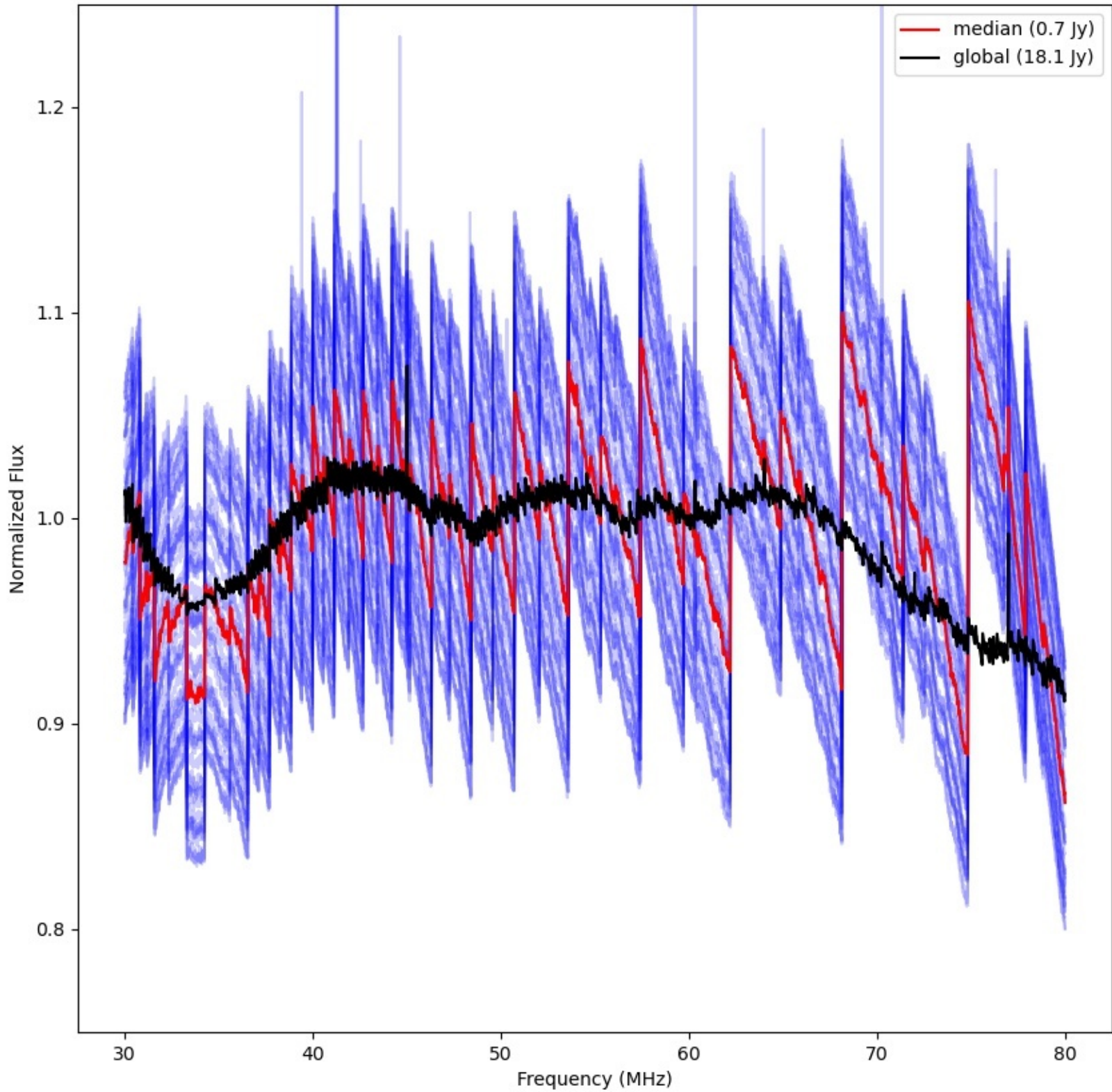
LWA169 - Correlator# 292 - XX - FLAGS:LowFlux
