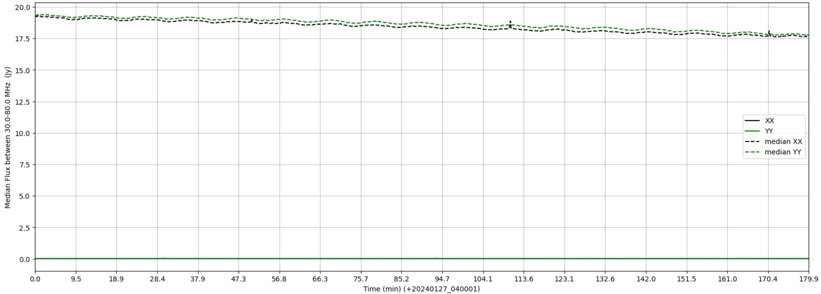
LWA365 - Correlator# 126 - XX FLAGS:LowFlux - YY FLAGS:LowFlux
