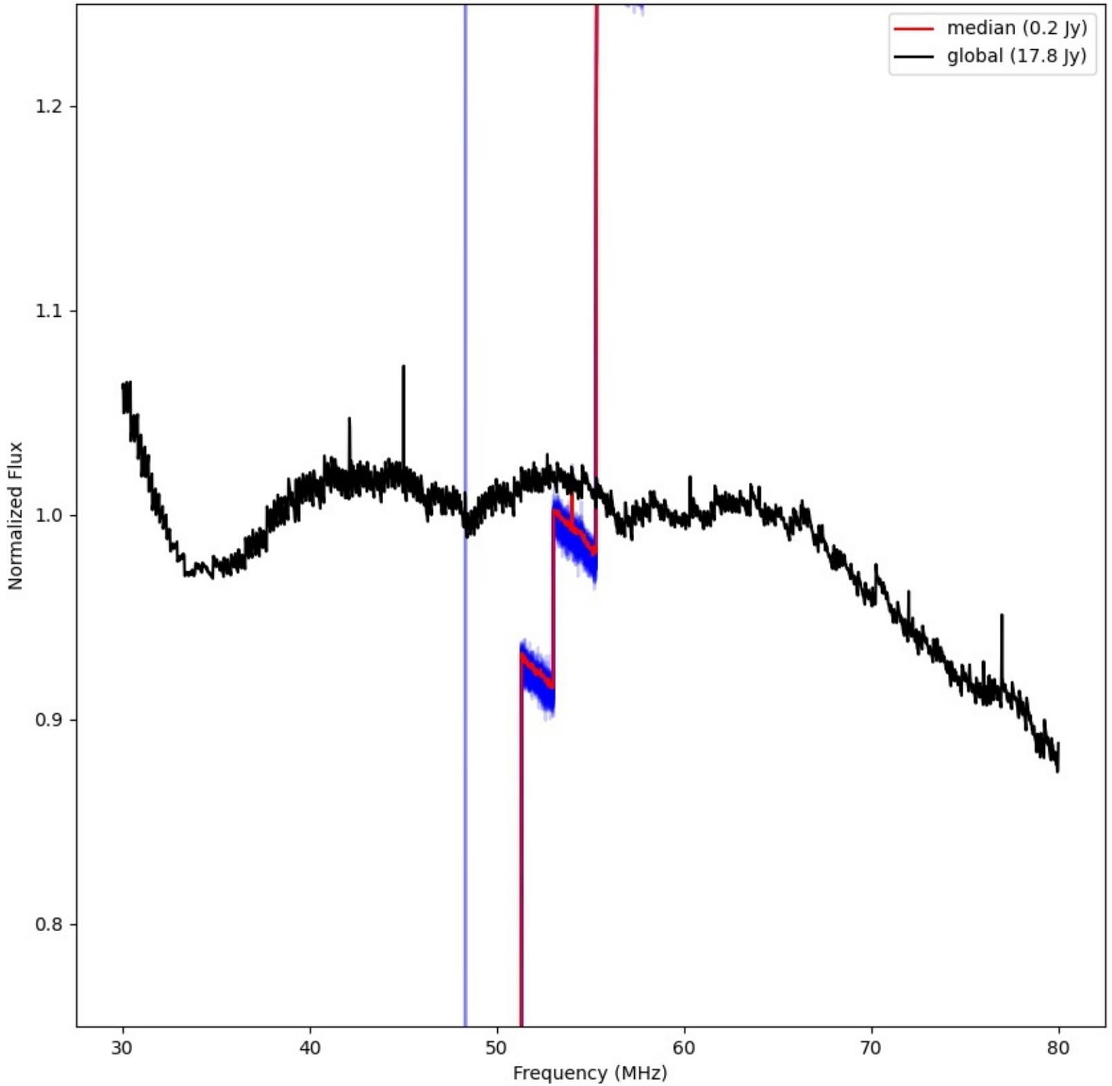
LWA320 - Correlator# 054 - XX - FLAGS:LowFlux
