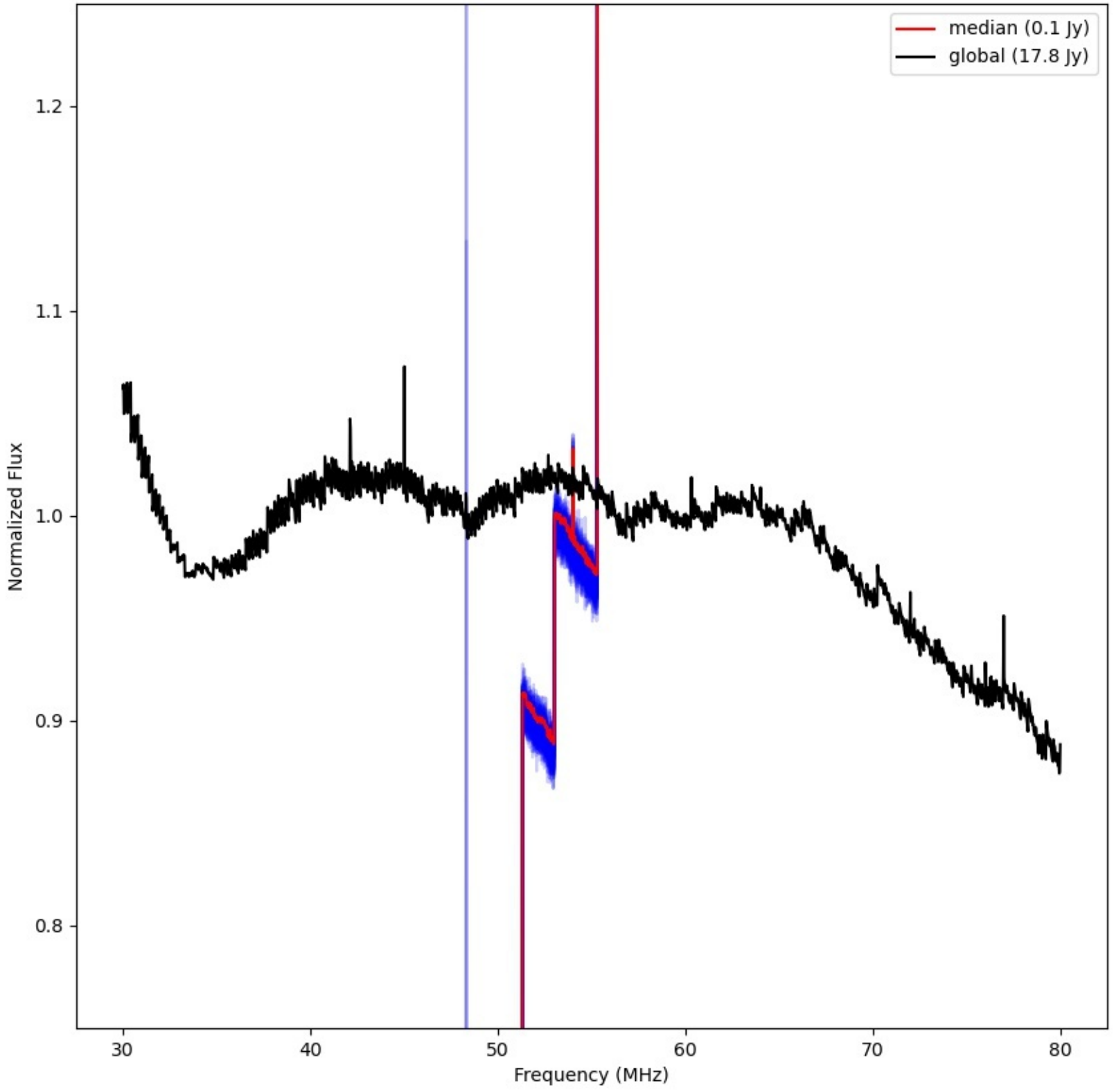
LWA334 - Correlator# 156 - XX - FLAGS:LowFlux
