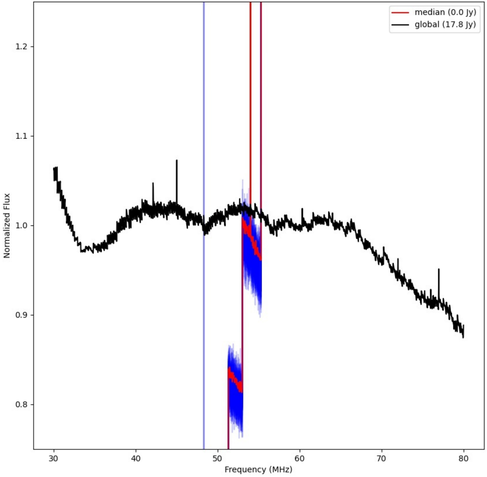
LWA257 - Correlator# 032 - XX - FLAGS:LowFlux
