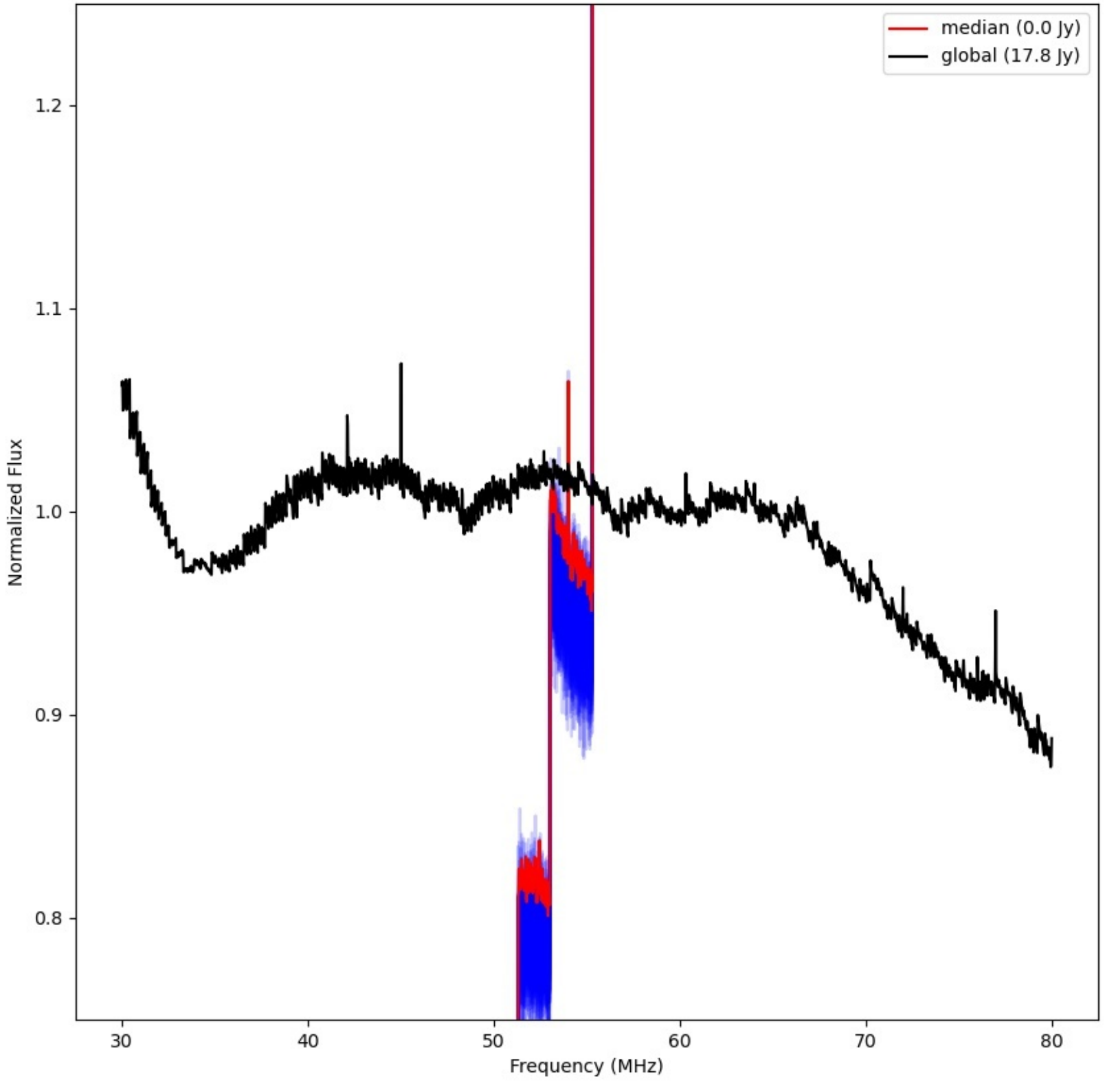
LWA304 - Correlator# 351 - XX - FLAGS:LowFlux
