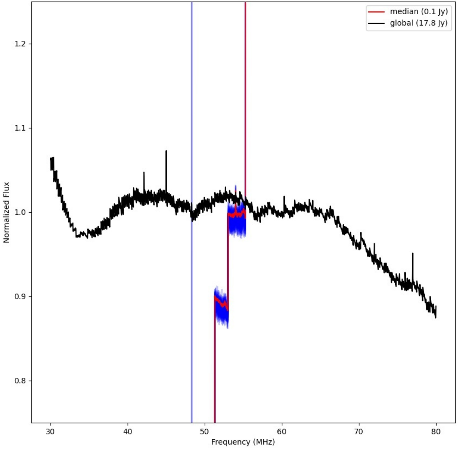
LWA297 - Correlator# 314 - XX - FLAGS:LowFlux
