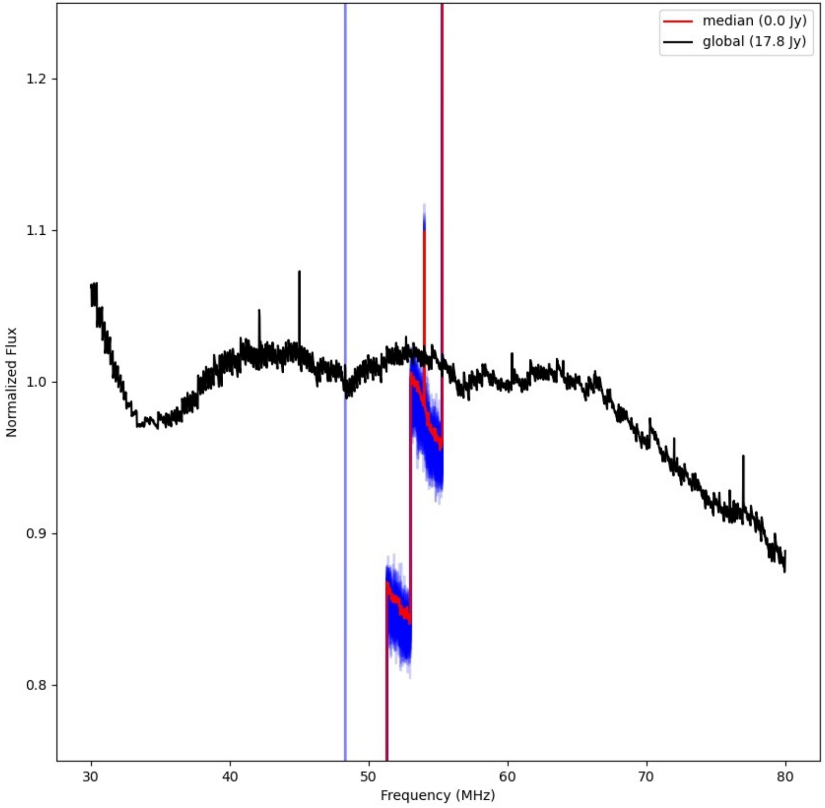
LWA325 - Correlator# 154 - XX - FLAGS:LowFlux
