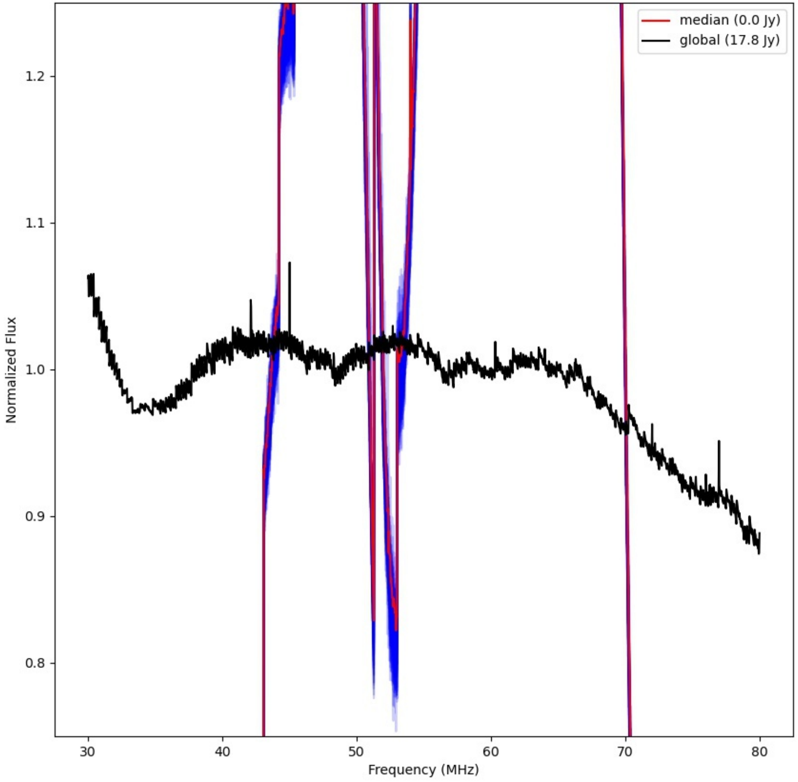
LWA335 - Correlator# 057 - XX - FLAGS:LowFlux
