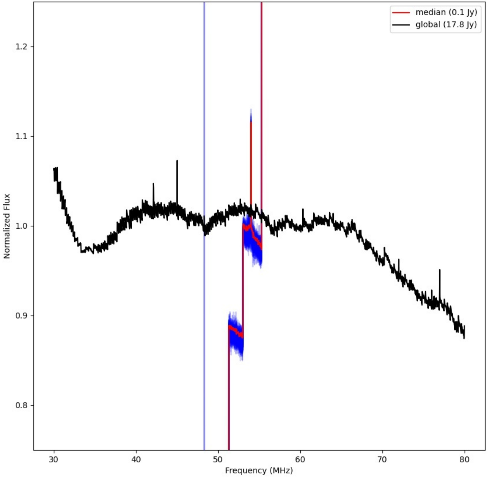
LWA337 - Correlator# 059 - XX - FLAGS:LowFlux
