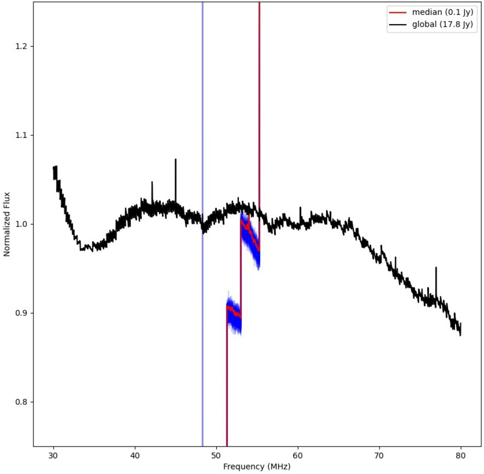
LWA351 - Correlator# 060 - XX - FLAGS:LowFlux
