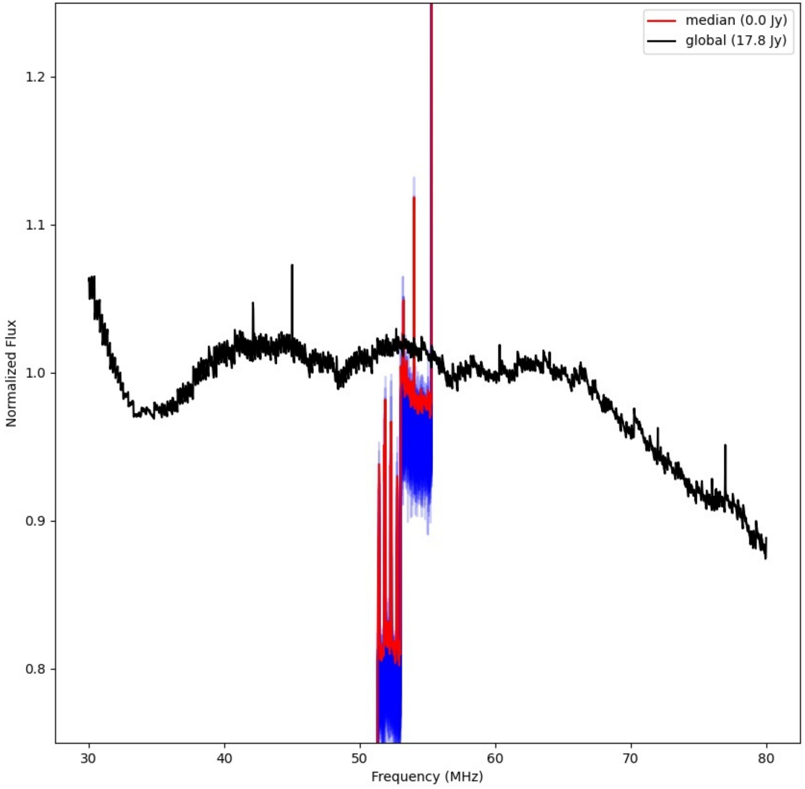
LWA303 - Correlator# 051 - XX - FLAGS:LowFlux
