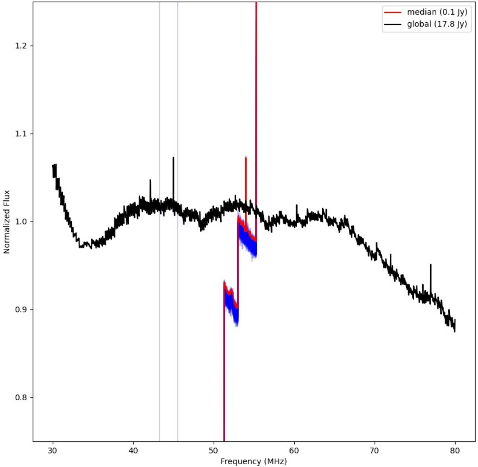
LWA324 - Correlator# 122 - XX - FLAGS:LowFlux
