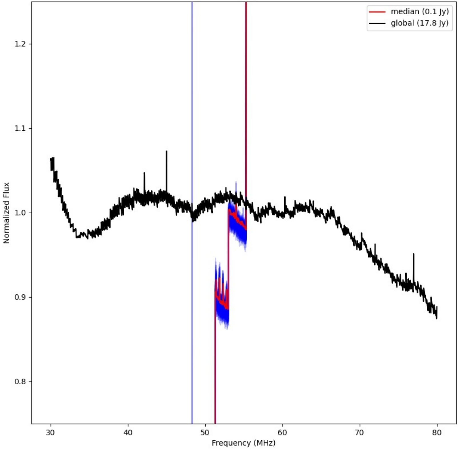
LWA298 - Correlator# 049 - XX - FLAGS:LowFlux
