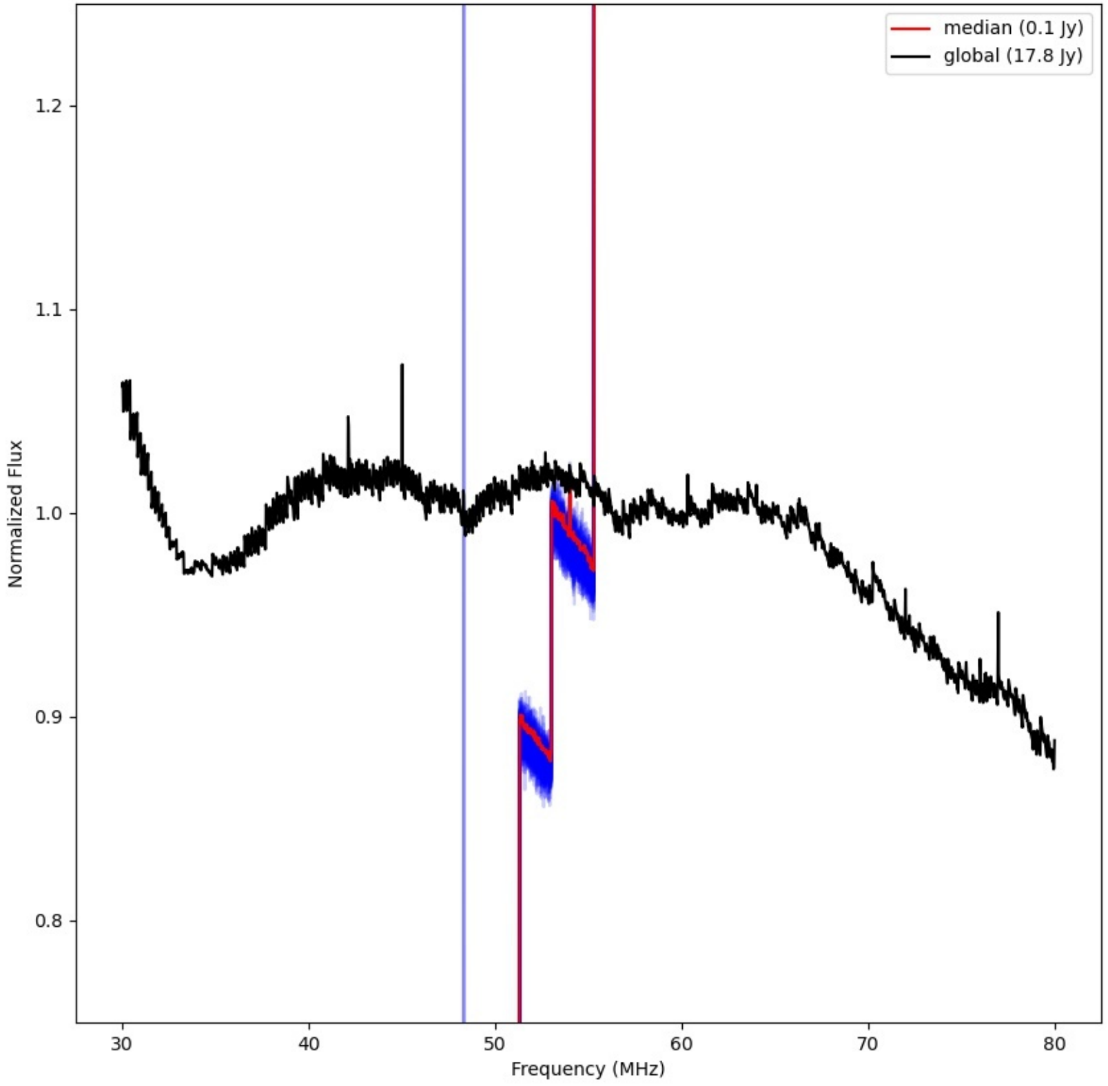
LWA343 - Correlator# 058 - XX - FLAGS:LowFlux
