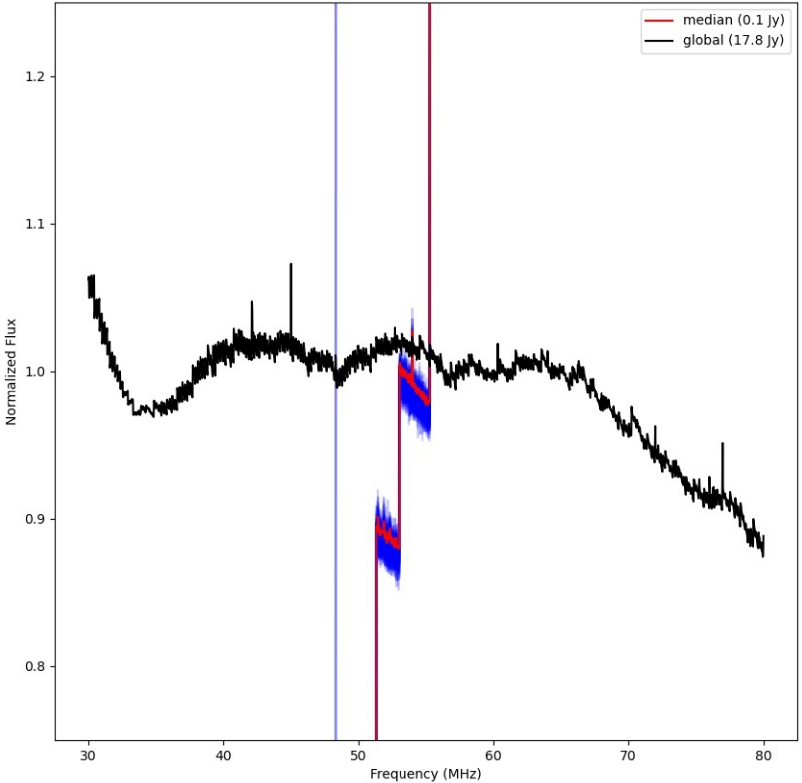
LWA292 - Correlator# 044 - XX - FLAGS:LowFlux
