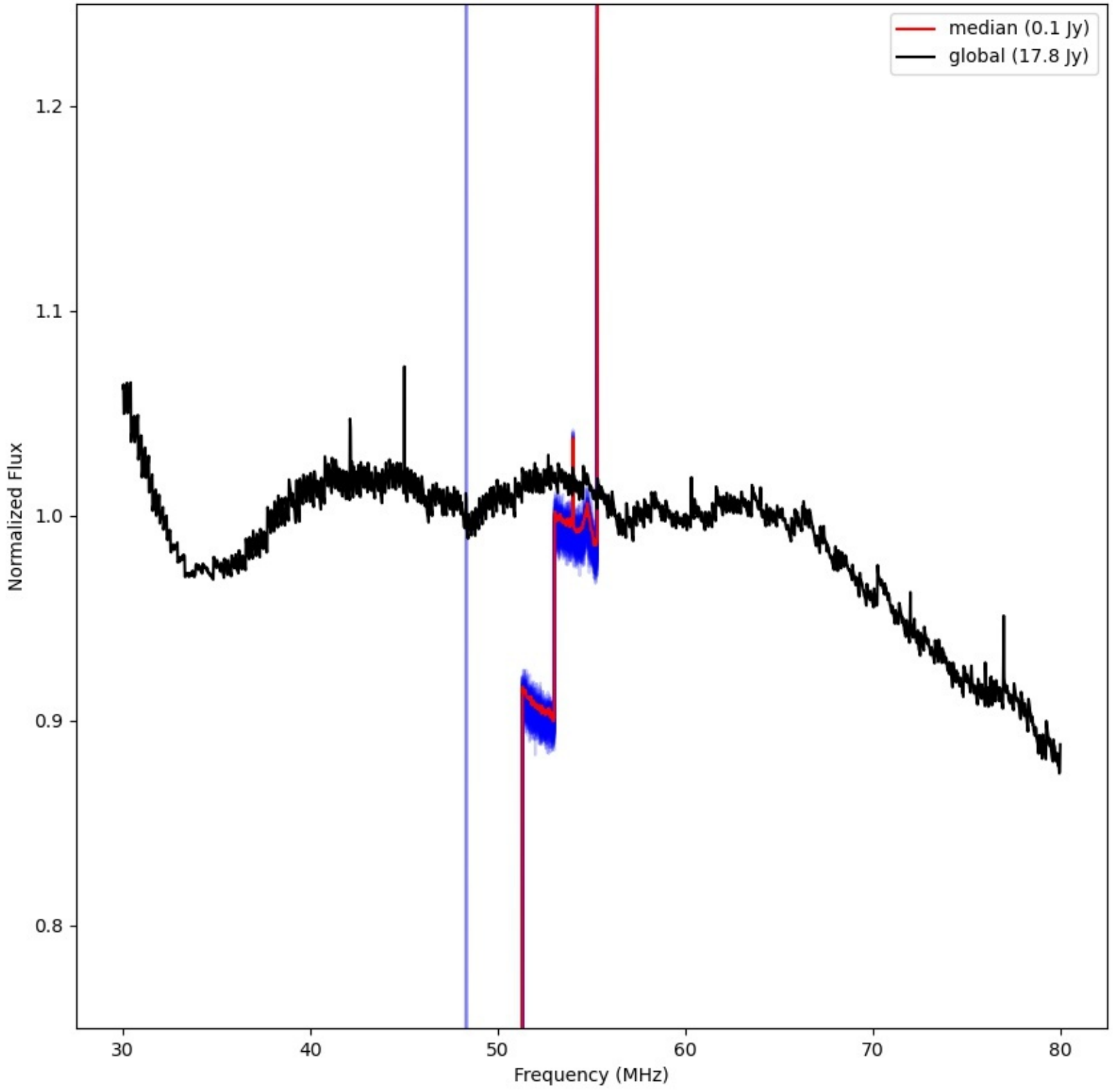
LWA350 - Correlator# 319 - XX - FLAGS:LowFlux
