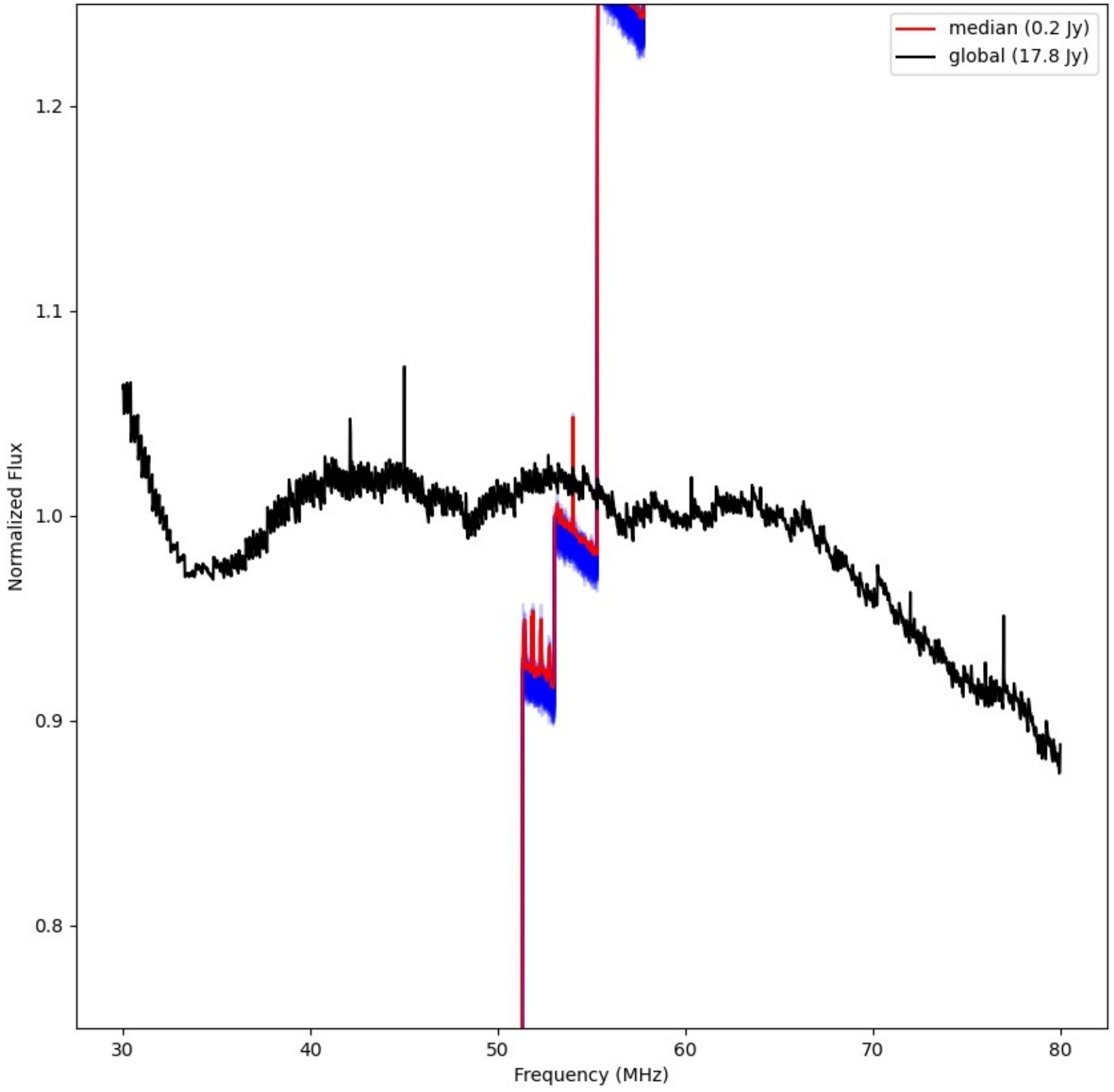
LWA305 - Correlator# 050 - XX - FLAGS:LowFlux
