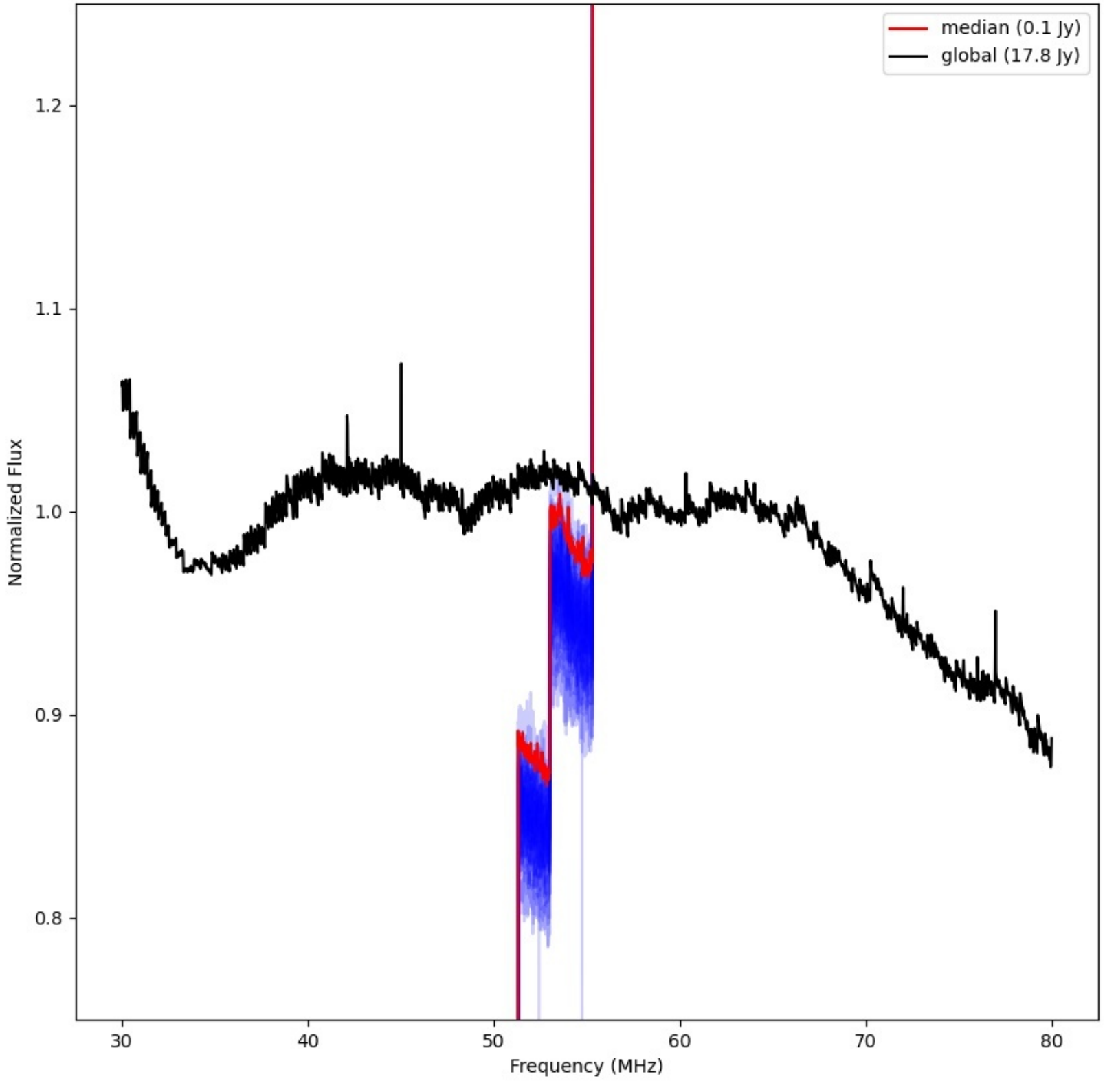
LWA299 - Correlator# 191 - XX - FLAGS:LowFlux
