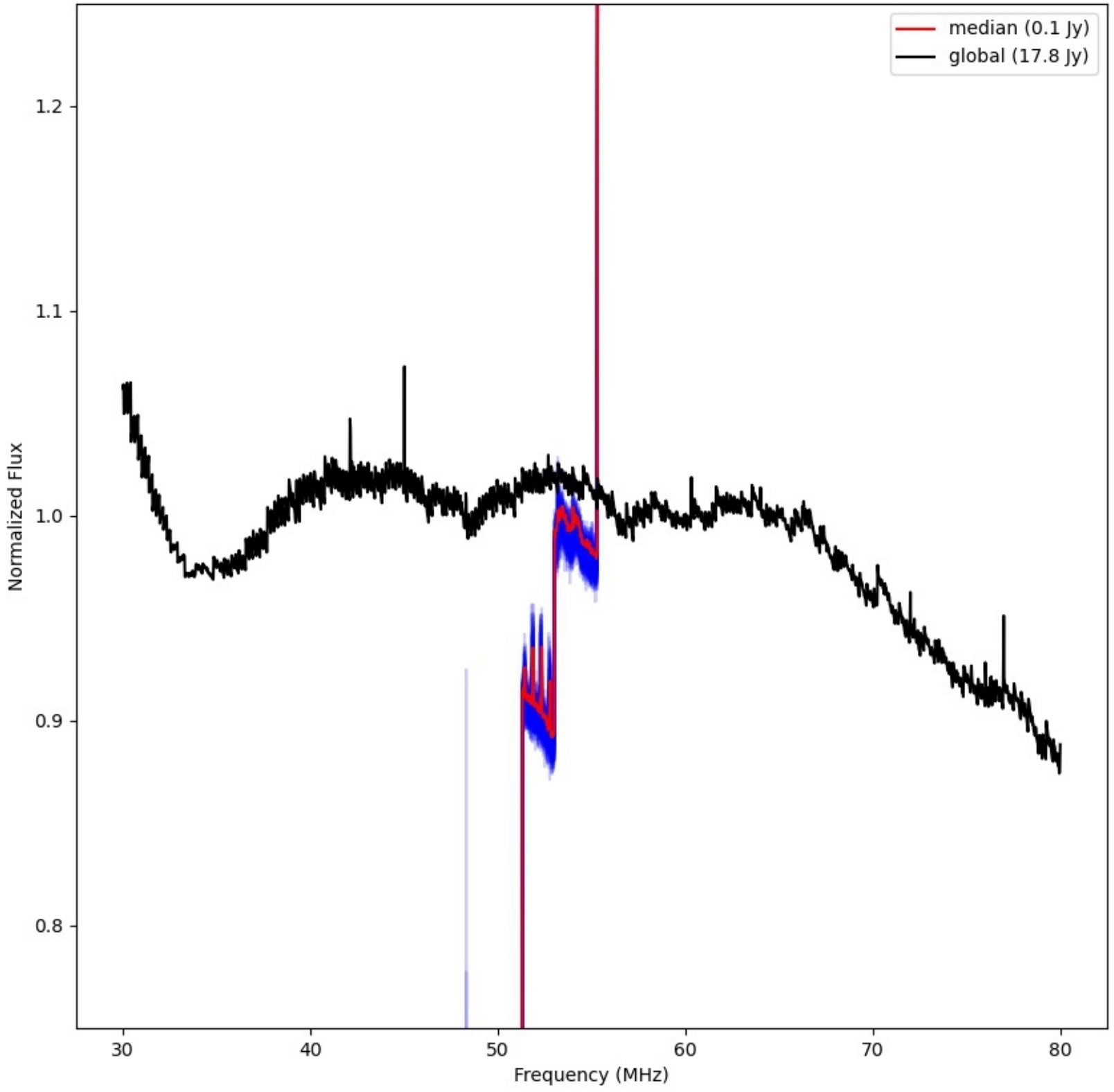
LWA309 - Correlator# 014 - XX - FLAGS:LowFlux
