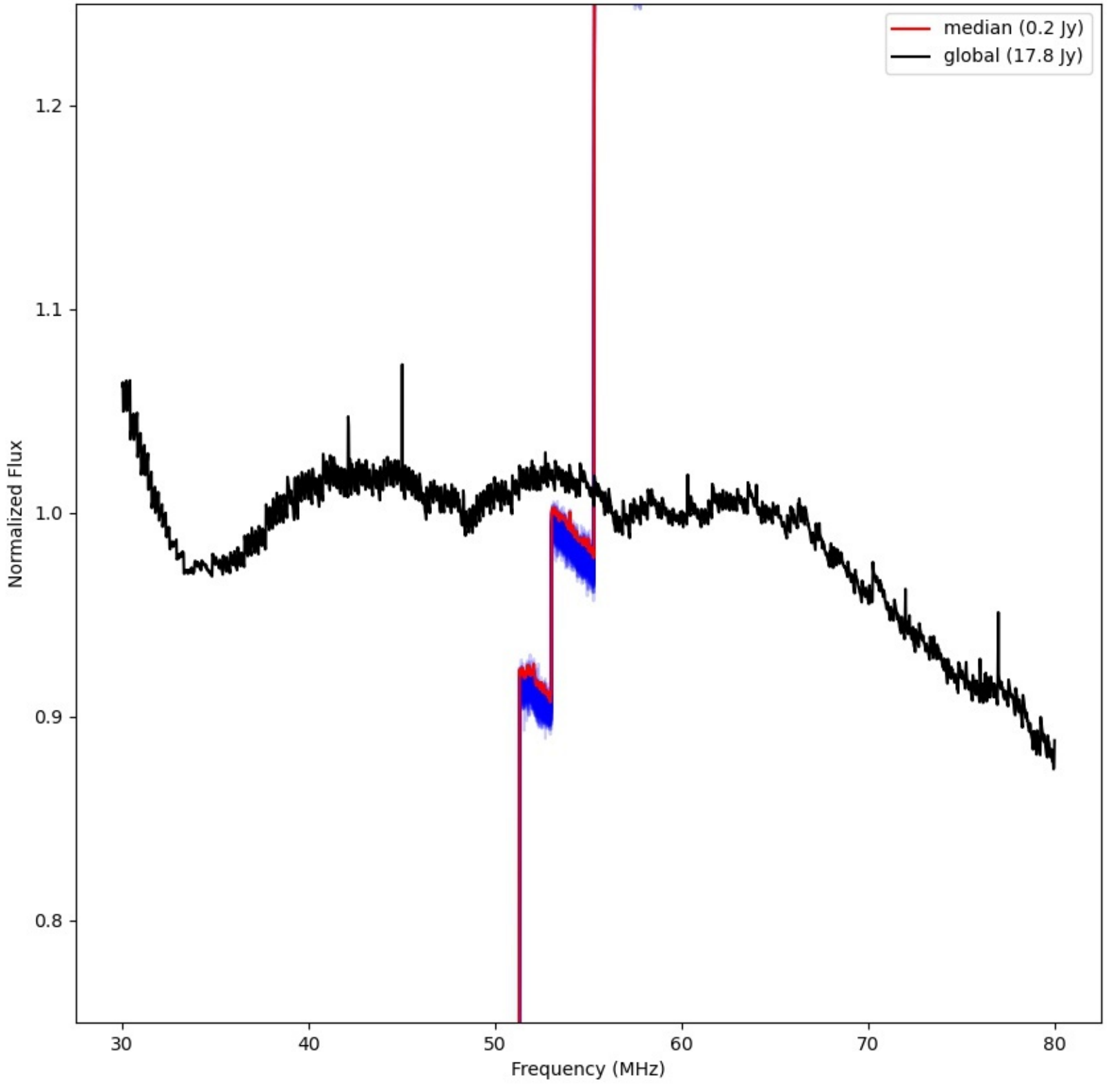
LWA294 - Correlator# 188 - XX - FLAGS:LowFlux
