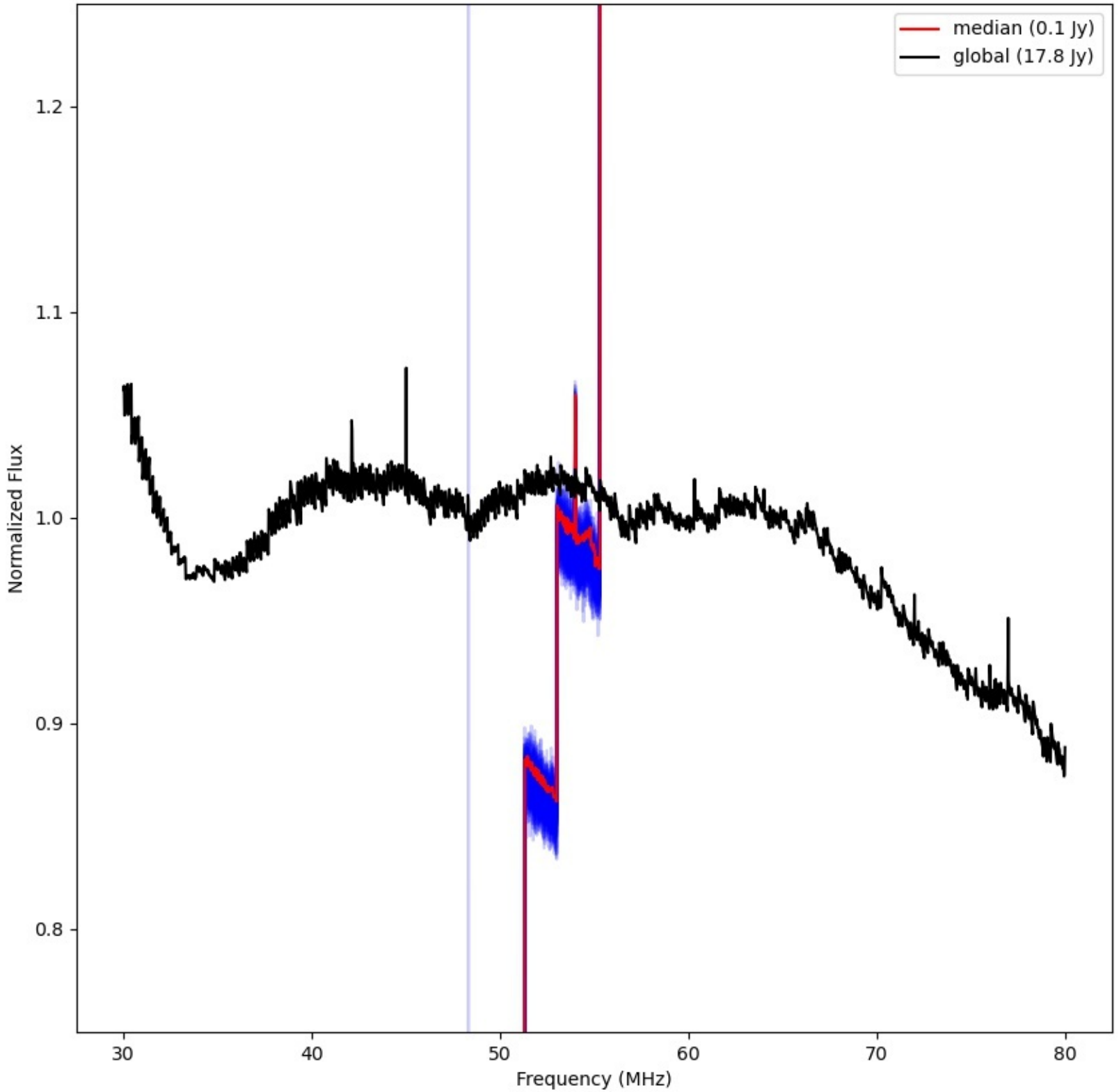
LWA259 - Correlator# 001 - XX - FLAGS:LowFlux
