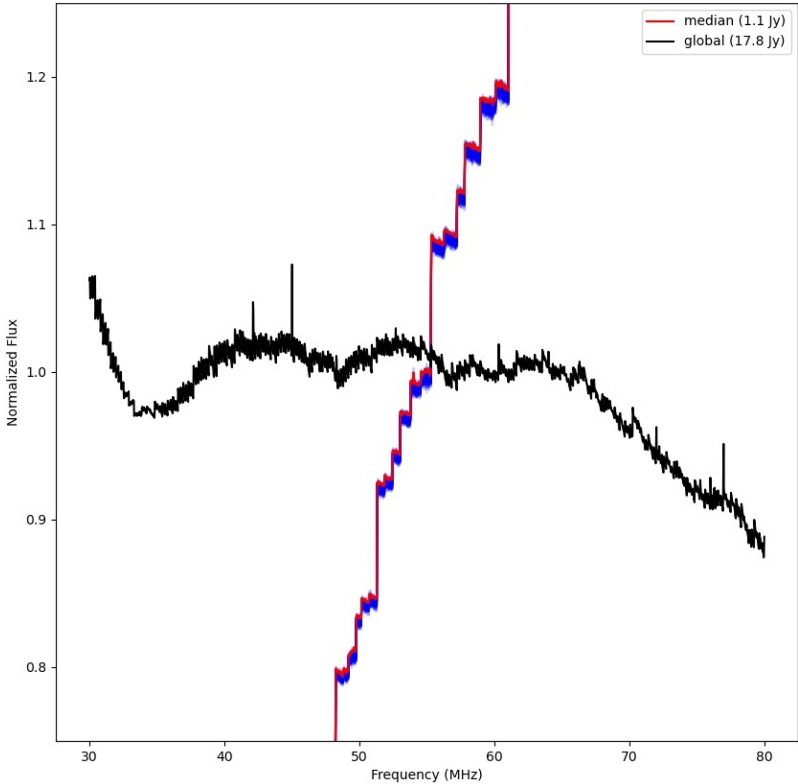
LWA317 - Correlator# 052 - XX - FLAGS:LowFlux
