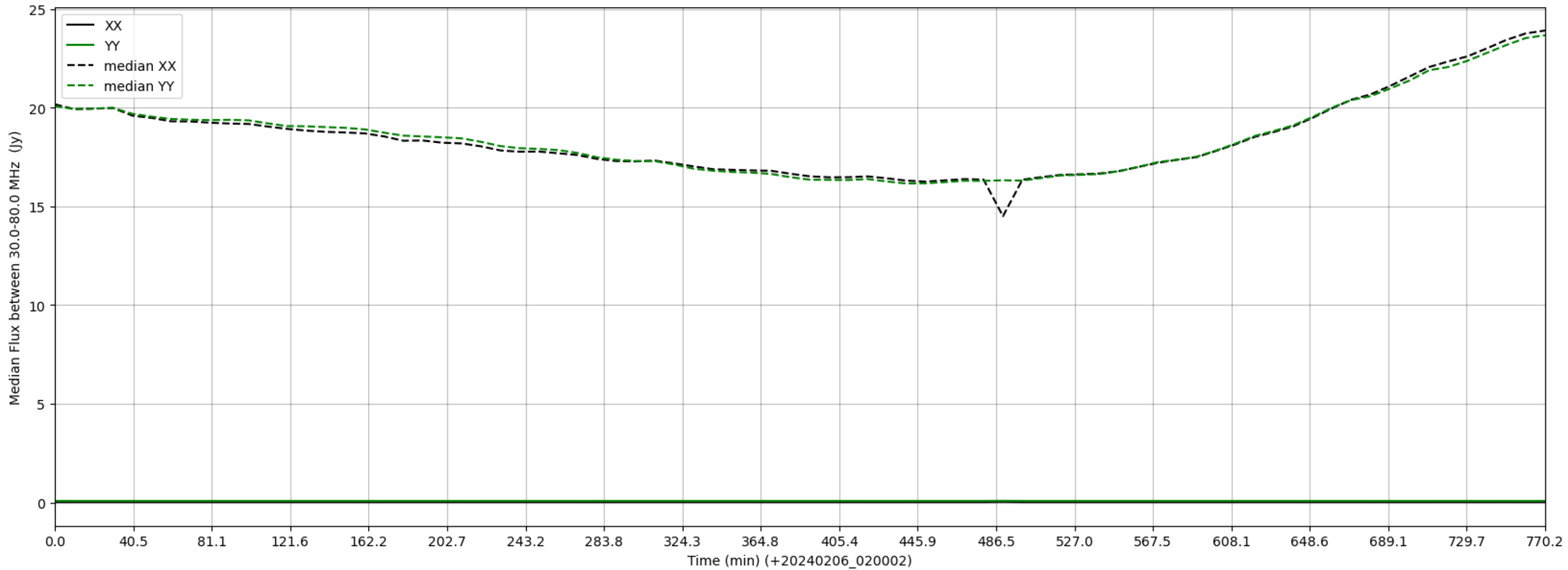
LWA263 - Correlator# 037 - XX FLAGS:LowFlux - YY FLAGS:LowFlux
