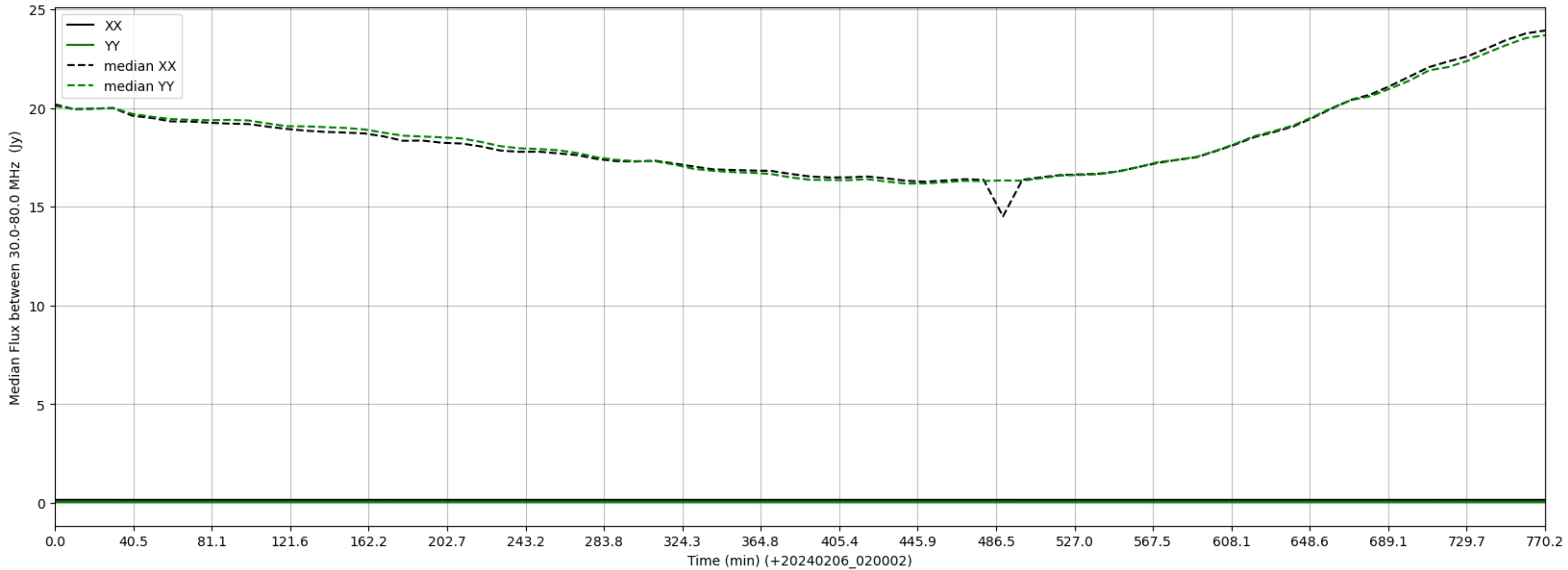
LWA301 - Correlator# 048 - XX FLAGS:LowFlux - YY FLAGS:LowFlux
