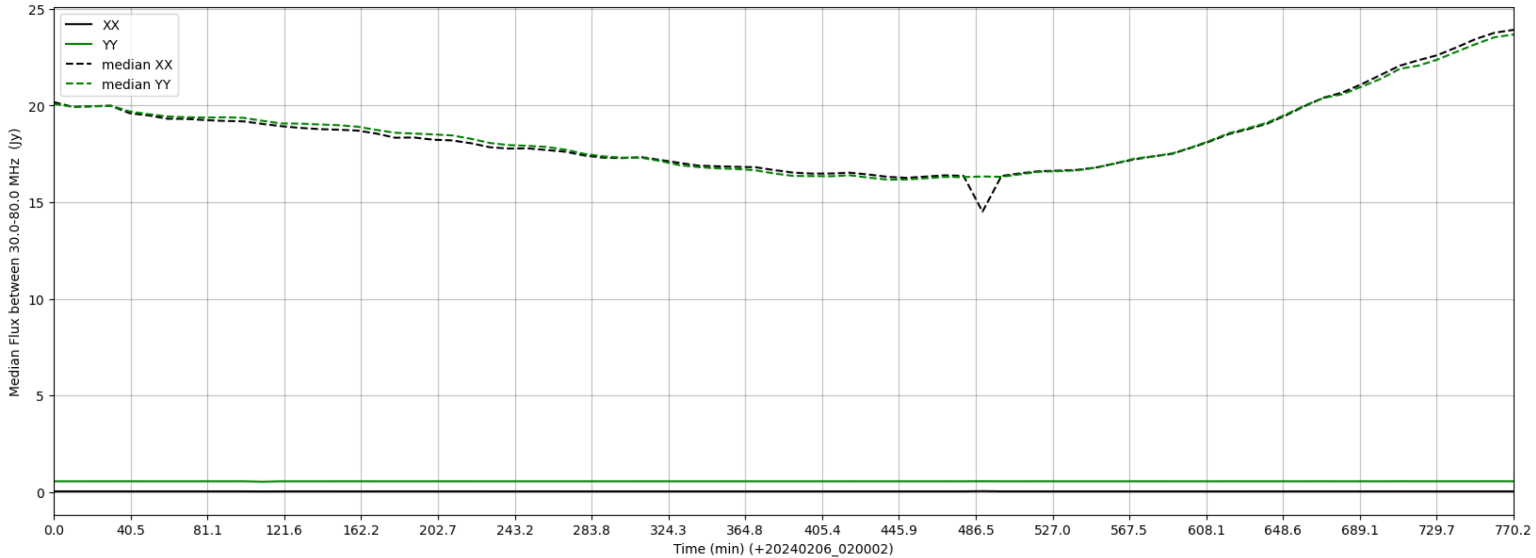
LWA302 - Correlator# 092 - XX FLAGS:LowFlux - YY FLAGS:LowFlux
