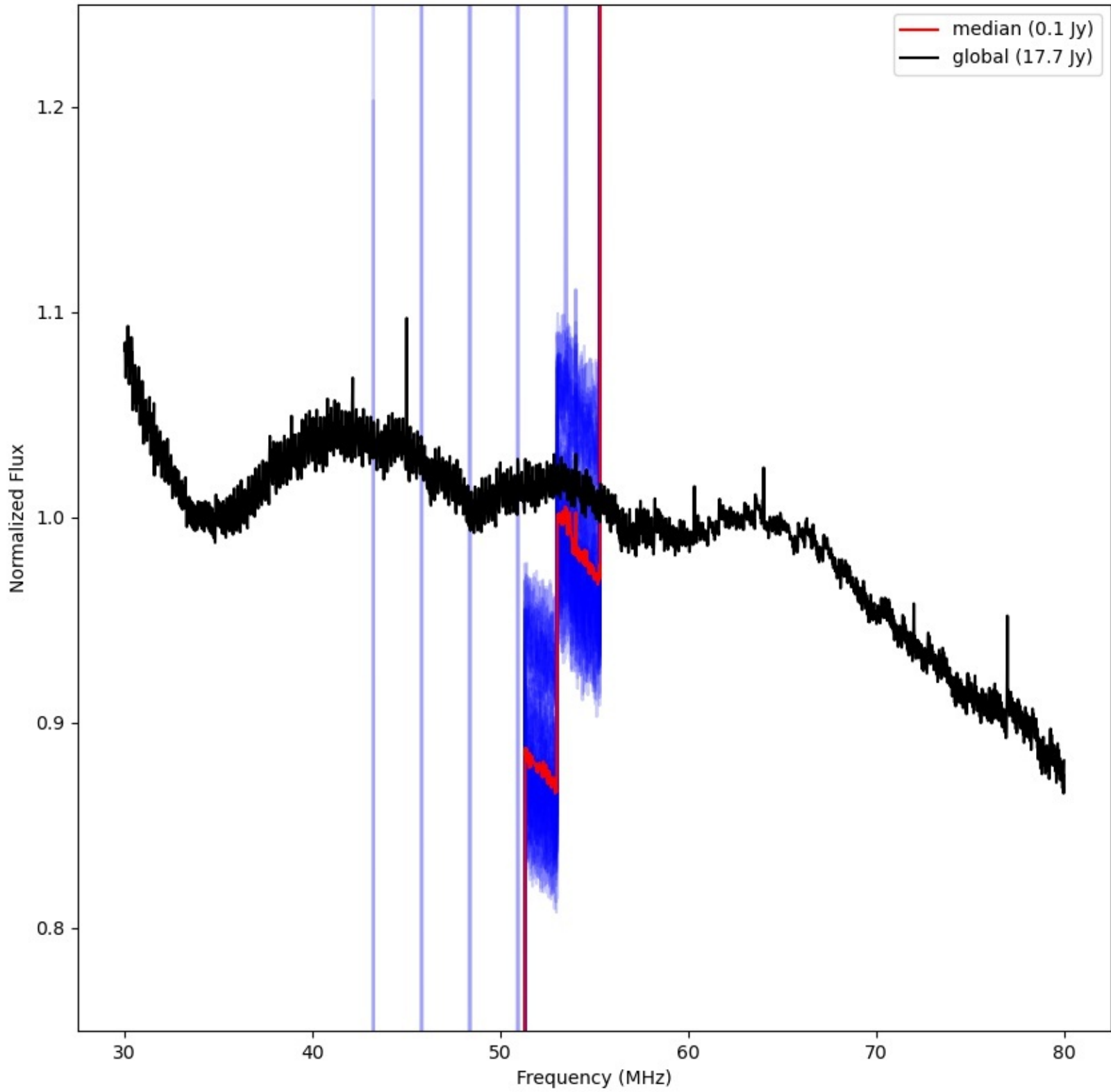
LWA299 - Correlator# 191 - XX - FLAGS:LowFlux
