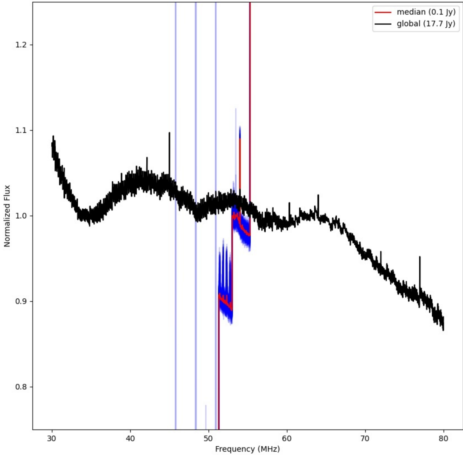
LWA306 - Correlator# 053 - XX - FLAGS:LowFlux
