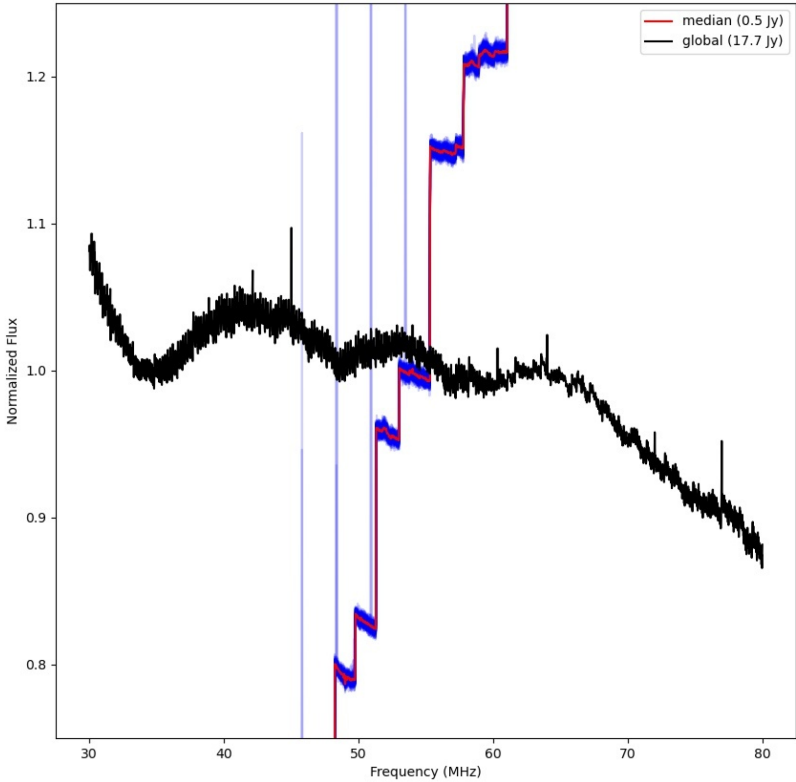
LWA363 - Correlator# 094 - XX - FLAGS:LowFlux
