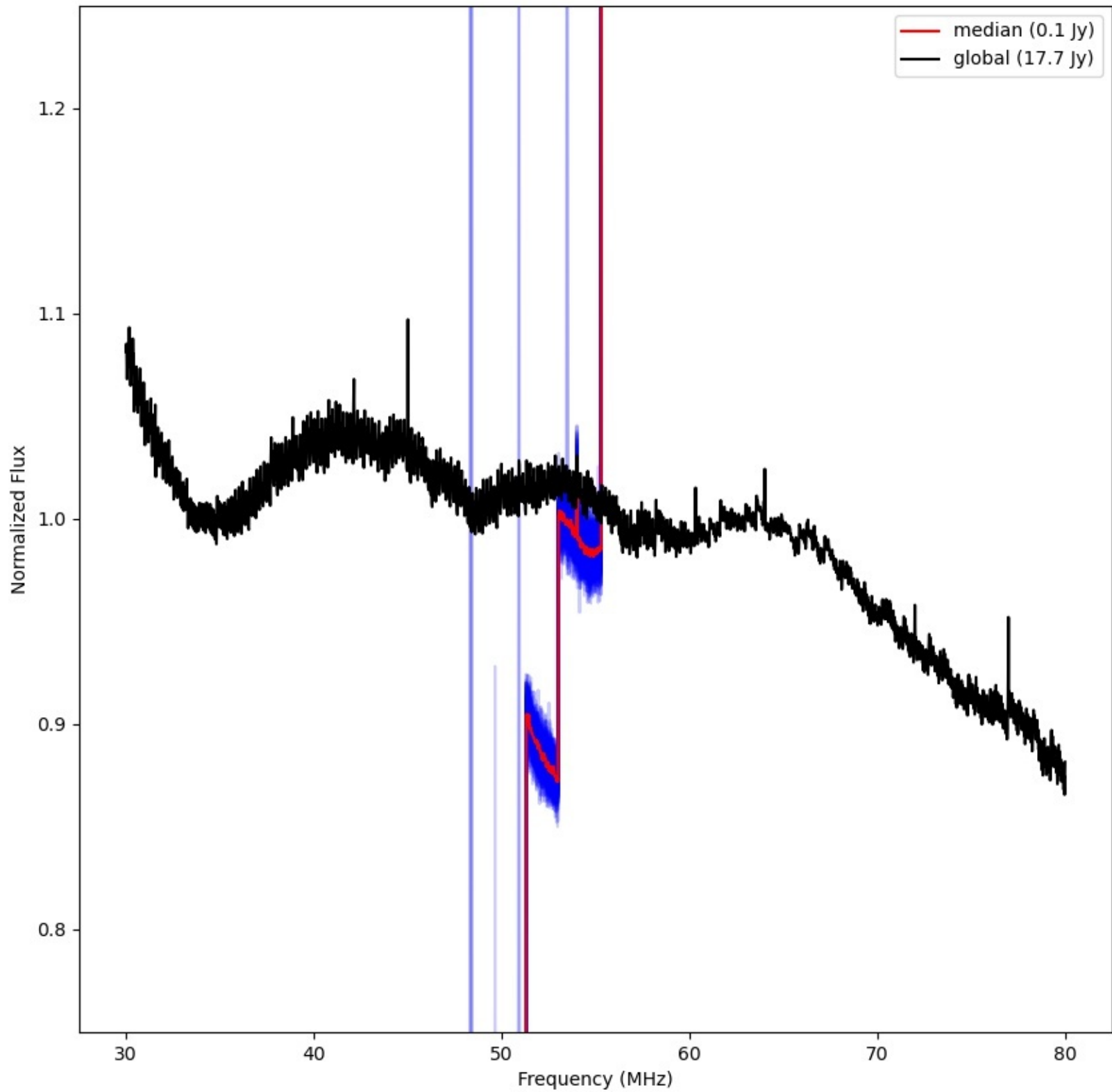
LWA364 - Correlator# 127 - XX - FLAGS:LowFlux
