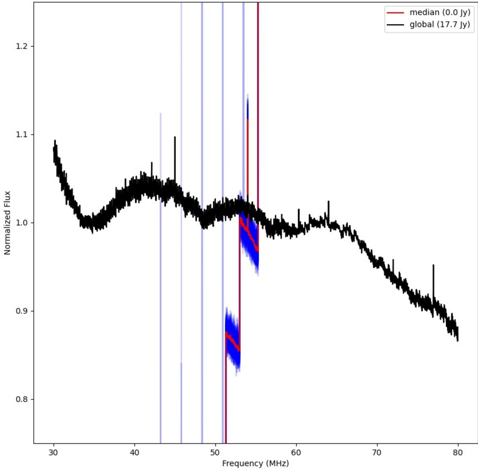
LWA265 - Correlator# 036 - XX - FLAGS:LowFlux
