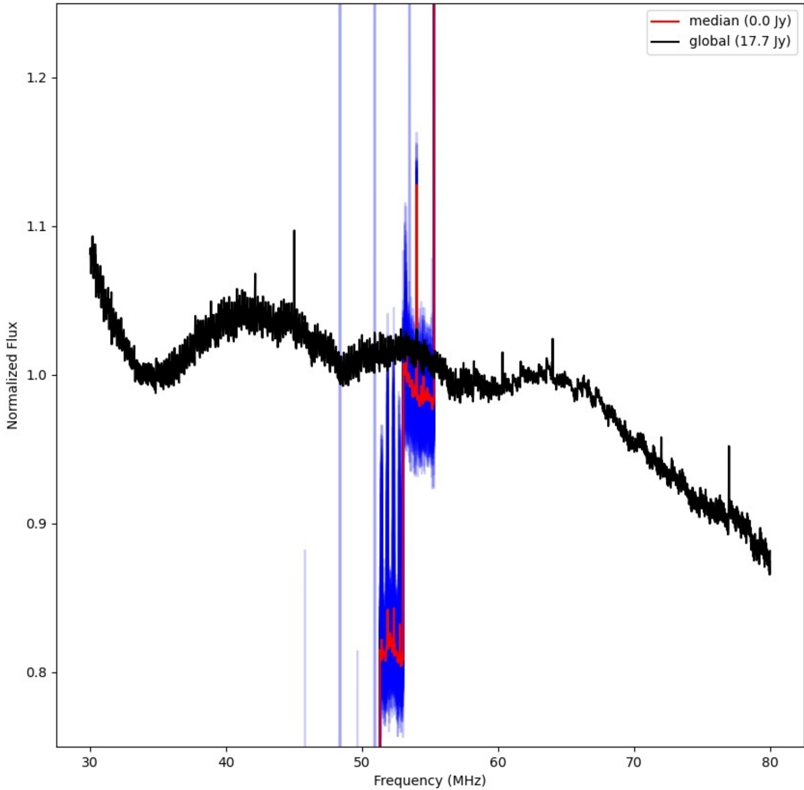
LWA303 - Correlator# 051 - XX - FLAGS:LowFlux
