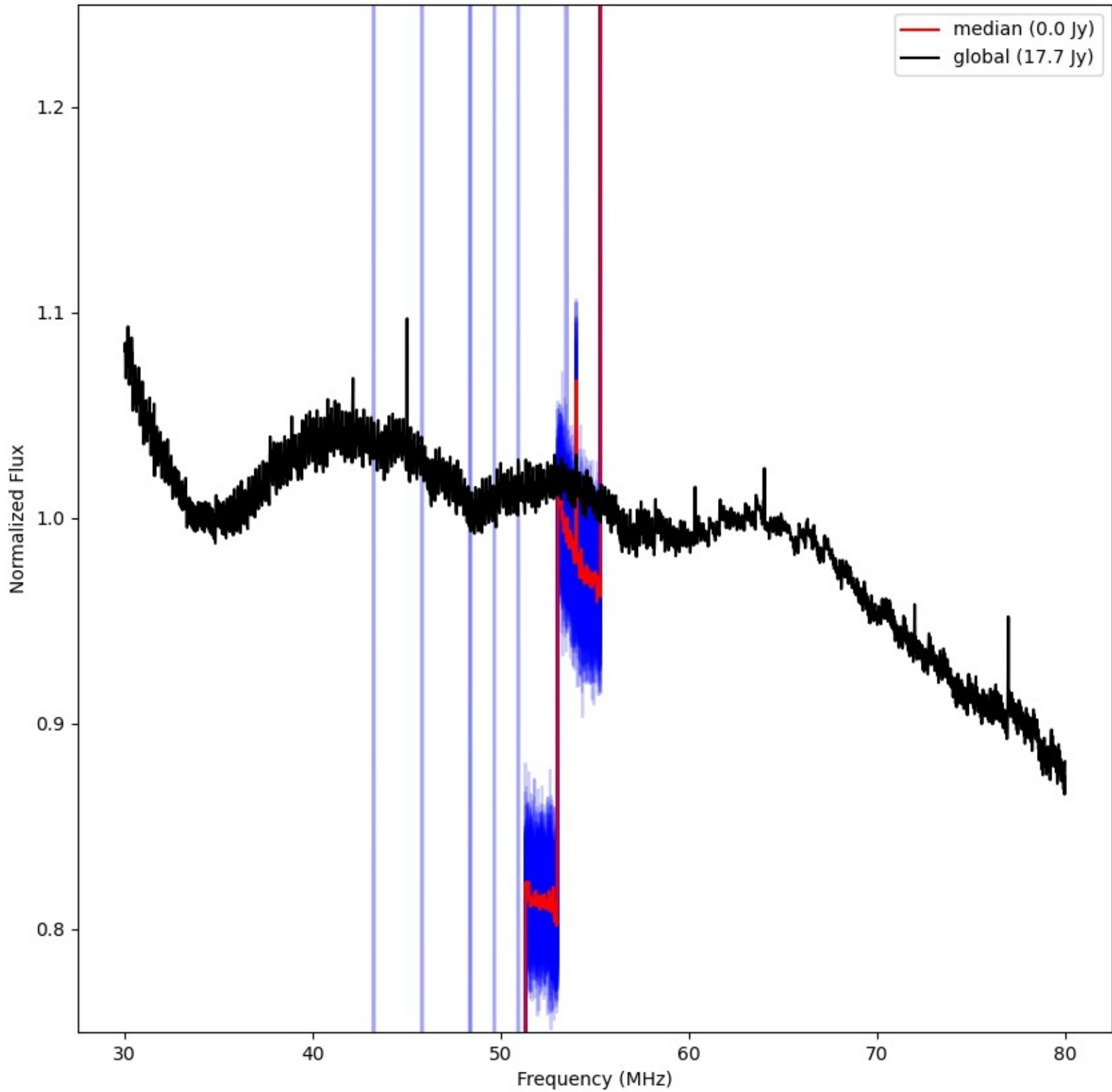
LWA304 - Correlator# 351 - XX - FLAGS:LowFlux
