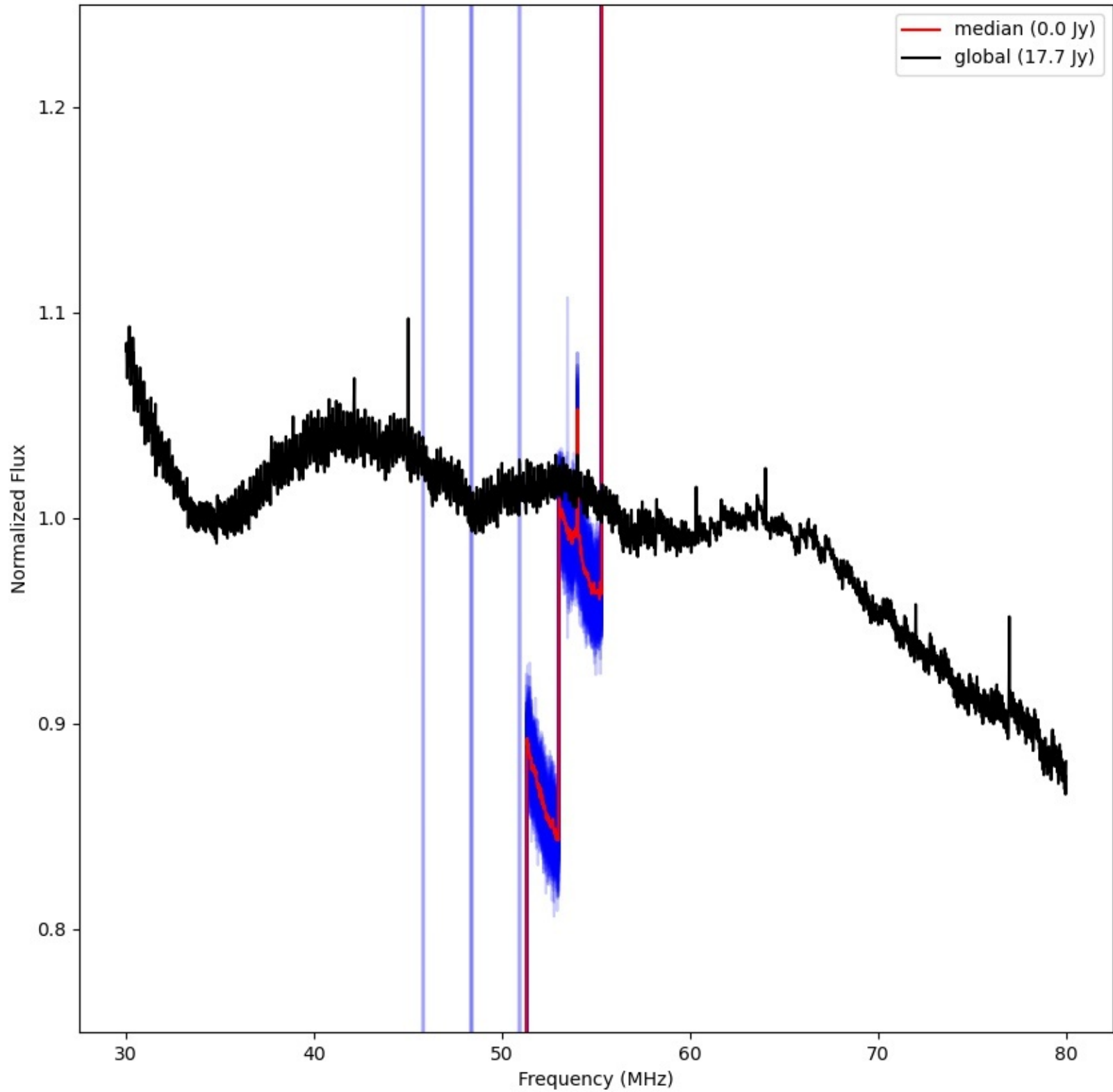
LWA359 - Correlator# 254 - XX - FLAGS:LowFlux
