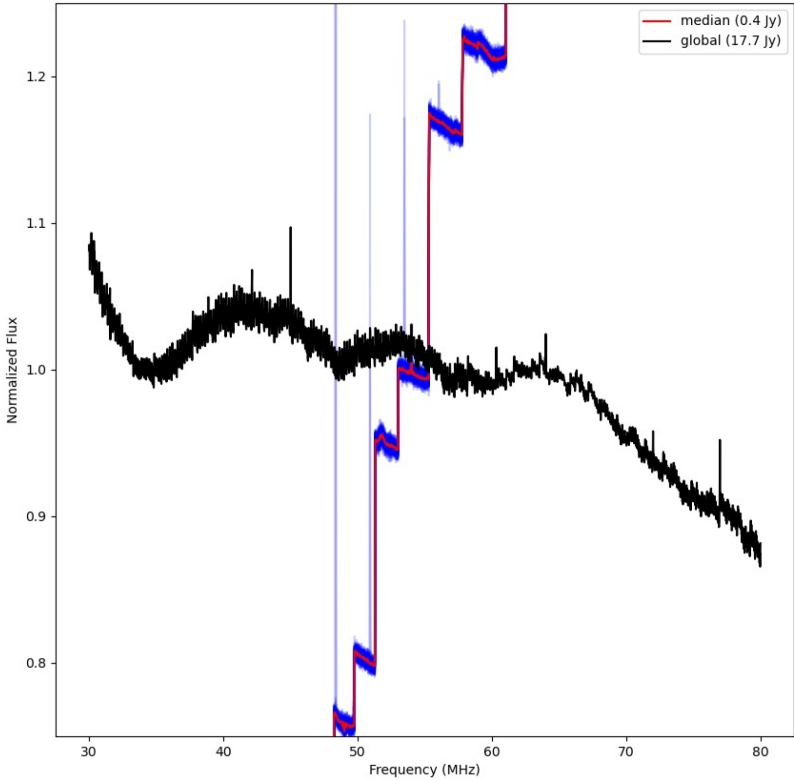
LWA362 - Correlator# 030 - XX - FLAGS:LowFlux
