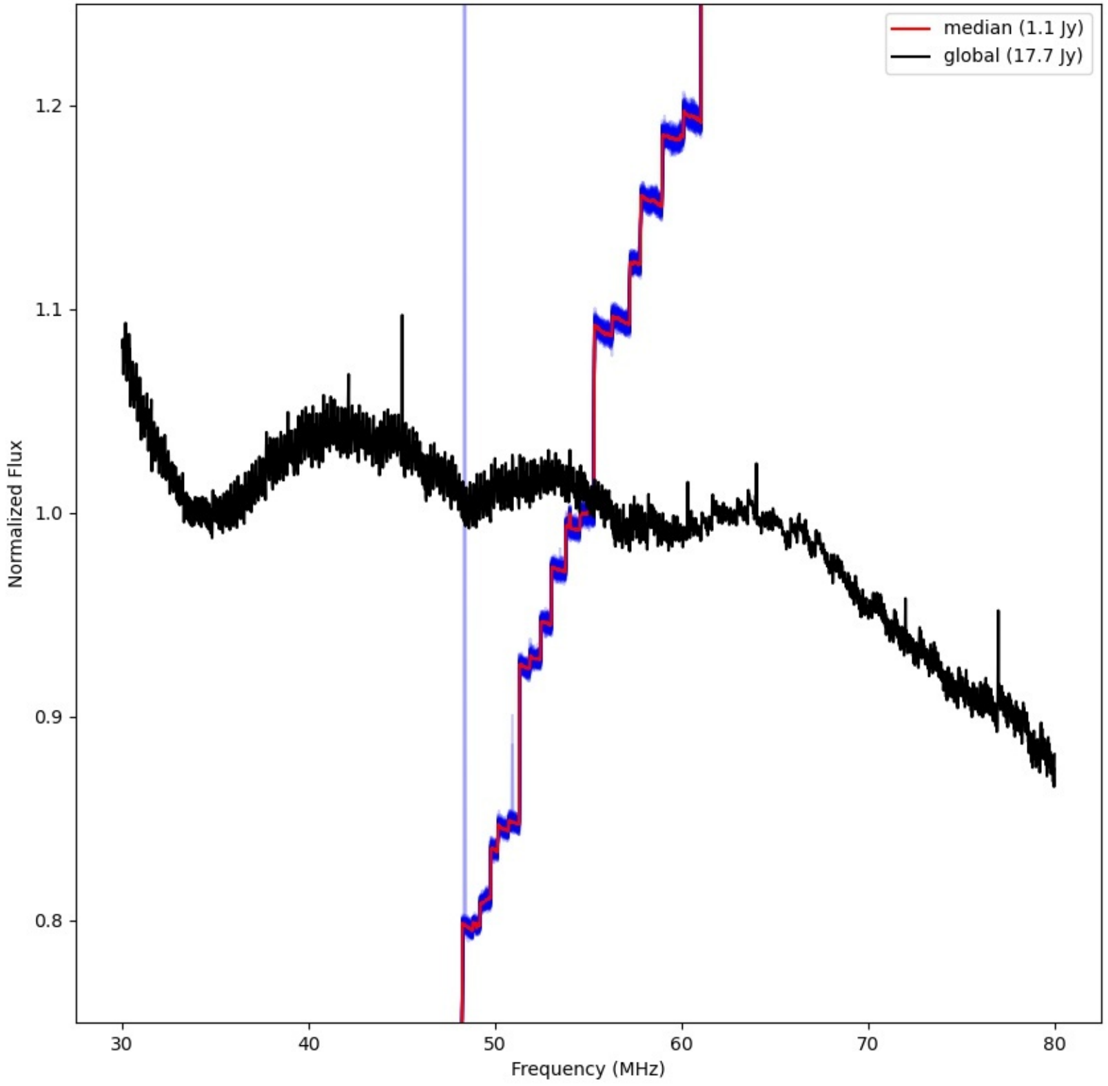
LWA317 - Correlator# 052 - XX - FLAGS:LowFlux
