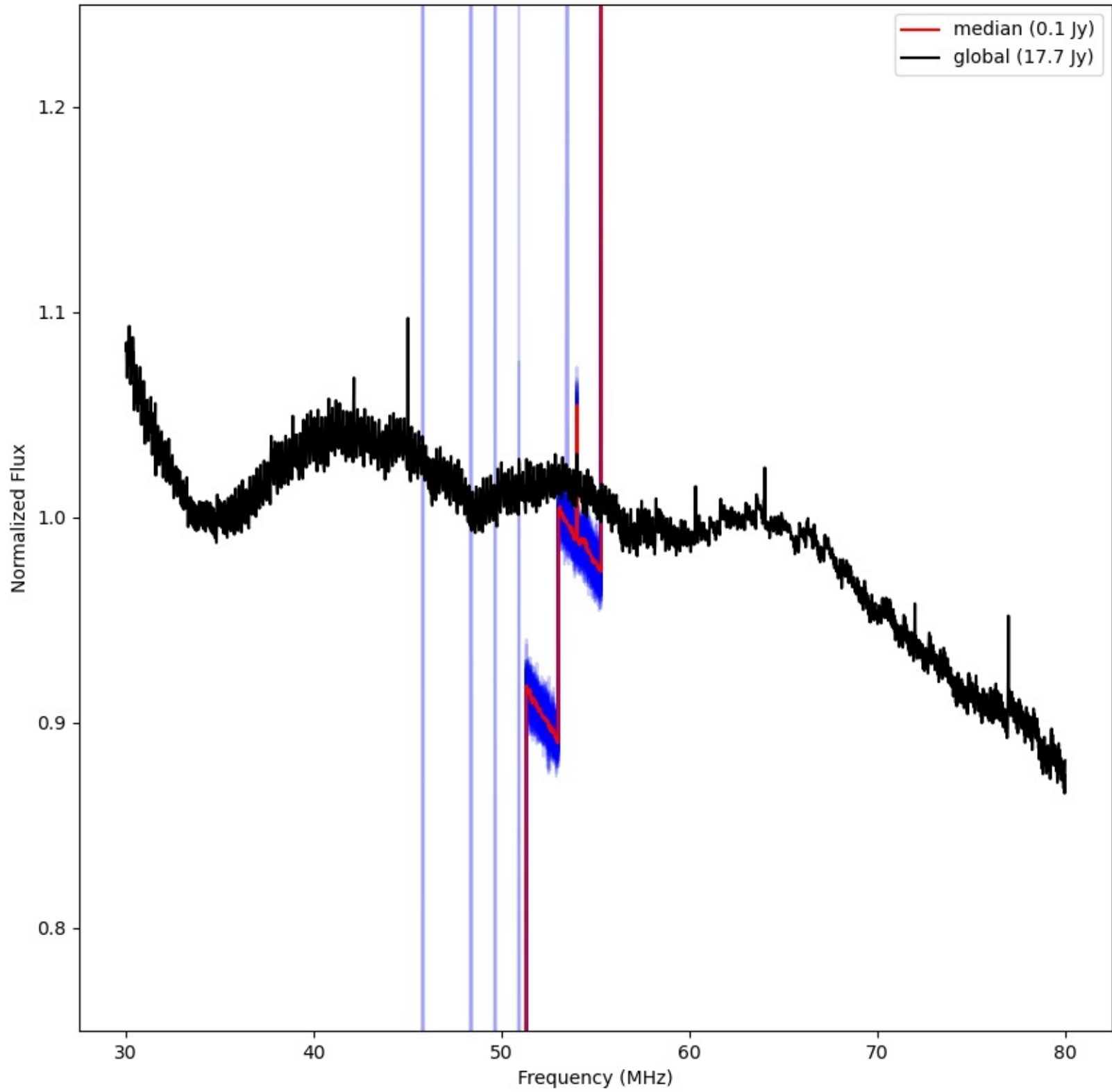
LWA361 - Correlator# 158 - XX - FLAGS:LowFlux
