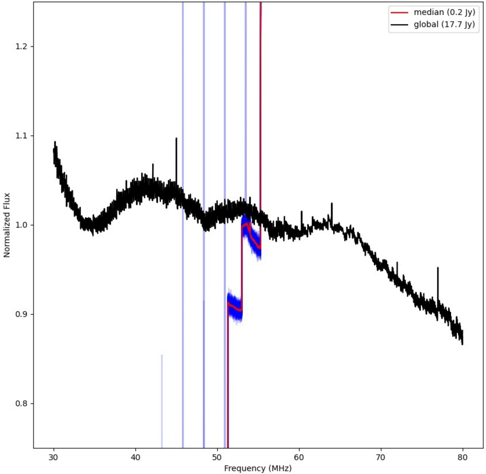
LWA279 - Correlator# 220 - XX - FLAGS:LowFlux
