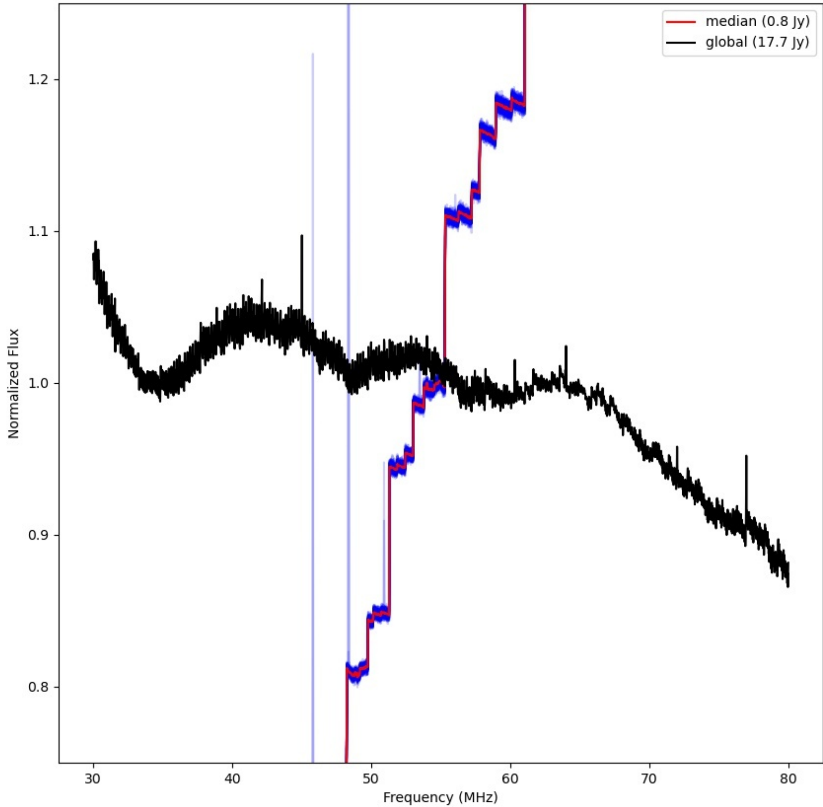
LWA318 - Correlator# 055 - XX - FLAGS:LowFlux
