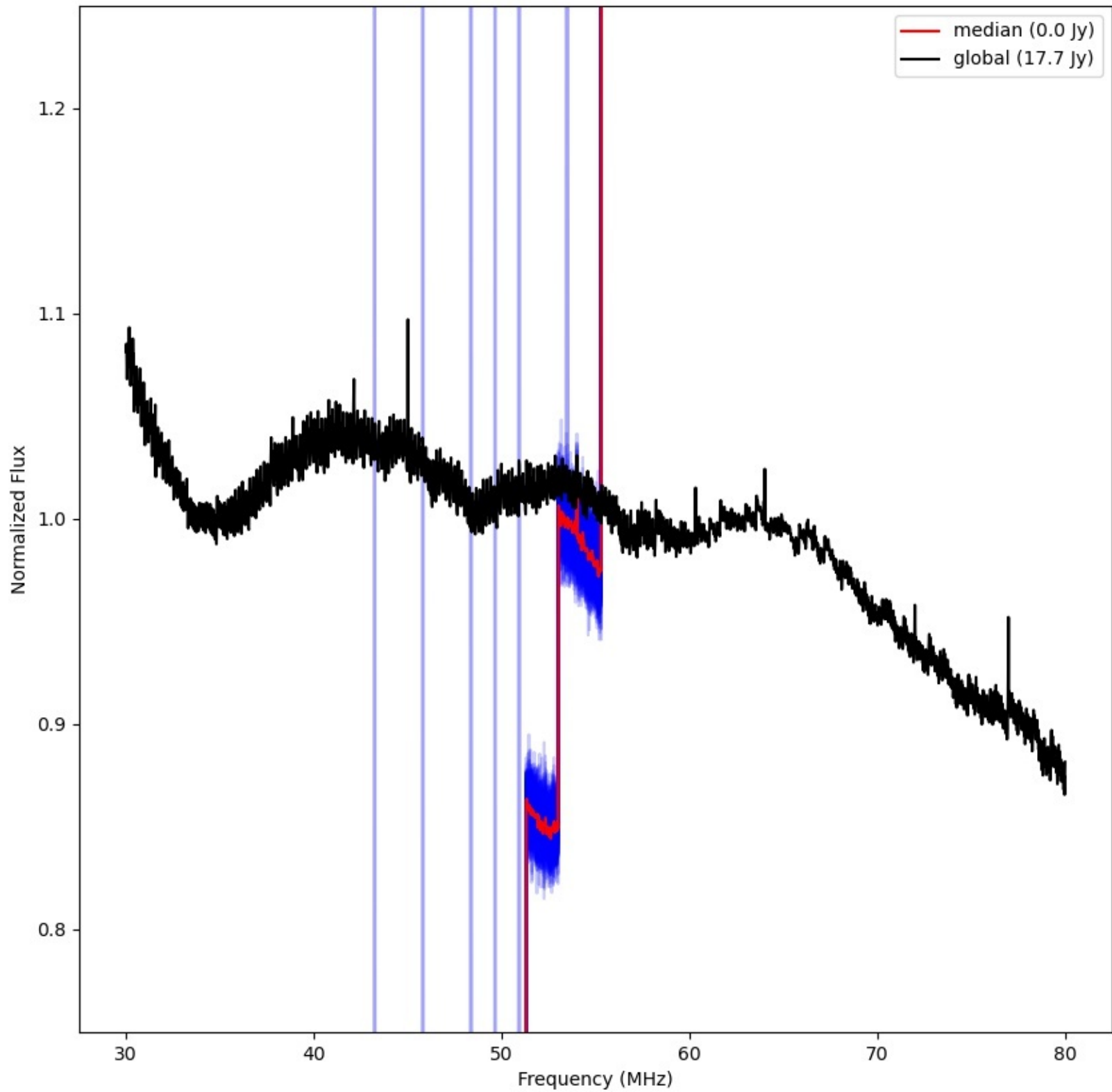
LWA274 - Correlator# 091 - XX - FLAGS:LowFlux
