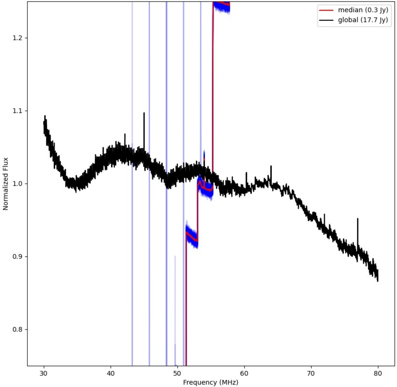
LWA329 - Correlator# 287 - XX - FLAGS:LowFlux
