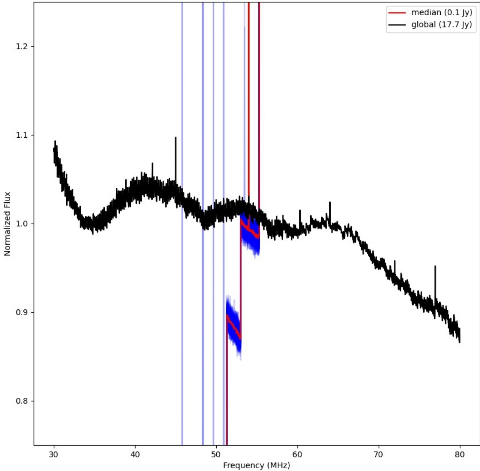
LWA262 - Correlator# 123 - XX - FLAGS:LowFlux
