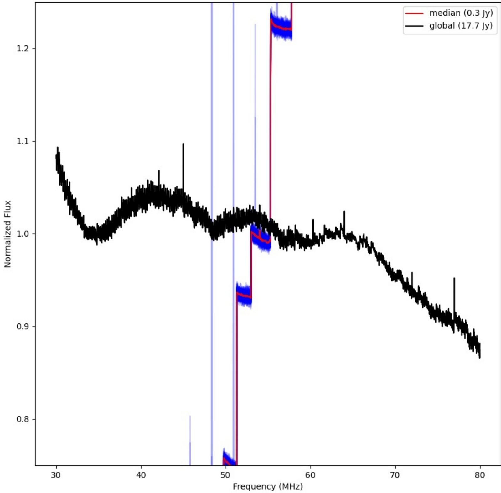
LWA300 - Correlator# 348 - XX - FLAGS:LowFlux
