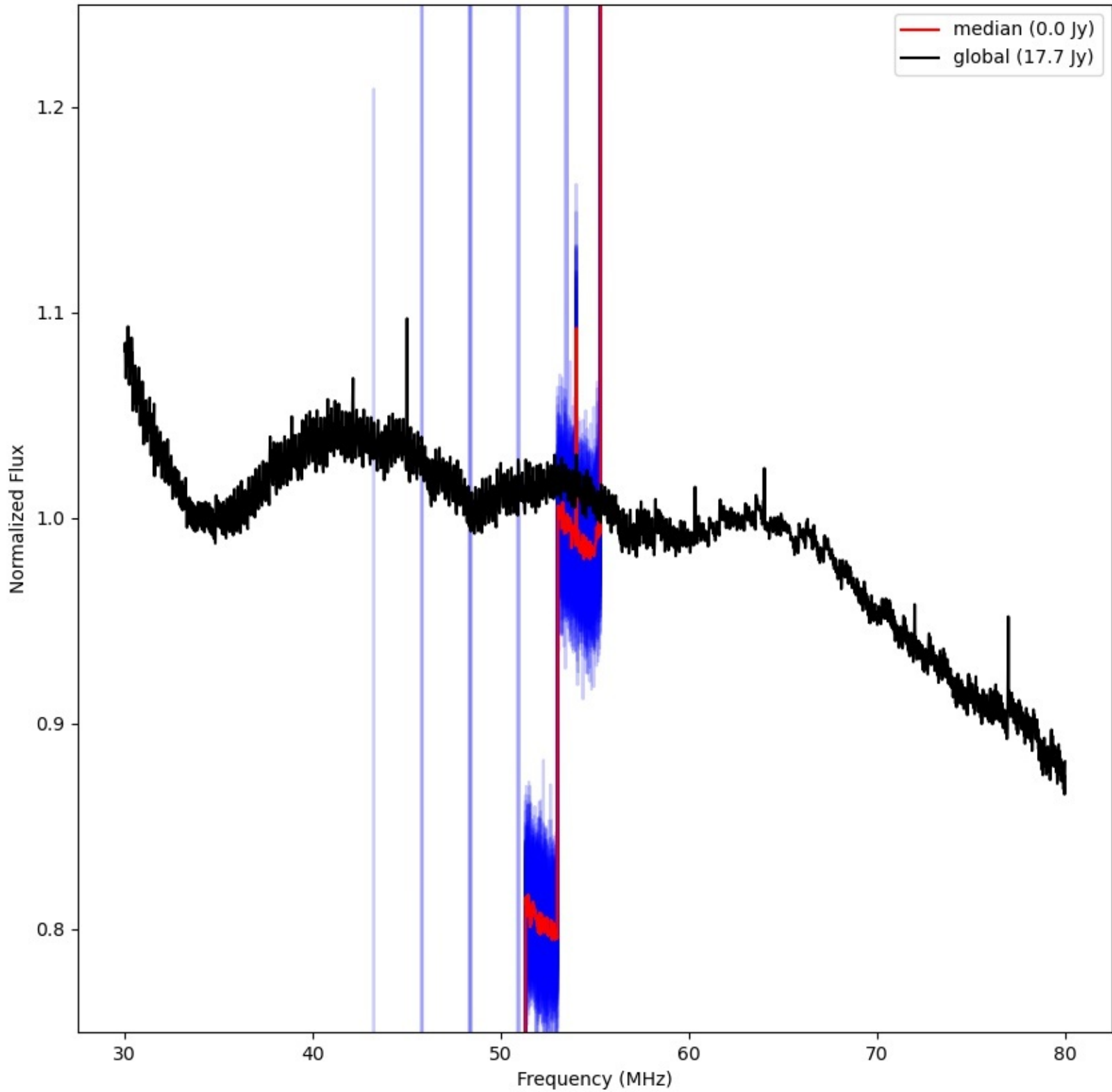
LWA346 - Correlator# 316 - XX - FLAGS:LowFlux
