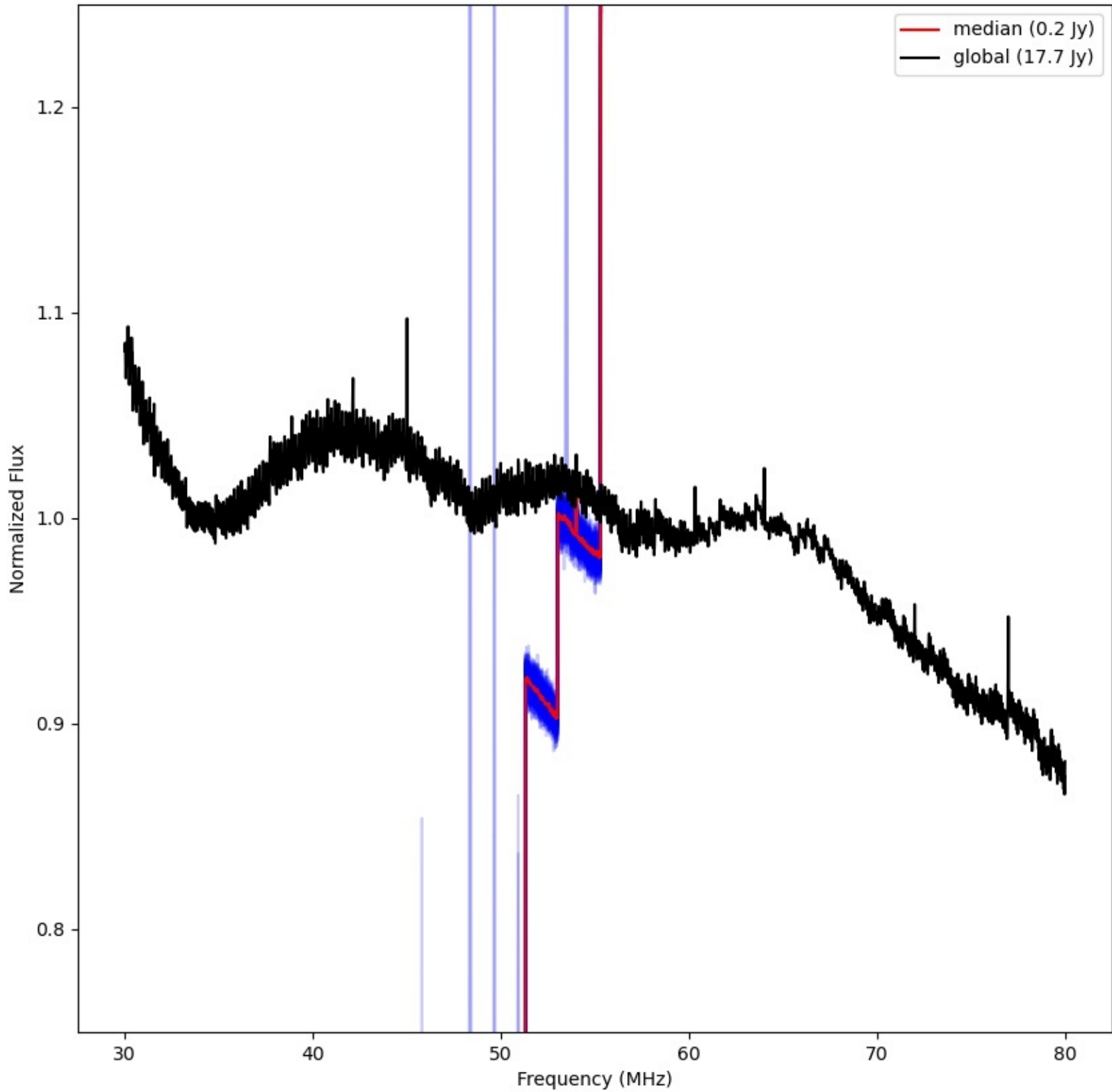
LWA358 - Correlator# 159 - XX - FLAGS:LowFlux
