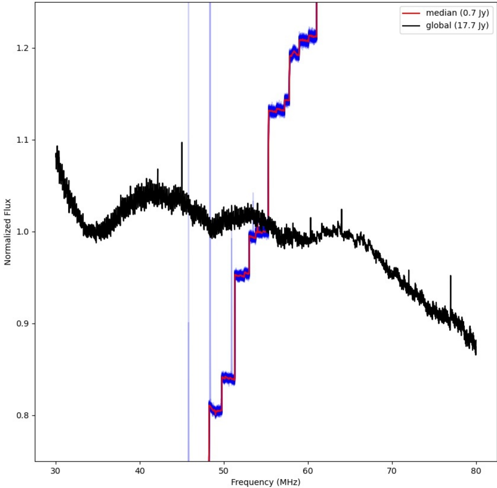
LWA356 - Correlator# 318 - XX - FLAGS:LowFlux
