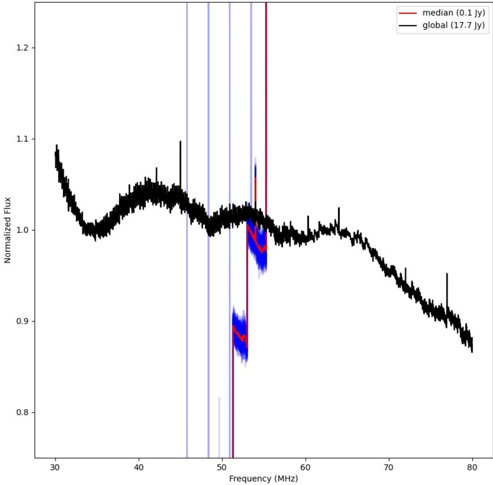
LWA360 - Correlator# 062 - XX - FLAGS:LowFlux
