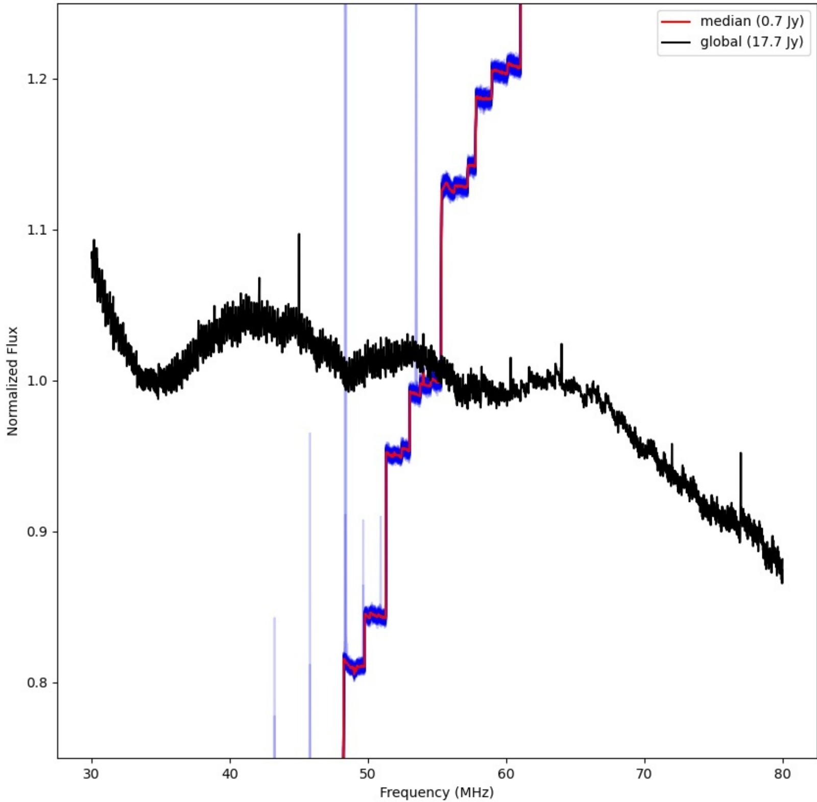
LWA357 - Correlator# 286 - XX - FLAGS:LowFlux
