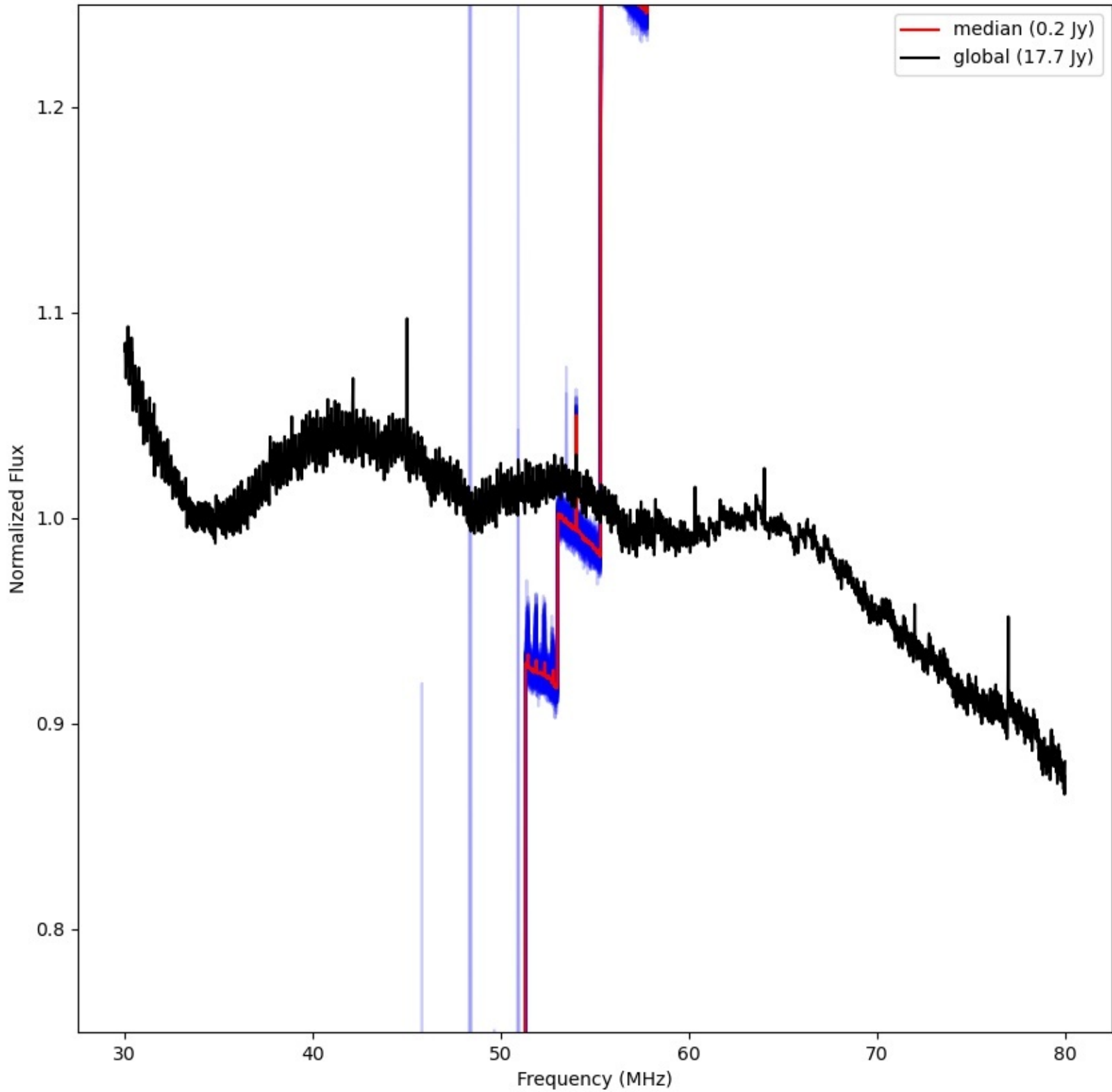
LWA305 - Correlator# 050 - XX - FLAGS:LowFlux
