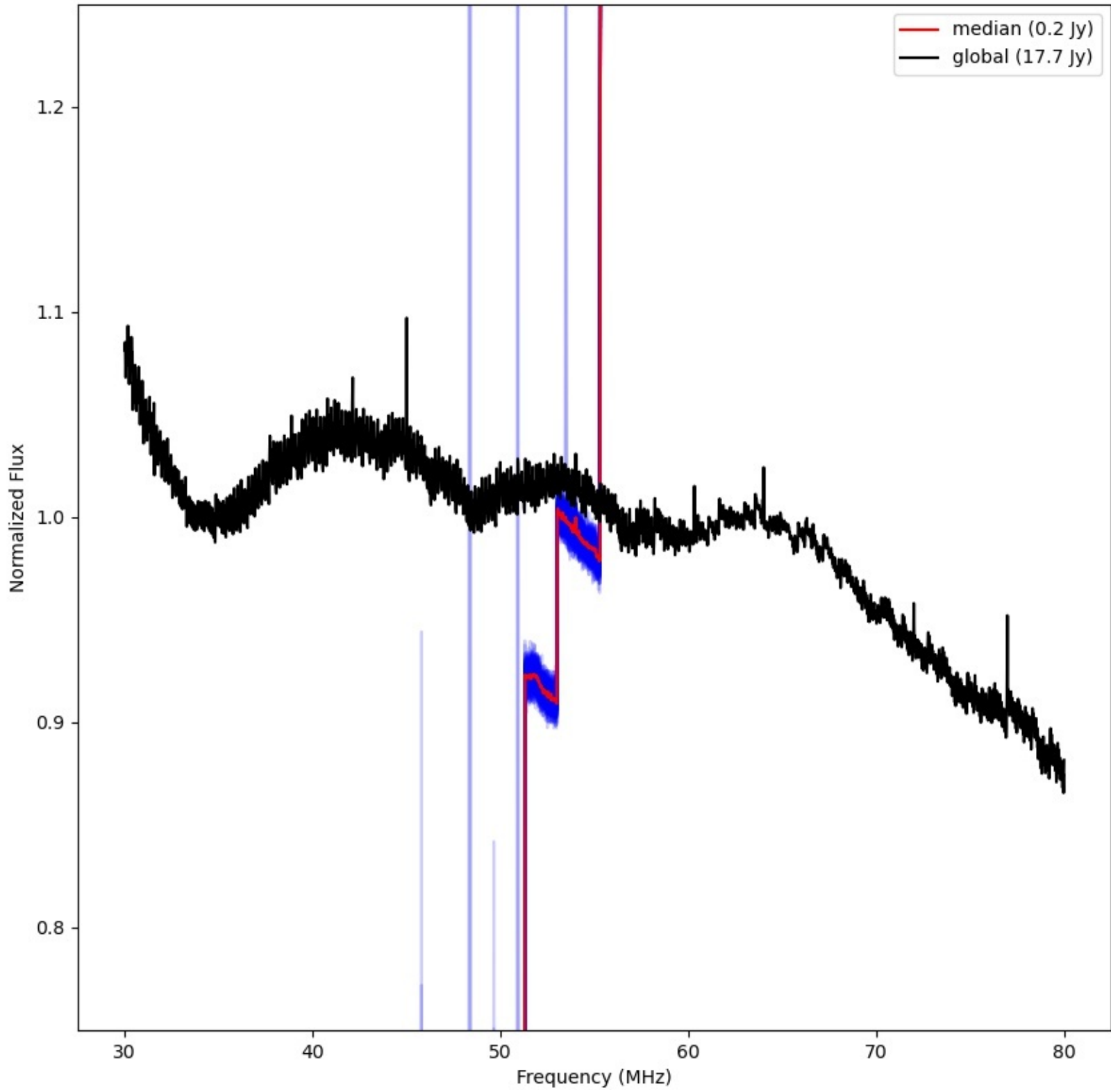
LWA294 - Correlator# 188 - XX - FLAGS:LowFlux
