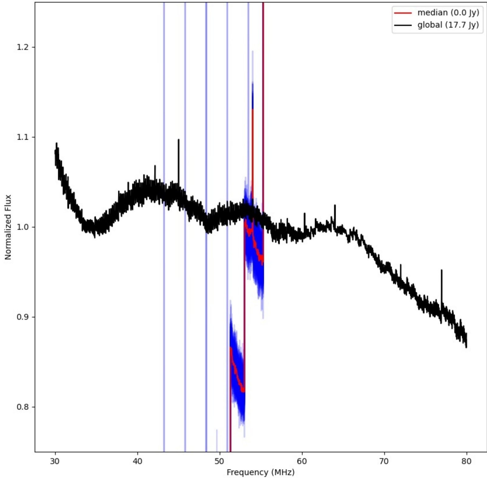
LWA345 - Correlator# 252 - XX - FLAGS:LowFlux
