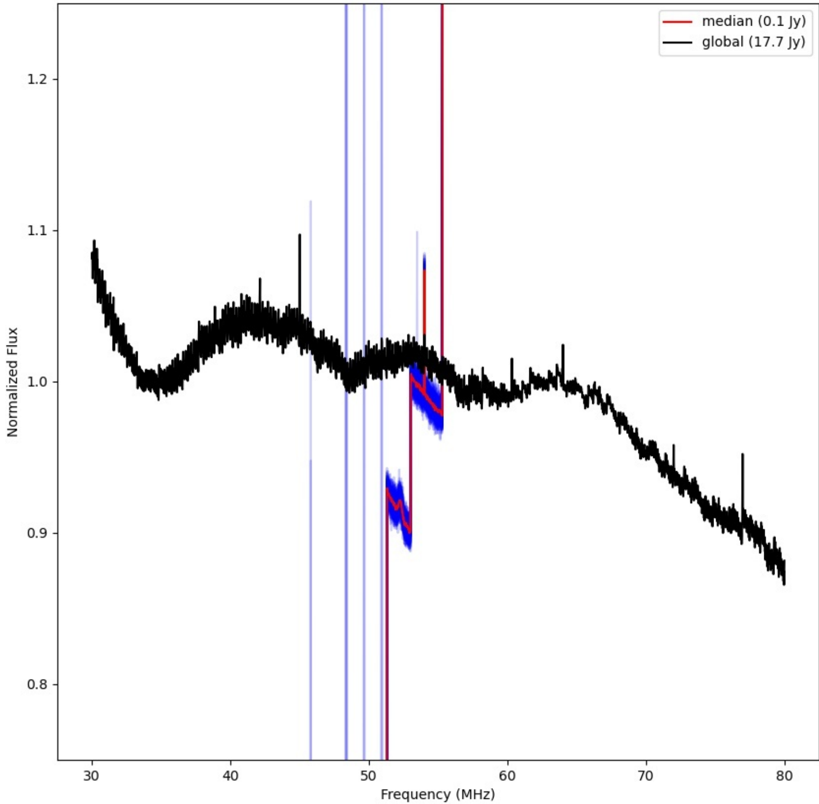
LWA324 - Correlator# 122 - XX - FLAGS:LowFlux
