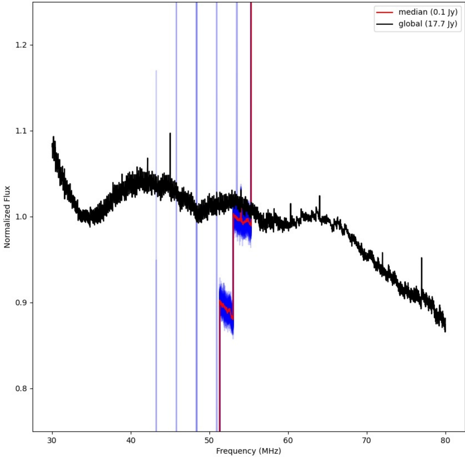
LWA293 - Correlator# 284 - XX - FLAGS:LowFlux
