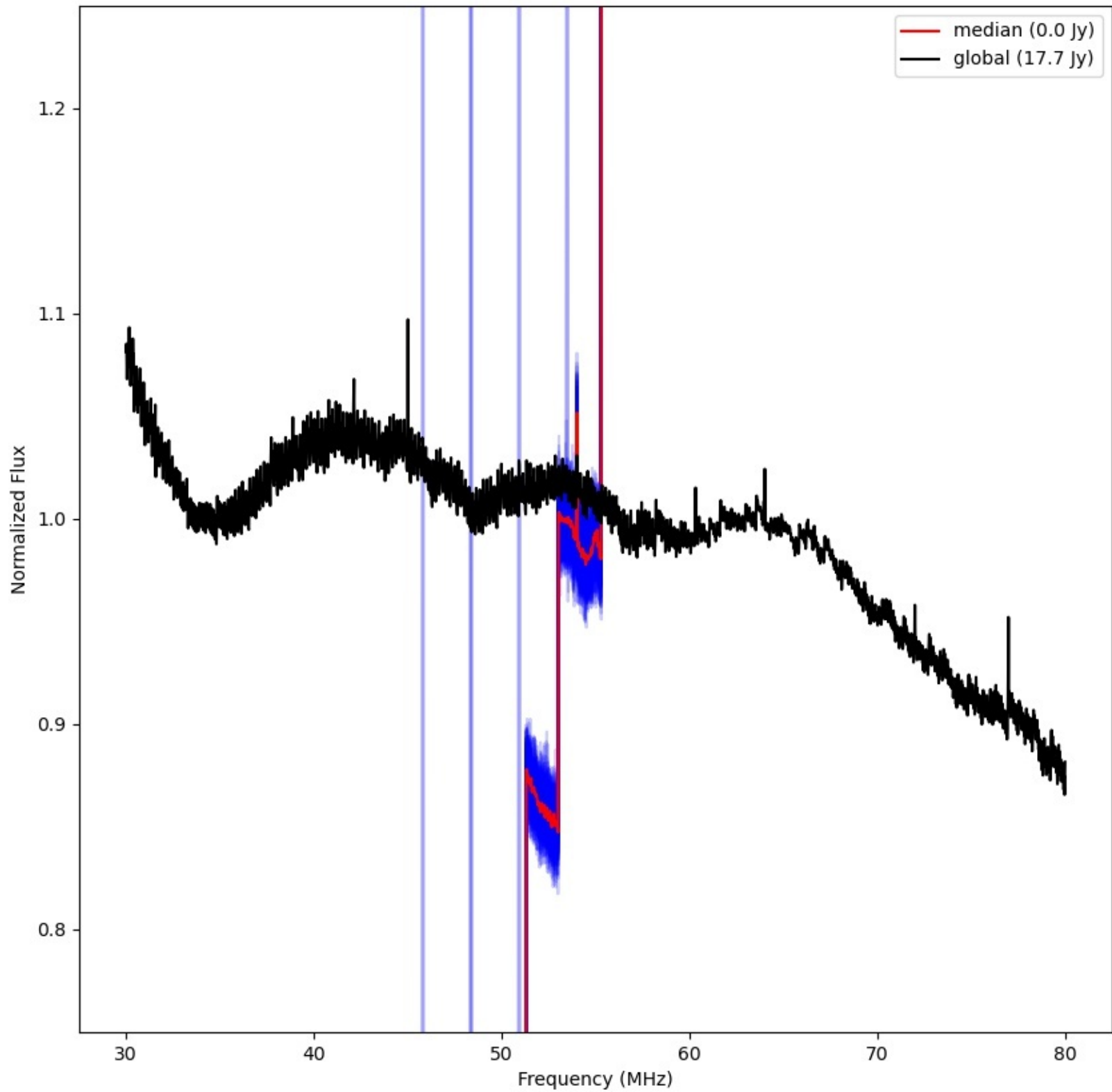
LWA323 - Correlator# 095 - XX - FLAGS:LowFlux
