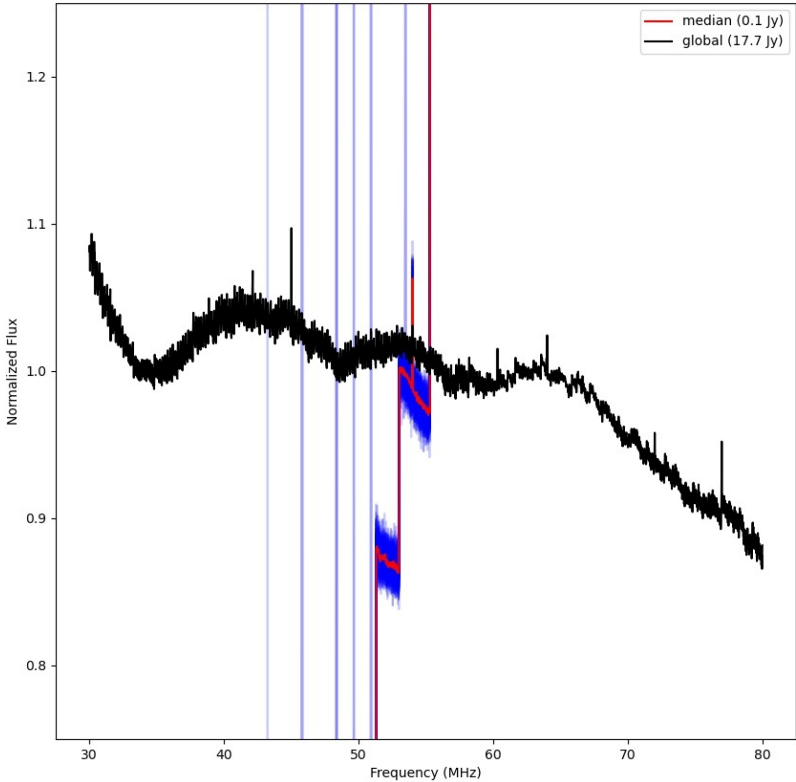
LWA355 - Correlator# 222 - XX - FLAGS:LowFlux
