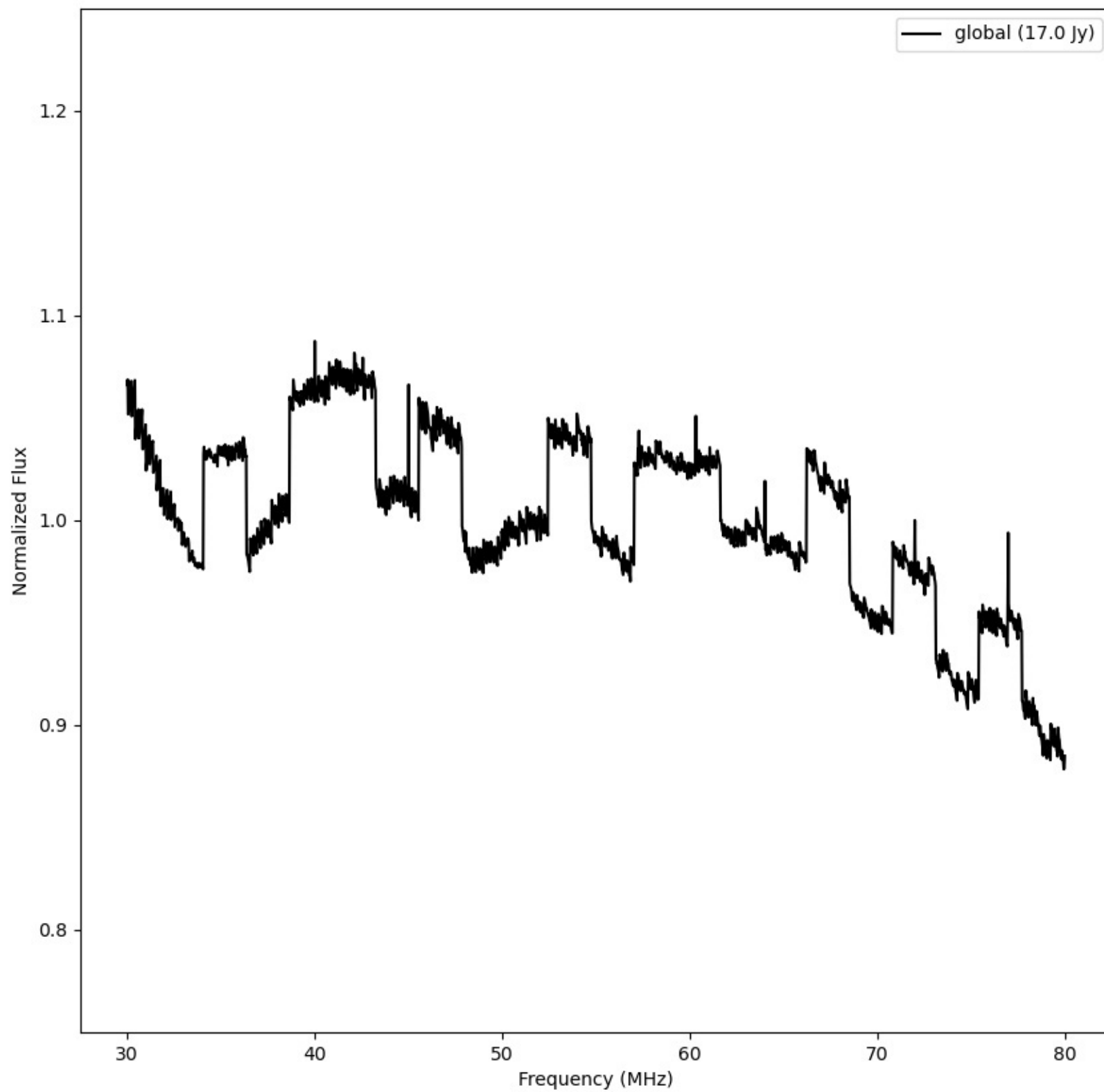
LWA162 - Correlator# 265 - XX - FLAGS:LowFlux
