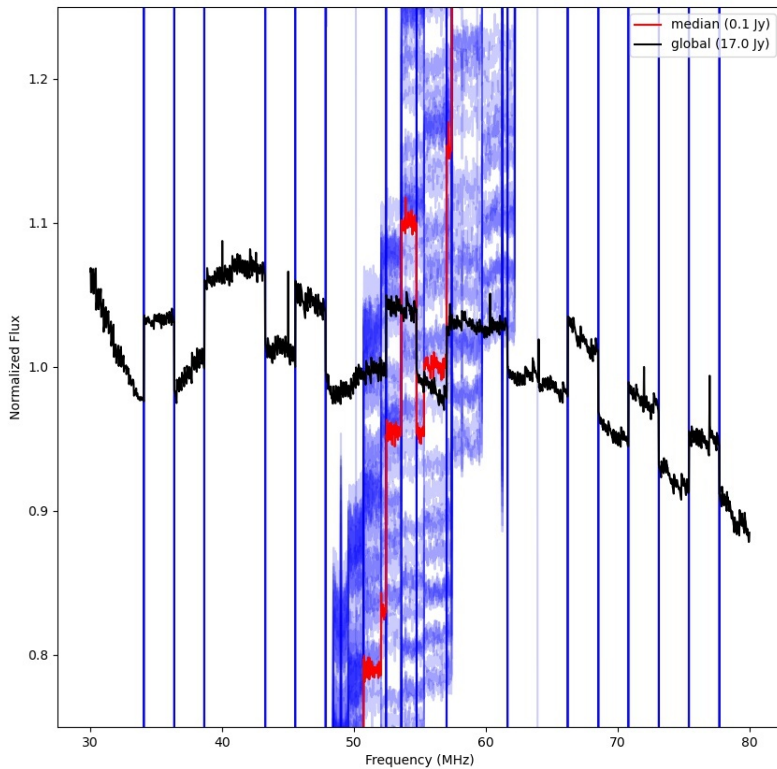
LWA136 - Correlator# 259 - XX - FLAGS:LowFlux
