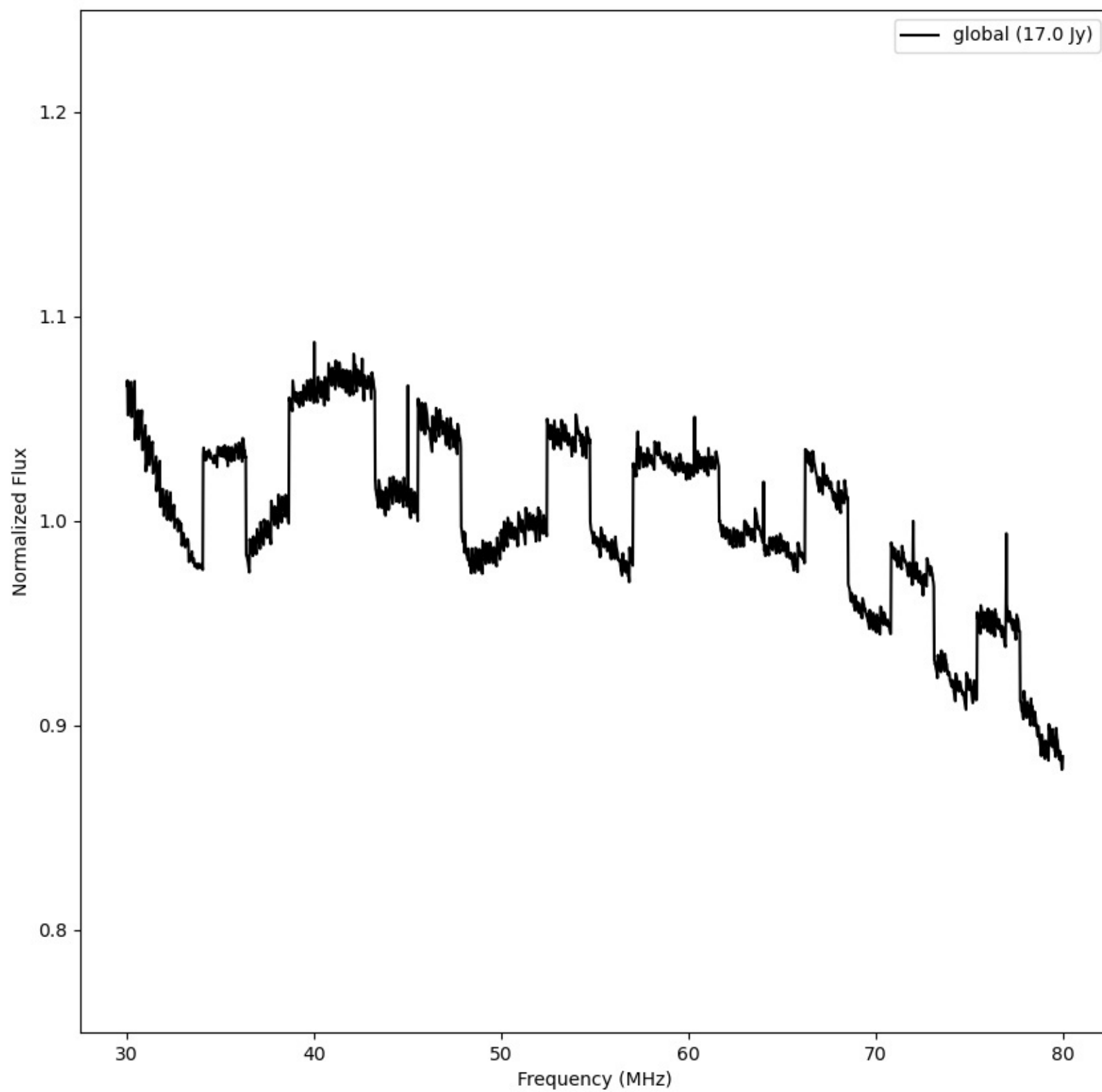
LWA167 - Correlator# 268 - XX - FLAGS:LowFlux
