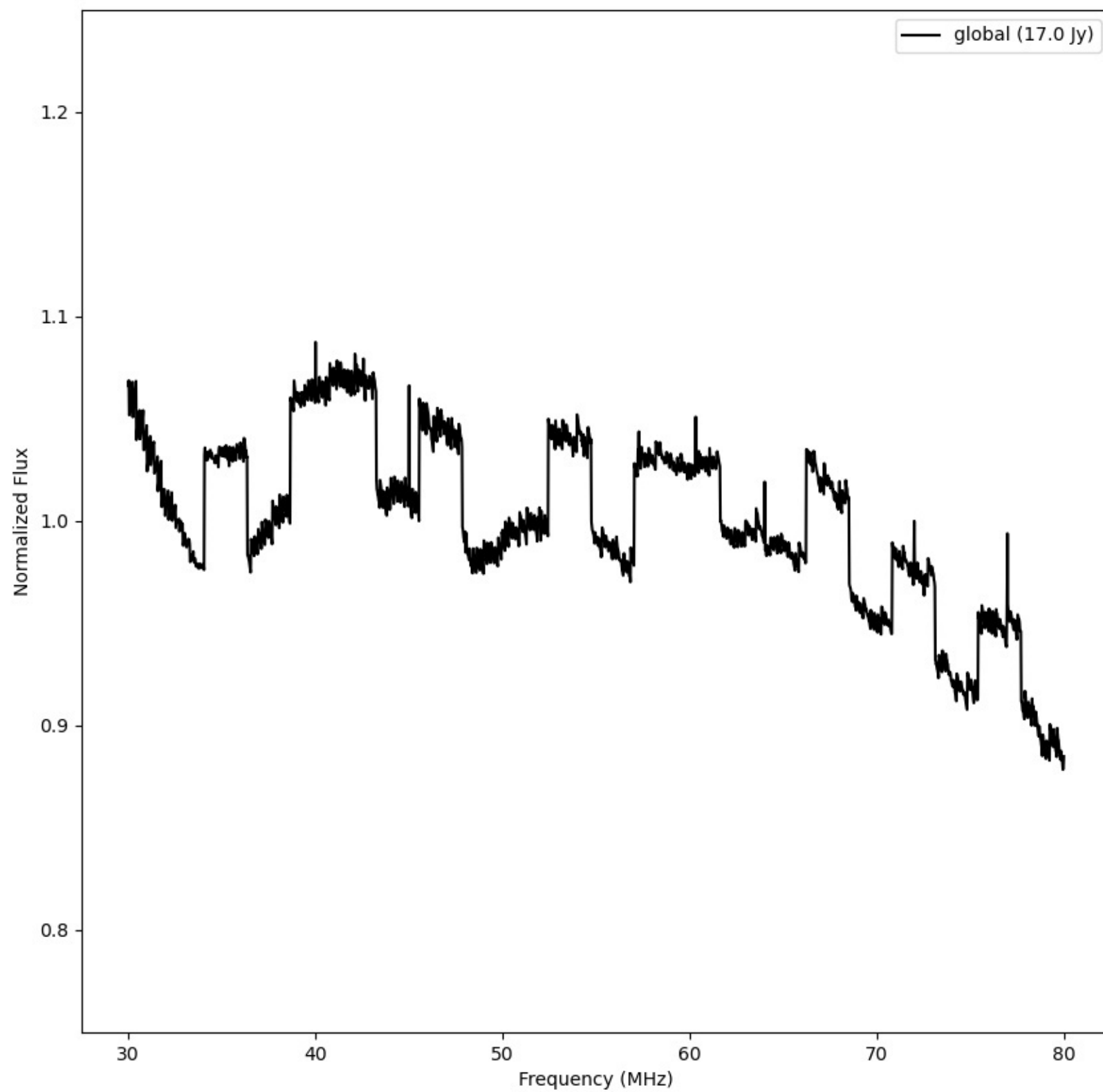
LWA198 - Correlator# 271 - XX - FLAGS:LowFlux
