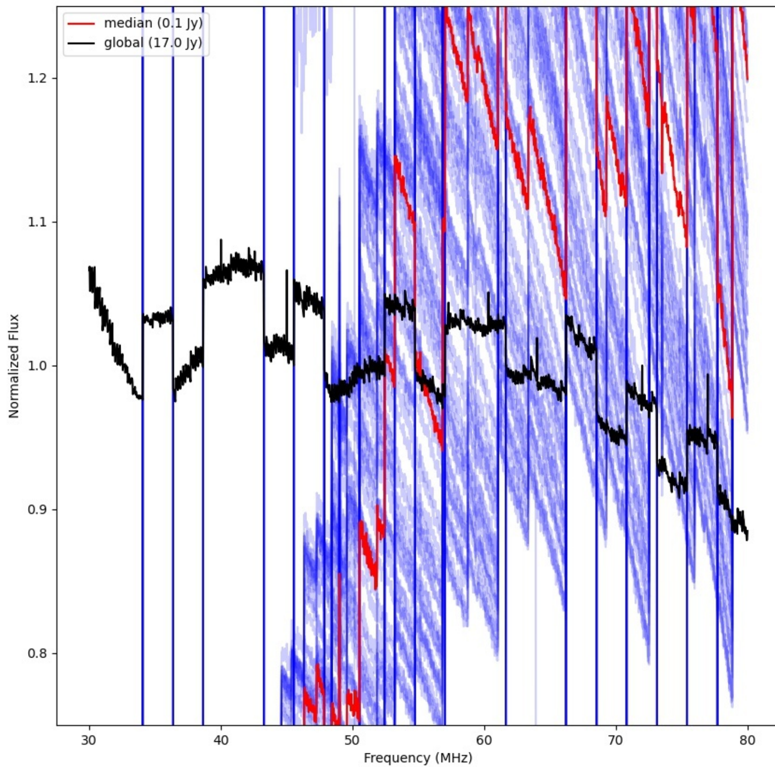
LWA137 - Correlator# 258 - XX - FLAGS:LowFlux
