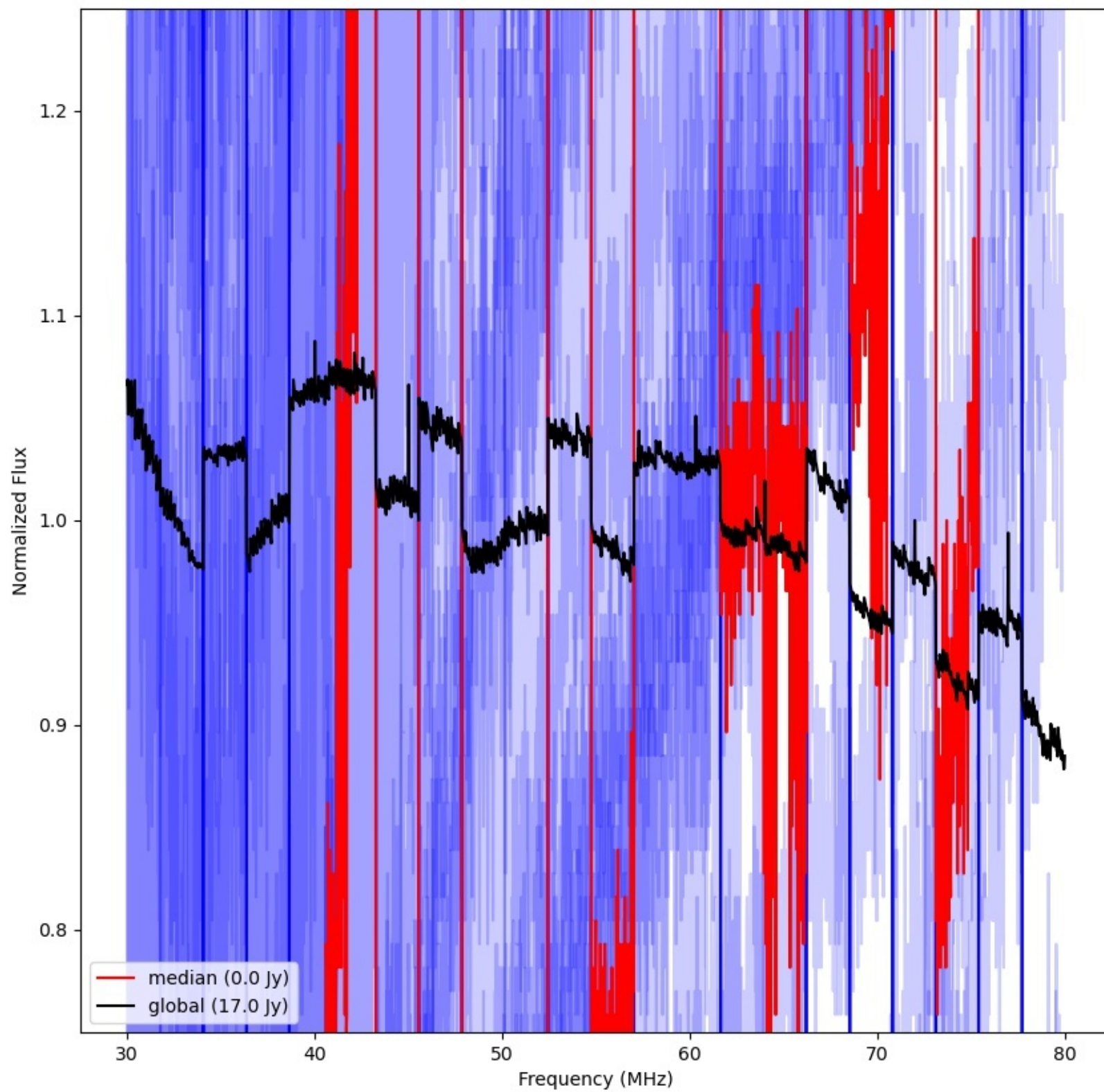
LWA165 - Correlator# 266 - XX - FLAGS:LowFlux
