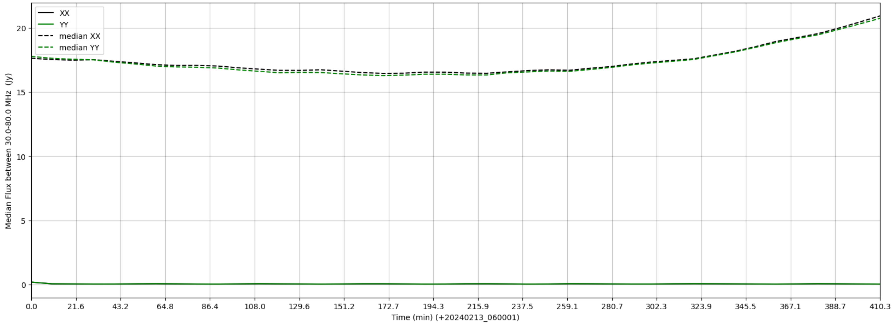
LWA136 - Correlator# 259 - XX FLAGS:LowFlux - YY FLAGS:LowFlux
