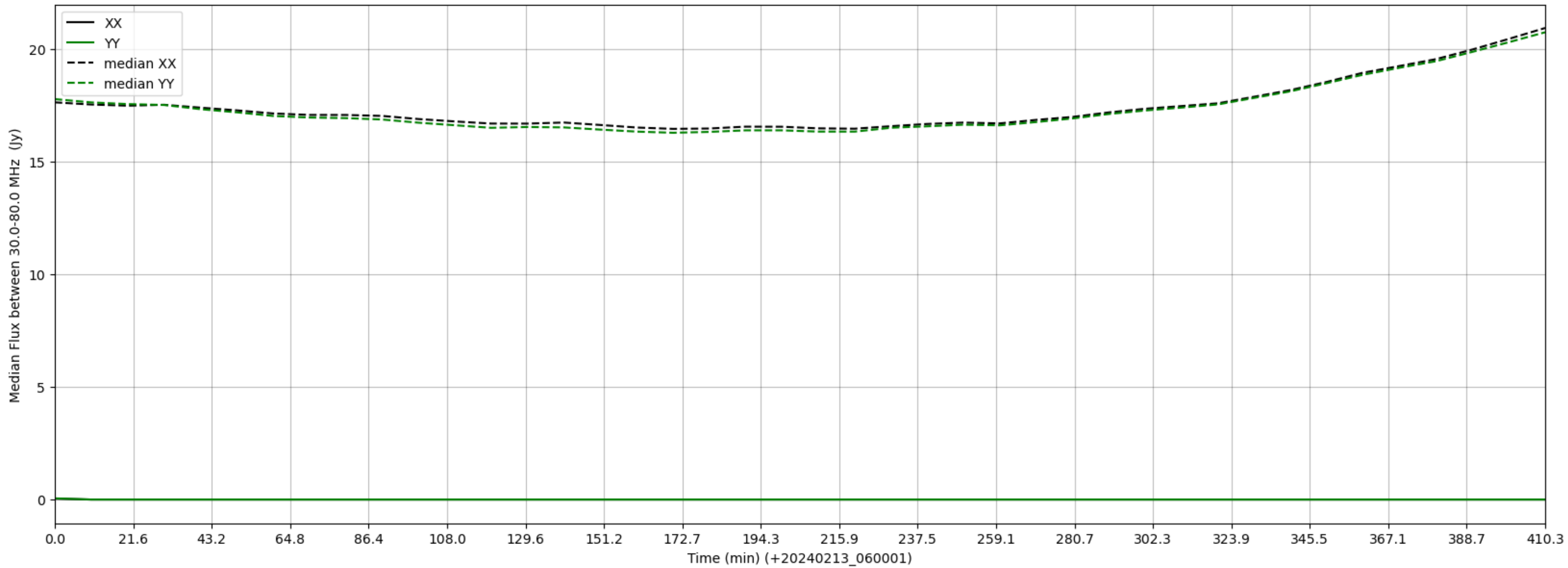
LWA162 - Correlator# 265 - XX FLAGS:LowFlux - YY FLAGS:LowFlux
