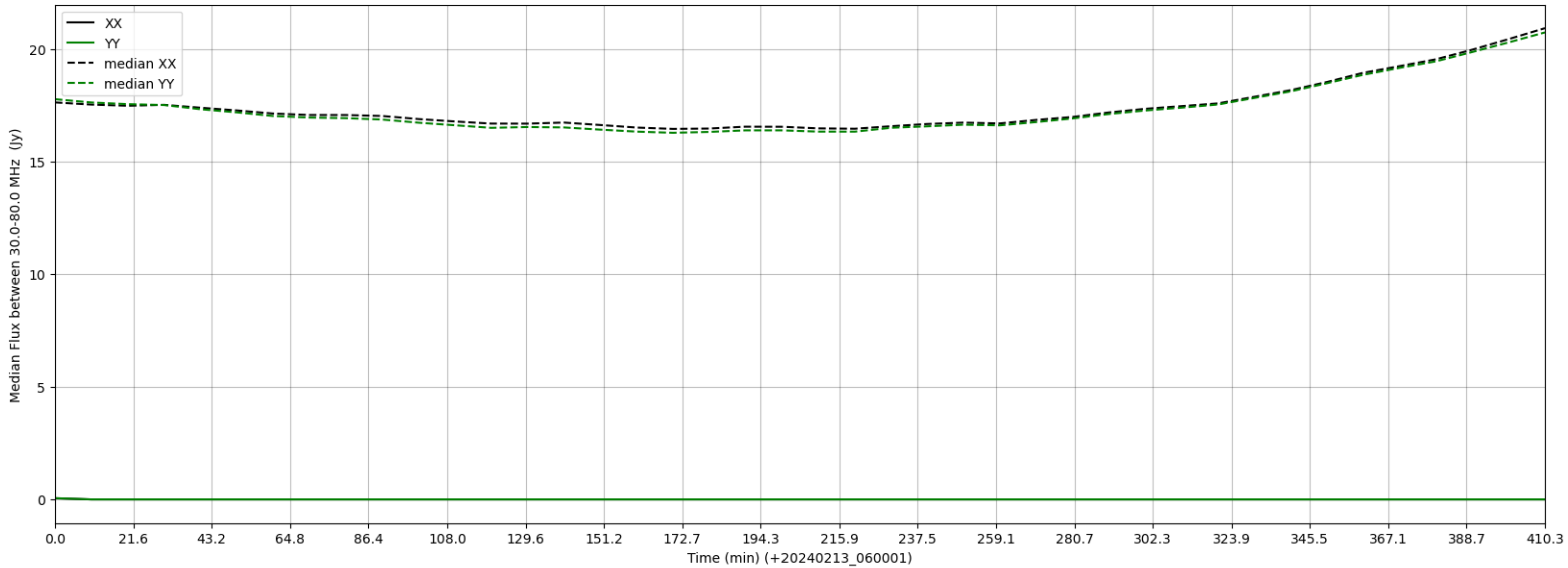
LWA138 - Correlator# 261 - XX FLAGS:LowFlux - YY FLAGS:LowFlux
