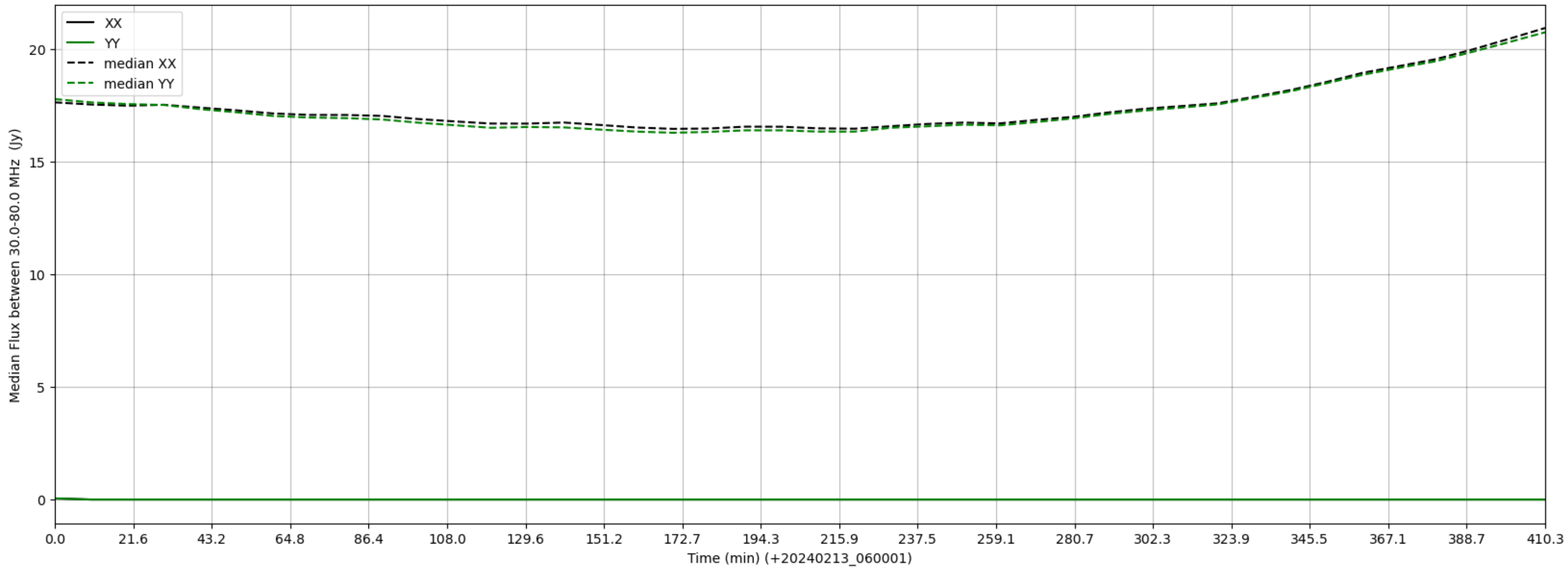
LWA164 - Correlator# 267 - XX FLAGS:LowFlux - YY FLAGS:LowFlux
