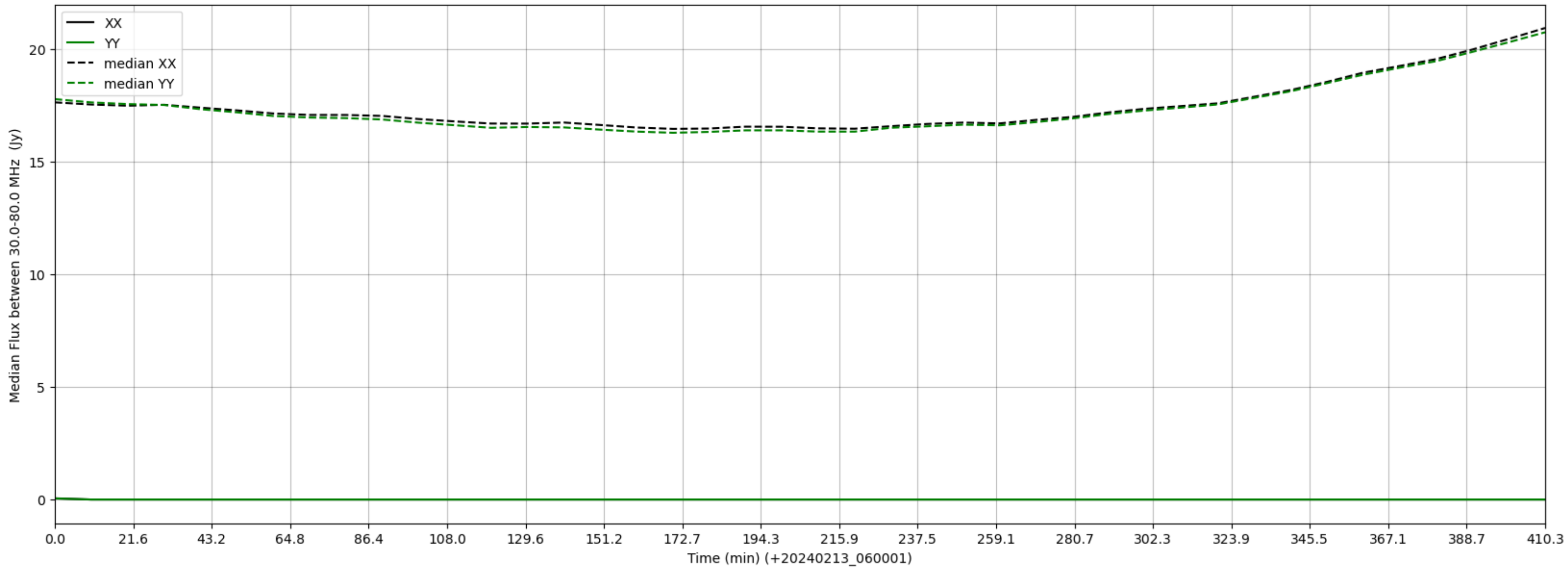
LWA198 - Correlator# 271 - XX FLAGS:LowFlux - YY FLAGS:LowFlux
