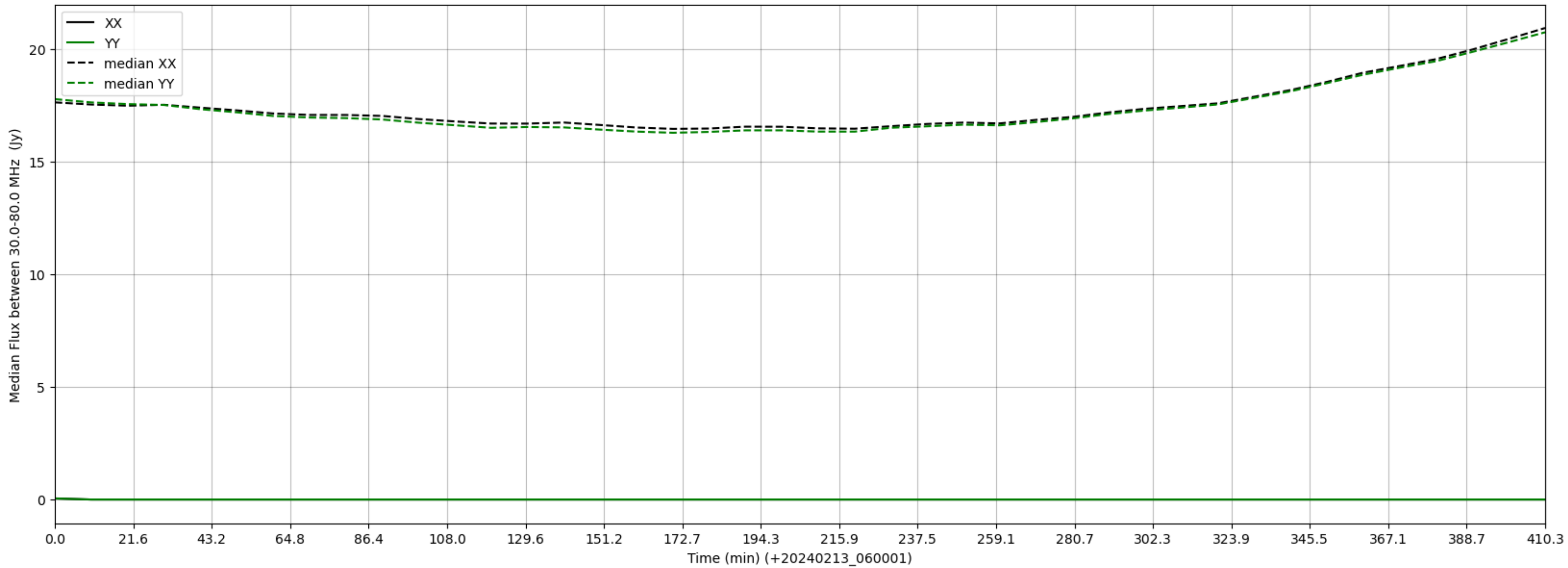
LWA141 - Correlator# 263 - XX FLAGS:LowFlux - YY FLAGS:LowFlux
