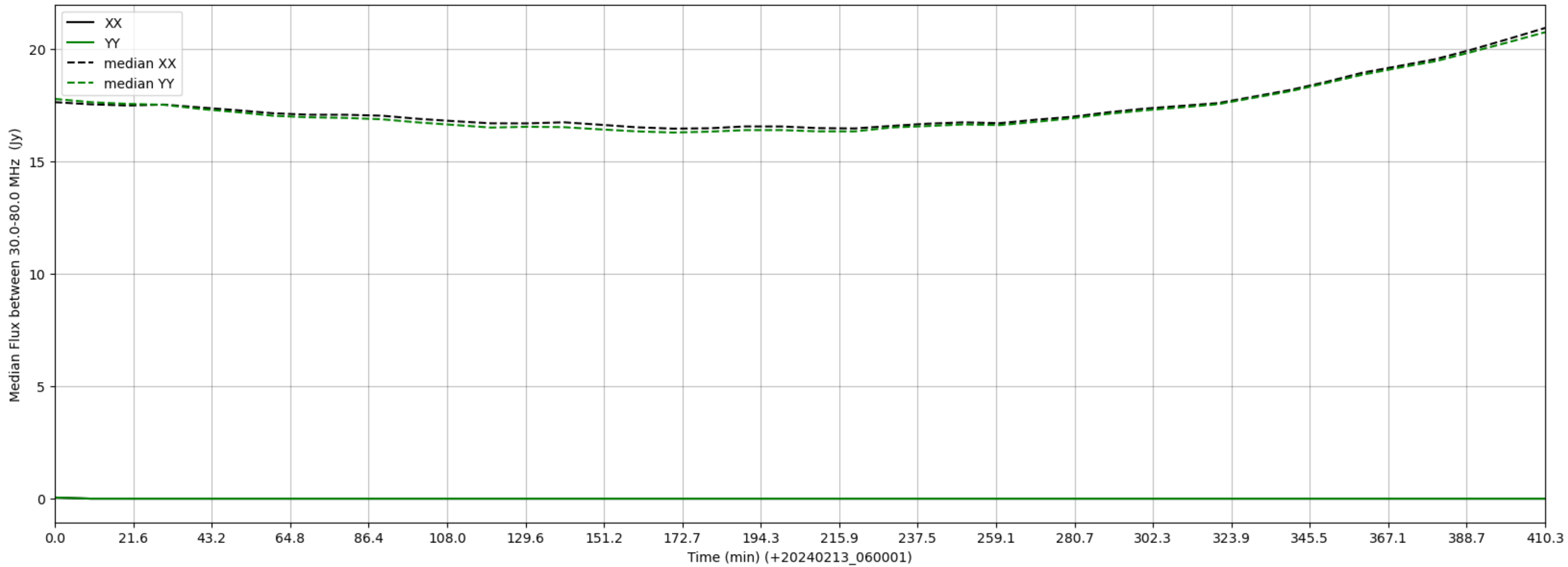
LWA167 - Correlator# 268 - XX FLAGS:LowFlux - YY FLAGS:LowFlux
