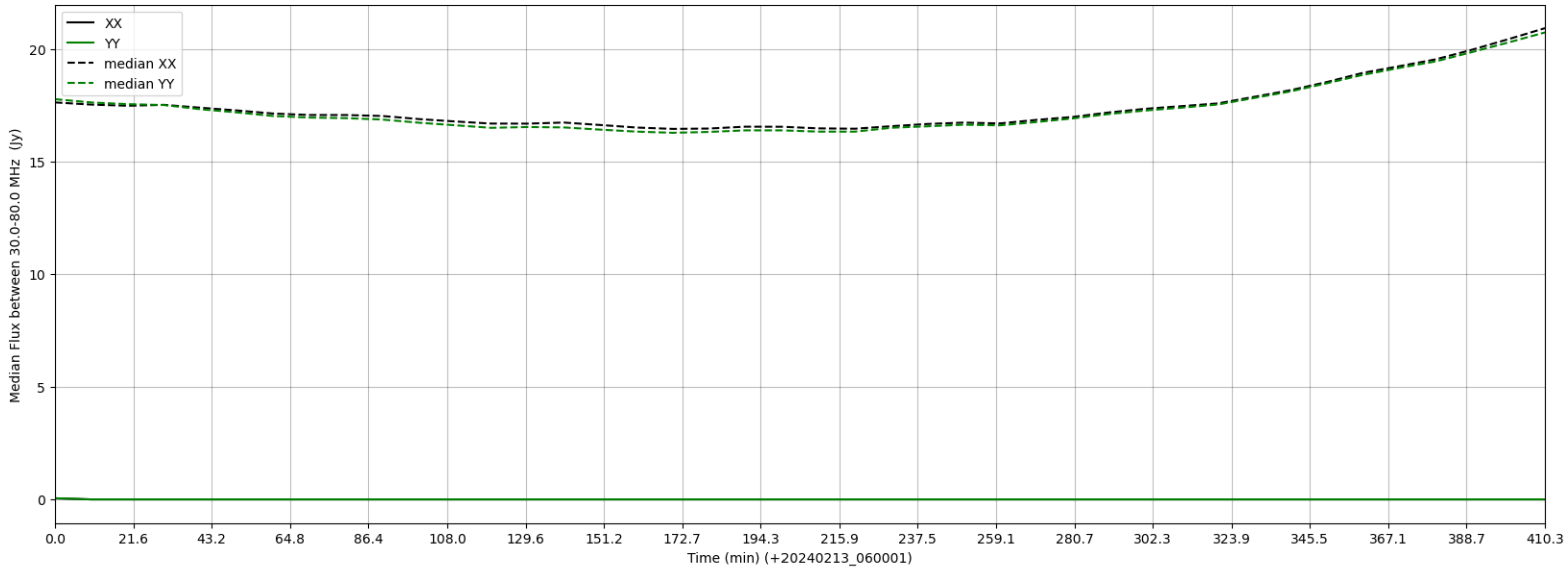
LWA161 - Correlator# 262 - XX FLAGS:LowFlux - YY FLAGS:LowFlux
