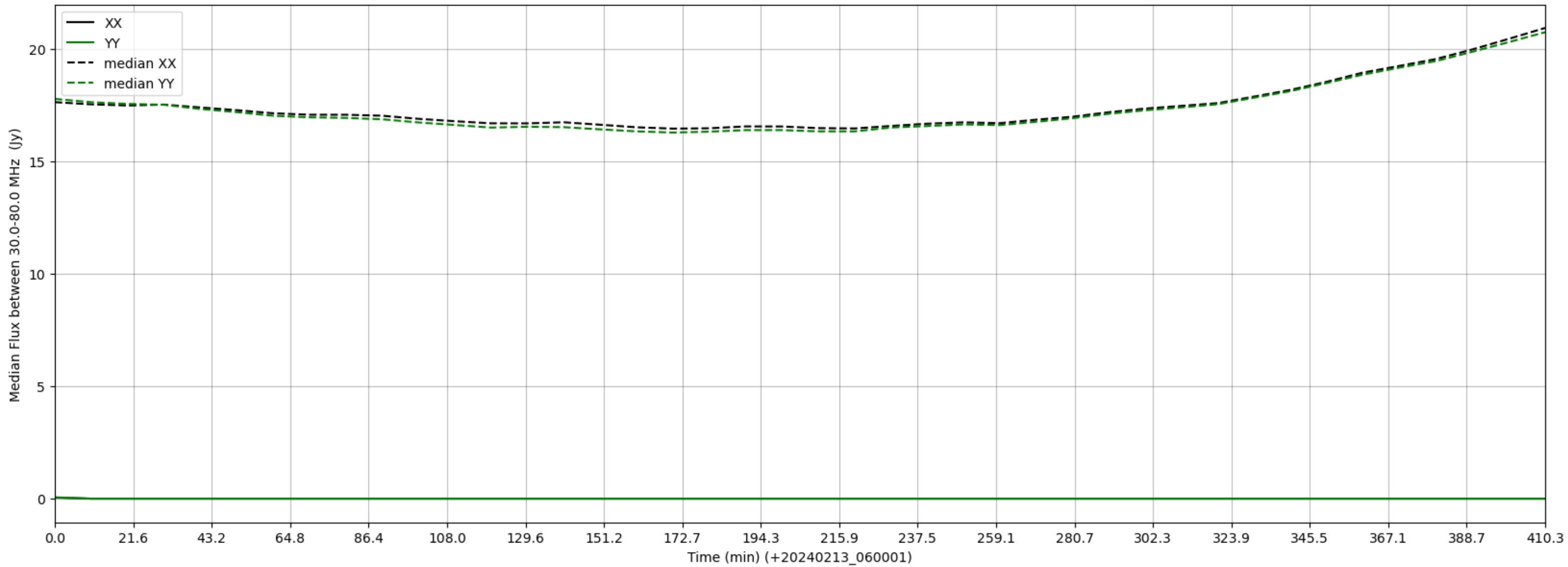
LWA140 - Correlator# 260 - XX FLAGS:LowFlux - YY FLAGS:LowFlux
