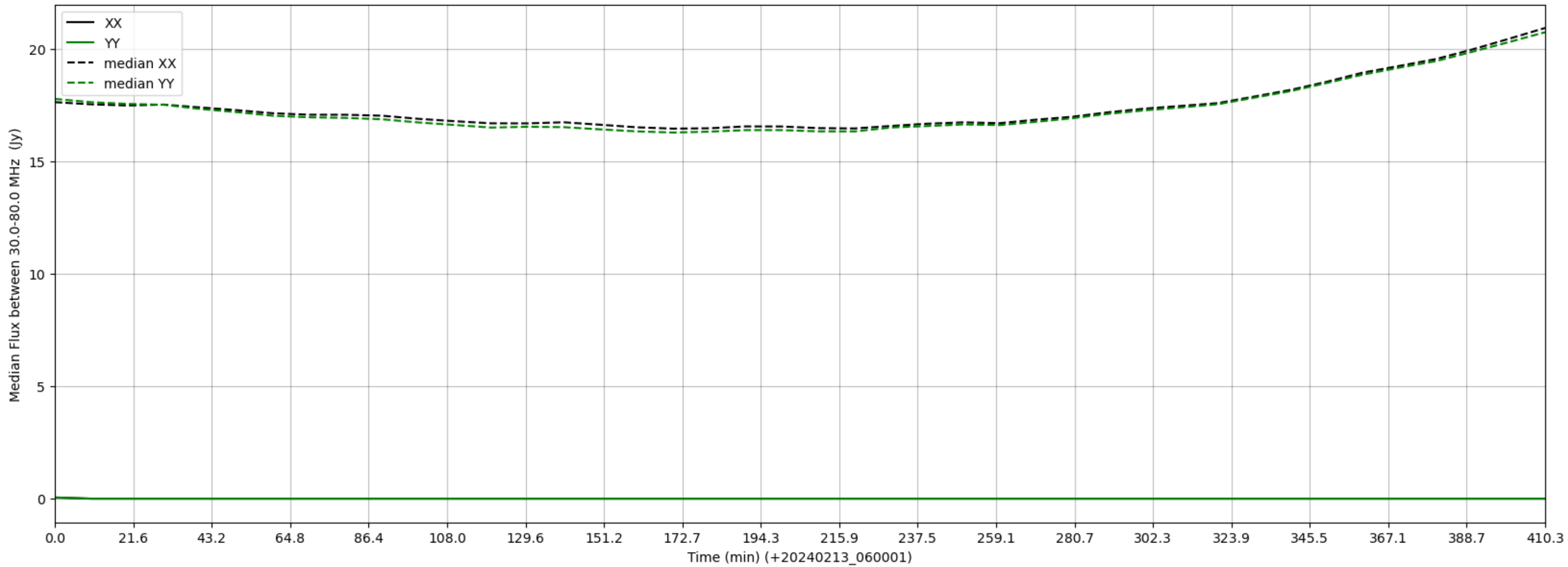
LWA193 - Correlator# 270 - XX FLAGS:LowFlux - YY FLAGS:LowFlux
