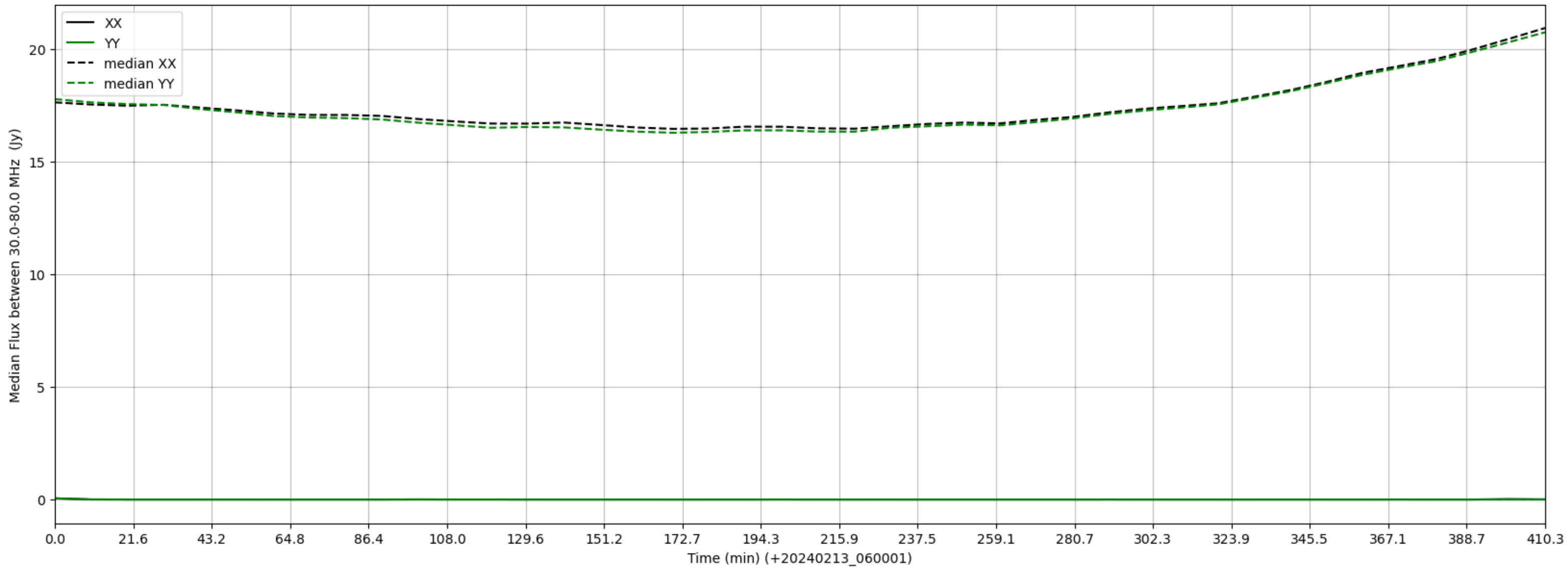
LWA165 - Correlator# 266 - XX FLAGS:LowFlux - YY FLAGS:LowFlux
