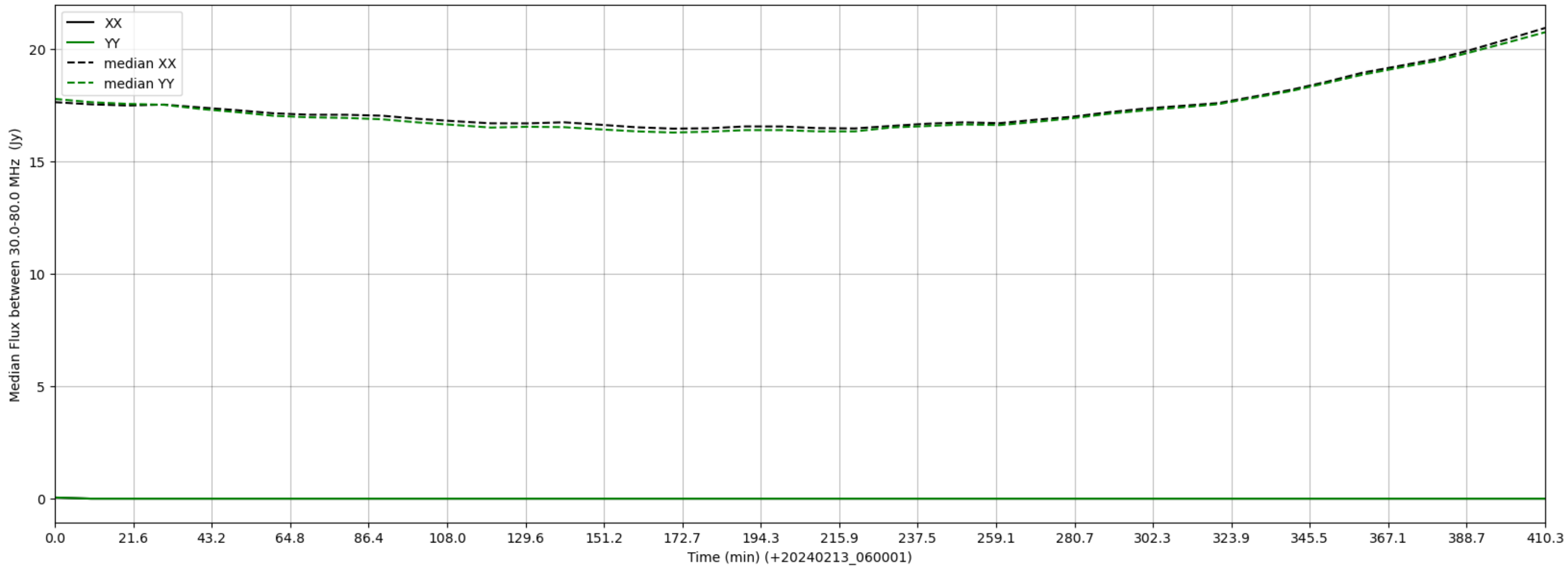
LWA166 - Correlator# 269 - XX FLAGS:LowFlux - YY FLAGS:LowFlux
