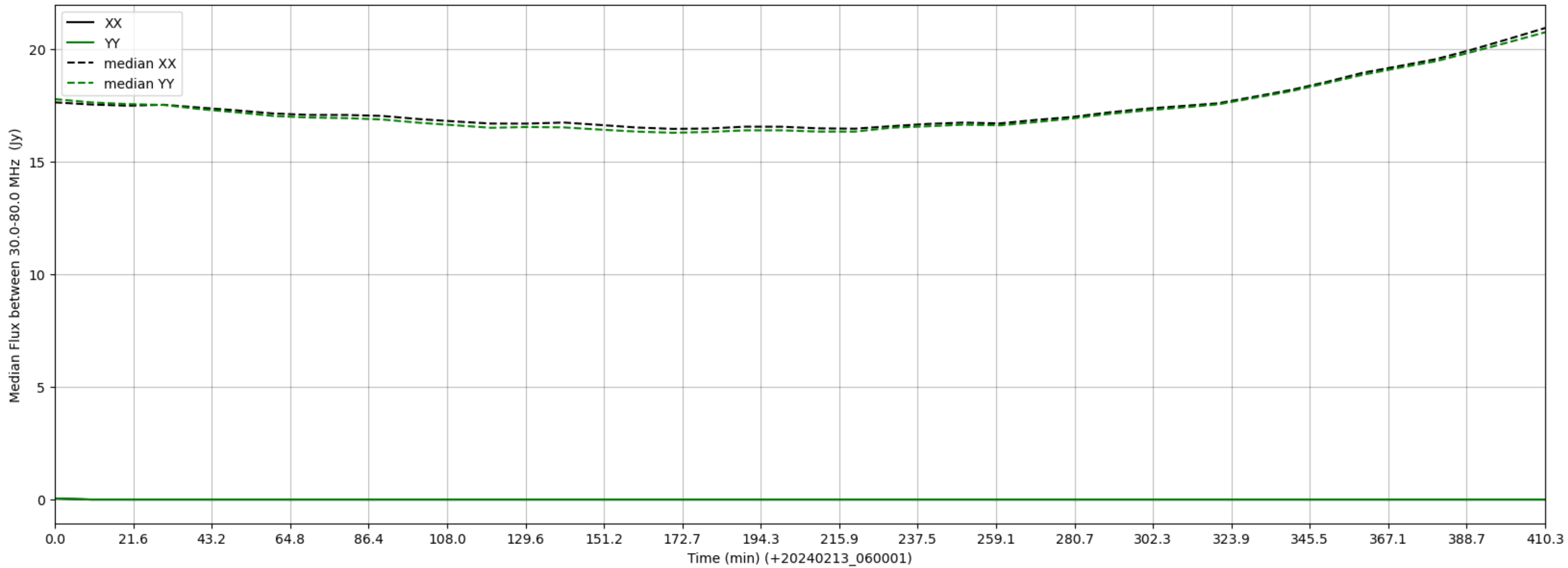
LWA163 - Correlator# 264 - XX FLAGS:LowFlux - YY FLAGS:LowFlux
