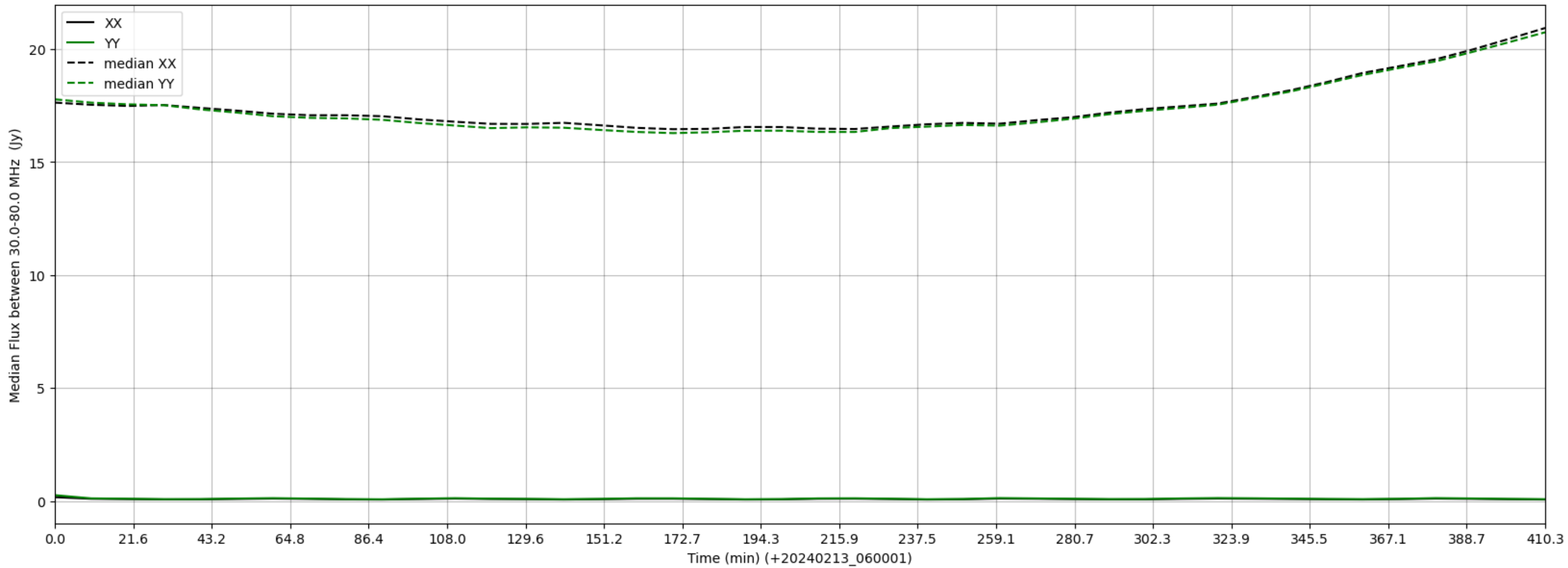
LWA137 - Correlator# 258 - XX FLAGS:LowFlux - YY FLAGS:LowFlux
