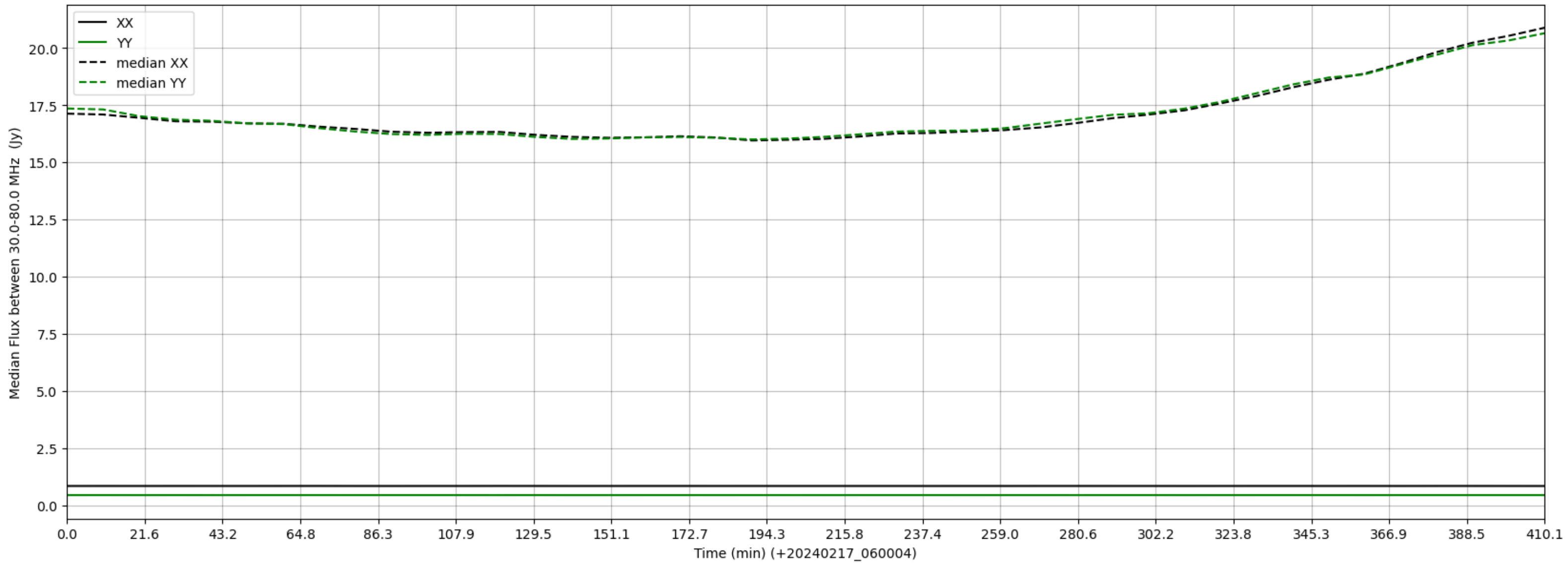
LWA286 - Correlator# 093 - XX FLAGS:LowFlux - YY FLAGS:LowFlux
