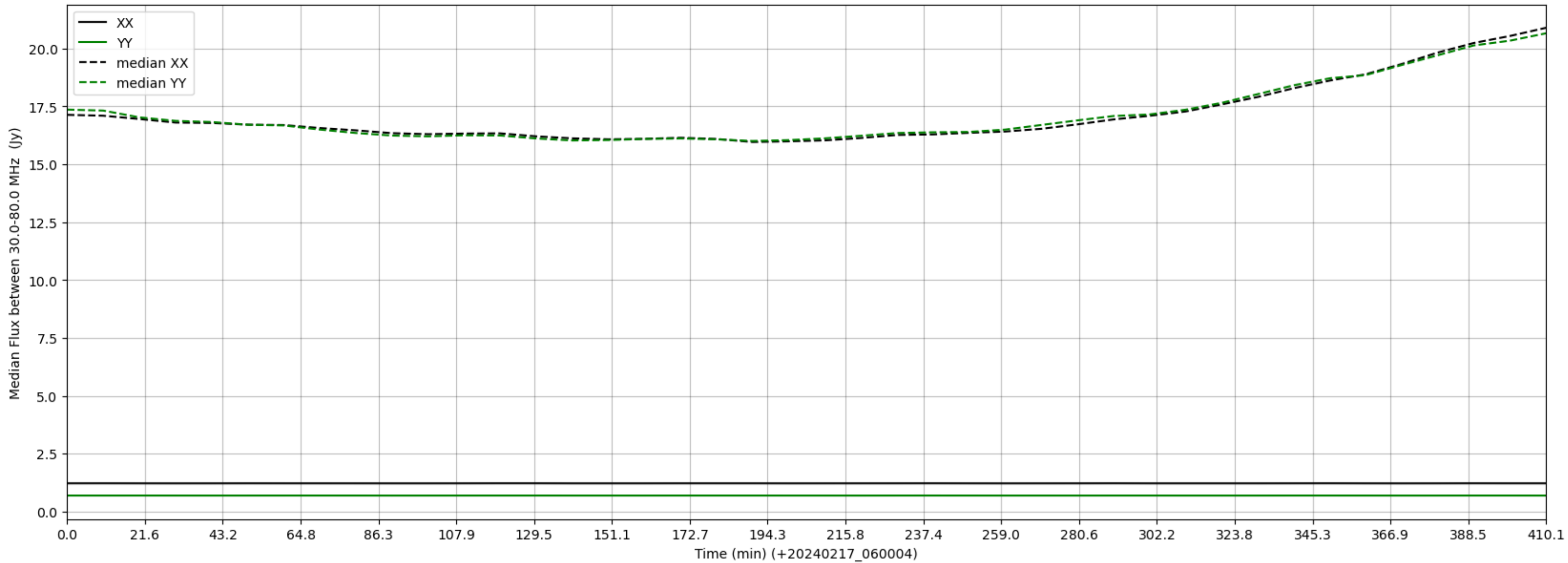
LWA277 - Correlator# 009 - XX FLAGS:LowFlux - YY FLAGS:LowFlux
