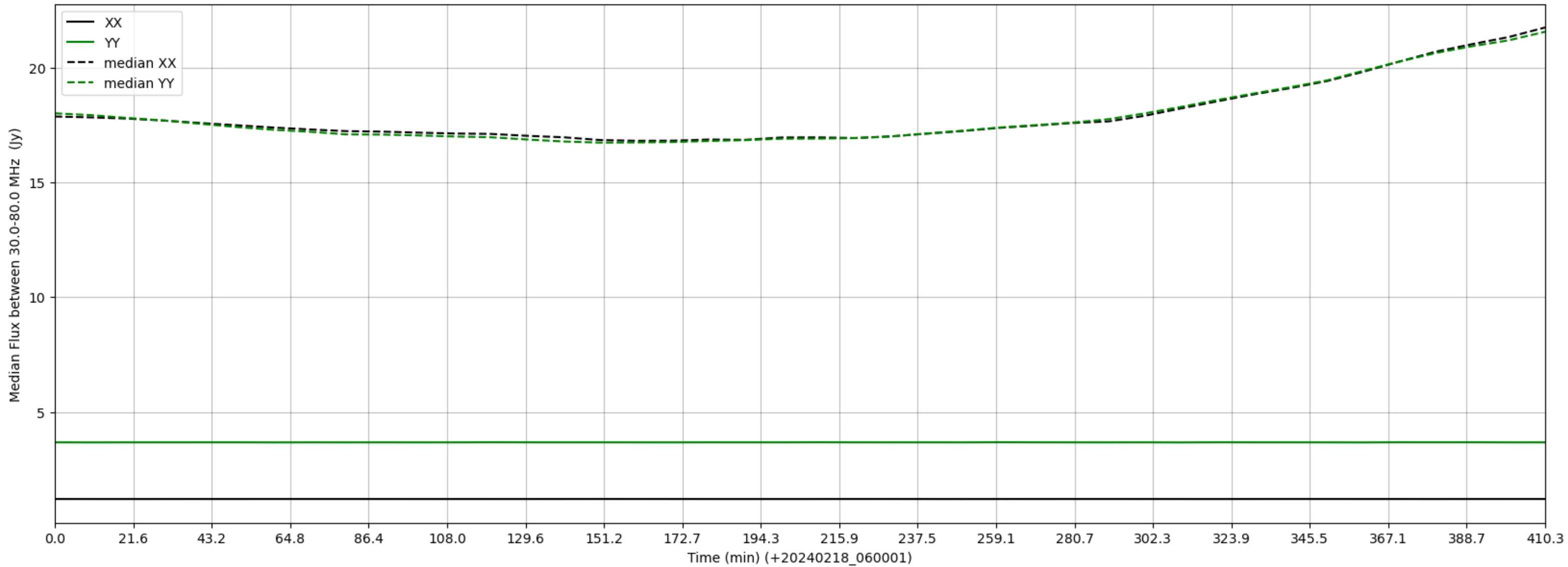
LWA344 - Correlator# 061 - XX FLAGS:LowFlux - YY FLAGS:BadSpecShape
