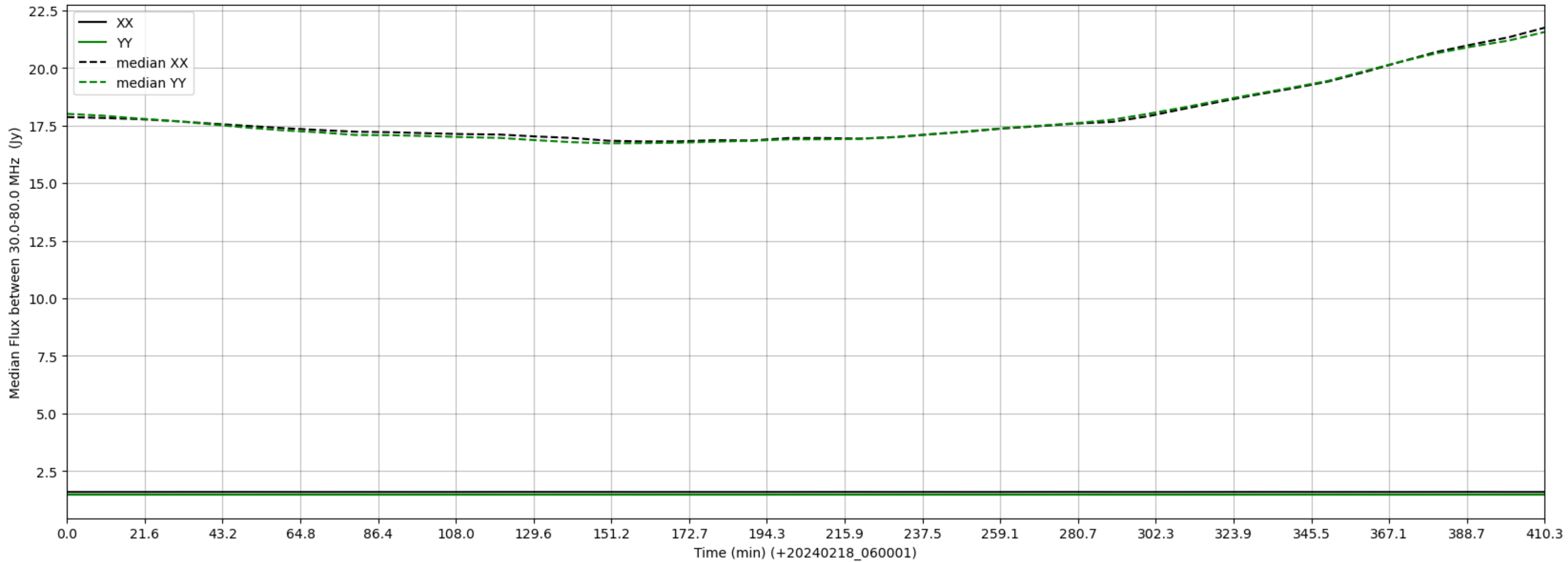
LWA334 - Correlator# 156 - XX FLAGS:LowFlux - YY FLAGS:LowFlux
