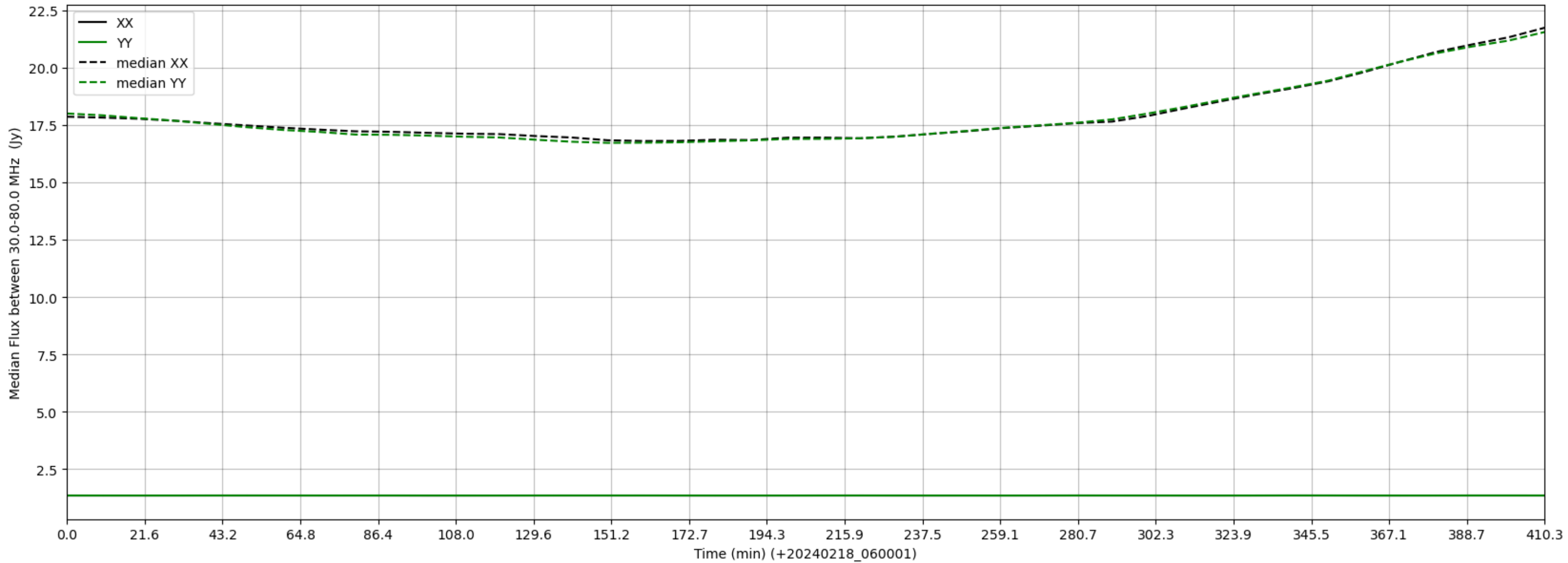
LWA319 - Correlator# 190 - XX FLAGS:LowFlux - YY FLAGS:LowFlux
