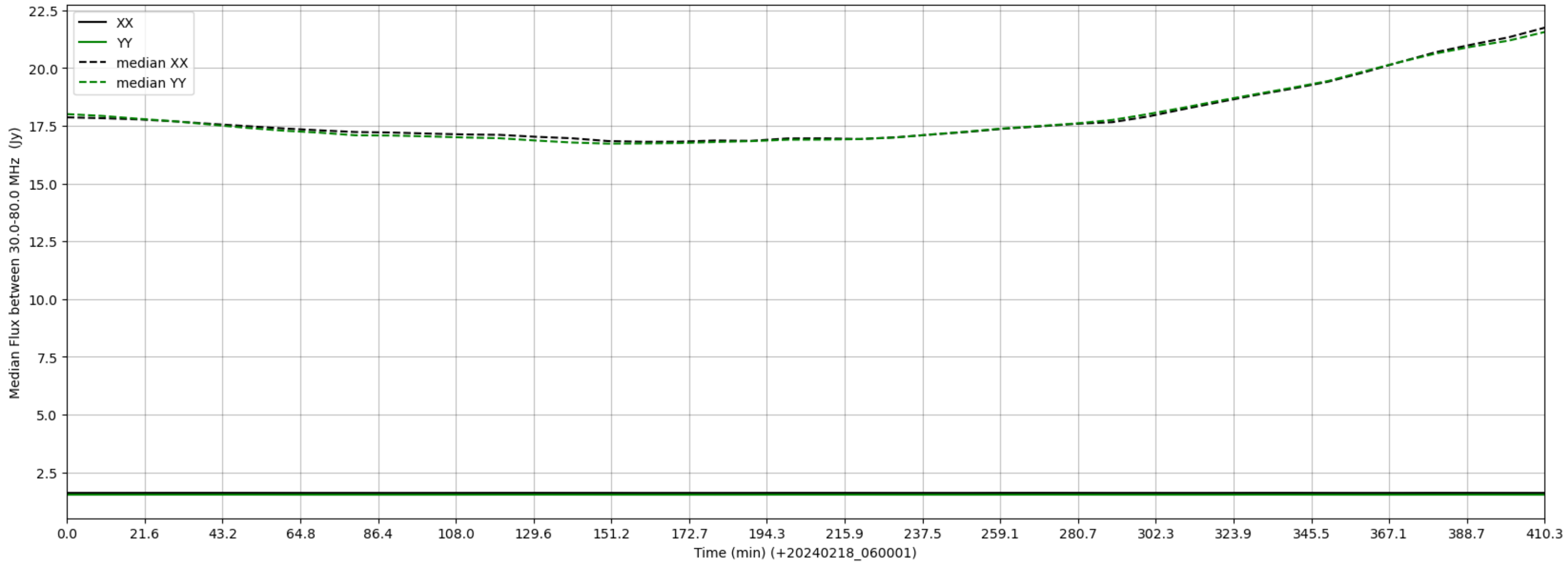
LWA340 - Correlator# 026 - XX FLAGS:LowFlux - YY FLAGS:LowFlux
