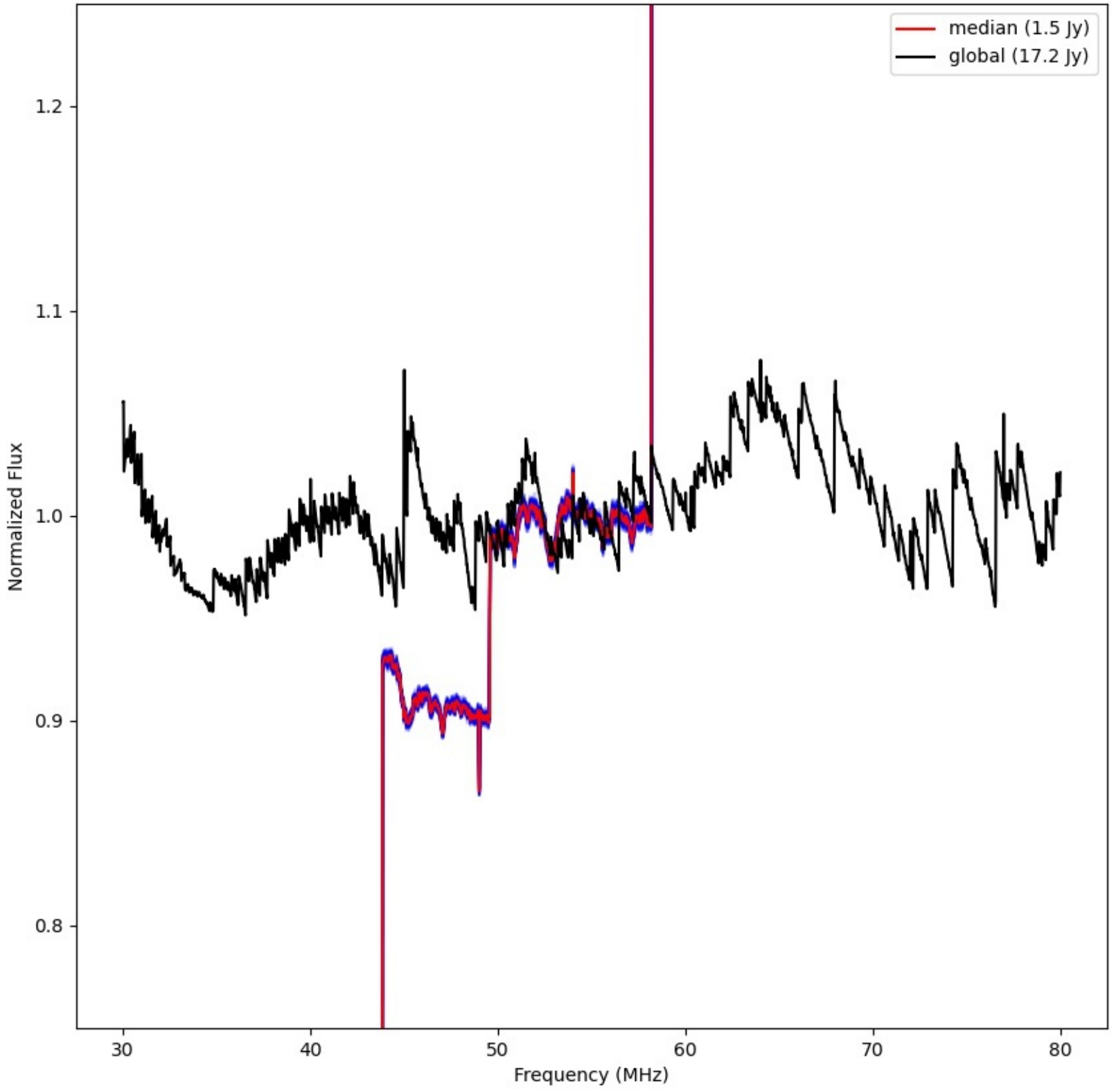
LWA341 - Correlator# 029 - XX - FLAGS:LowFlux
