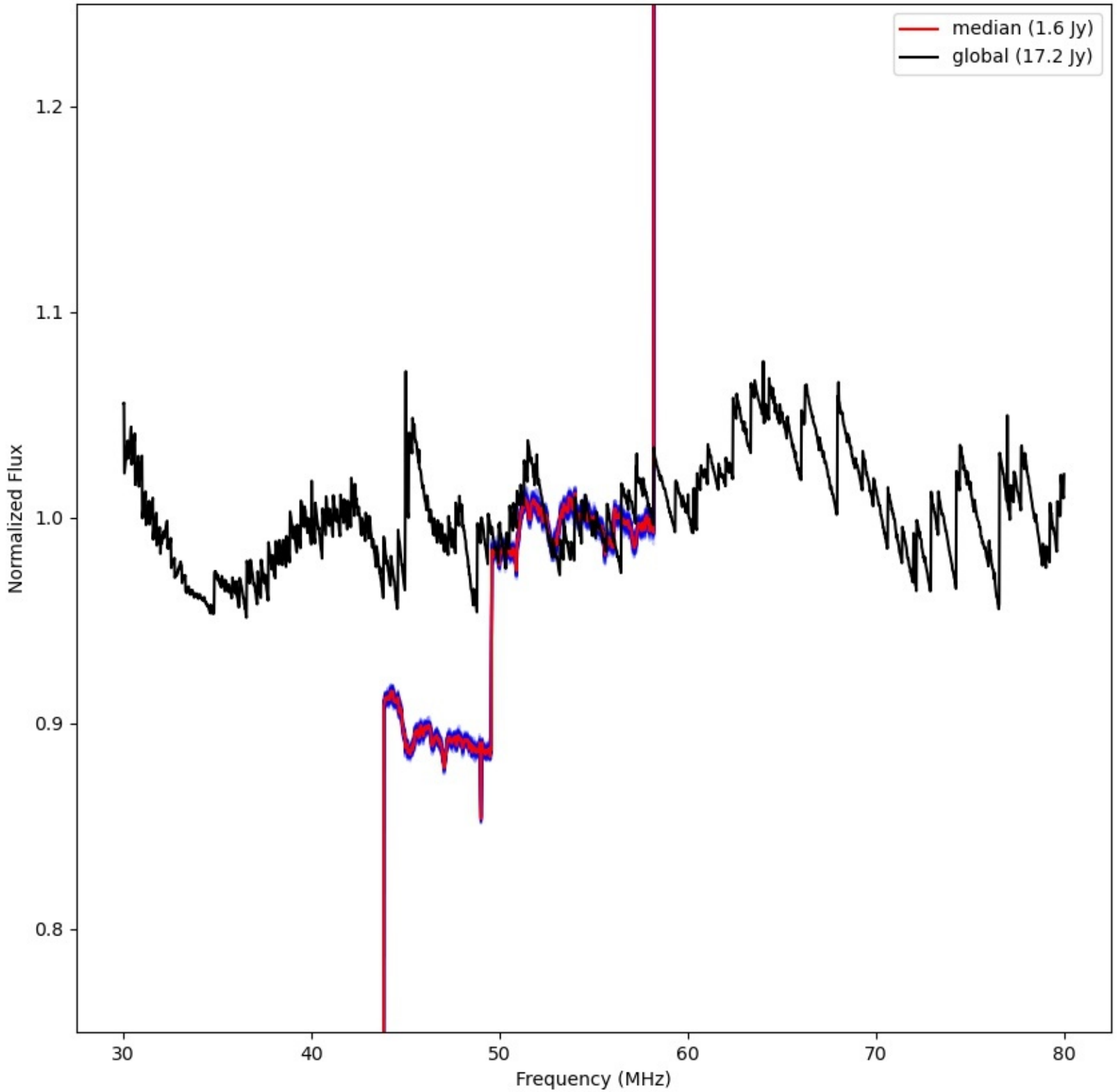
LWA340 - Correlator# 026 - XX - FLAGS:LowFlux
