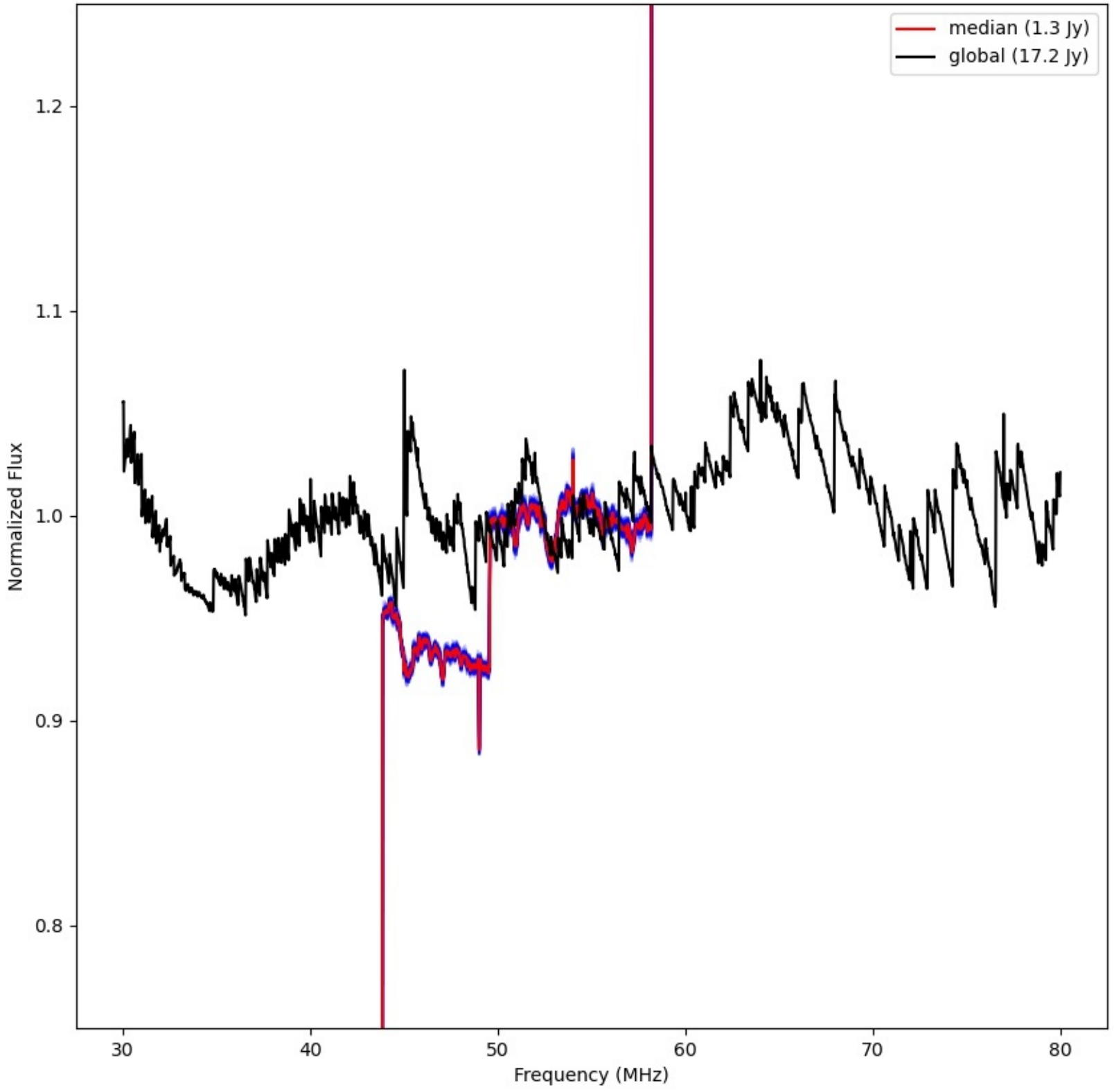
LWA282 - Correlator# 010 - XX - FLAGS:LowFlux
