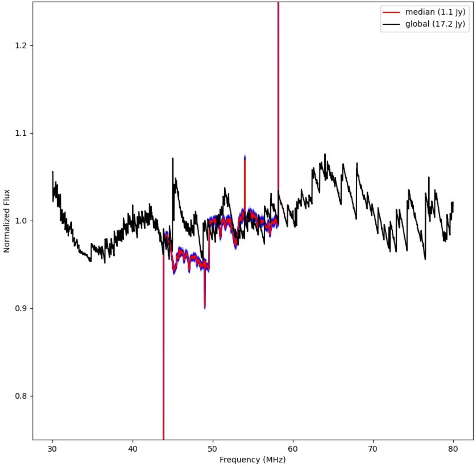
LWA296 - Correlator# 046 - XX - FLAGS:LowFlux
