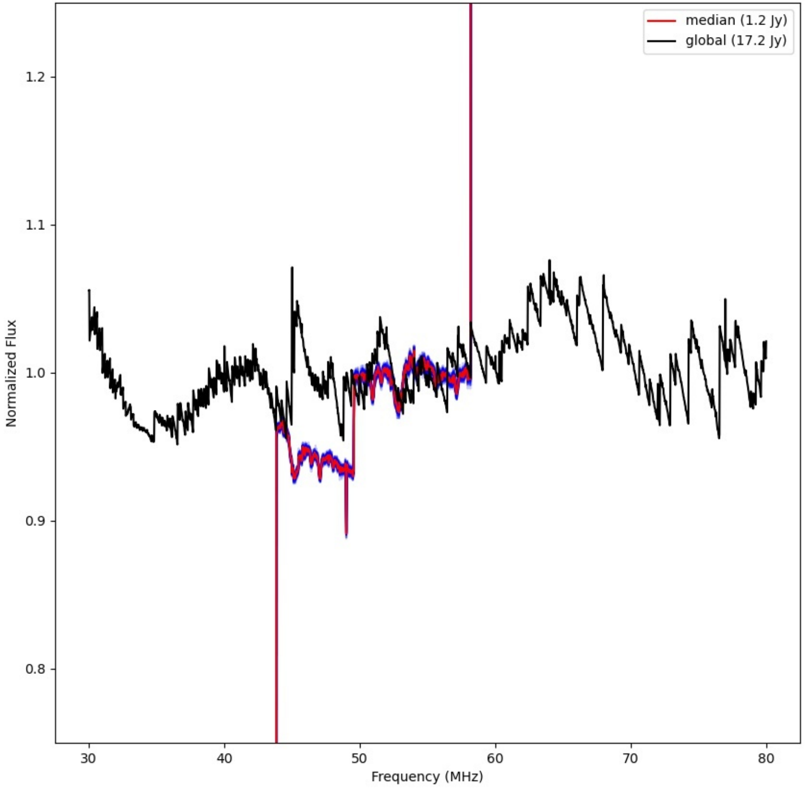
LWA344 - Correlator# 061 - XX - FLAGS:LowFlux
