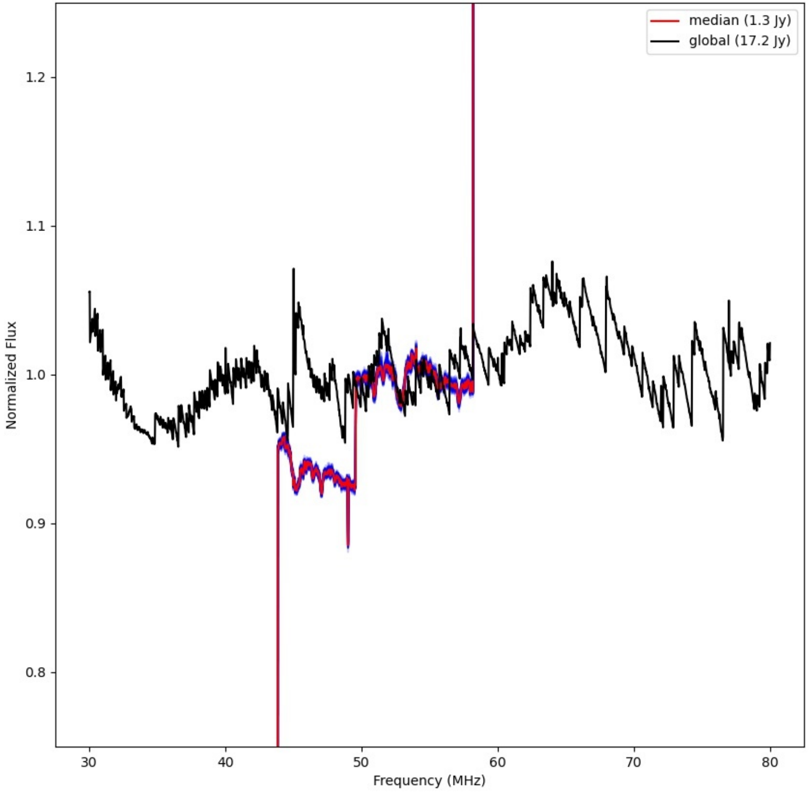
LWA268 - Correlator# 002 - XX - FLAGS:LowFlux
