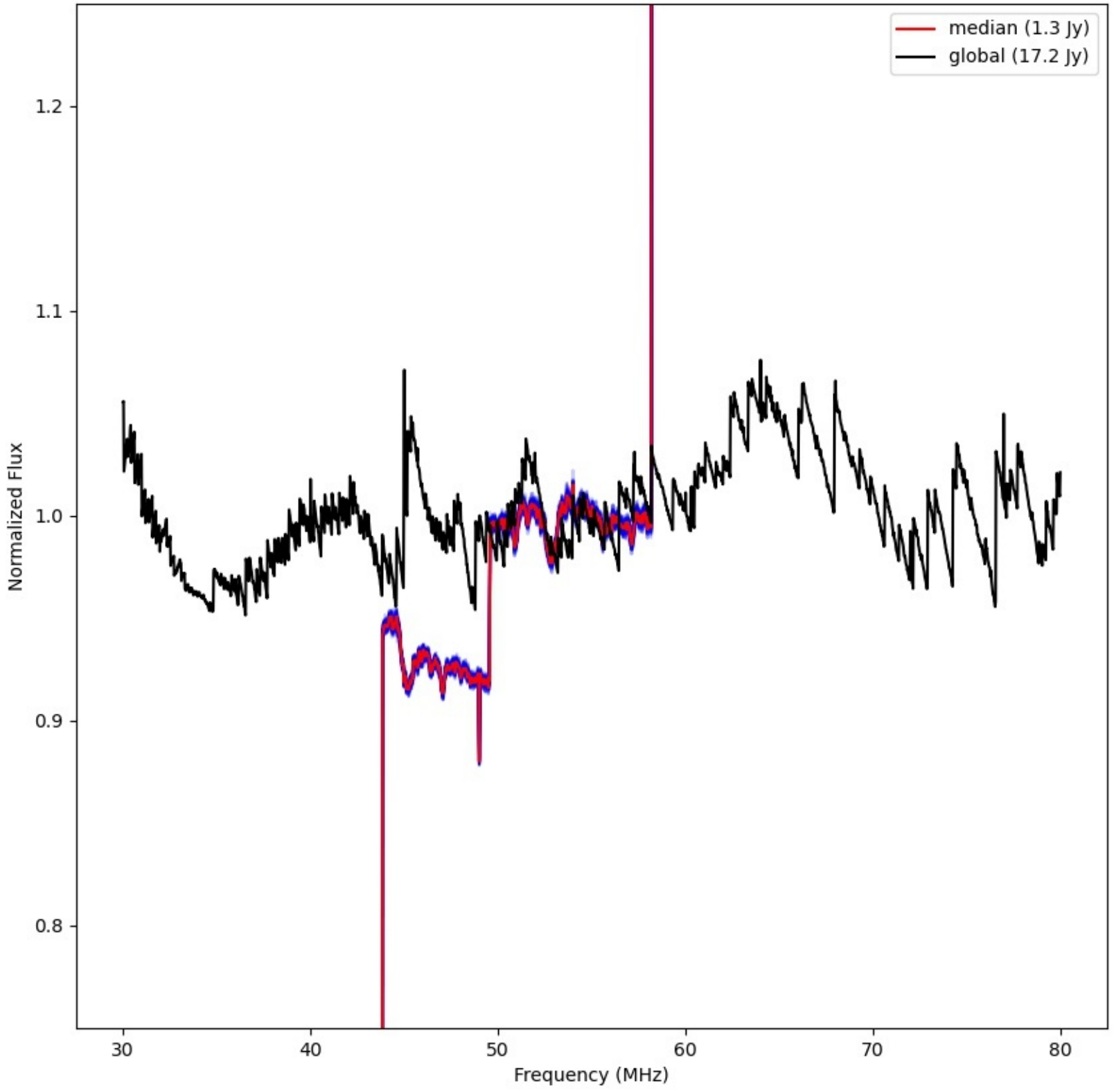
LWA308 - Correlator# 015 - XX - FLAGS:LowFlux
