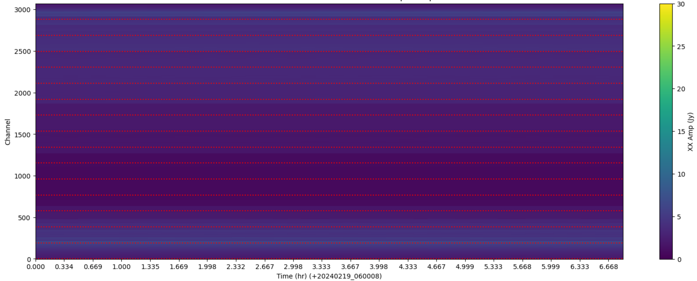
LWA320 - Correlator# 054 - XX - FLAGS: BadSpecShape
