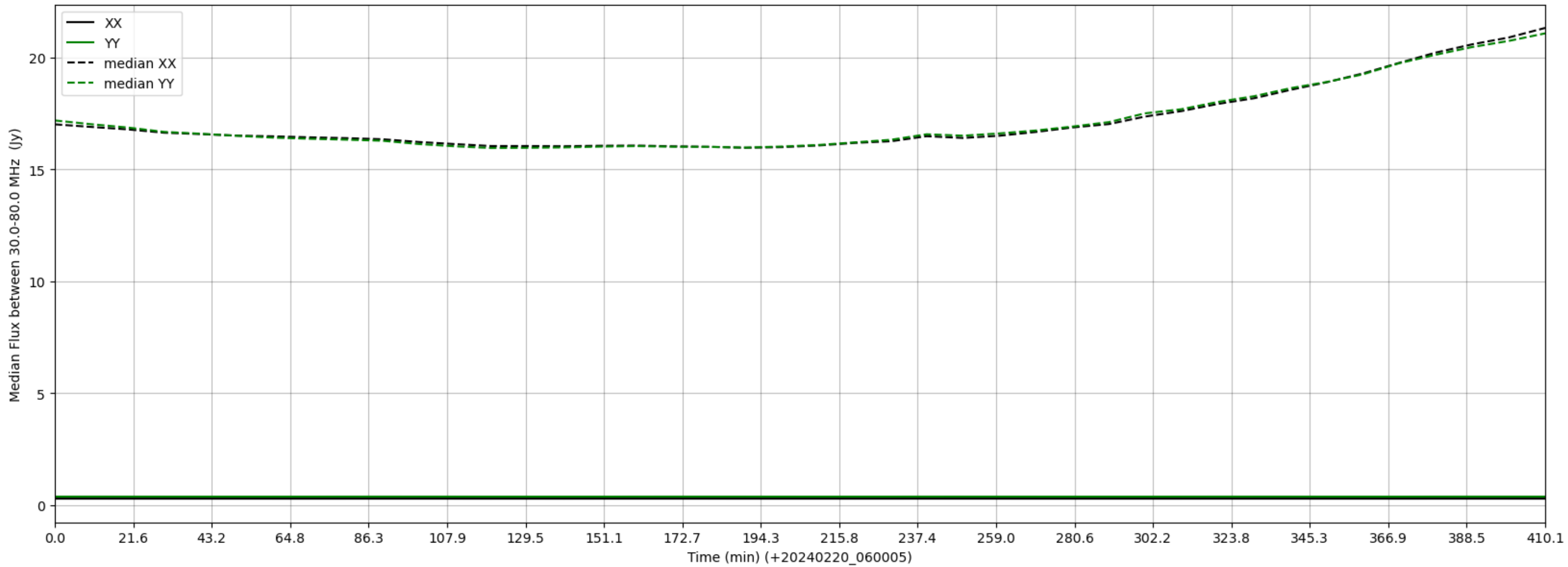
LWA338 - Correlator# 024 - XX FLAGS:LowFlux - YY FLAGS:LowFlux
