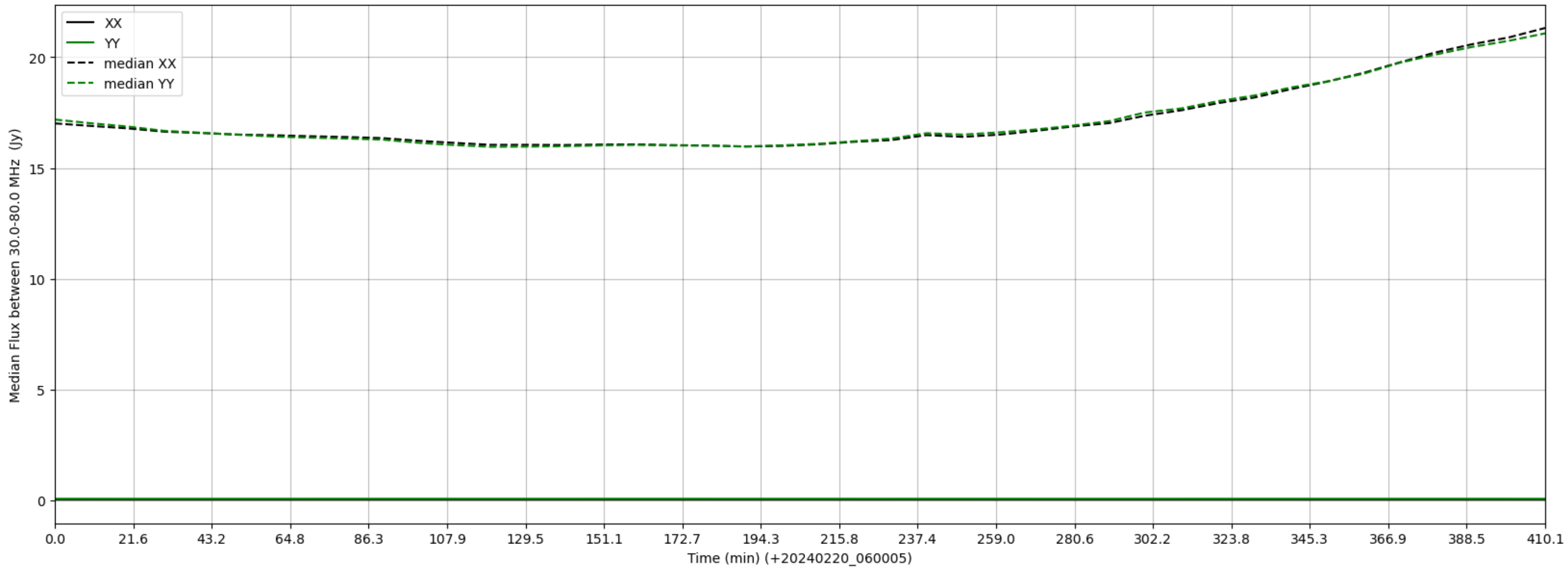
LWA347 - Correlator# 255 - XX FLAGS:LowFlux - YY FLAGS:LowFlux
