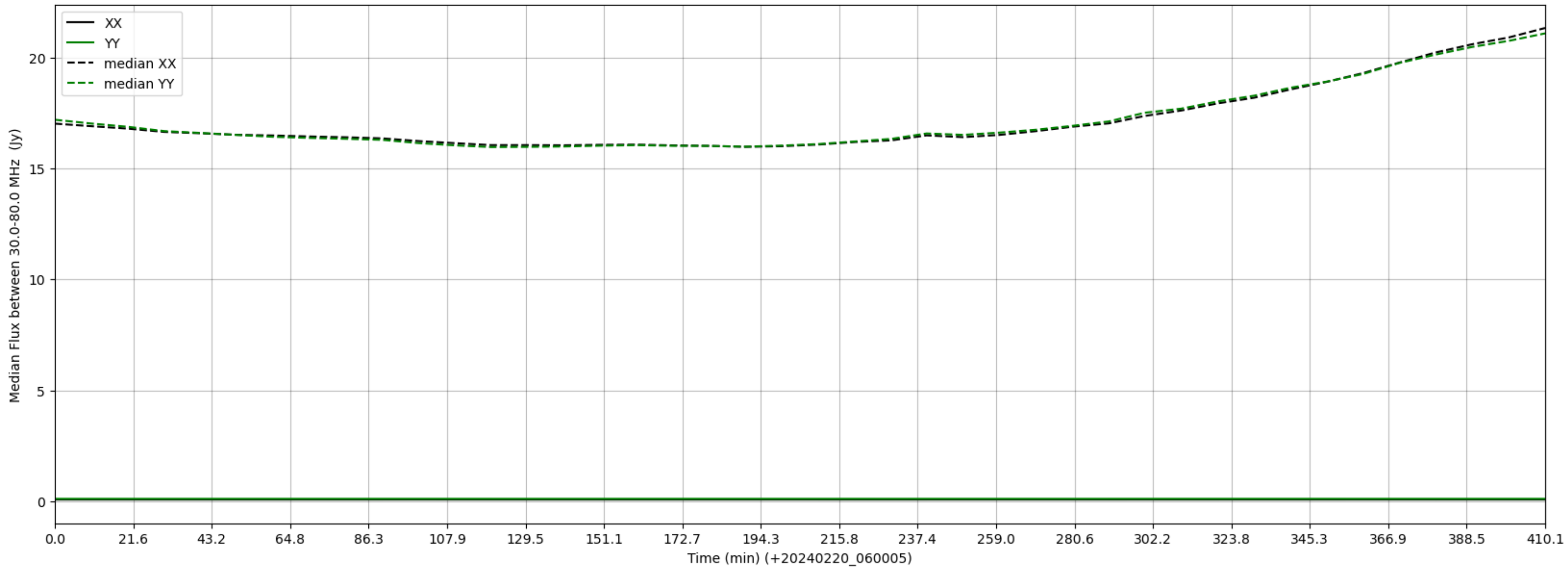
LWA343 - Correlator# 058 - XX FLAGS:LowFlux - YY FLAGS:LowFlux
