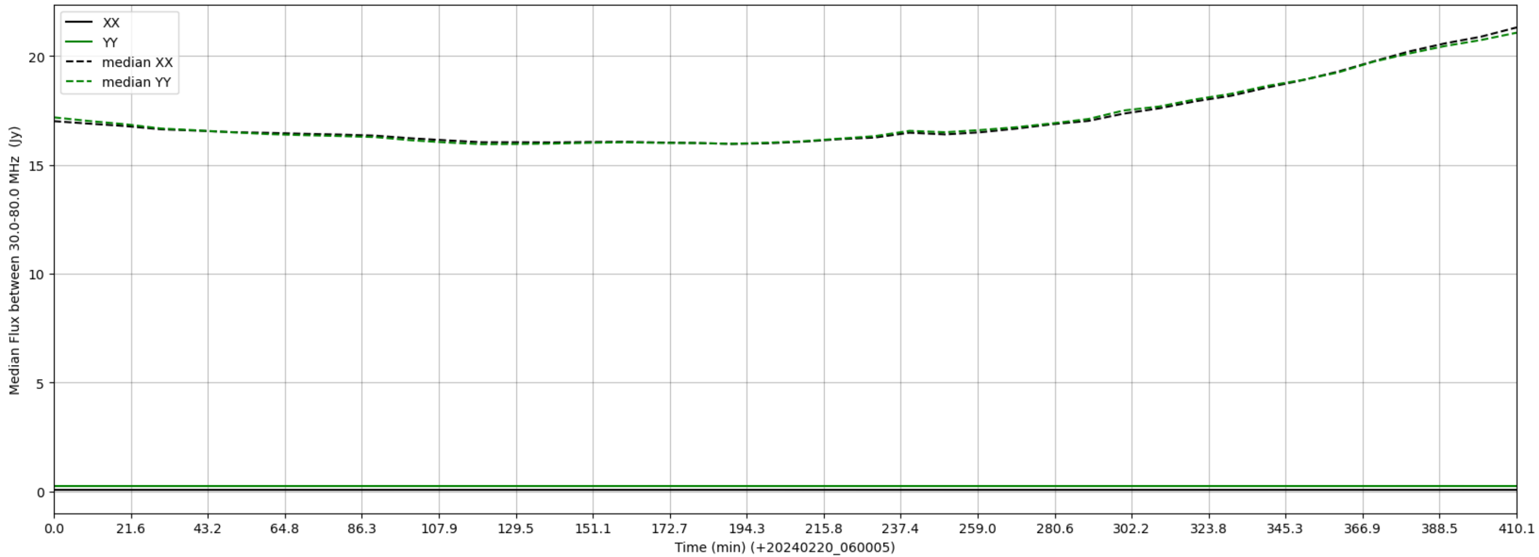
LWA291 - Correlator# 045 - XX FLAGS:LowFlux - YY FLAGS:LowFlux
