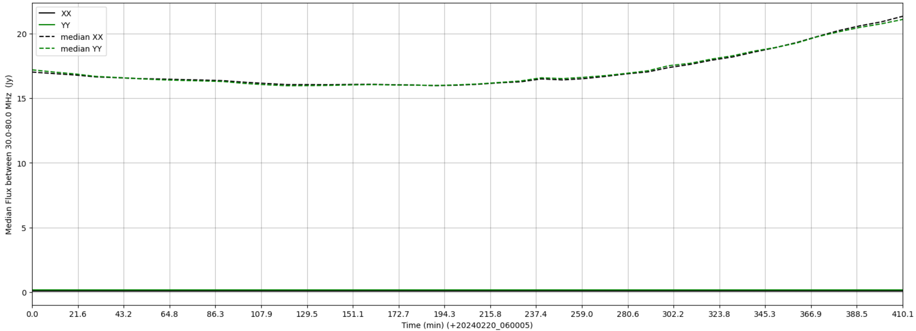
LWA271 - Correlator# 004 - XX FLAGS:LowFlux - YY FLAGS:LowFlux
