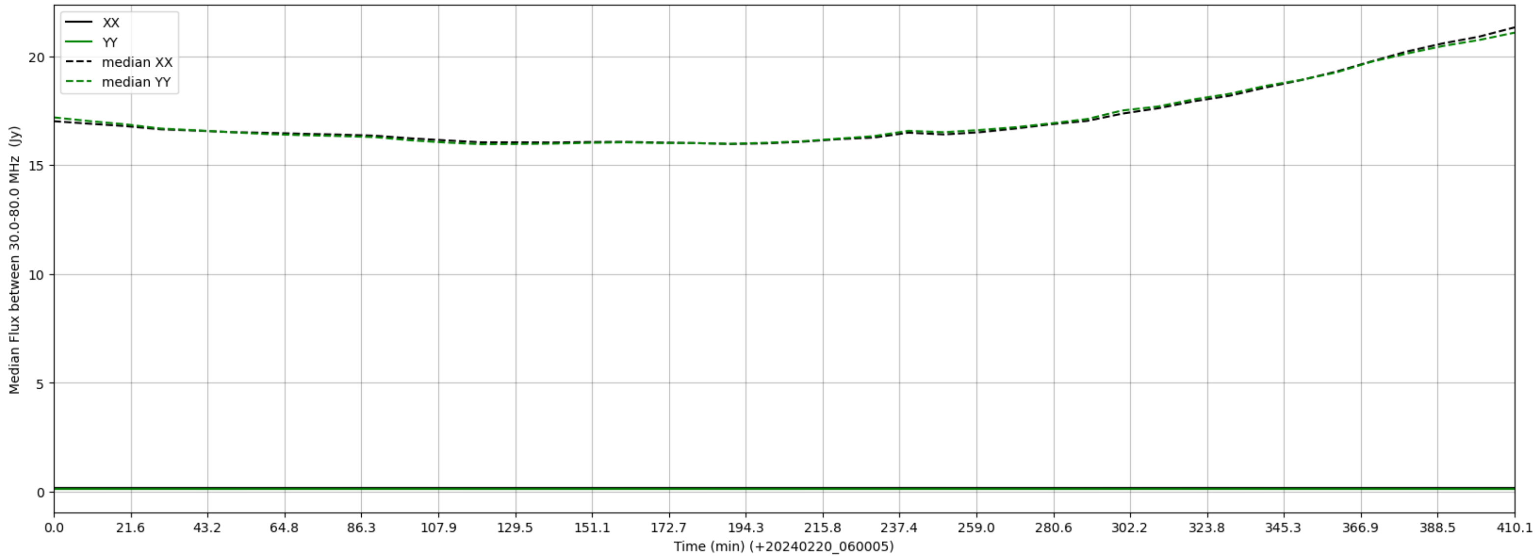
LWA270 - Correlator# 039 - XX FLAGS:LowFlux - YY FLAGS:LowFlux
