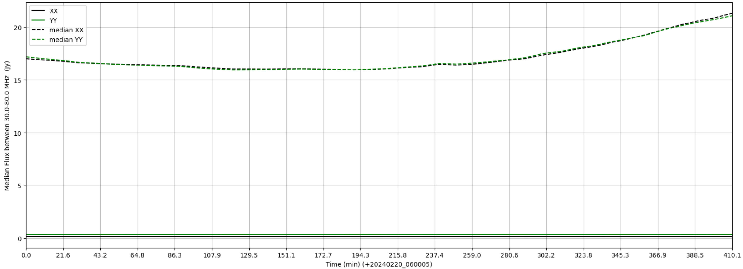
LWA272 - Correlator# 038 - XX FLAGS:LowFlux - YY FLAGS:LowFlux
