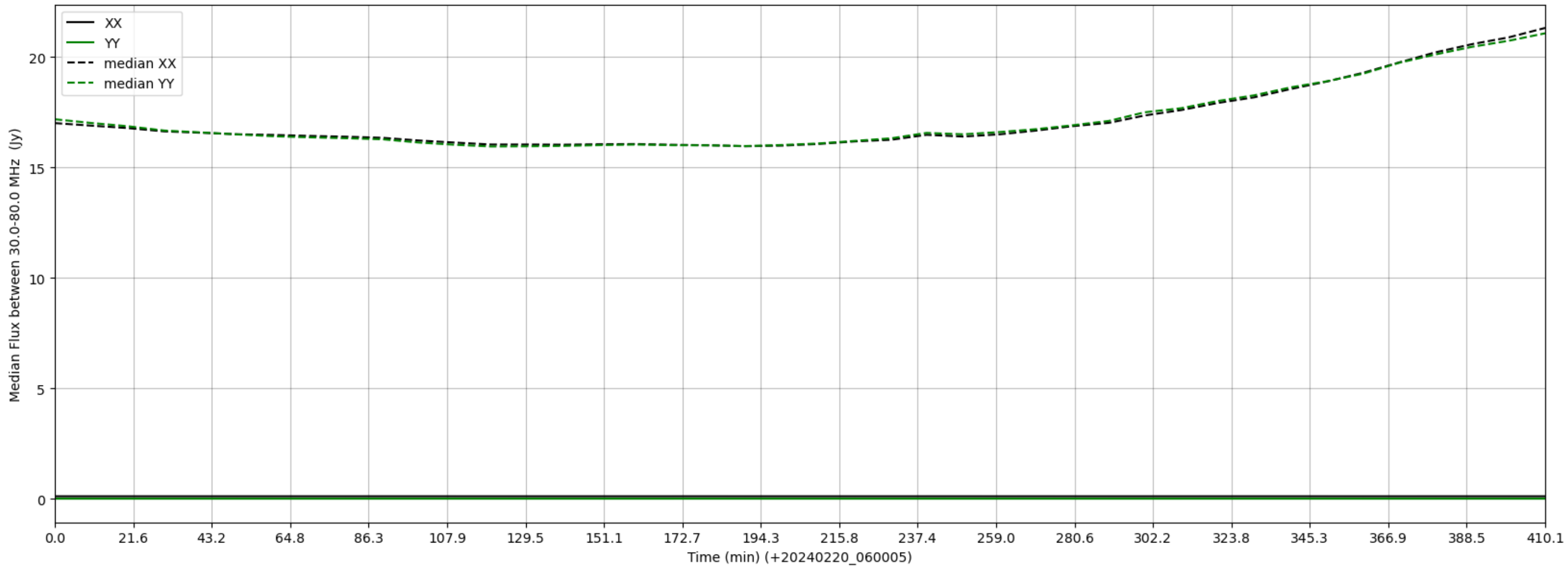
LWA285 - Correlator# 013 - XX FLAGS:LowFlux - YY FLAGS:LowFlux
