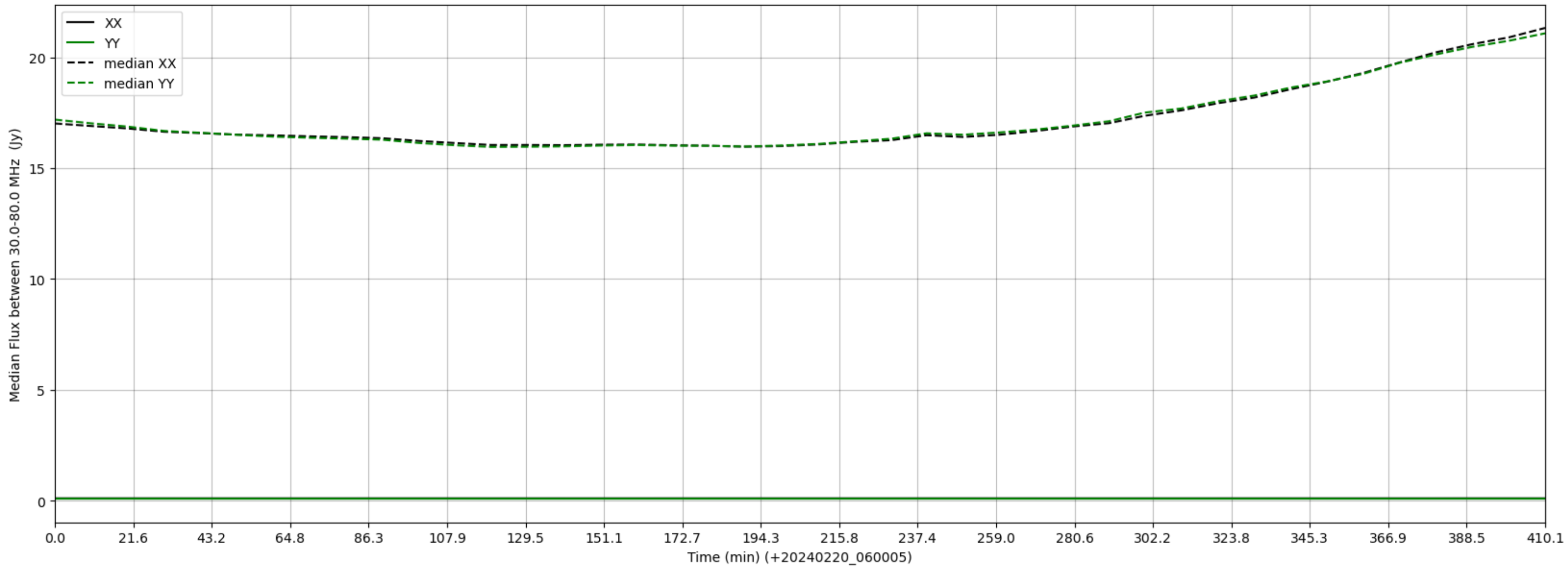
LWA340 - Correlator# 026 - XX FLAGS:LowFlux - YY FLAGS:LowFlux
