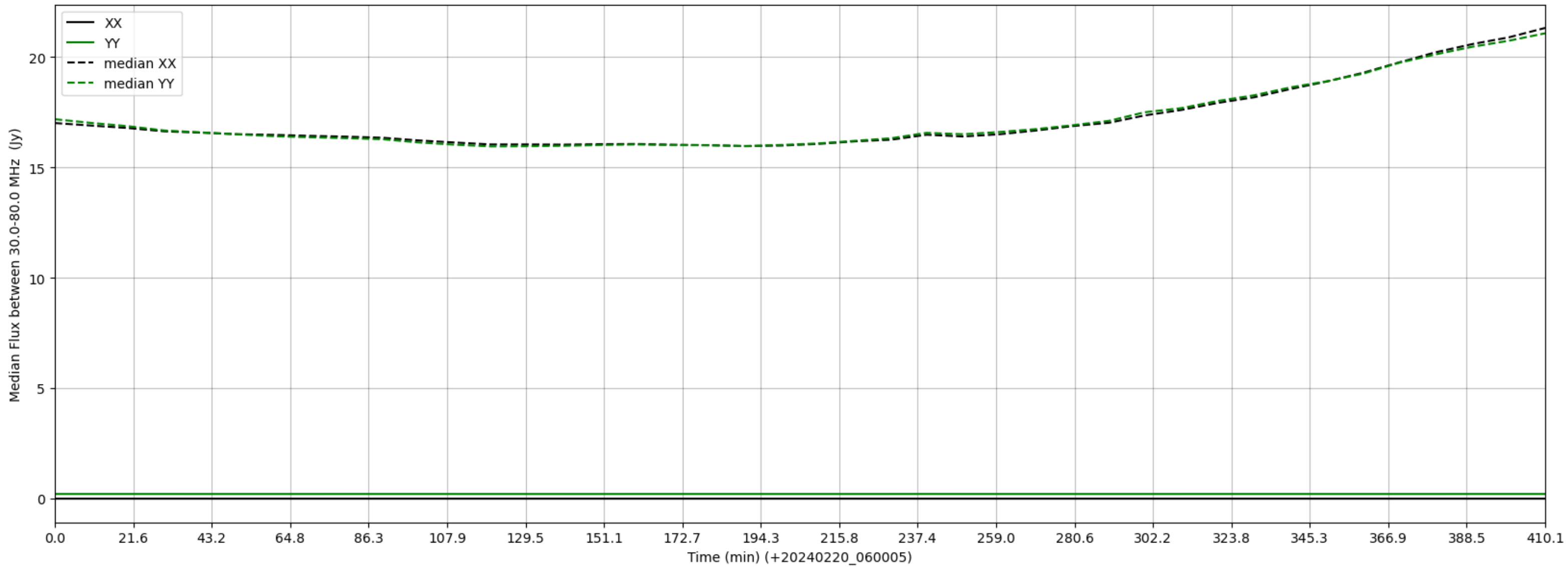
LWA322 - Correlator# 251 - XX FLAGS:LowFlux - YY FLAGS:LowFlux
