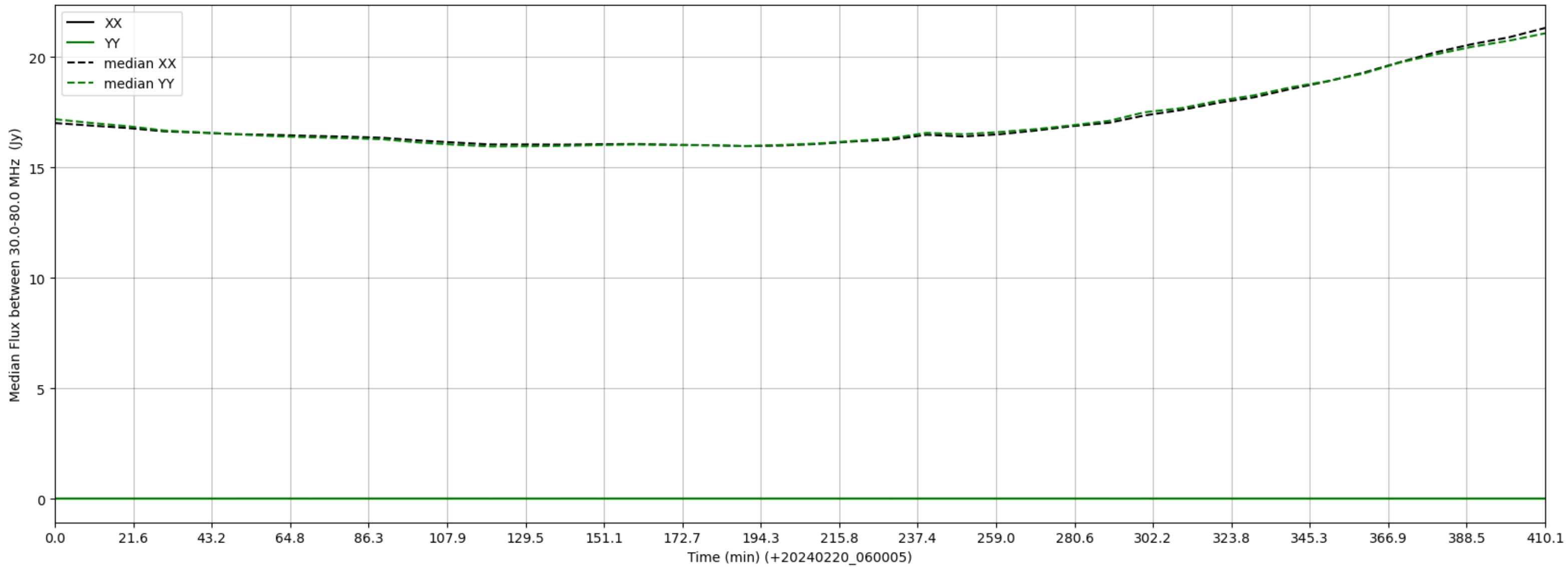
LWA281 - Correlator# 011 - XX FLAGS:LowFlux - YY FLAGS:LowFlux
