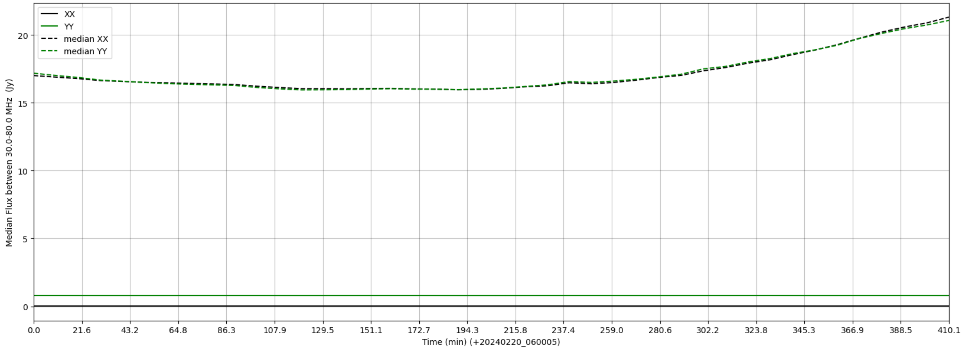
LWA335 - Correlator# 057 - XX FLAGS:LowFlux - YY FLAGS:LowFlux
