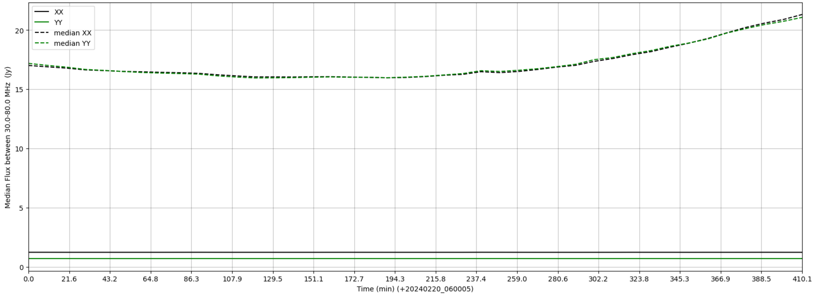
LWA277 - Correlator# 009 - XX FLAGS:LowFlux - YY FLAGS:LowFlux
