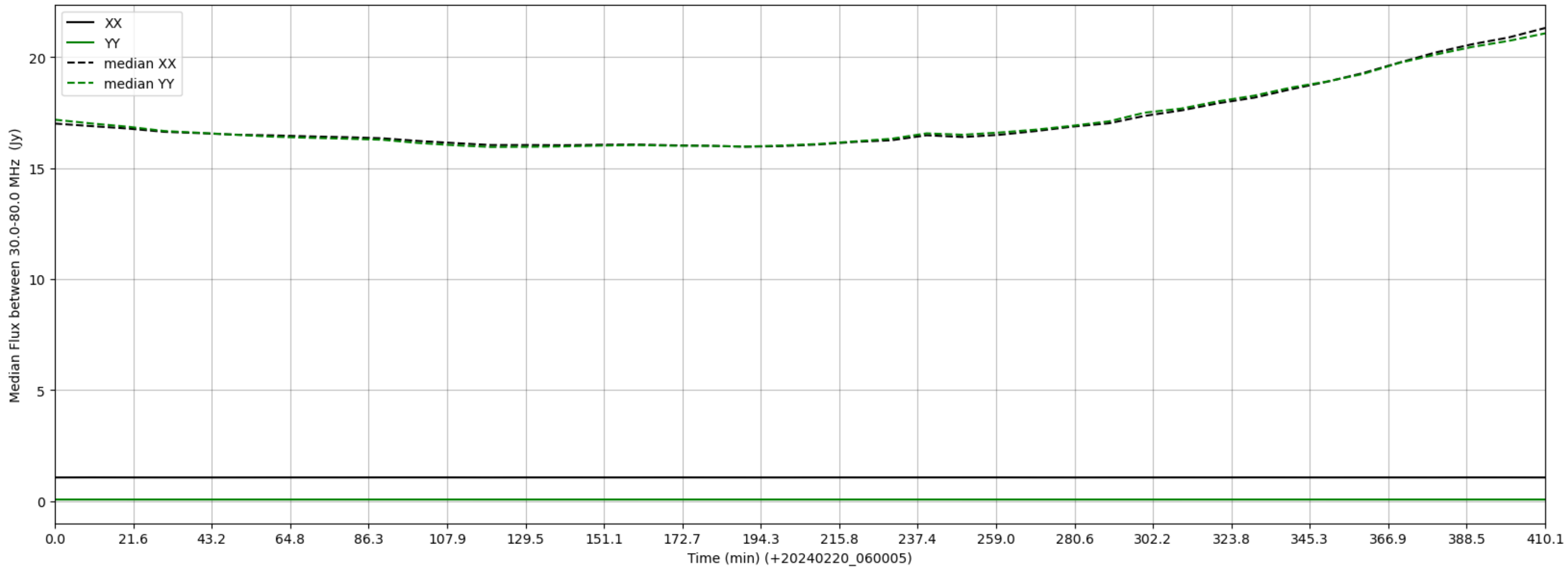
LWA315 - Correlator# 350 - XX FLAGS:LowFlux - YY FLAGS:LowFlux
