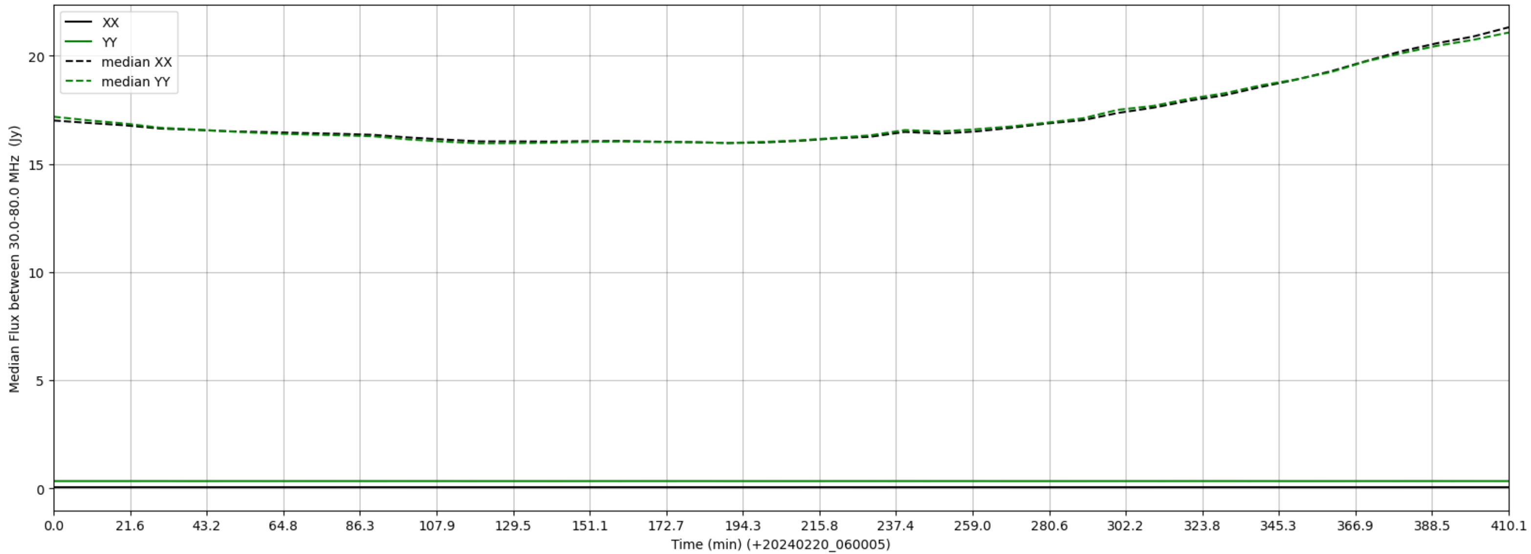
LWA308 - Correlator# 015 - XX FLAGS:LowFlux - YY FLAGS:LowFlux
