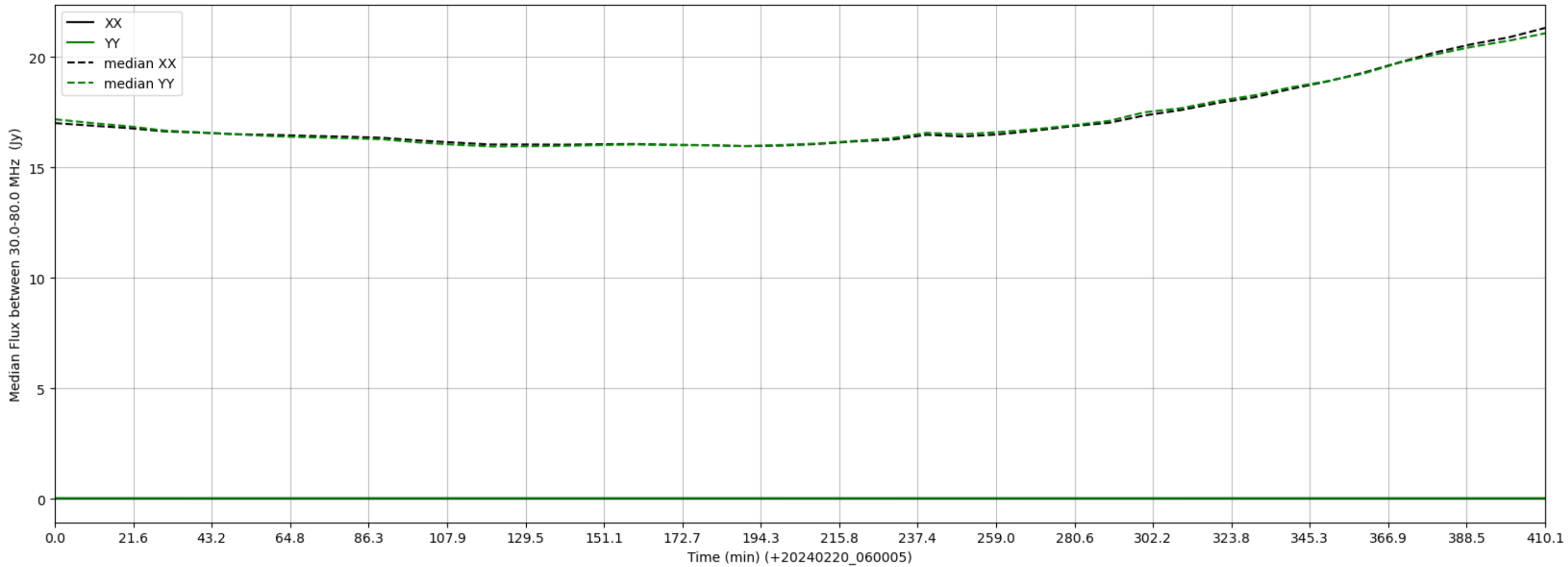
LWA295 - Correlator# 047 - XX FLAGS:LowFlux - YY FLAGS:LowFlux
