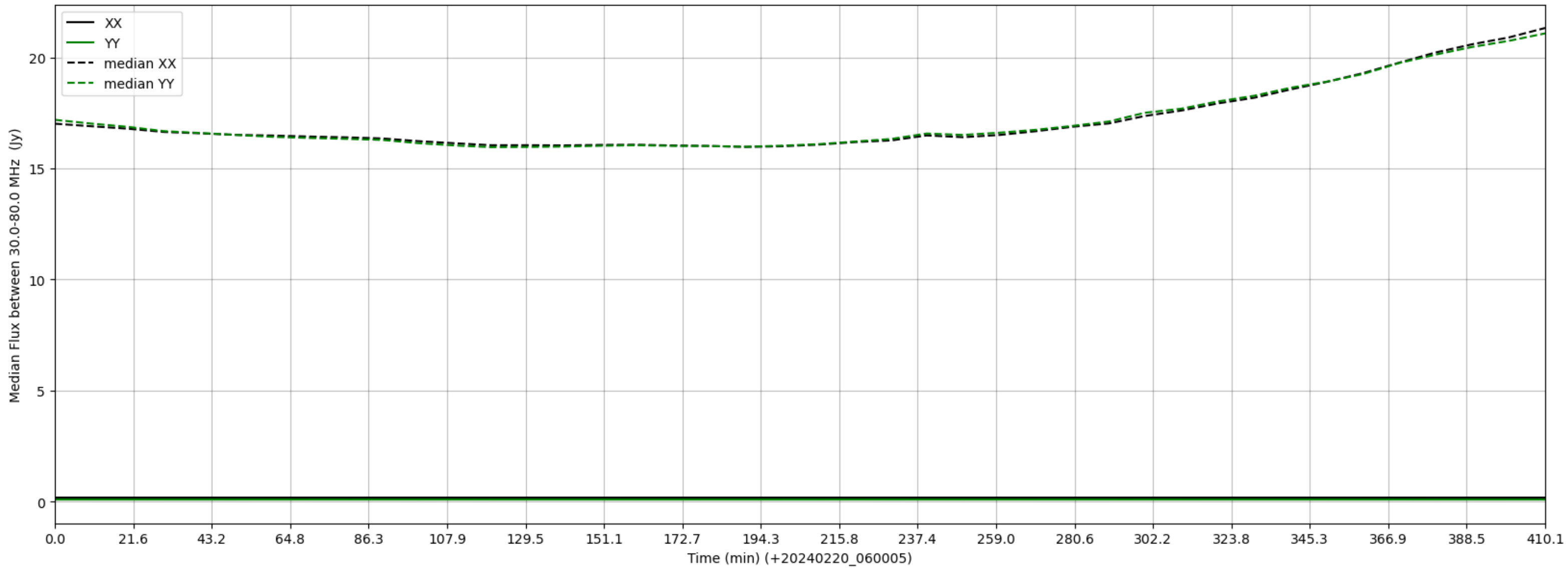
LWA287 - Correlator# 223 - XX FLAGS:LowFlux - YY FLAGS:LowFlux
