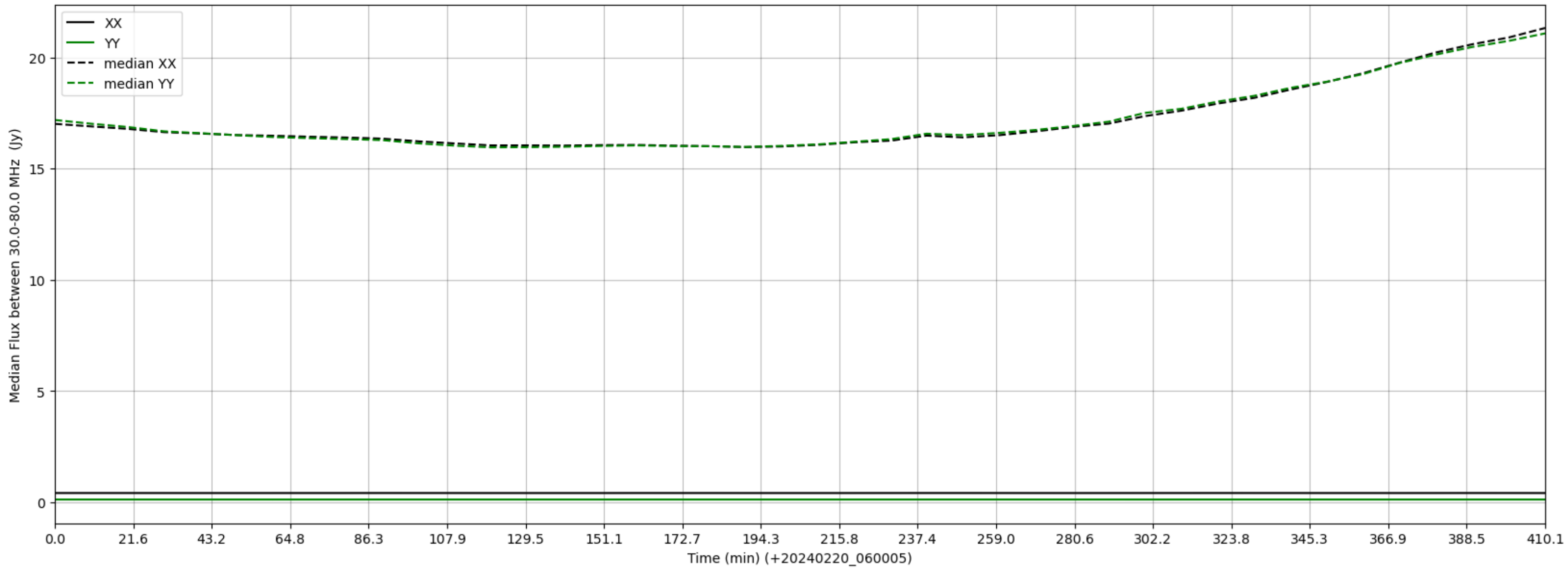
LWA339 - Correlator# 027 - XX FLAGS:LowFlux - YY FLAGS:LowFlux
