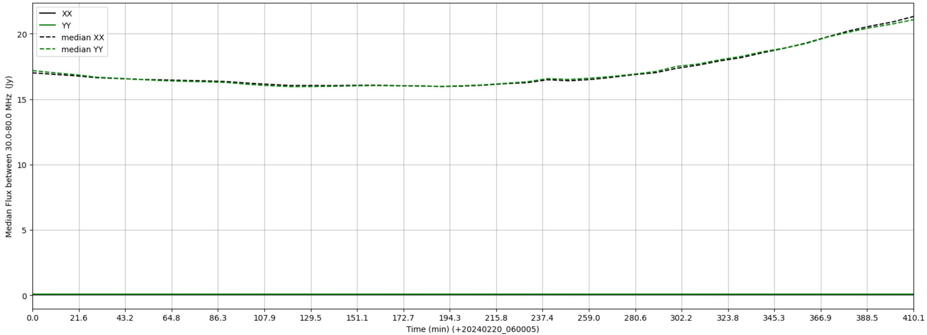
LWA268 - Correlator# 002 - XX FLAGS:LowFlux - YY FLAGS:LowFlux
