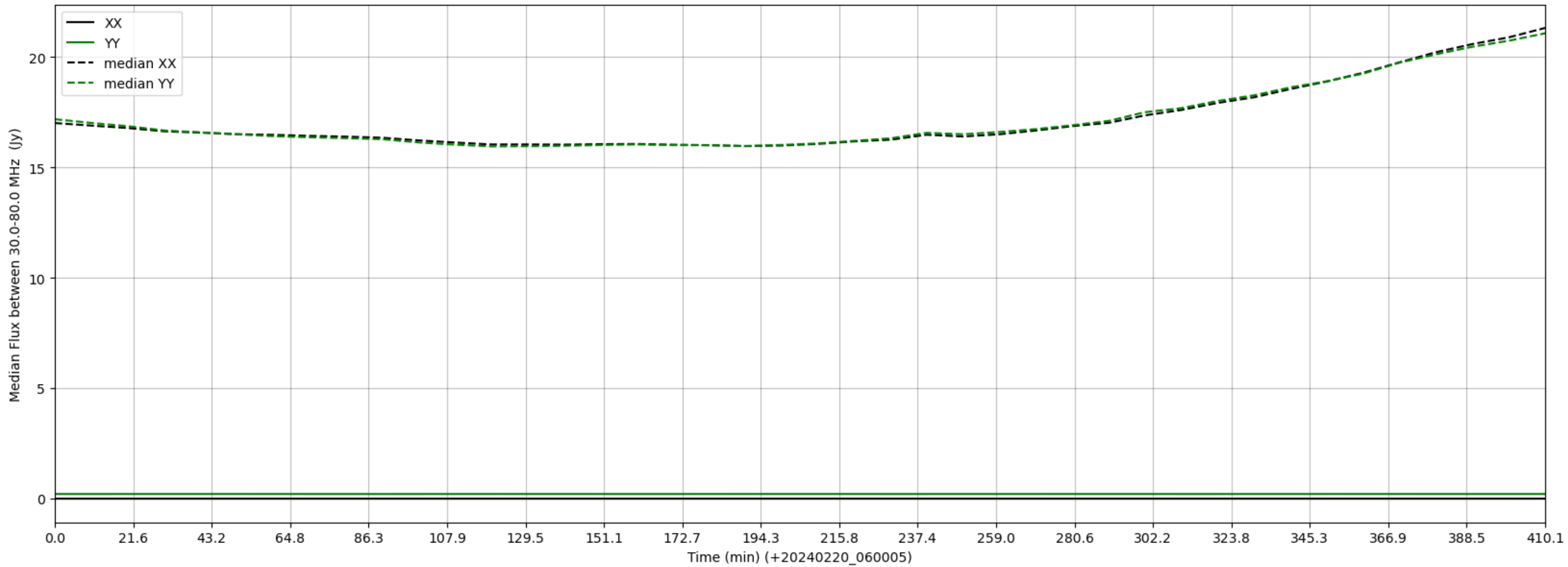
LWA348 - Correlator# 124 - XX FLAGS:LowFlux - YY FLAGS:LowFlux
