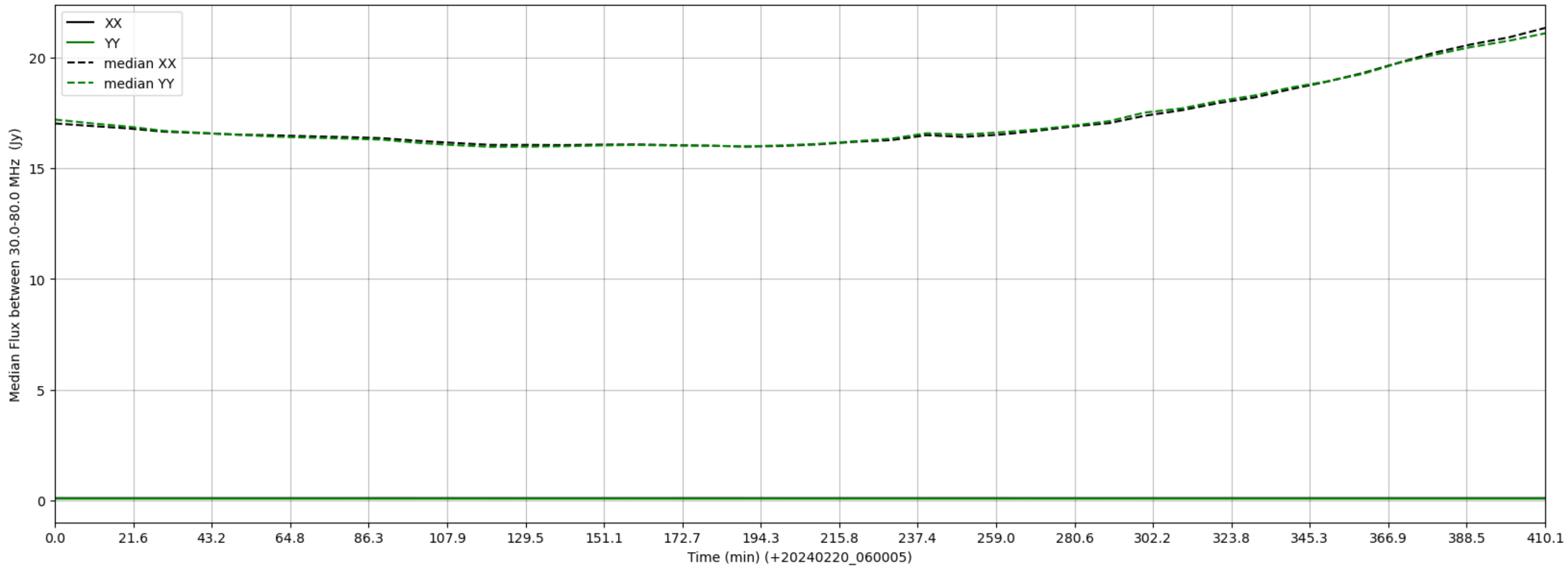
LWA334 - Correlator# 156 - XX FLAGS:LowFlux - YY FLAGS:LowFlux
