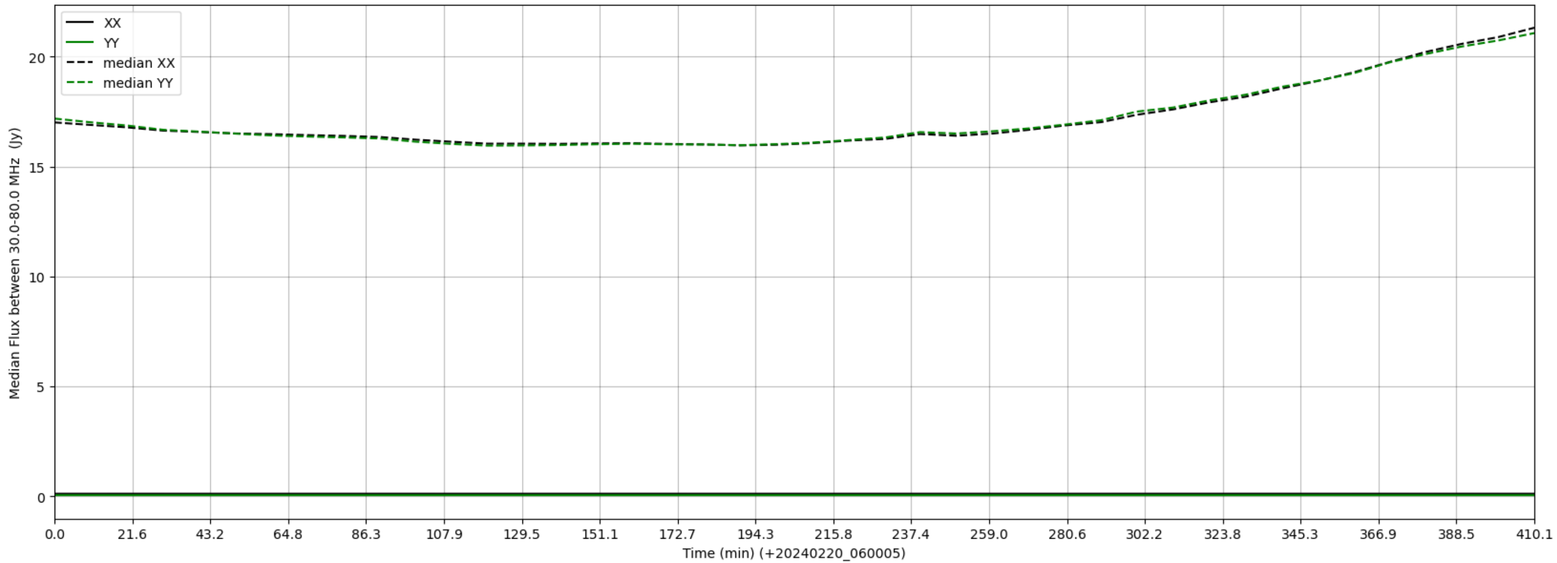
LWA351 - Correlator# 060 - XX FLAGS:LowFlux - YY FLAGS:LowFlux
