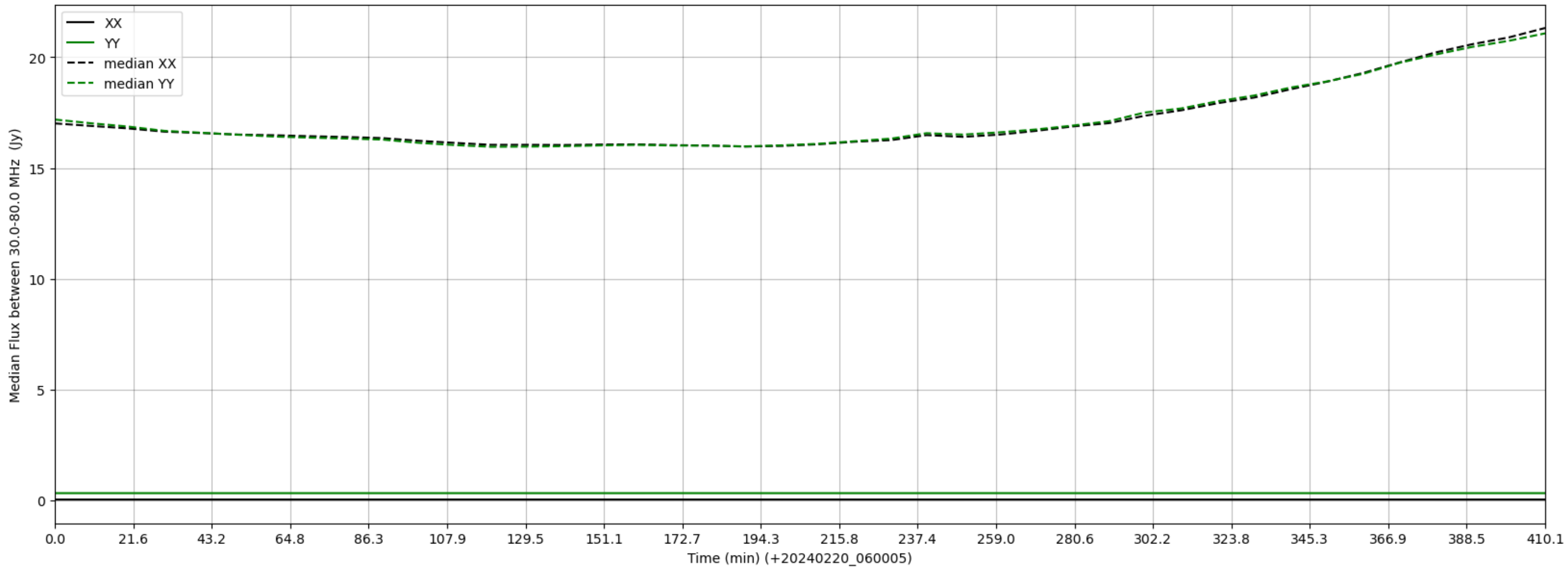
LWA332 - Correlator# 025 - XX FLAGS:LowFlux - YY FLAGS:LowFlux
