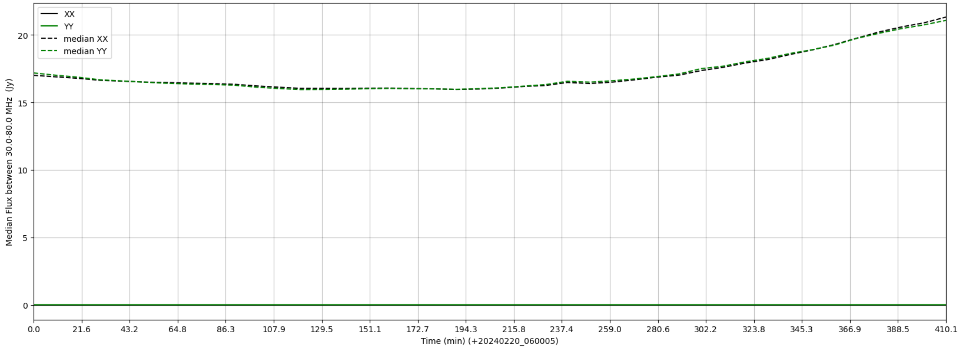
LWA352 - Correlator# 028 - XX FLAGS:LowFlux - YY FLAGS:LowFlux
