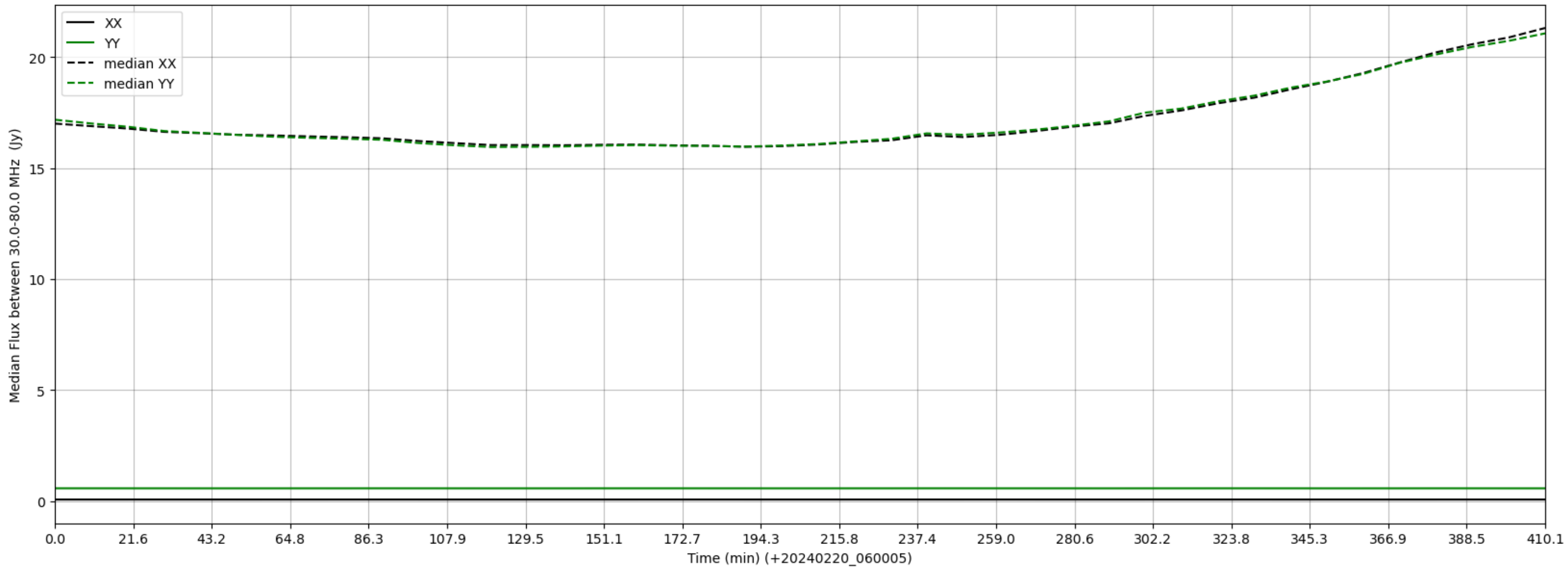
LWA269 - Correlator# 005 - XX FLAGS:LowFlux - YY FLAGS:LowFlux
