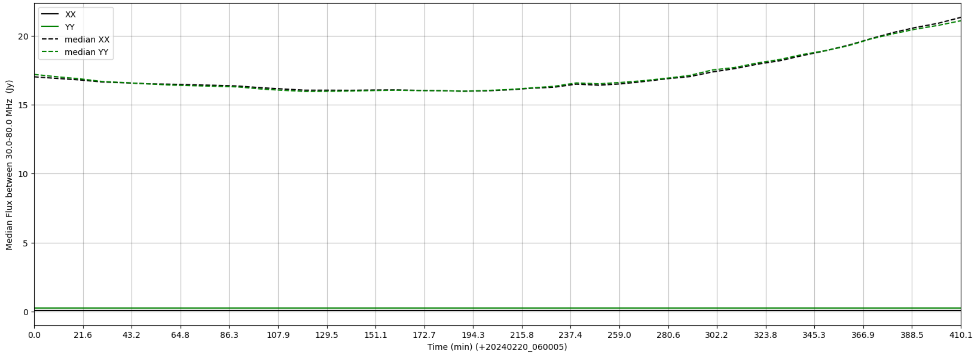
LWA337 - Correlator# 059 - XX FLAGS:LowFlux - YY FLAGS:LowFlux
