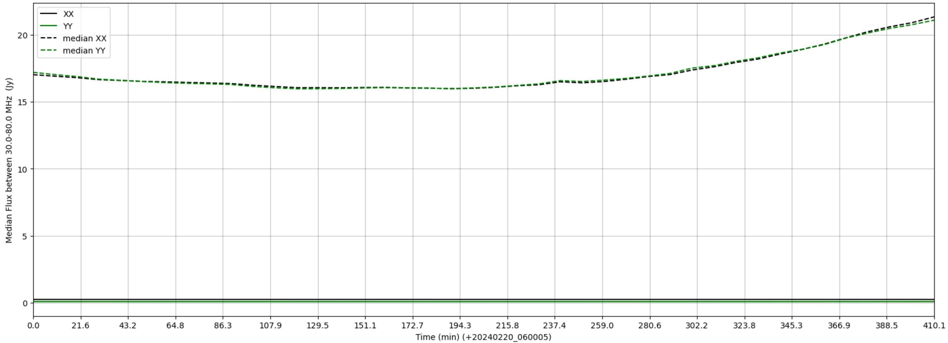
LWA329 - Correlator# 287 - XX FLAGS:LowFlux - YY FLAGS:LowFlux
