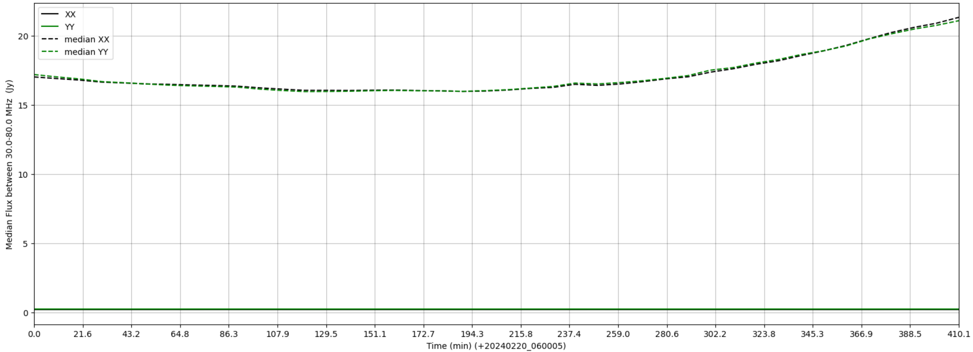
LWA312 - Correlator# 019 - XX FLAGS:LowFlux - YY FLAGS:LowFlux
