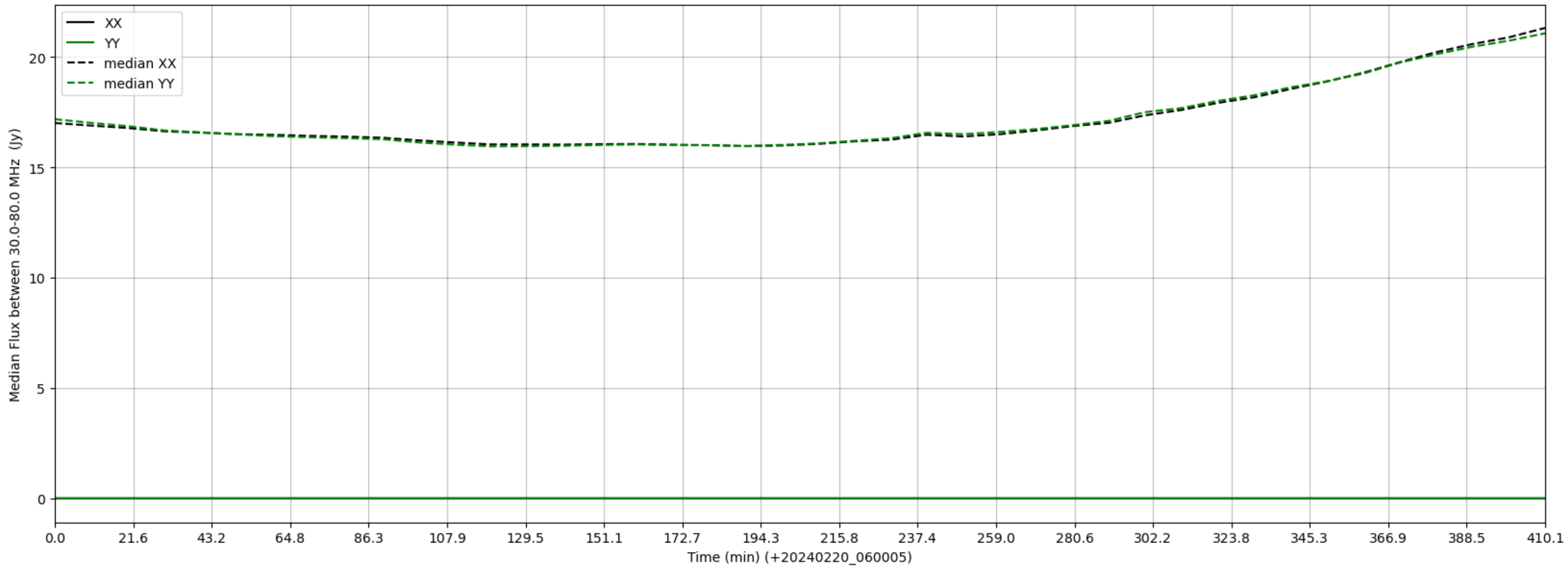
LWA307 - Correlator# 012 - XX FLAGS:LowFlux - YY FLAGS:LowFlux
