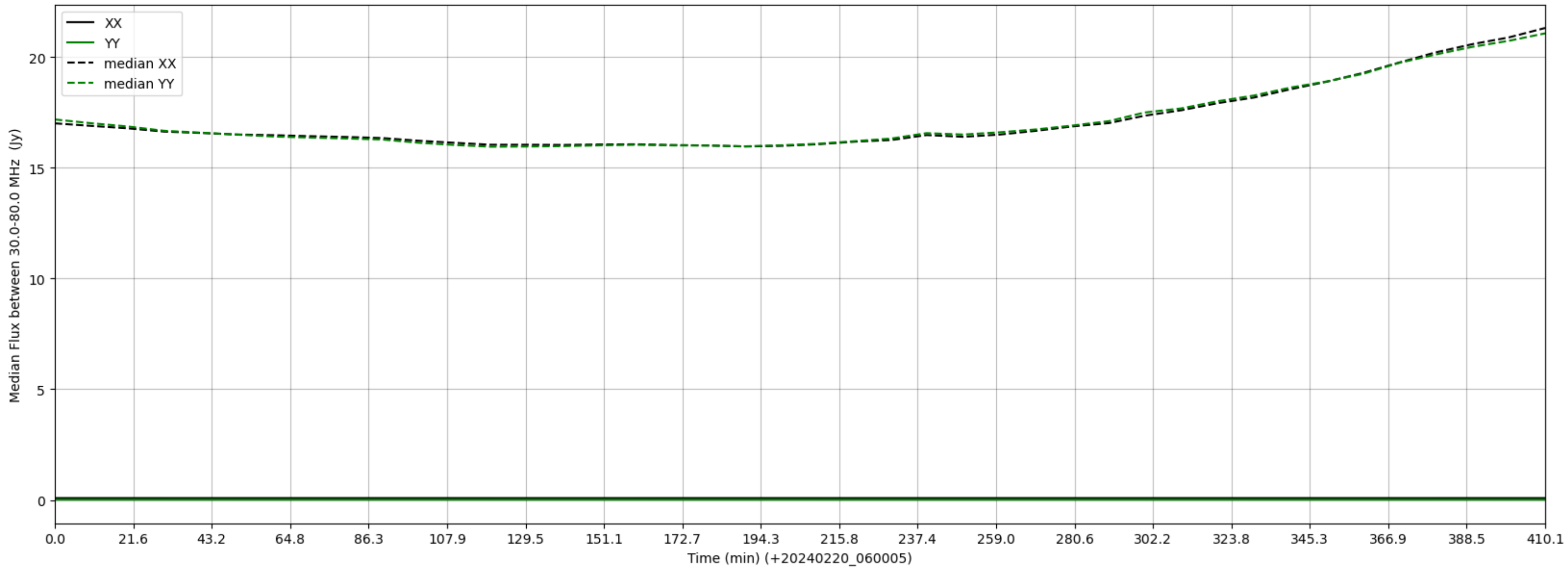
LWA341 - Correlator# 029 - XX FLAGS:LowFlux - YY FLAGS:LowFlux
