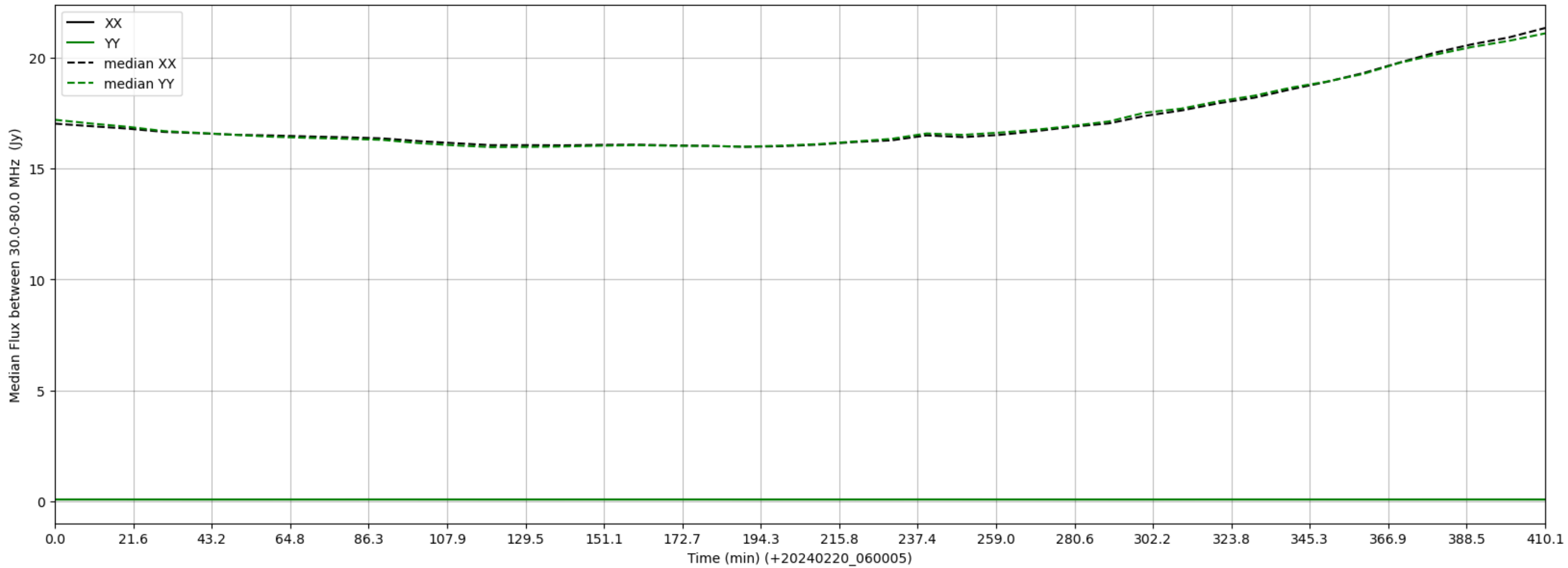
LWA349 - Correlator# 282 - XX FLAGS:LowFlux - YY FLAGS:LowFlux
