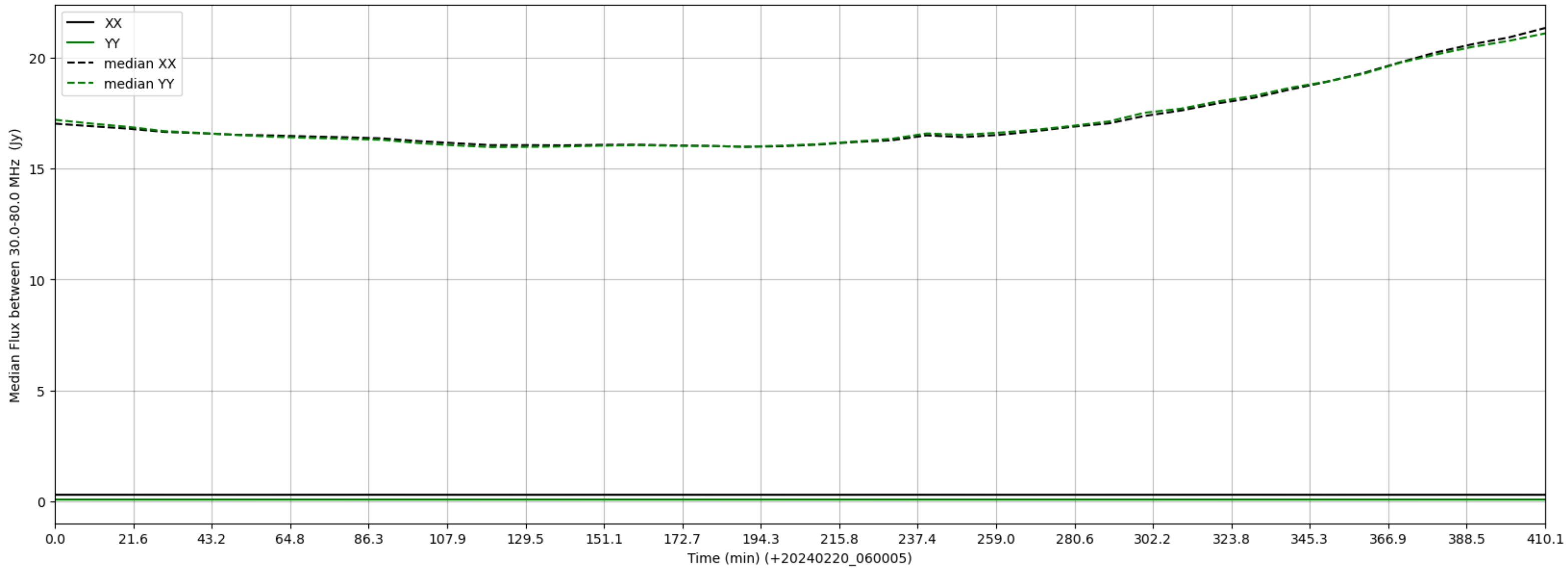
LWA330 - Correlator# 022 - XX FLAGS:LowFlux - YY FLAGS:LowFlux
