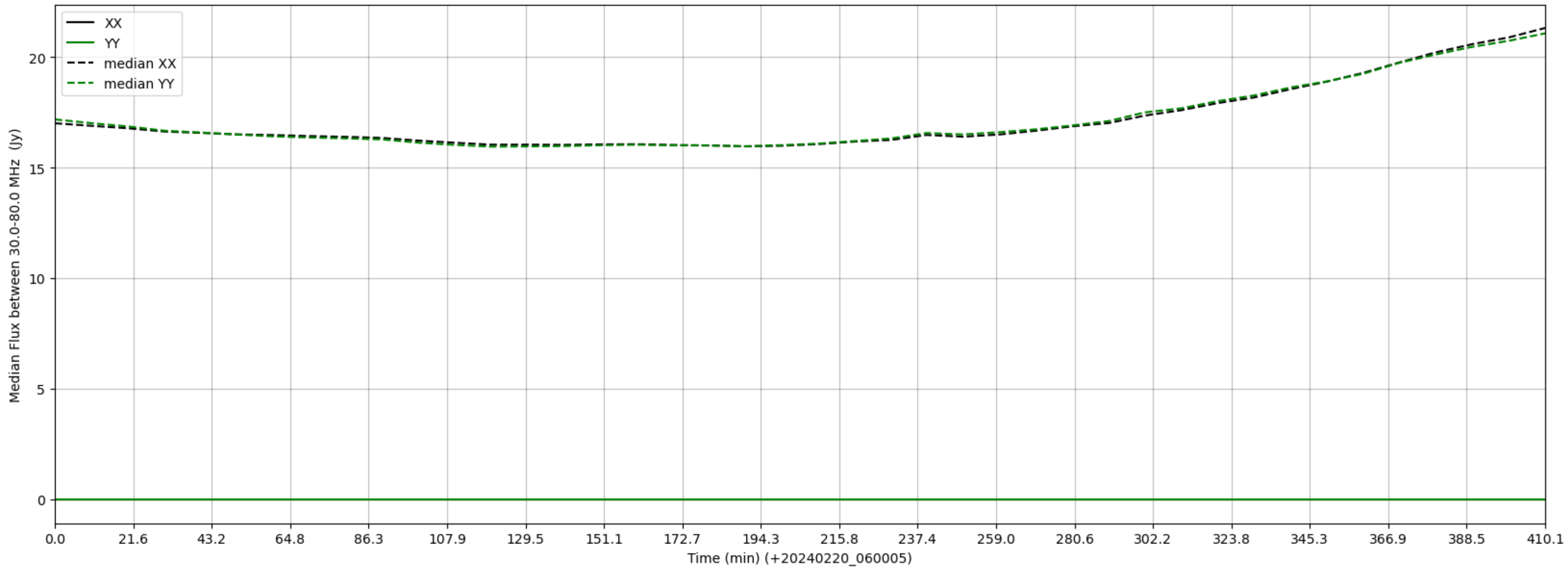
LWA314 - Correlator# 021 - XX FLAGS:LowFlux - YY FLAGS:LowFlux
