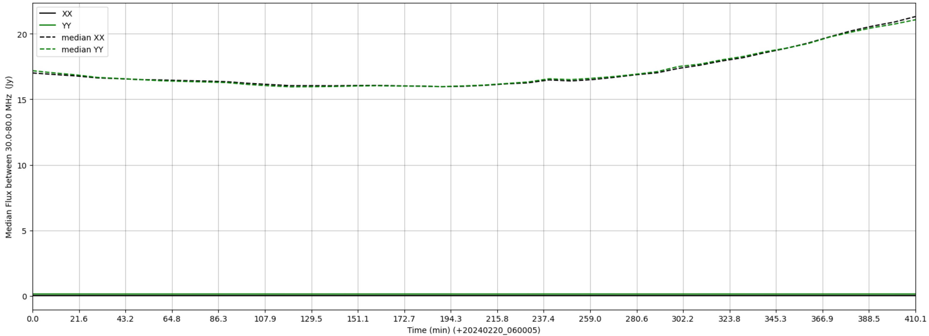
LWA296 - Correlator# 046 - XX FLAGS:LowFlux - YY FLAGS:LowFlux
