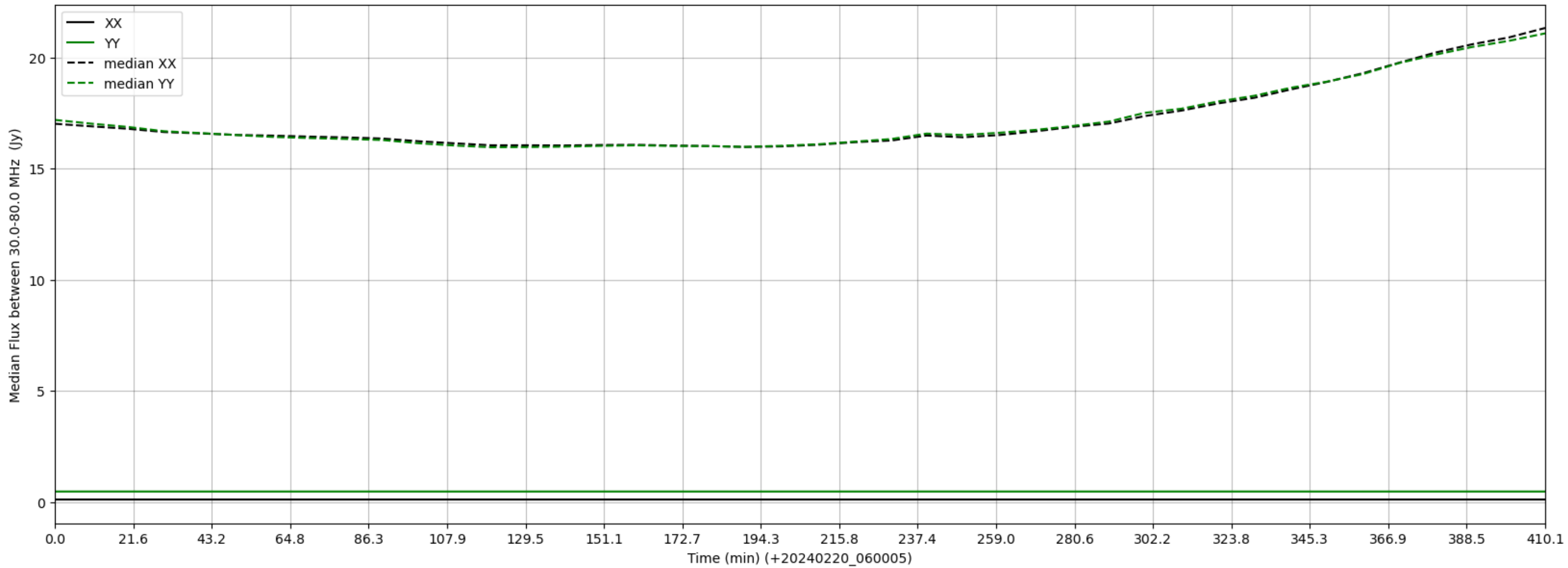
LWA342 - Correlator# 317 - XX FLAGS:LowFlux - YY FLAGS:LowFlux
