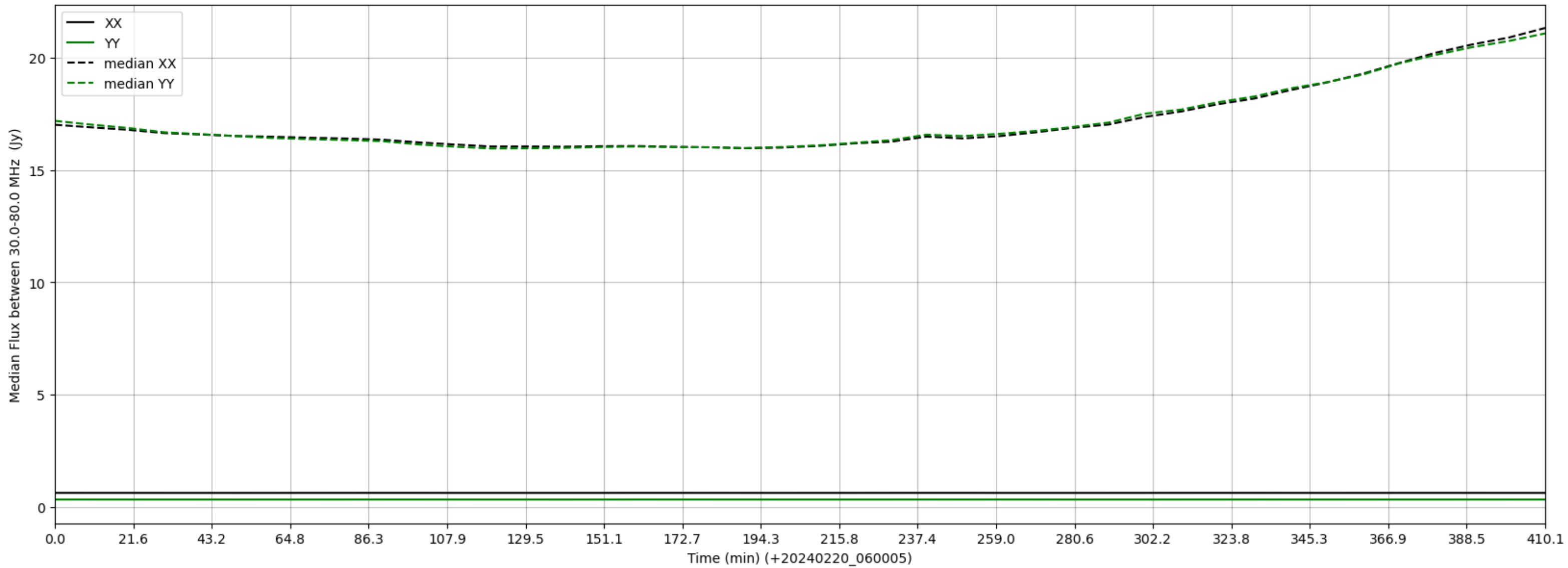
LWA321 - Correlator# 020 - XX FLAGS:LowFlux - YY FLAGS:LowFlux
