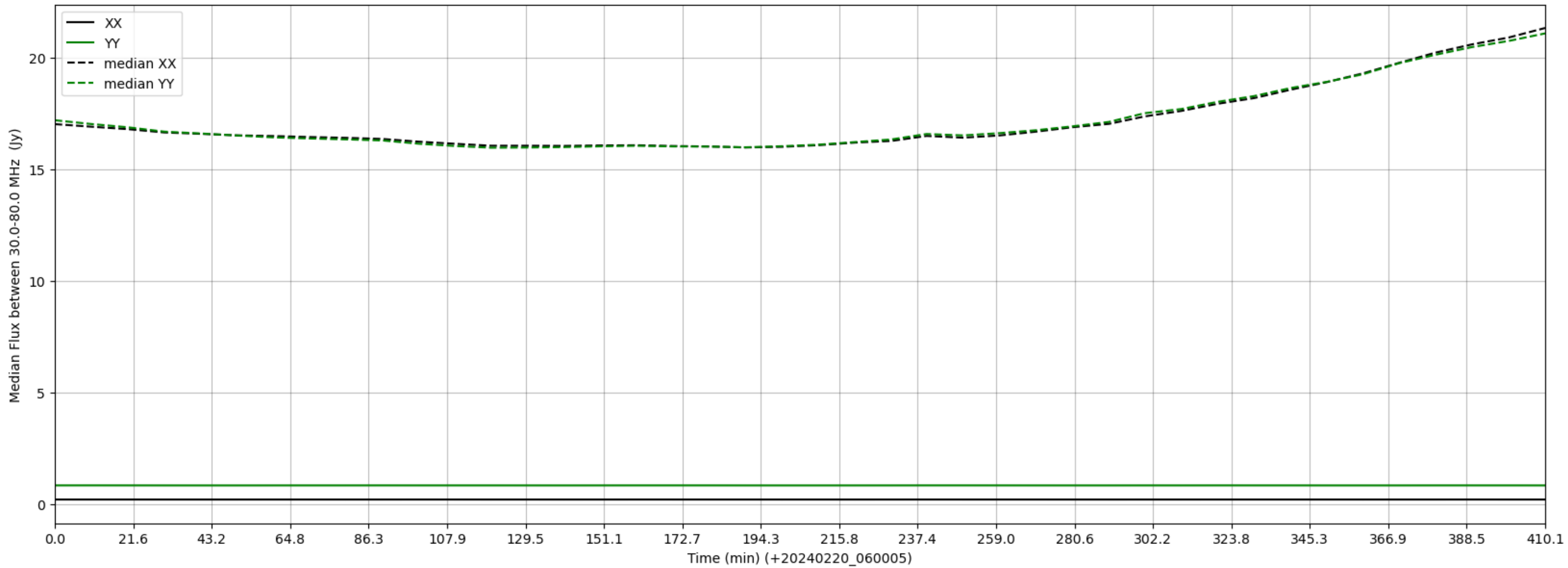
LWA328 - Correlator# 157 - XX FLAGS:LowFlux - YY FLAGS:LowFlux
