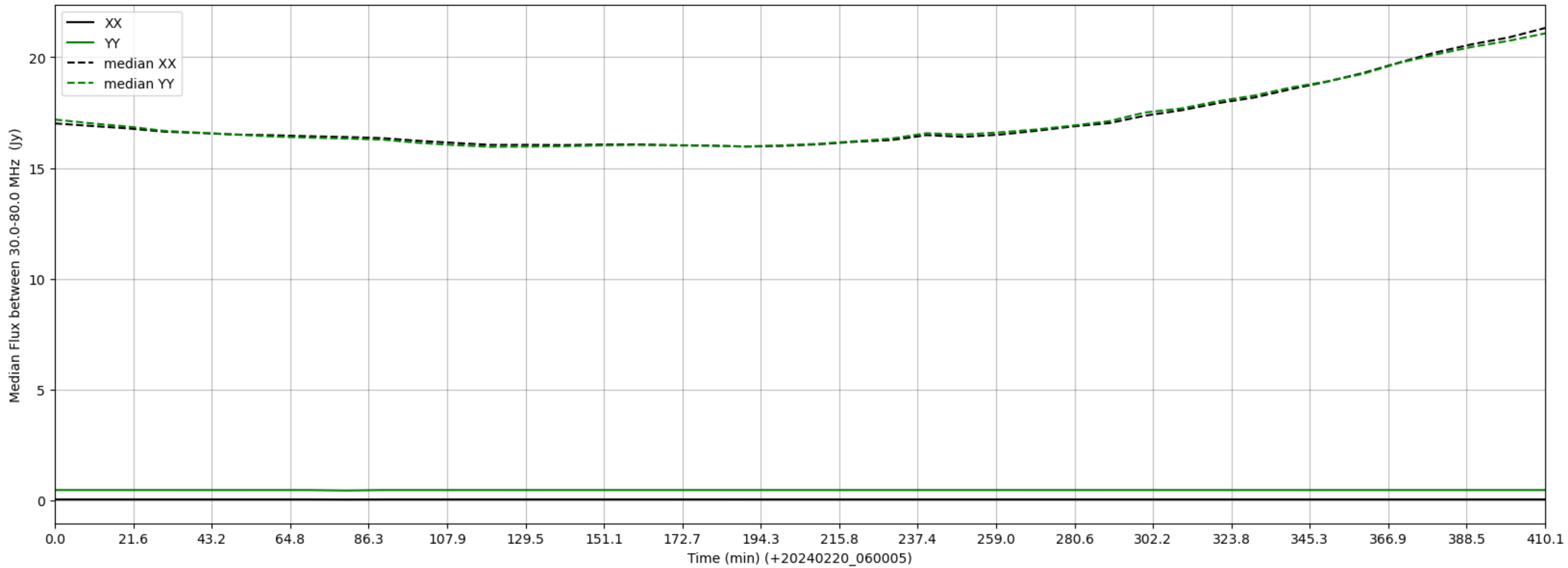
LWA344 - Correlator# 061 - XX FLAGS:LowFlux - YY FLAGS:LowFlux
