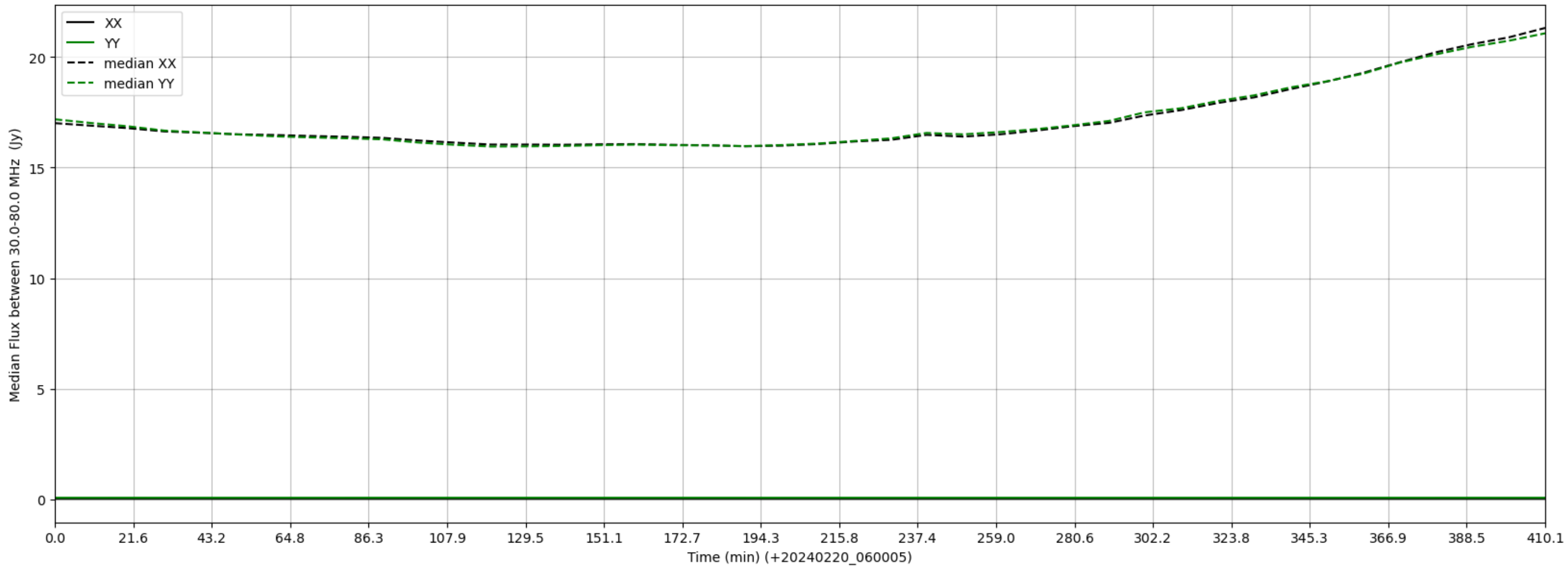
LWA278 - Correlator# 008 - XX FLAGS:LowFlux - YY FLAGS:LowFlux
