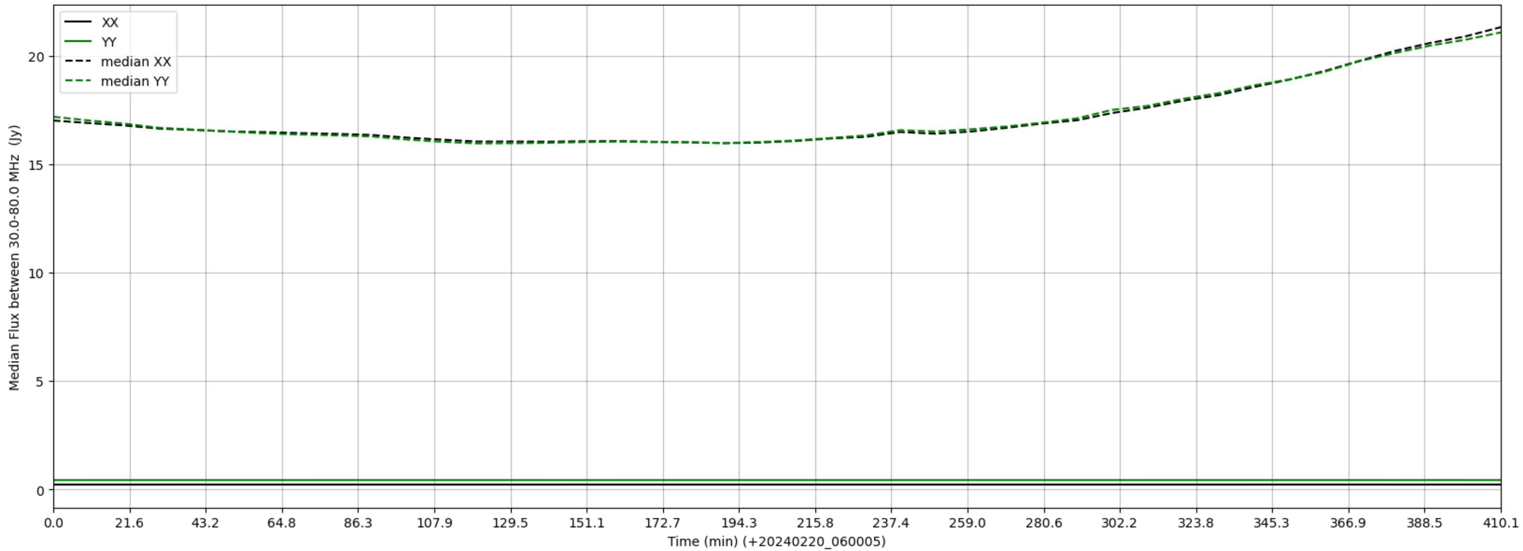
LWA275 - Correlator# 090 - XX FLAGS:LowFlux - YY FLAGS:LowFlux
