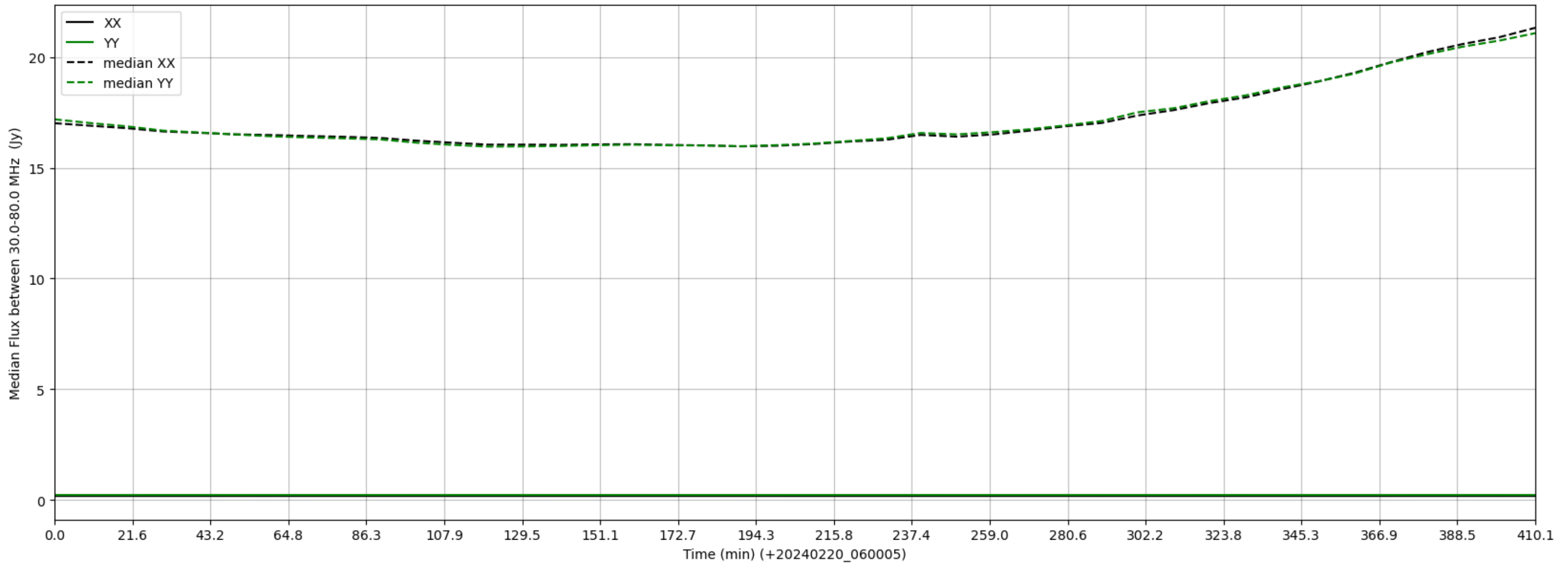
LWA327 - Correlator# 023 - XX FLAGS:LowFlux - YY FLAGS:LowFlux
