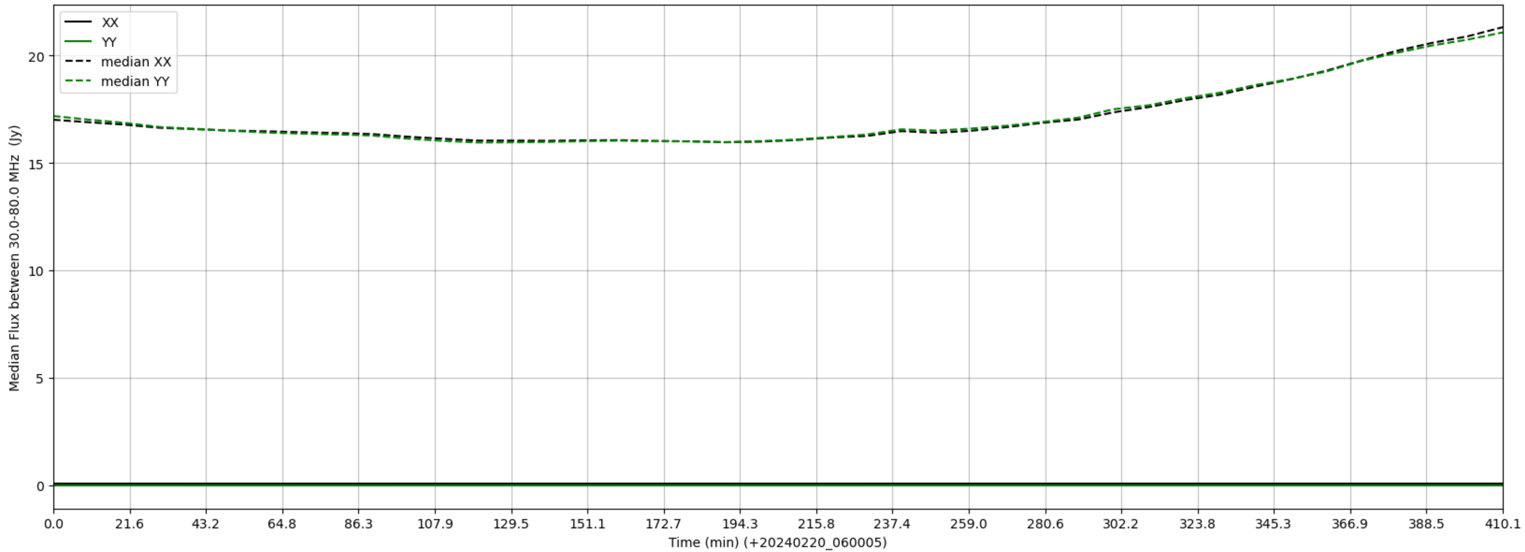
LWA292 - Correlator# 044 - XX FLAGS:LowFlux - YY FLAGS:LowFlux
