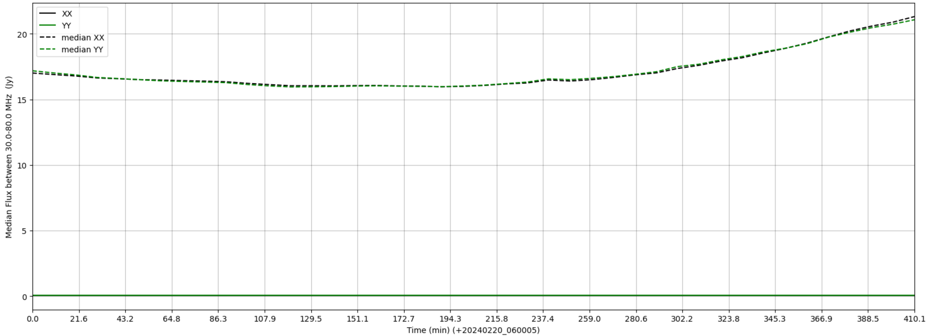
LWA336 - Correlator# 056 - XX FLAGS:LowFlux - YY FLAGS:LowFlux
