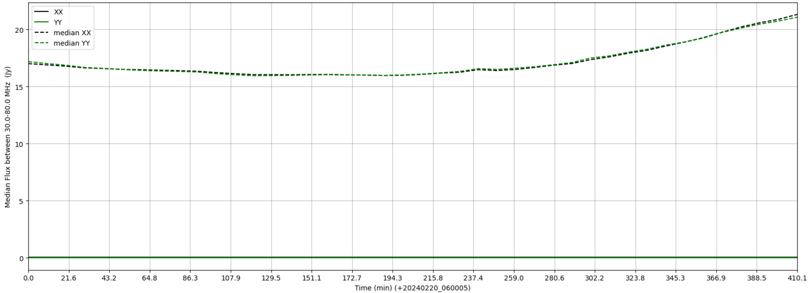
LWA284 - Correlator# 043 - XX FLAGS:LowFlux - YY FLAGS:LowFlux
