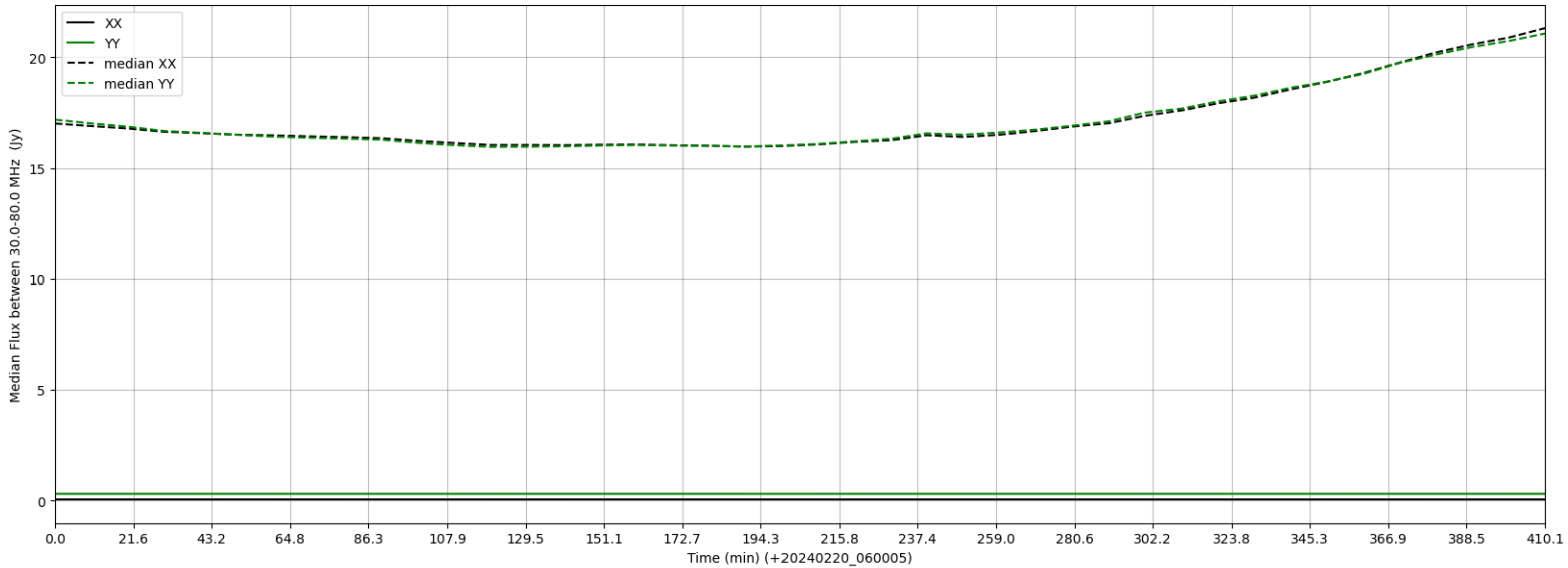
LWA259 - Correlator# 001 - XX FLAGS:LowFlux - YY FLAGS:LowFlux
