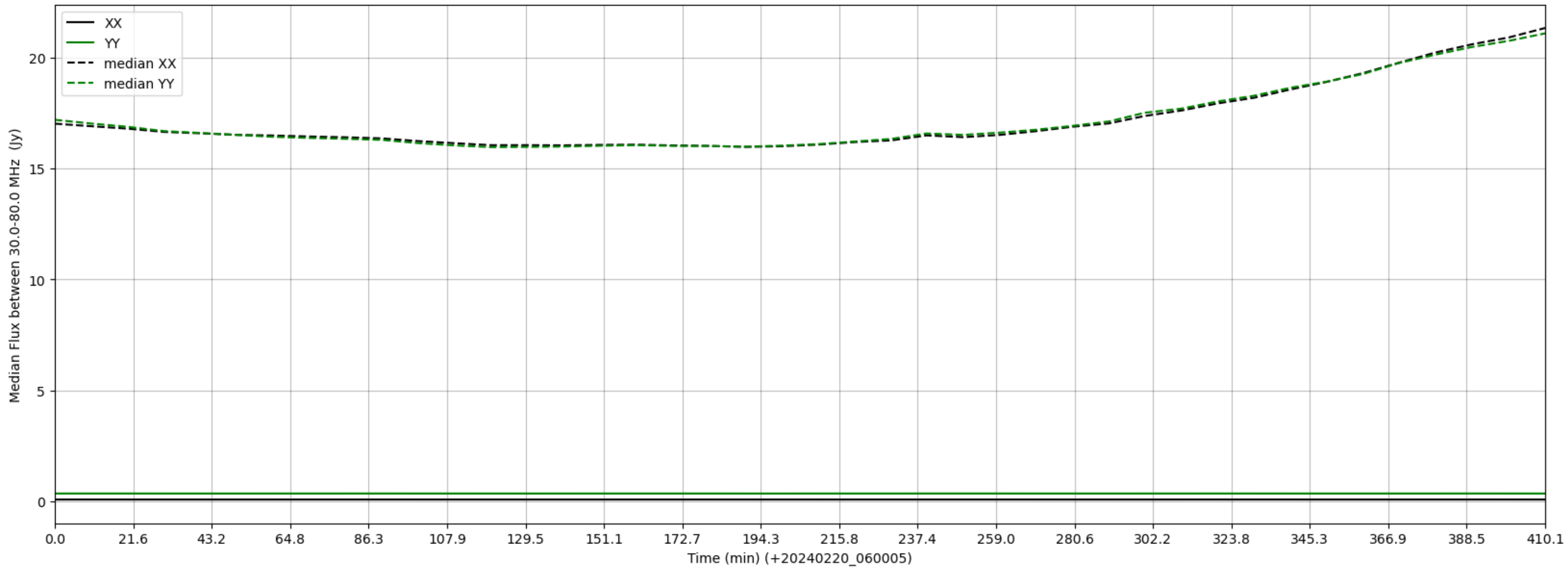
LWA290 - Correlator# 285 - XX FLAGS:LowFlux - YY FLAGS:LowFlux
