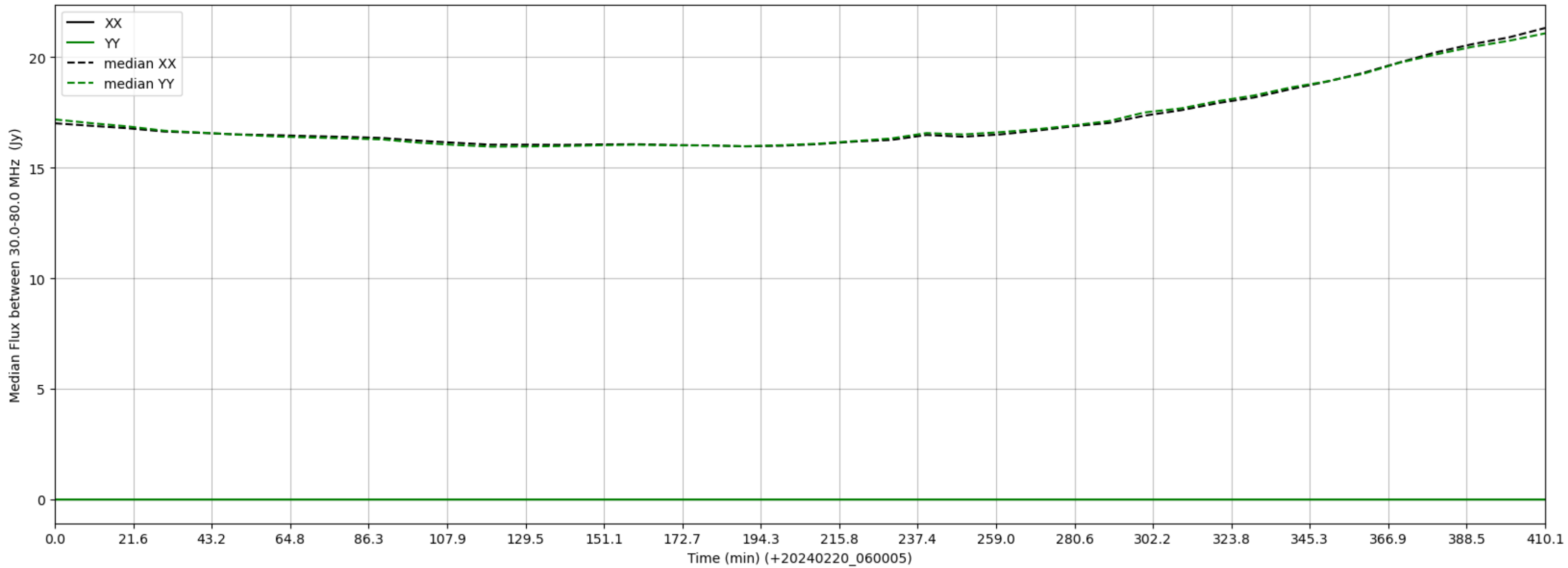
LWA260 - Correlator# 034 - XX FLAGS:LowFlux - YY FLAGS:LowFlux
