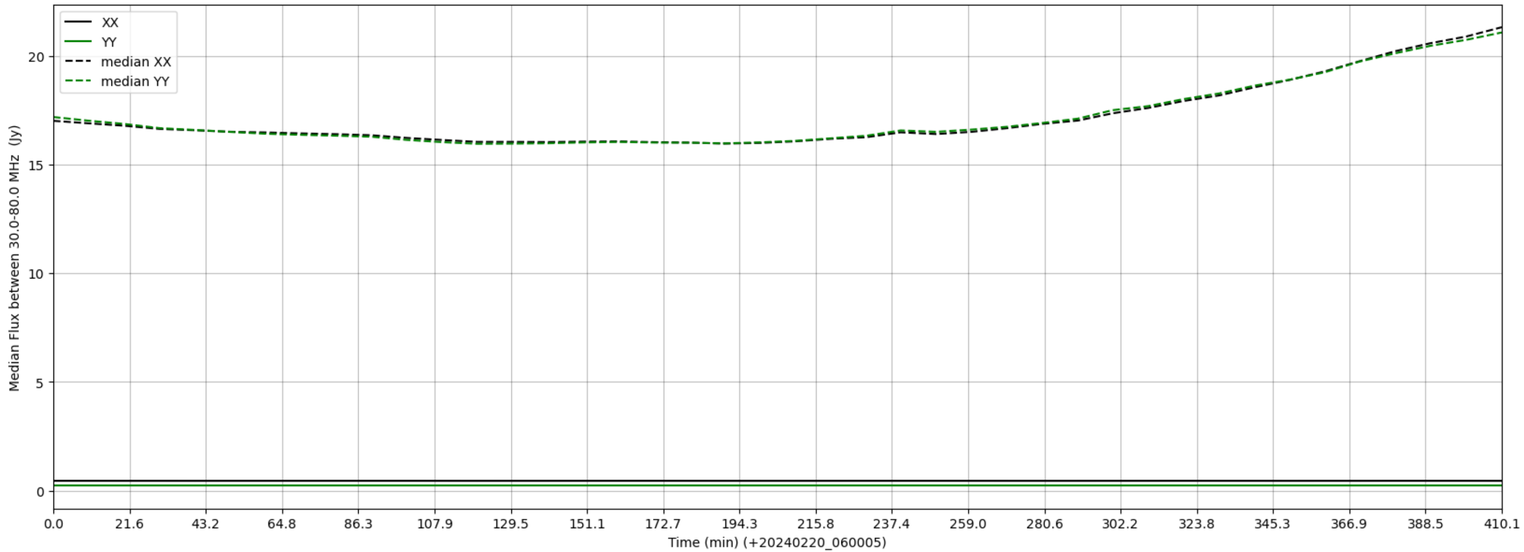
LWA333 - Correlator# 253 - XX FLAGS:LowFlux - YY FLAGS:LowFlux
