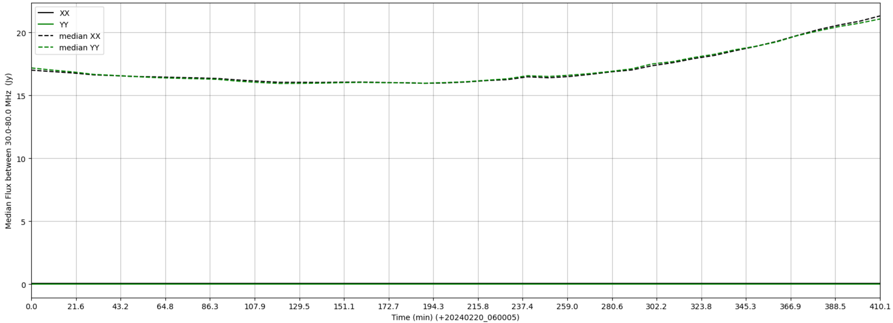
LWA273 - Correlator# 007 - XX FLAGS:LowFlux - YY FLAGS:LowFlux
