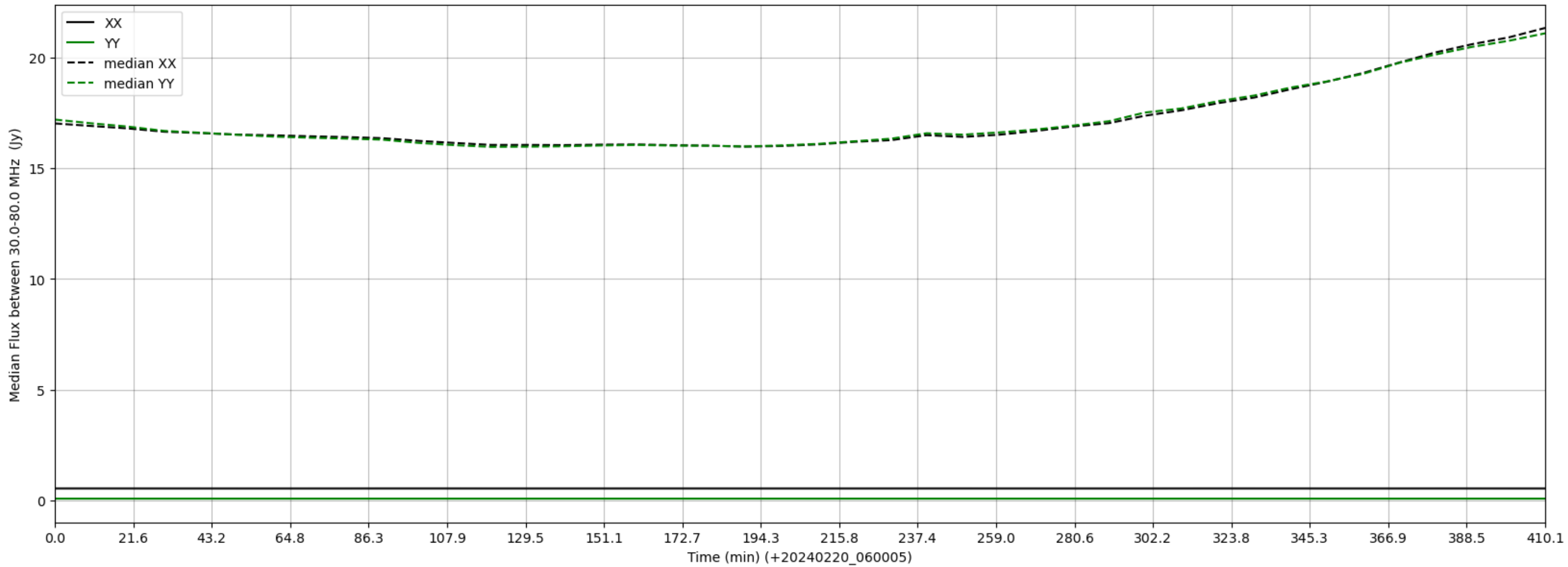
LWA264 - Correlator# 349 - XX FLAGS:LowFlux - YY FLAGS:LowFlux
