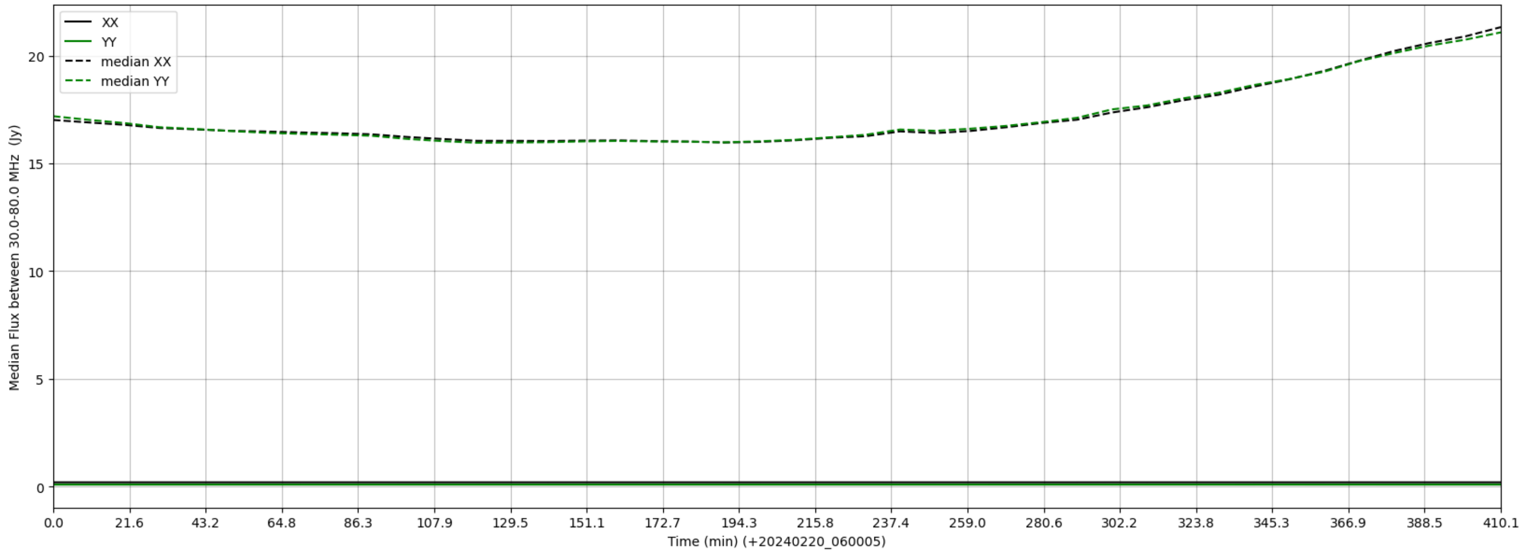
LWA320 - Correlator# 054 - XX FLAGS:LowFlux - YY FLAGS:LowFlux
