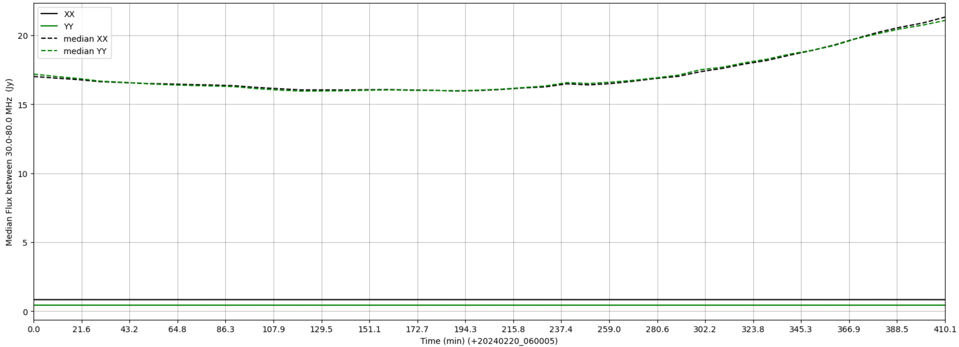
LWA286 - Correlator# 093 - XX FLAGS:LowFlux - YY FLAGS:LowFlux
