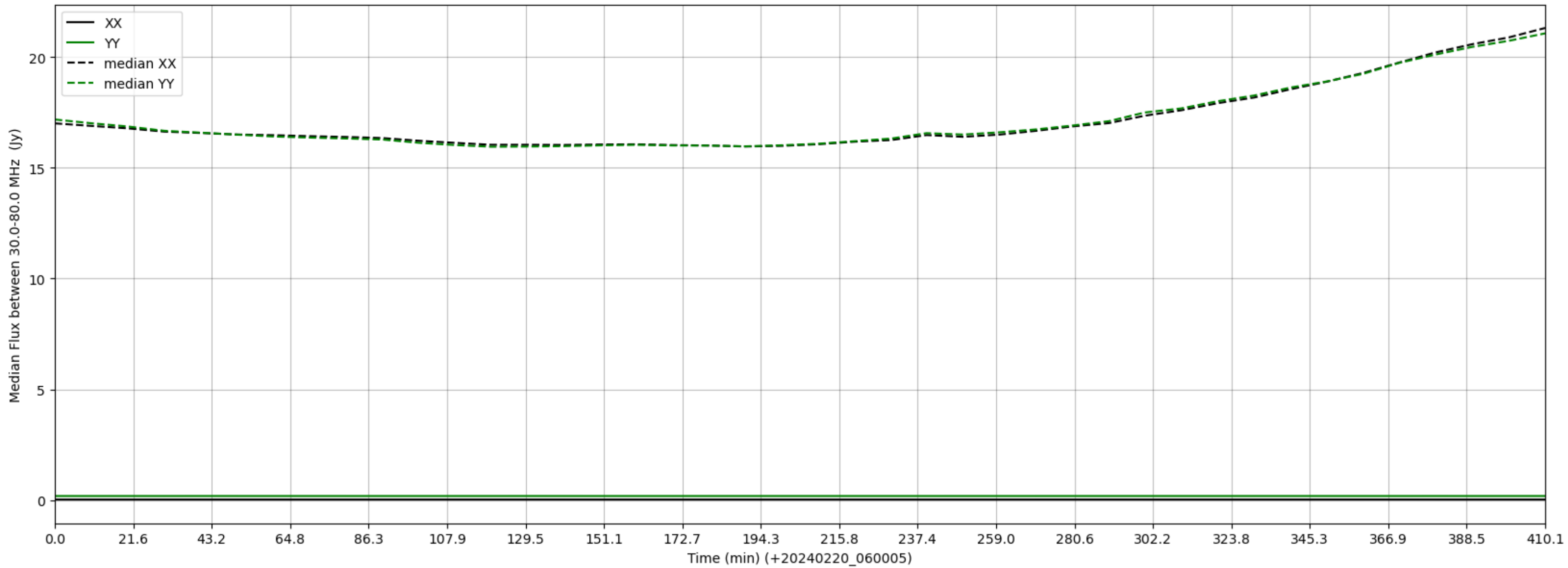
LWA289 - Correlator# 189 - XX FLAGS:LowFlux - YY FLAGS:LowFlux
