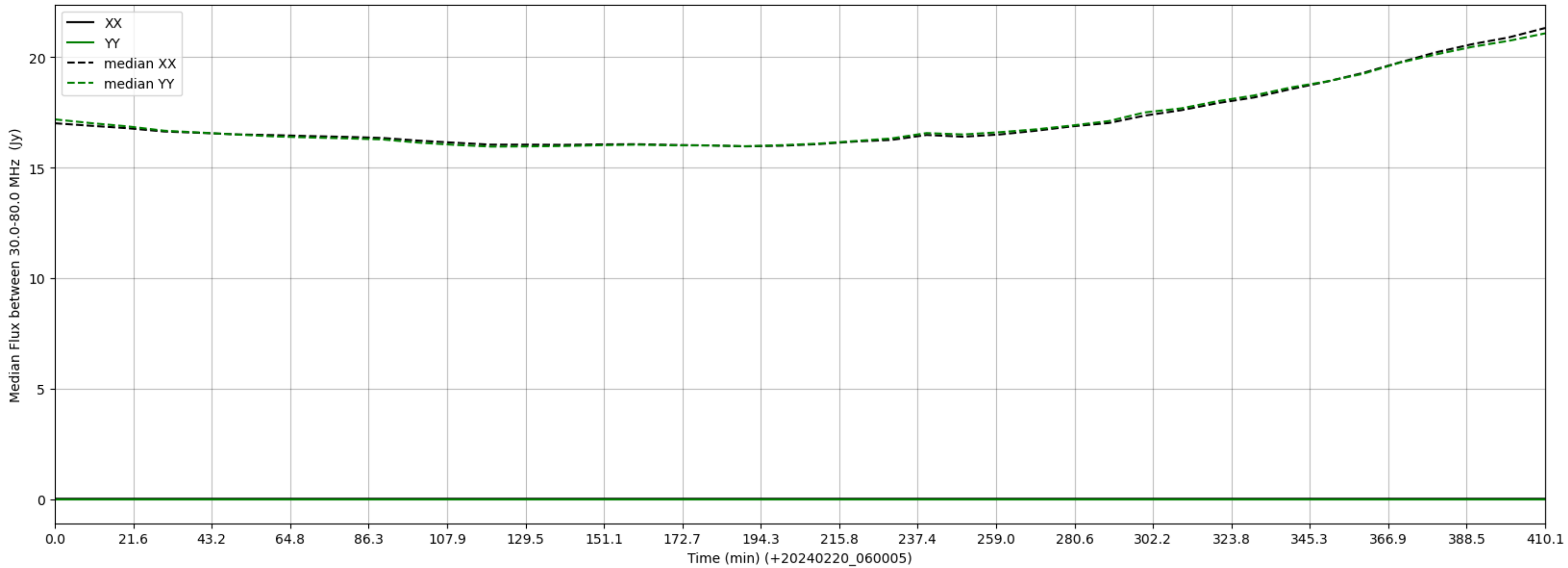
LWA325 - Correlator# 154 - XX FLAGS:LowFlux - YY FLAGS:LowFlux
