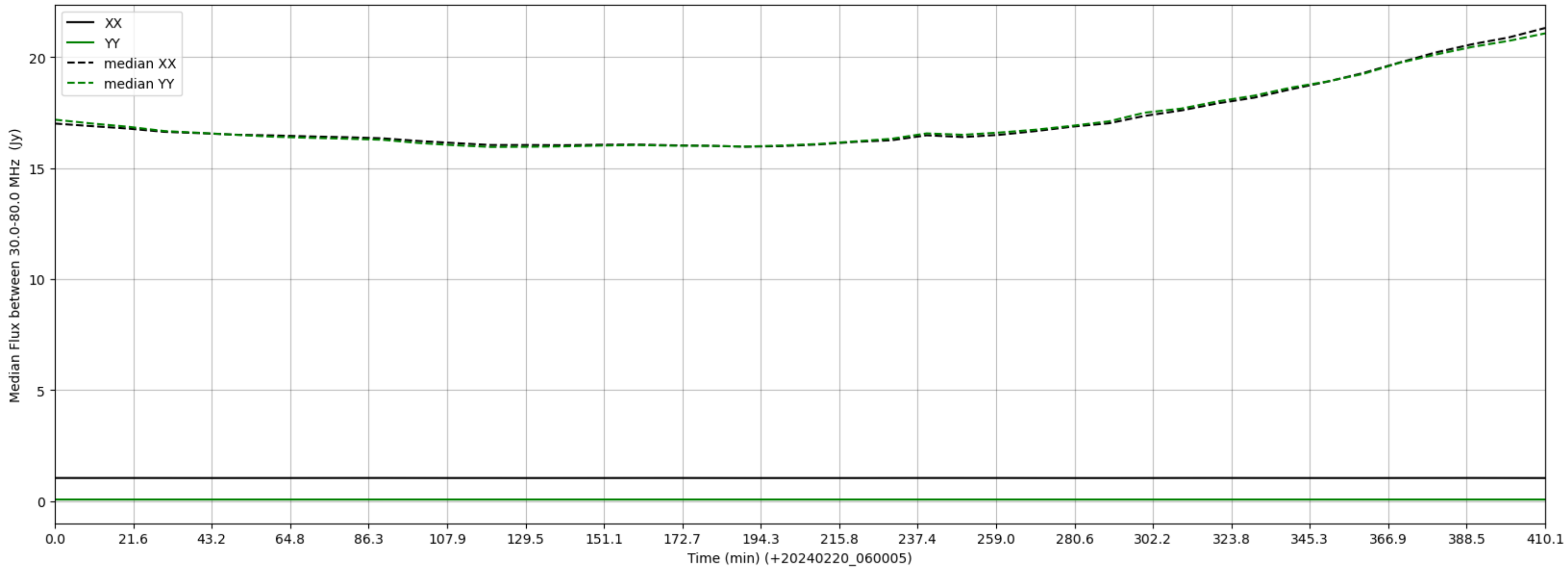
LWA313 - Correlator# 018 - XX FLAGS:LowFlux - YY FLAGS:LowFlux
