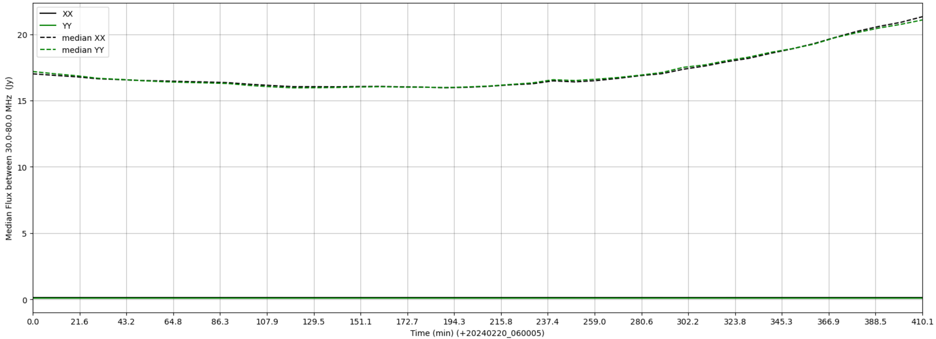
LWA350 - Correlator# 319 - XX FLAGS:LowFlux - YY FLAGS:LowFlux
