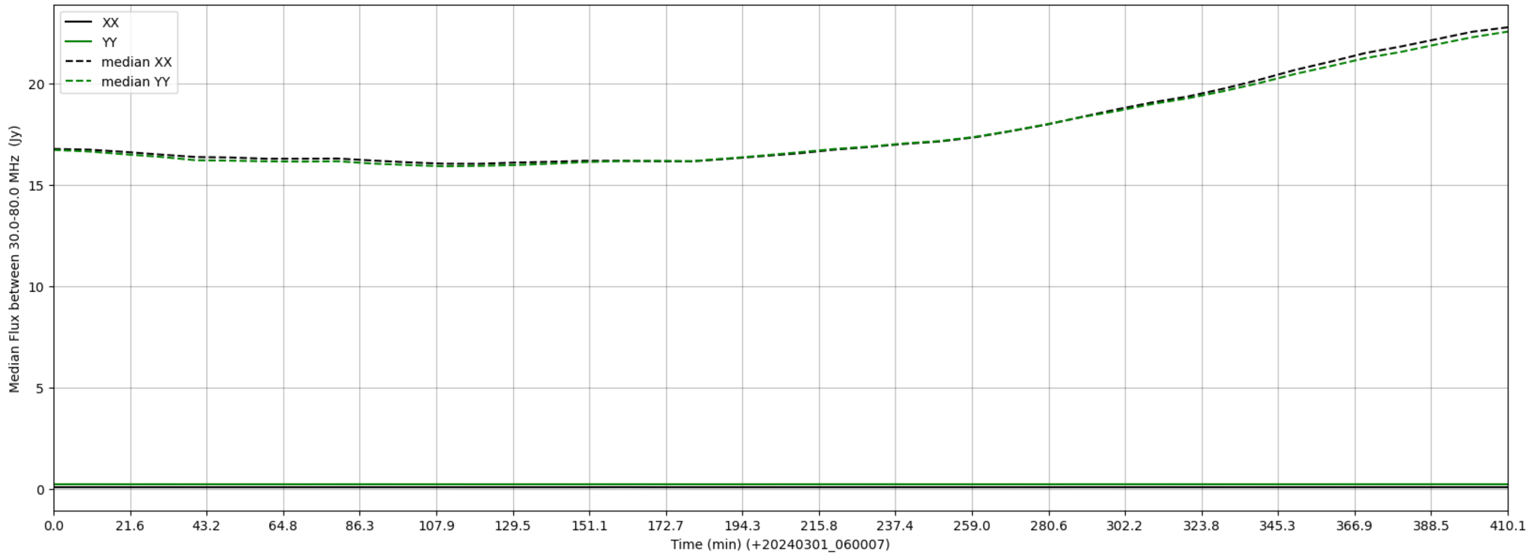
LWA297 - Correlator# 314 - XX FLAGS:LowFlux - YY FLAGS:LowFlux
