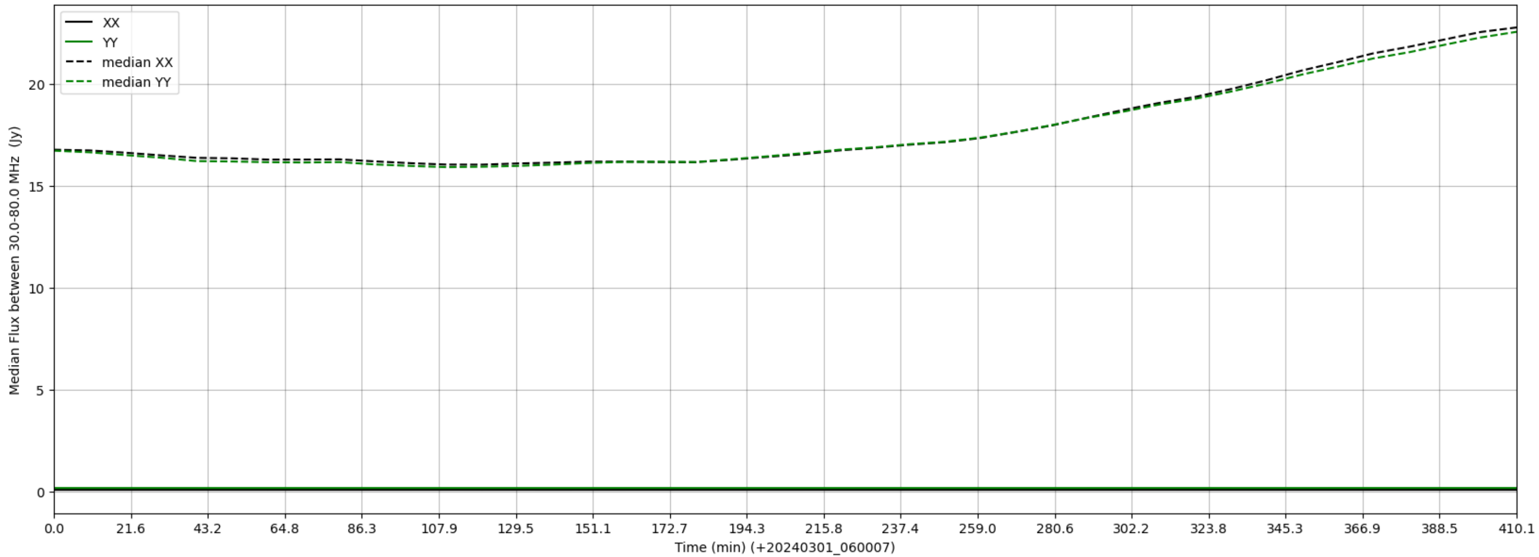
LWA298 - Correlator# 049 - XX FLAGS:LowFlux - YY FLAGS:LowFlux
