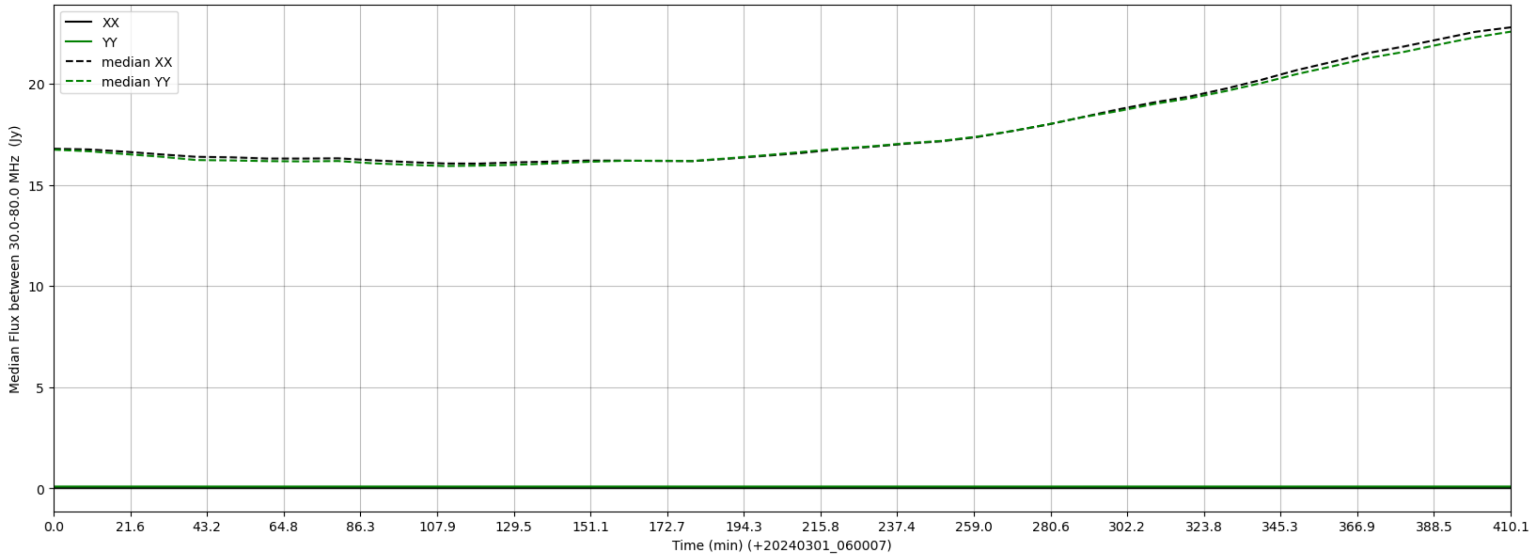
LWA261 - Correlator# 346 - XX FLAGS:LowFlux - YY FLAGS:LowFlux
