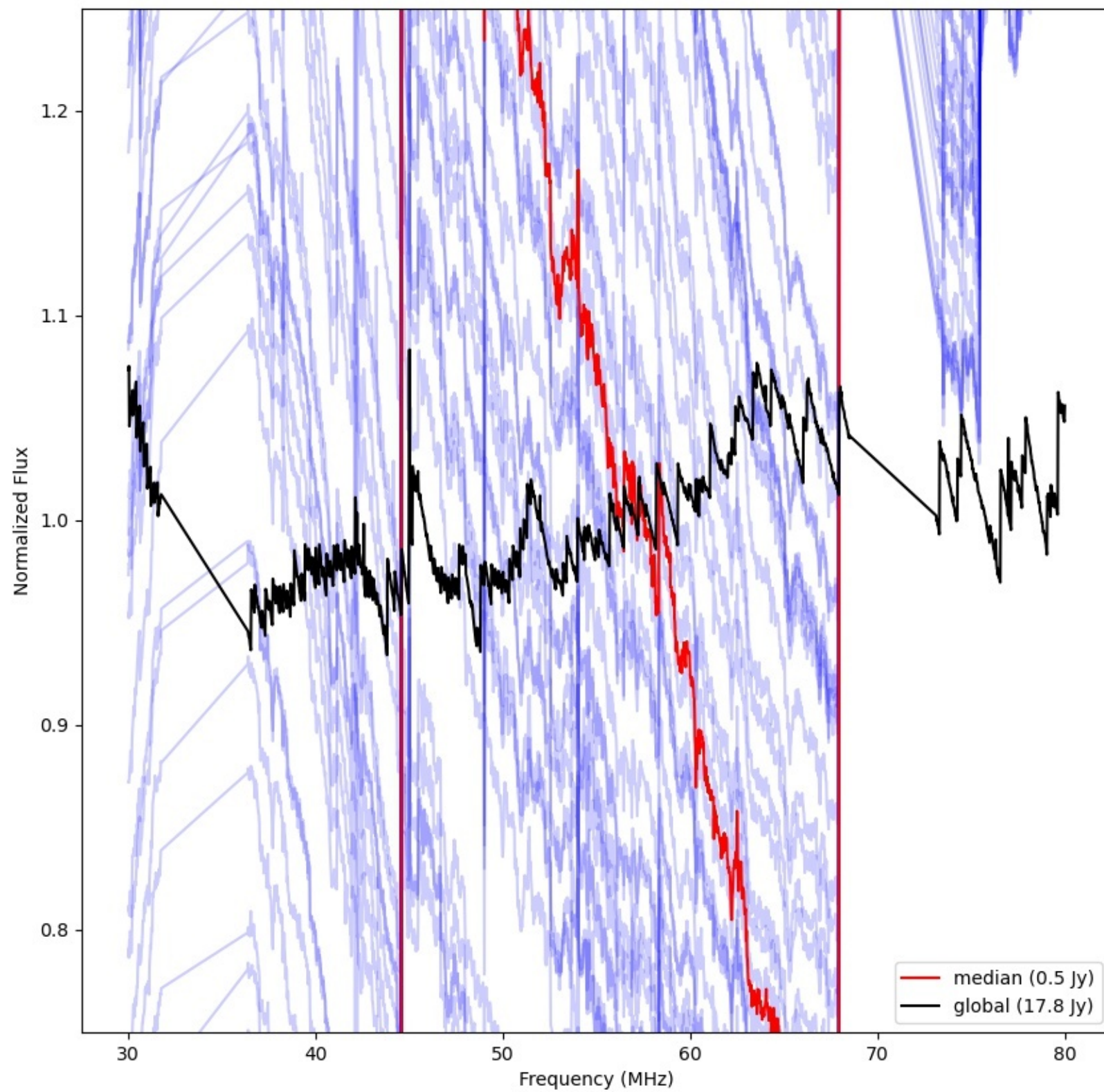
LWA052 - Correlator# 117 - XX - FLAGS:LowFlux
