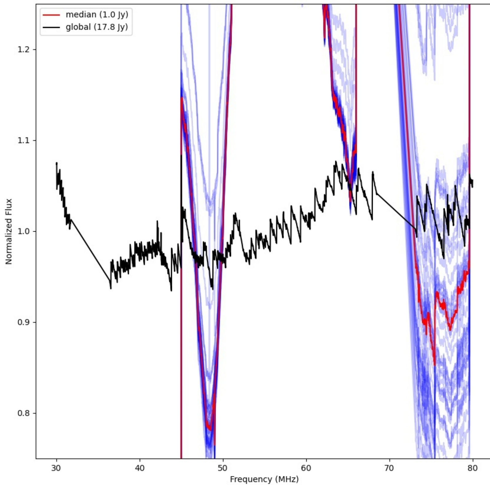
LWA105 - Correlator# 178 - XX - FLAGS:LowFlux
