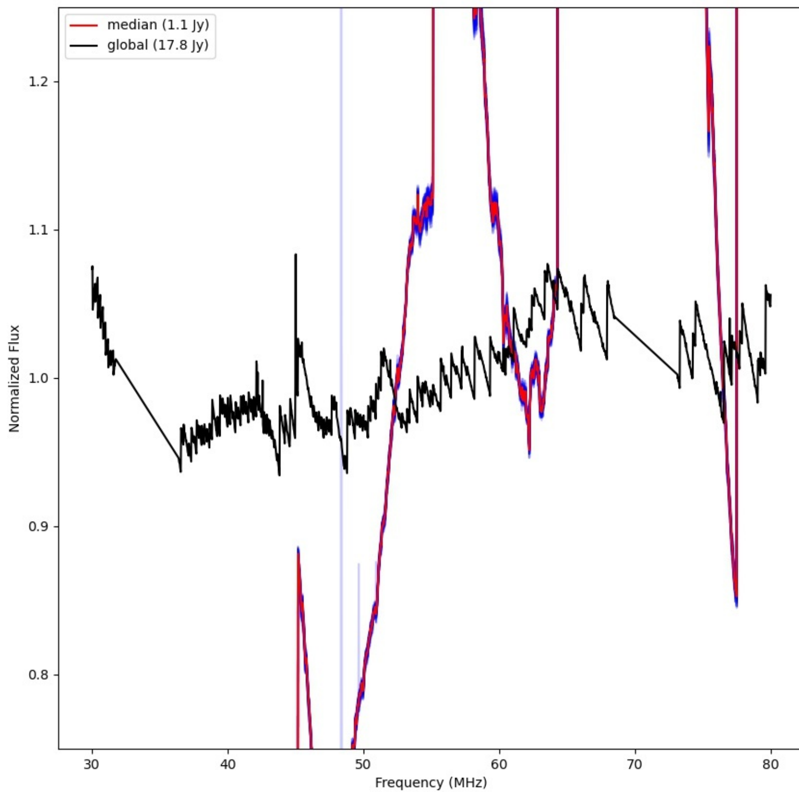
LWA232 - Correlator# 307 - XX - FLAGS:LowFlux
