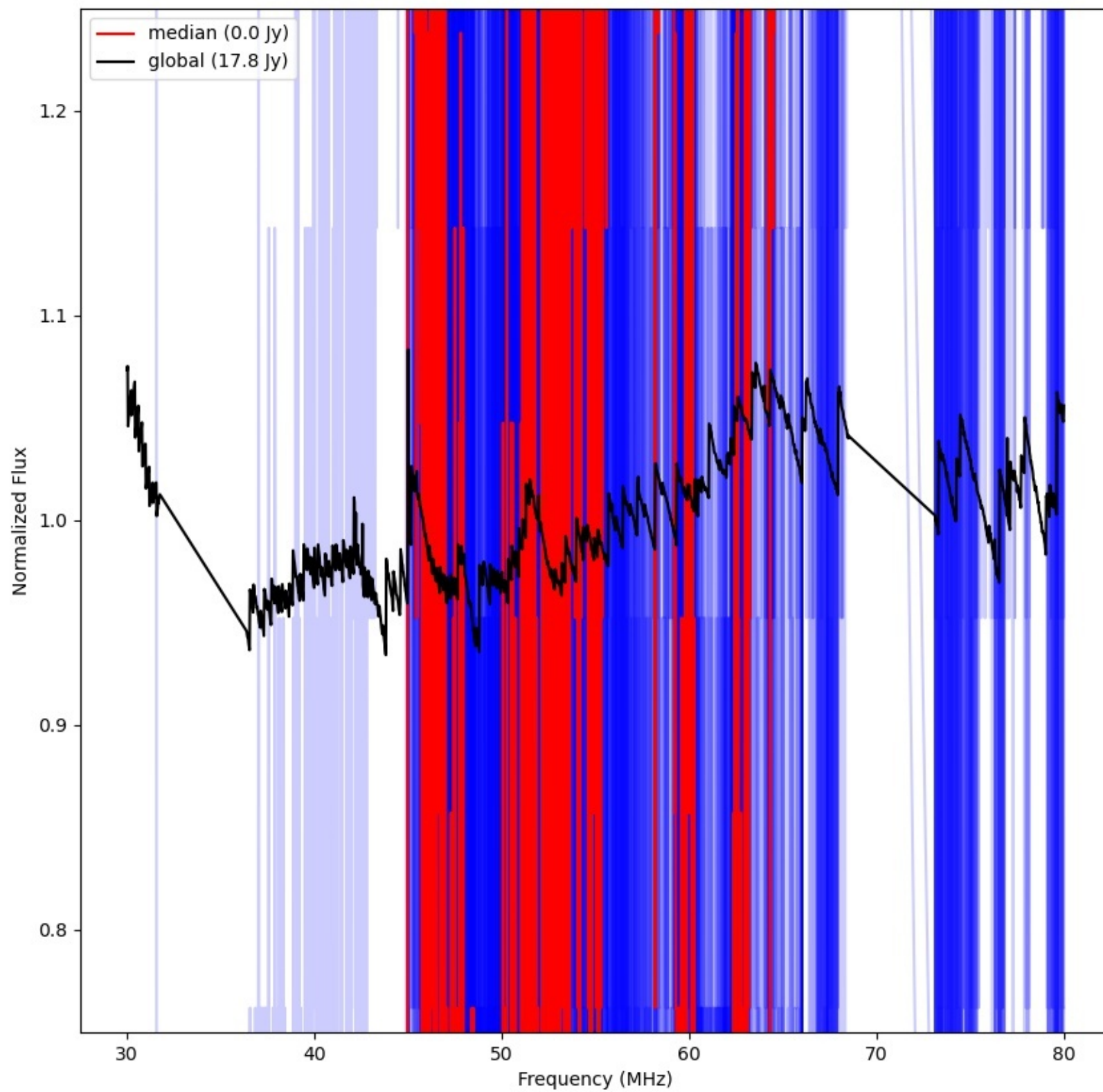
LWA209 - Correlator# 301 - XX - FLAGS:LowFlux
