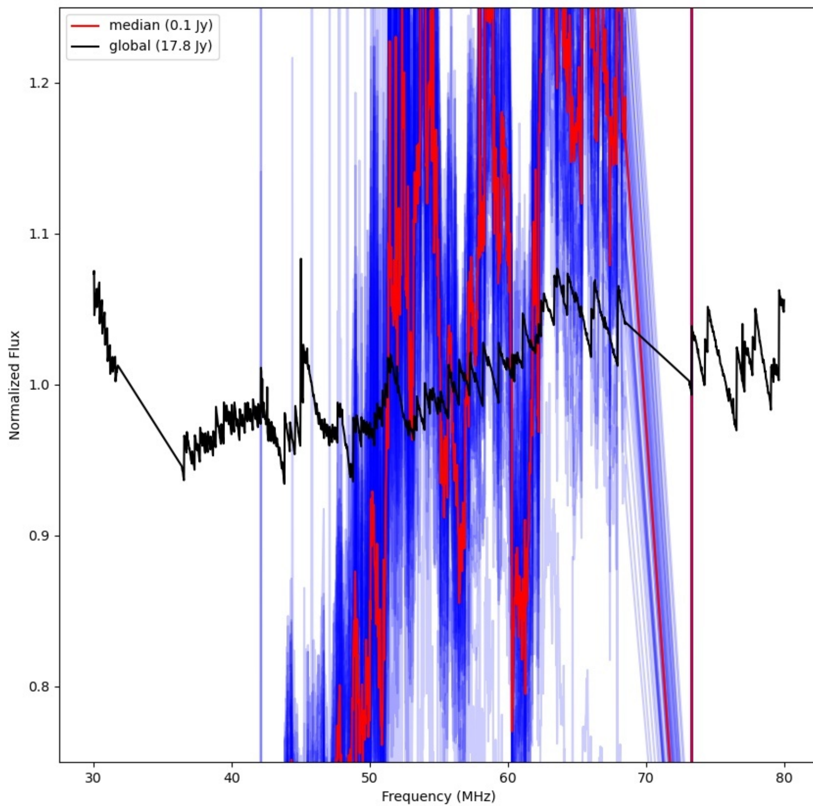
LWA255 - Correlator# 033 - XX - FLAGS:LowFlux
