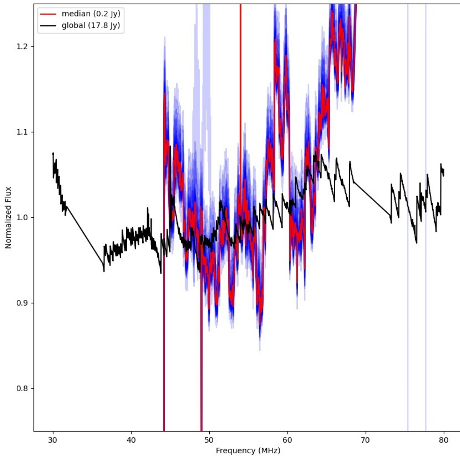
LWA187 - Correlator# 242 - XX - FLAGS:LowFlux
