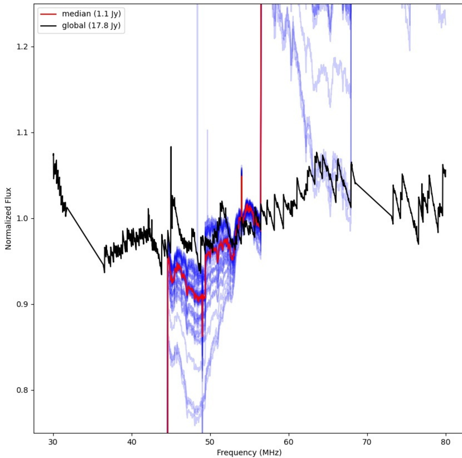
LWA111 - Correlator# 201 - XX - FLAGS:LowFlux
