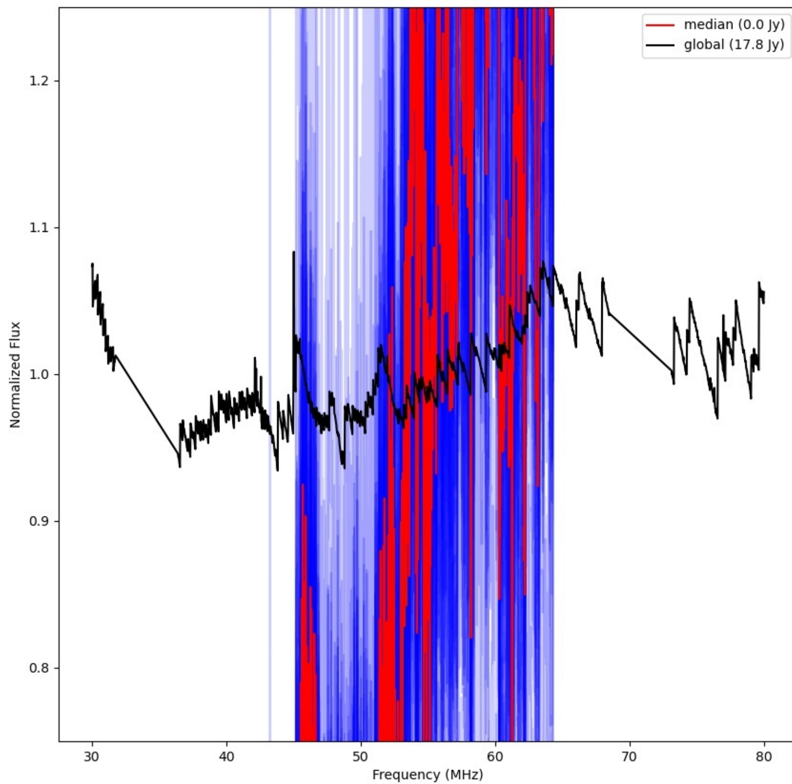
LWA041 - Correlator# 079 - XX - FLAGS:LowFlux
