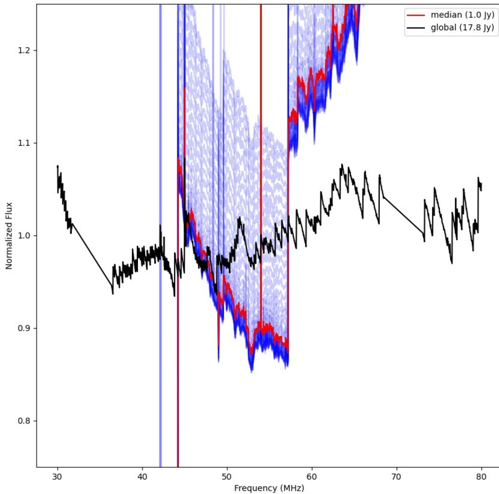
LWA153 - Correlator# 230 - XX - FLAGS:LowFlux
