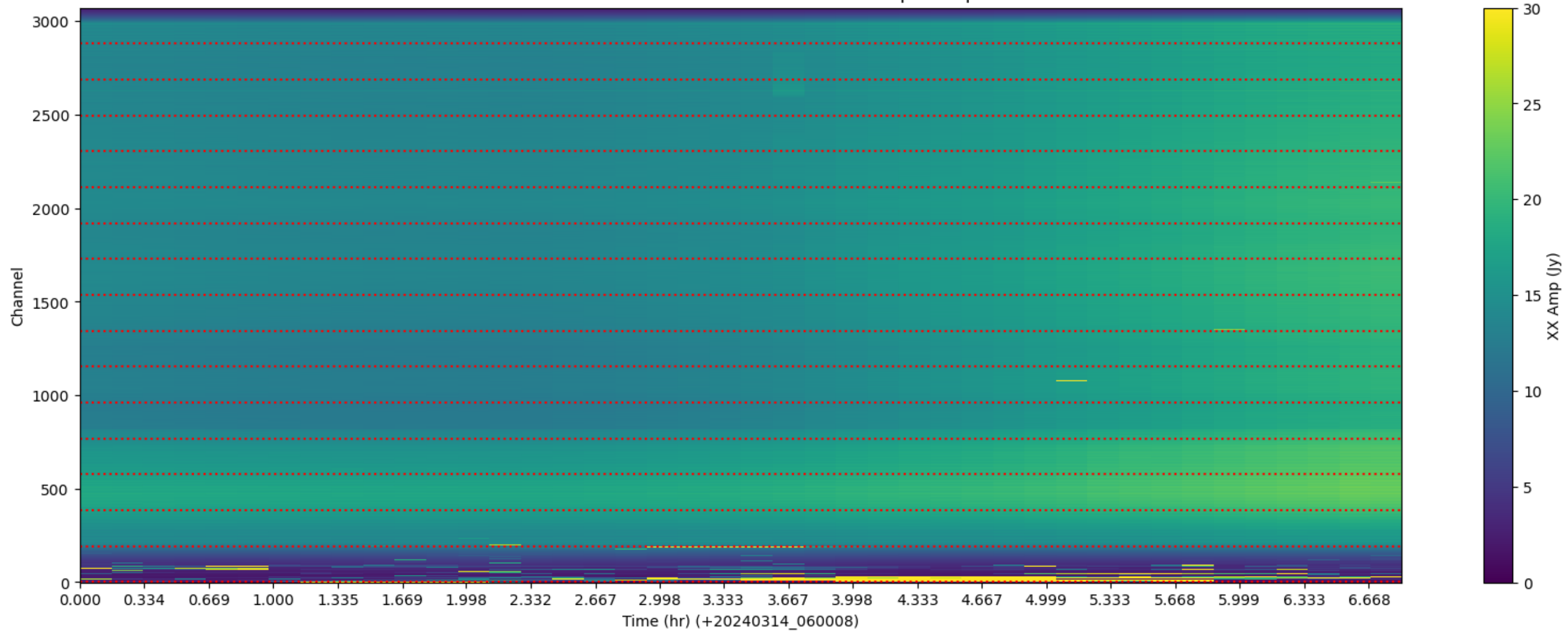
LWA305 - Correlator# 050 - XX - FLAGS: BadSpecShape
