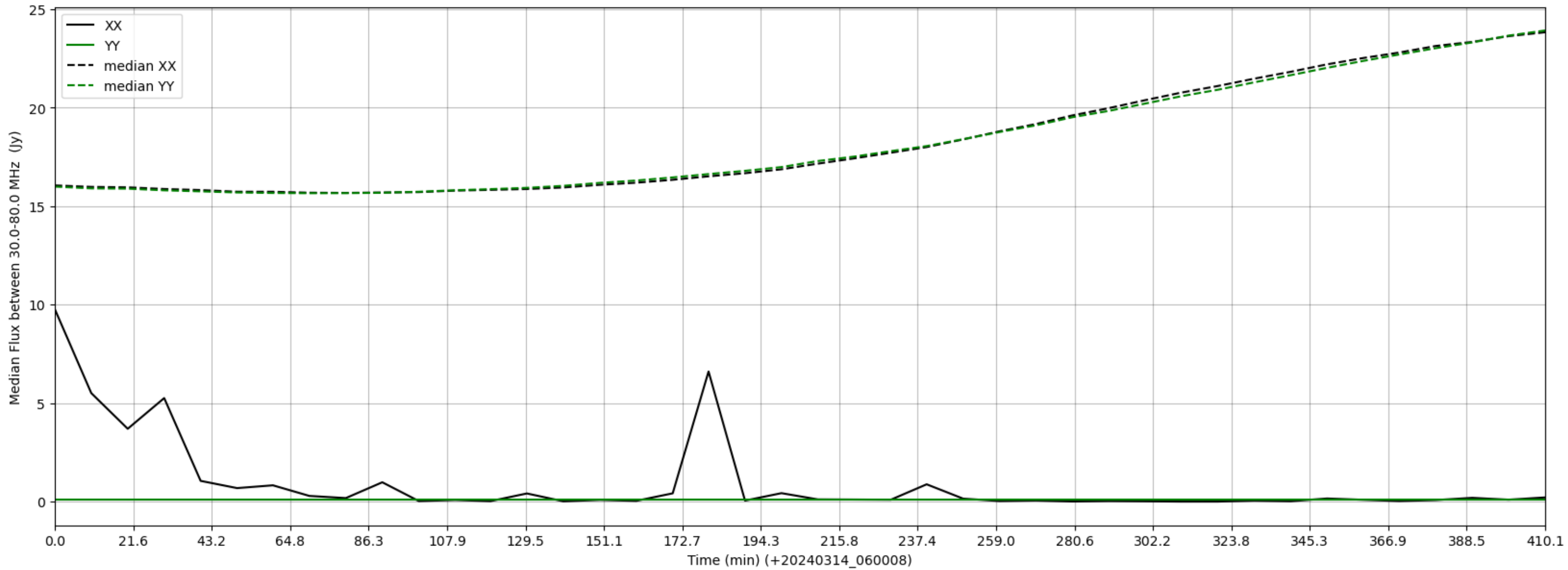
LWA353 - Correlator# 031 - XX FLAGS:LowFlux - YY FLAGS:LowFlux
