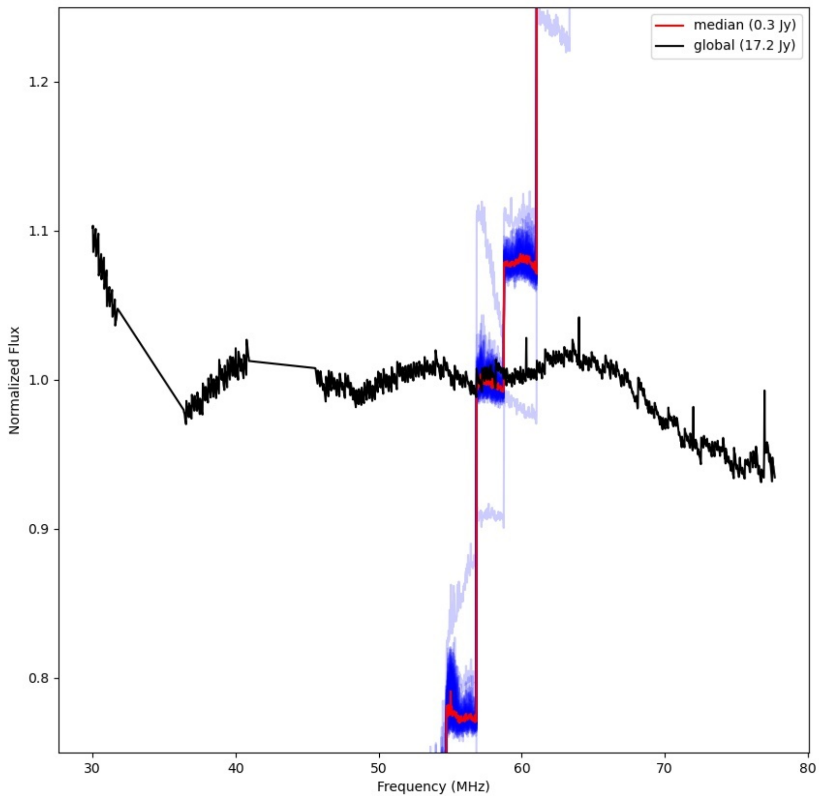
LWA041 - Correlator# 079 - YY - FLAGS:LowFlux
