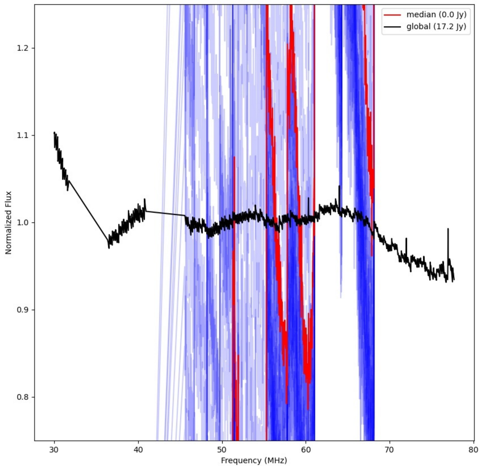
LWA309 - Correlator# 014 - YY - FLAGS:LowFlux
