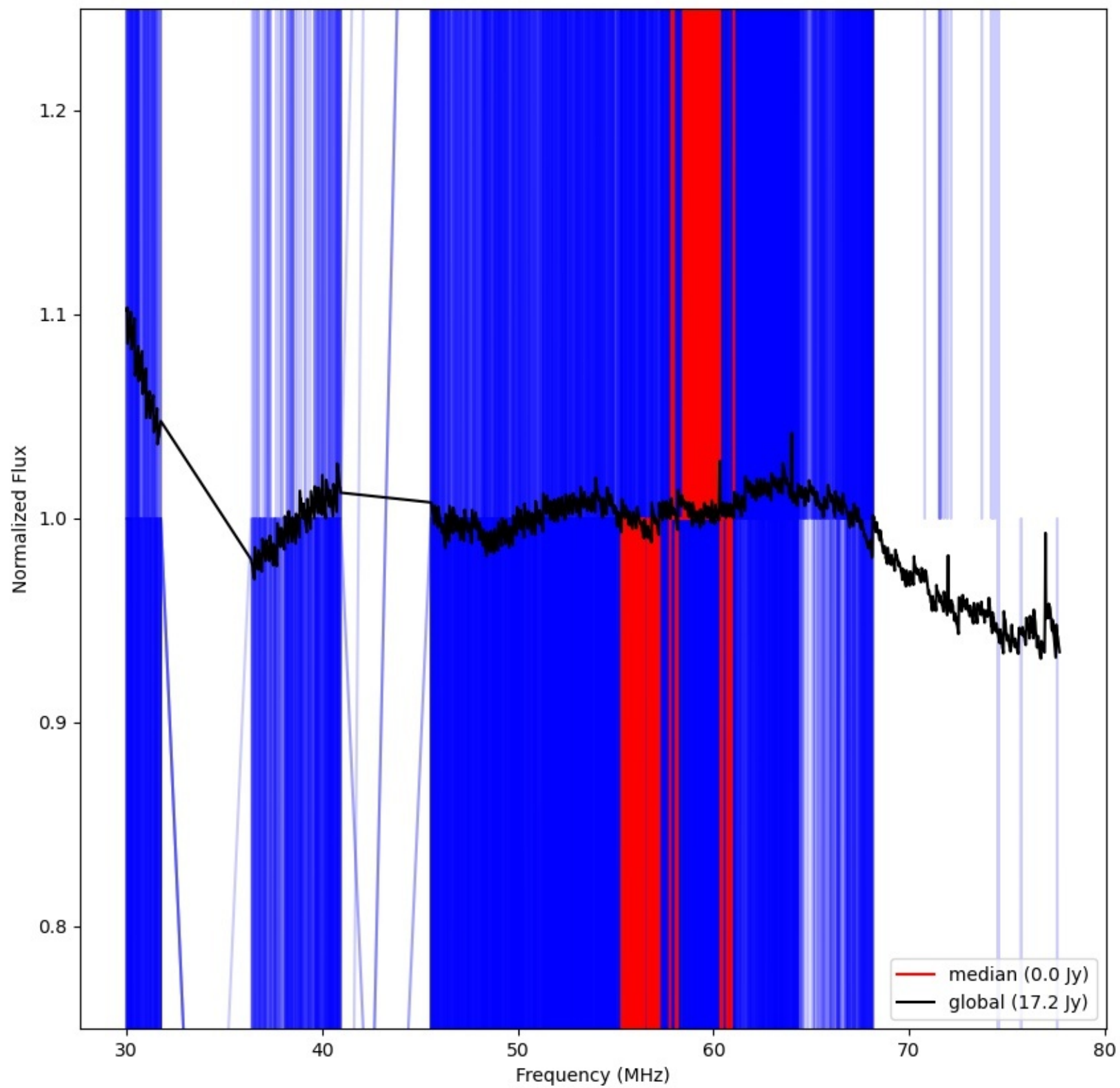
LWA325 - Correlator# 154 - YY - FLAGS:LowFlux
