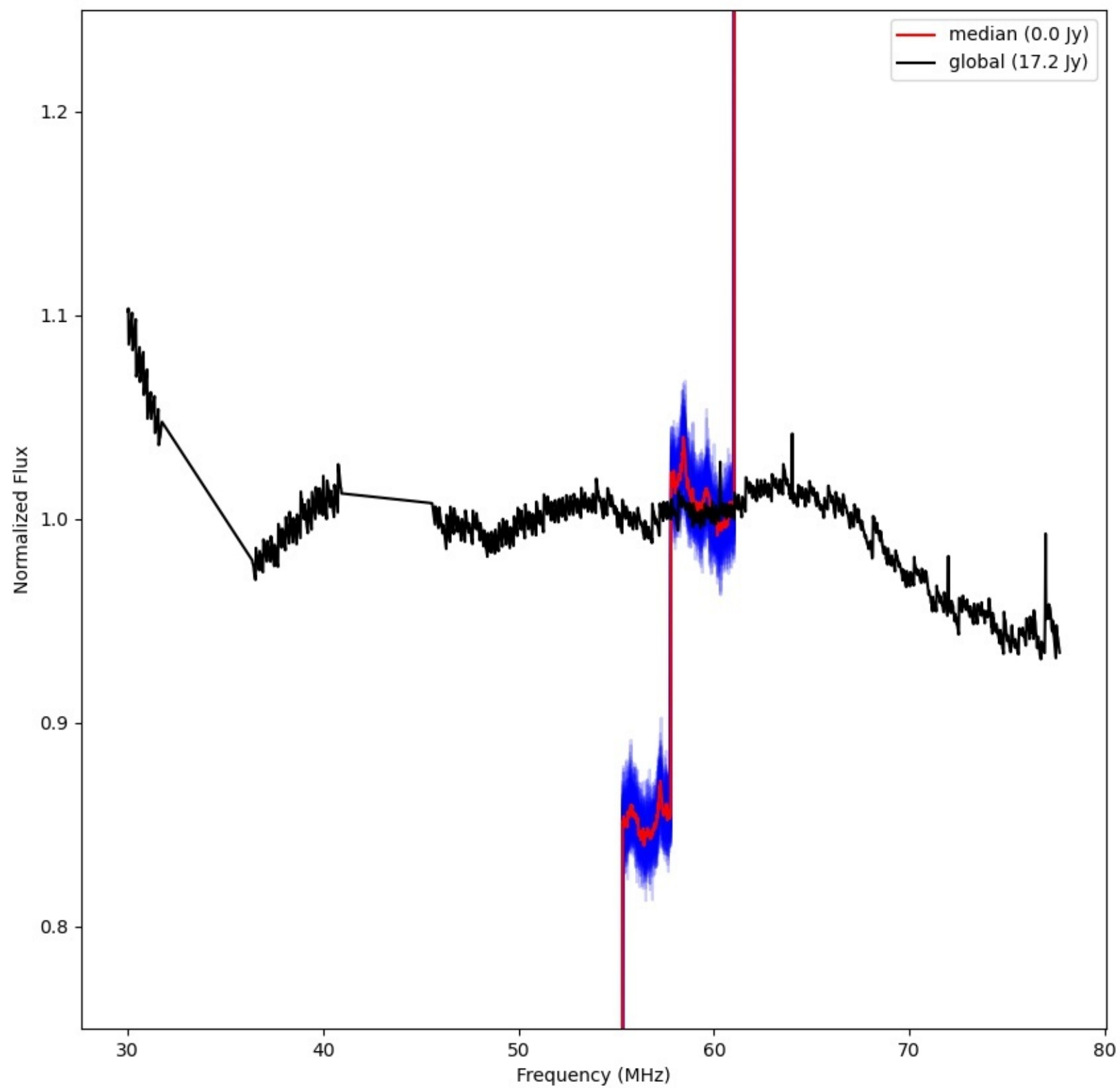
LWA365 - Correlator# 126 - YY - FLAGS:LowFlux
