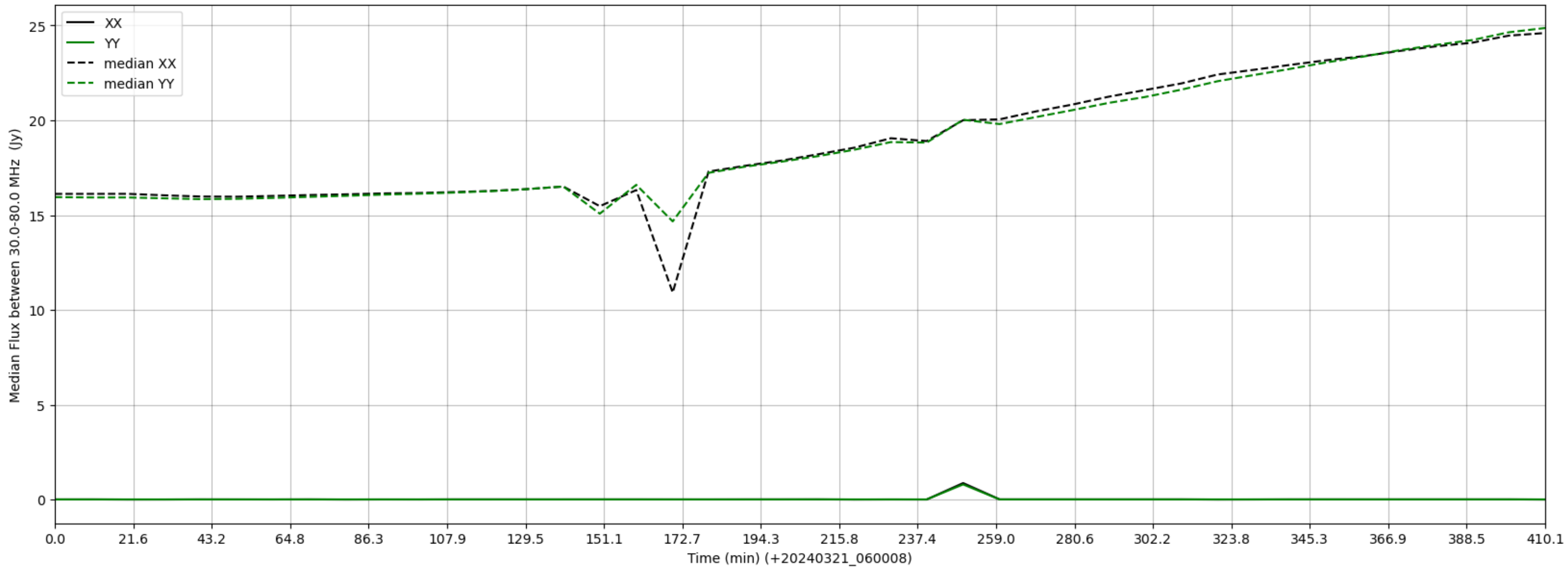
LWA120 - Correlator# 208 - XX FLAGS:LowFlux - YY FLAGS:LowFlux
