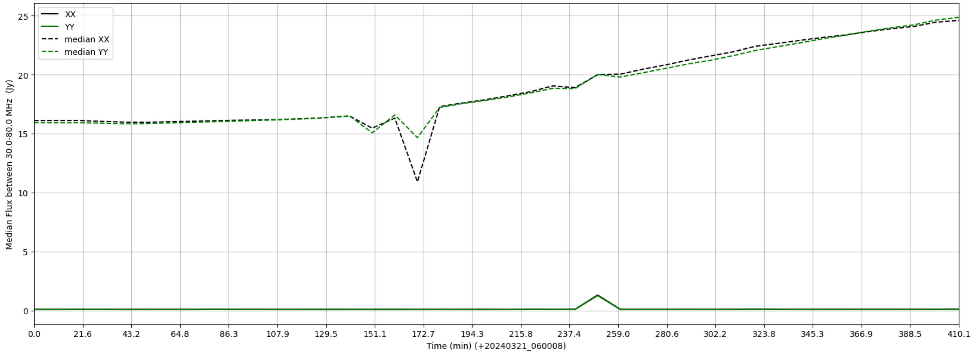
LWA142 - Correlator# 211 - XX FLAGS:LowFlux - YY FLAGS:LowFlux
