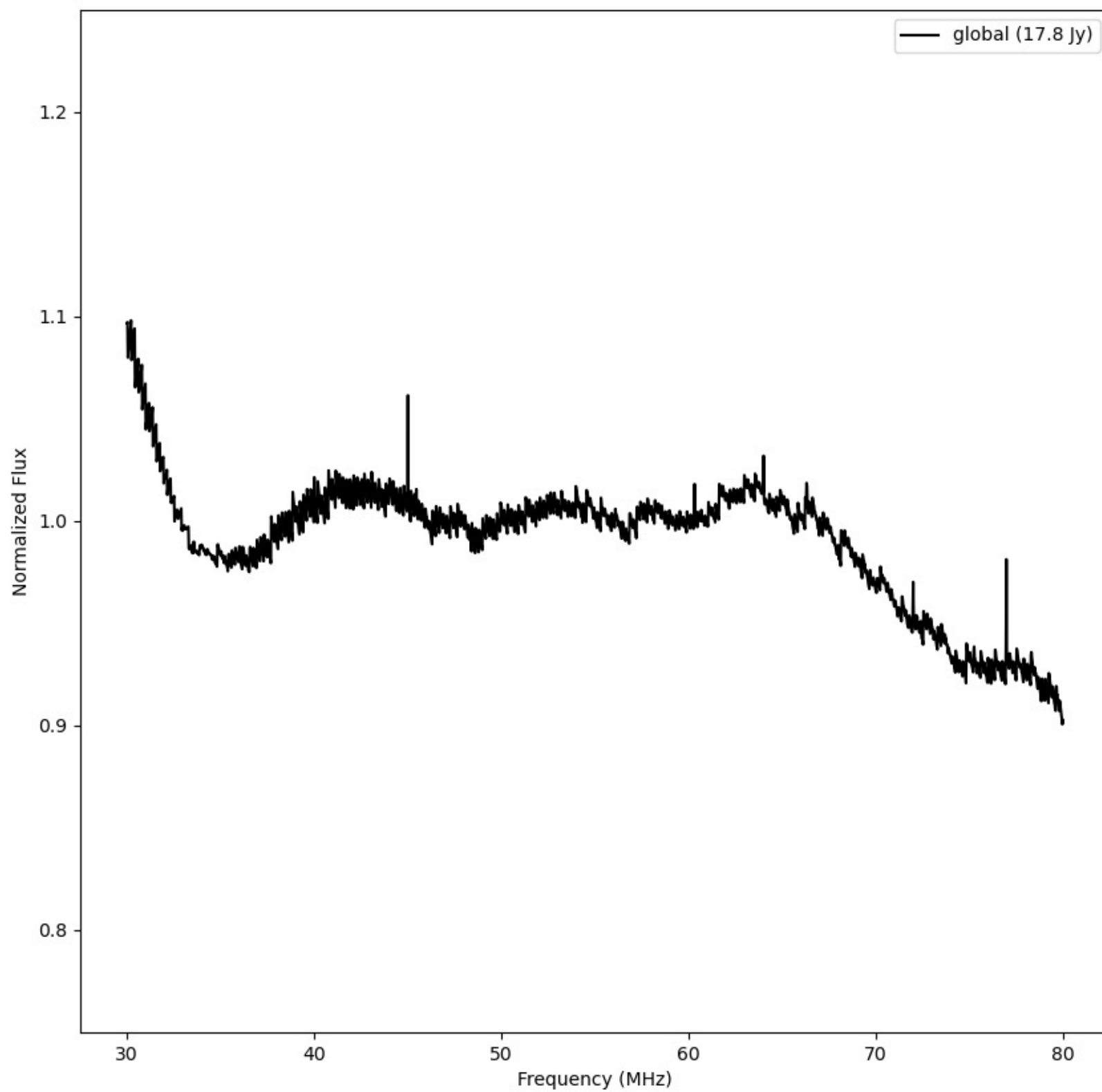
LWA280 - Correlator# 041 - YY - FLAGS:LowFlux
