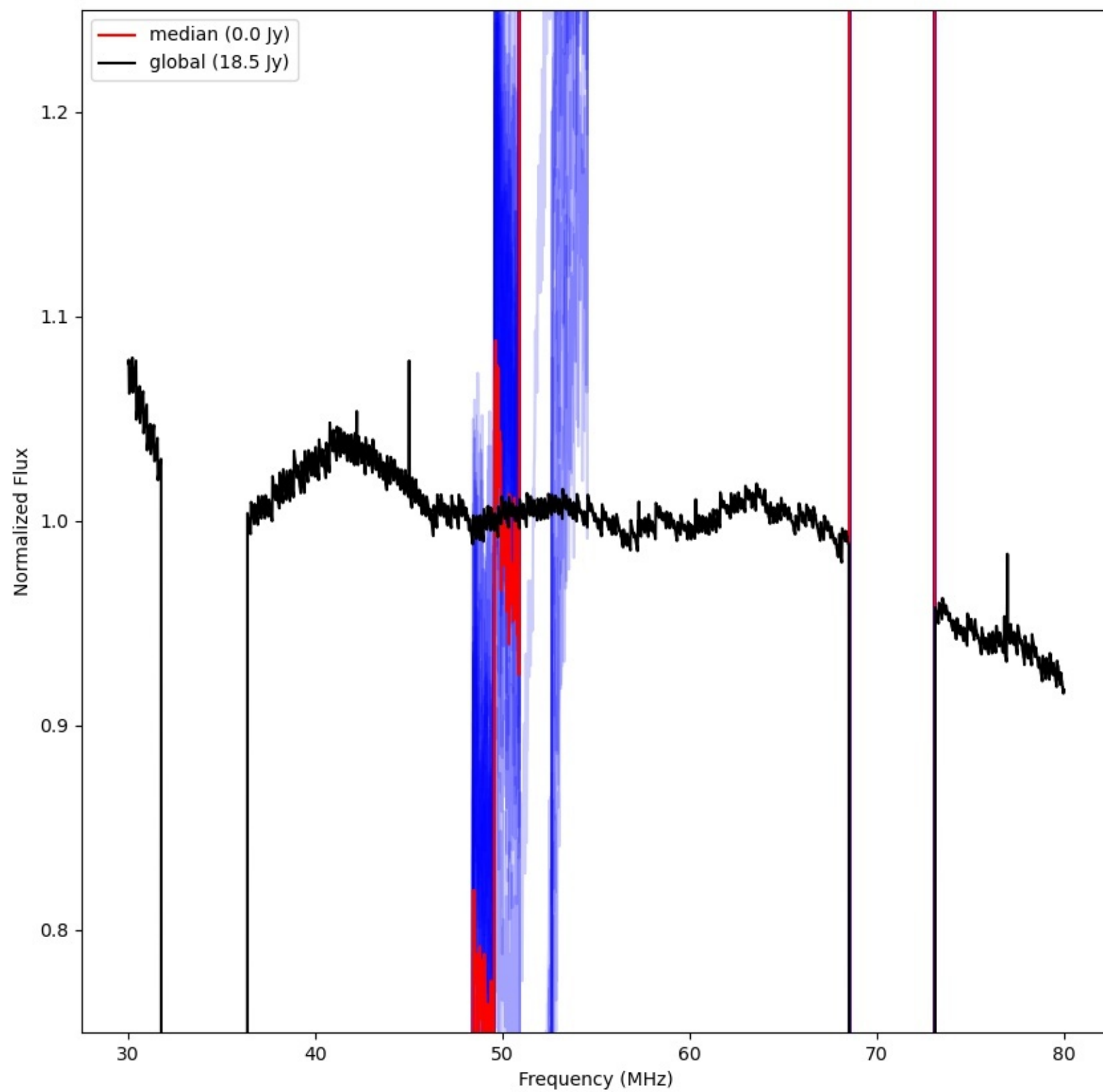
LWA120 - Correlator# 208 - XX - FLAGS:LowFlux
