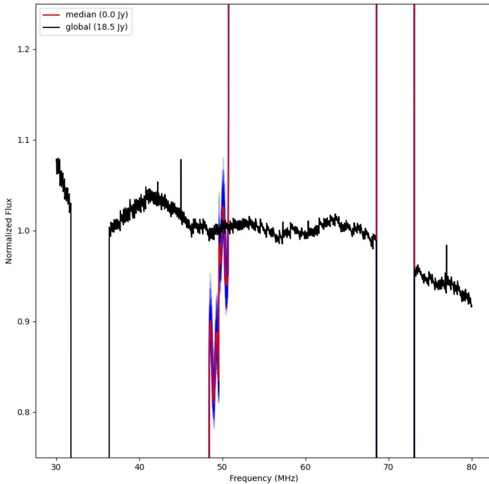
LWA142 - Correlator# 211 - XX - FLAGS:LowFlux
