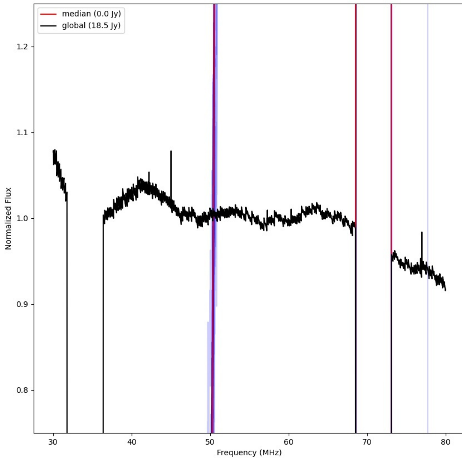
LWA151 - Correlator# 218 - XX - FLAGS:LowFlux
