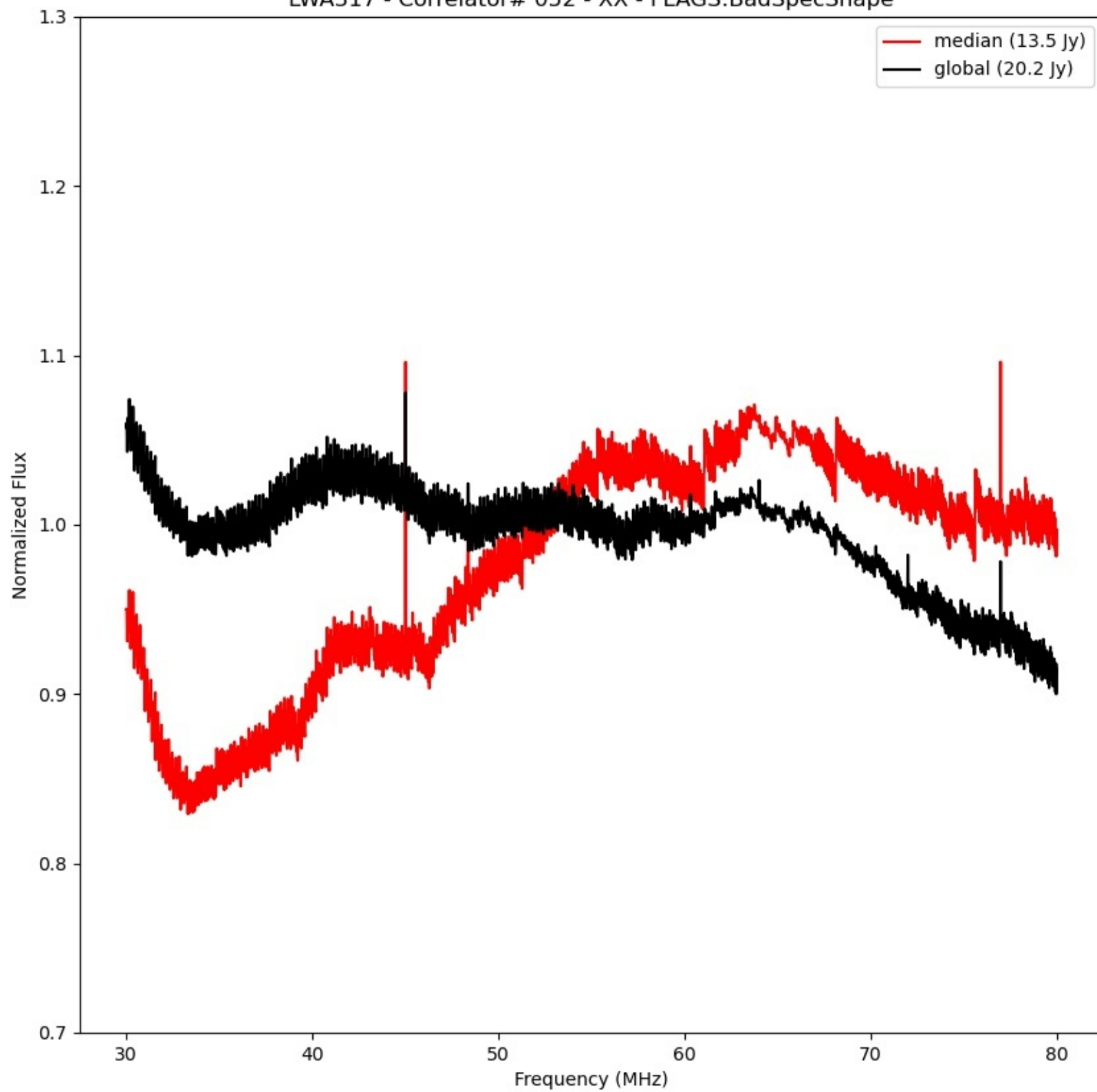
LWA317 - Correlator# 052 - XX - FLAGS:BadSpecShape
