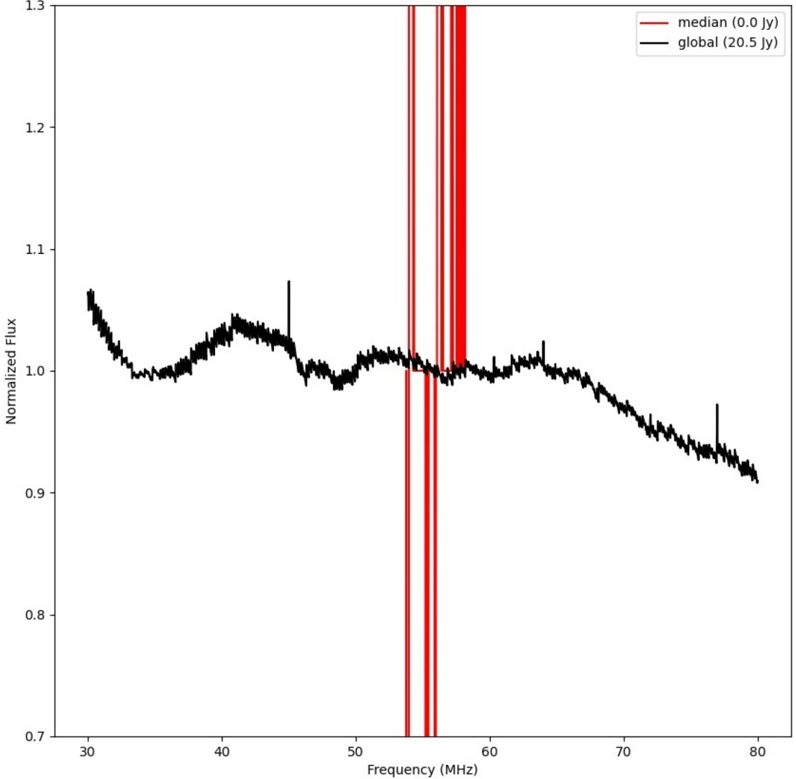
LWA052 - Correlator# 117 - XX - FLAGS:LowFlux
