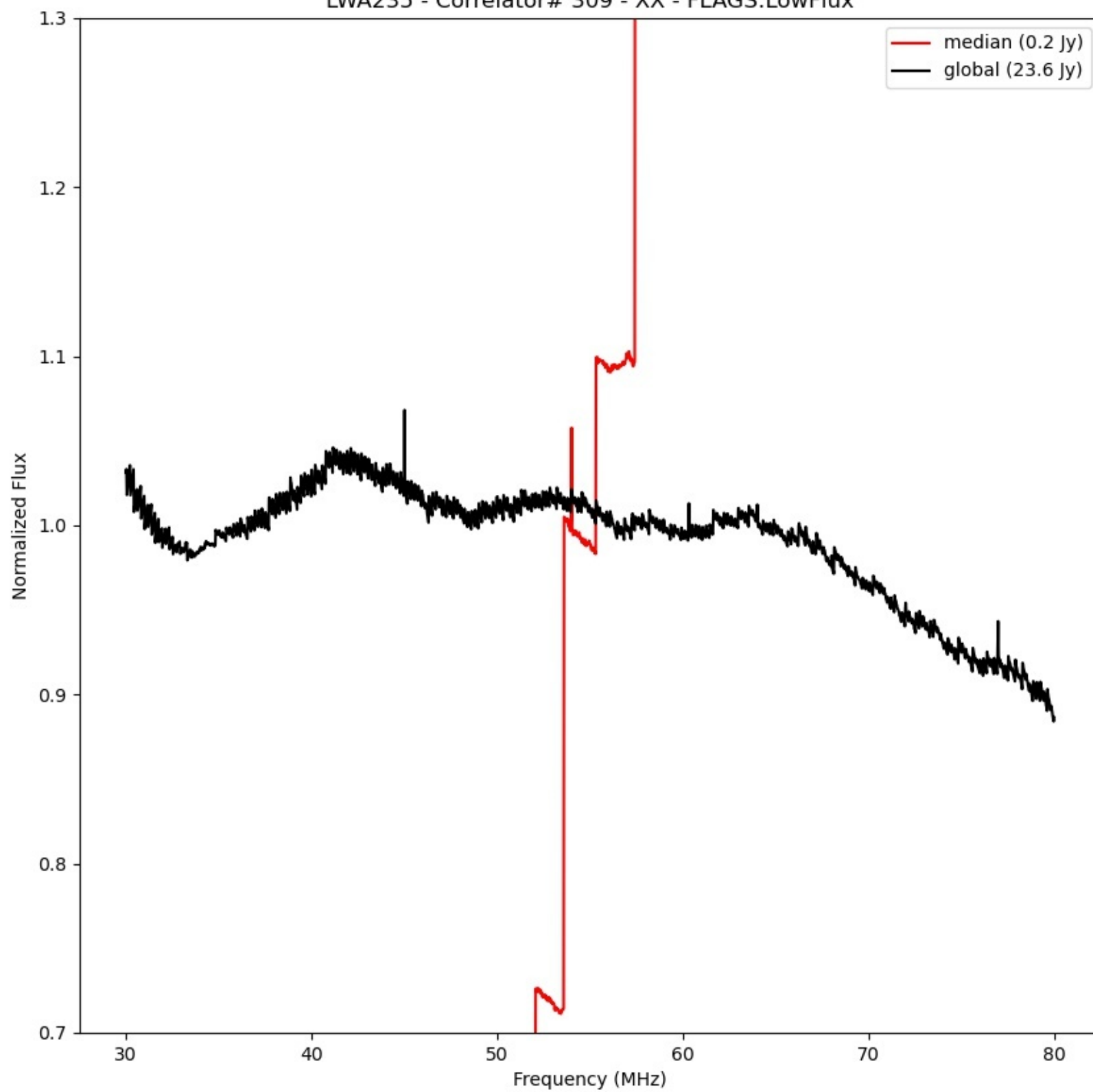
LWA235 - Correlator# 309 - XX - FLAGS:LowFlux
