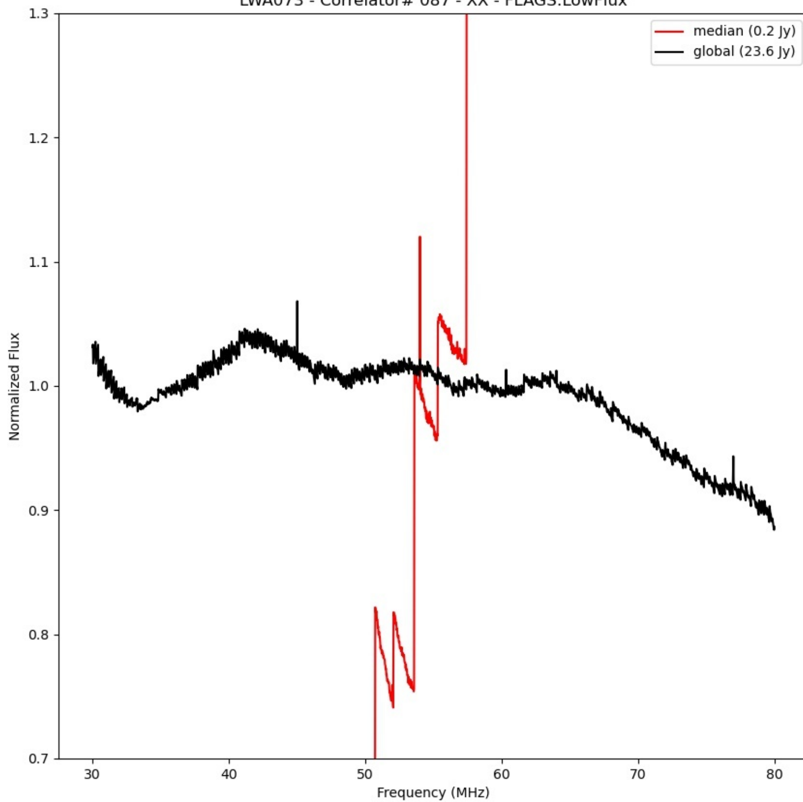
LWA073 - Correlator# 087 - XX - FLAGS:LowFlux
