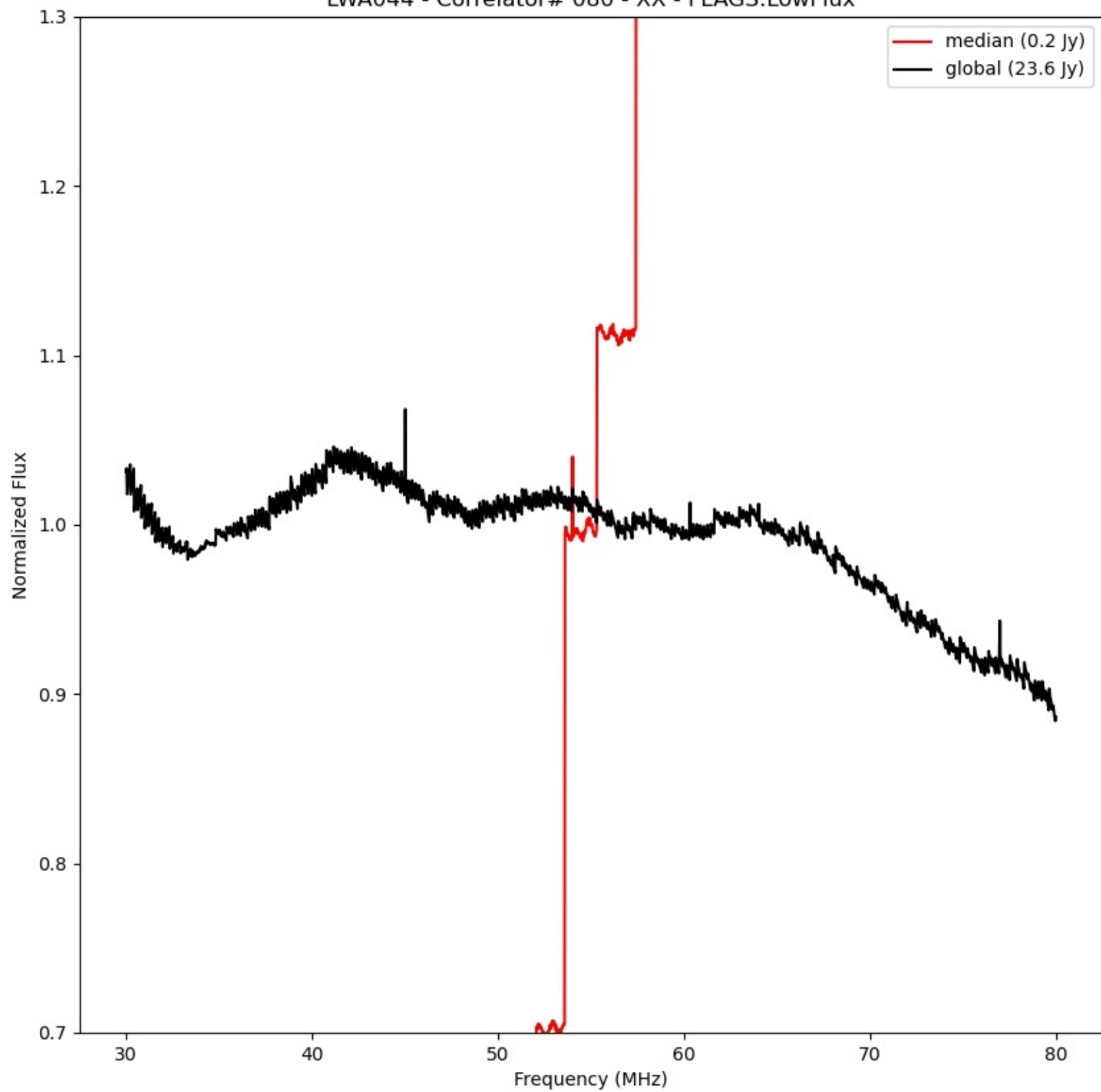
LWA044 - Correlator# 080 - XX - FLAGS:LowFlux
