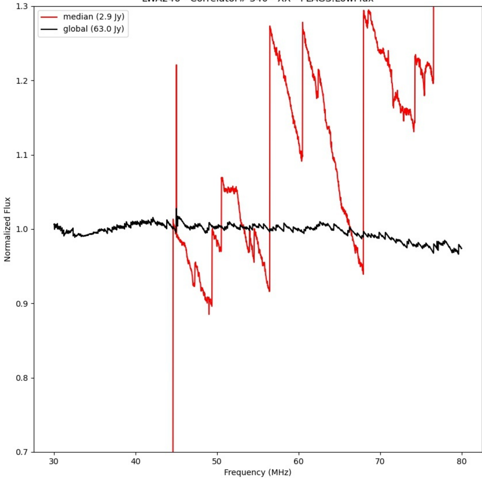
LWA246 - Correlator# 340 - XX - FLAGS:LowFlux
