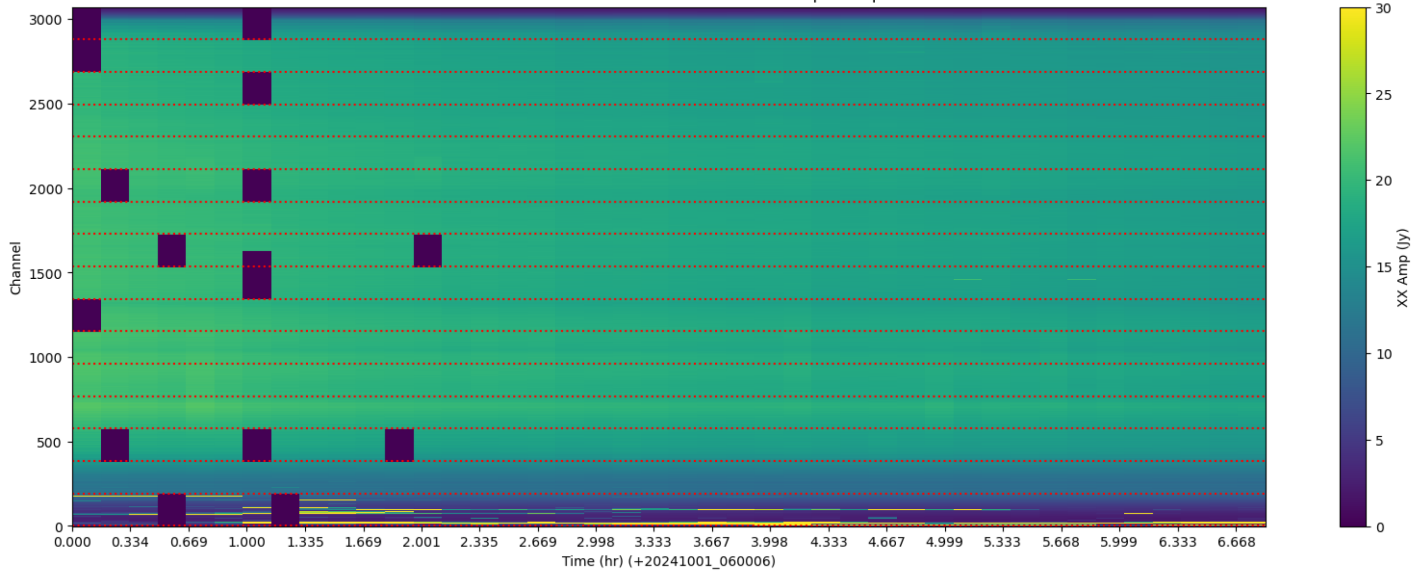
LWA340 - Correlator# 026 - XX - FLAGS: BadSpecShape
