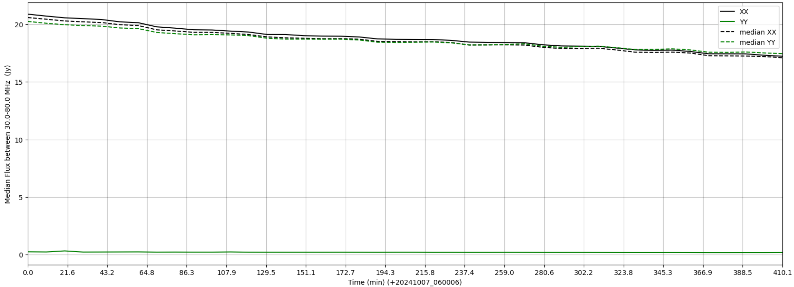
LWA190 - Correlator# 244 - XX FLAGS:Good - YY FLAGS:LowFlux
