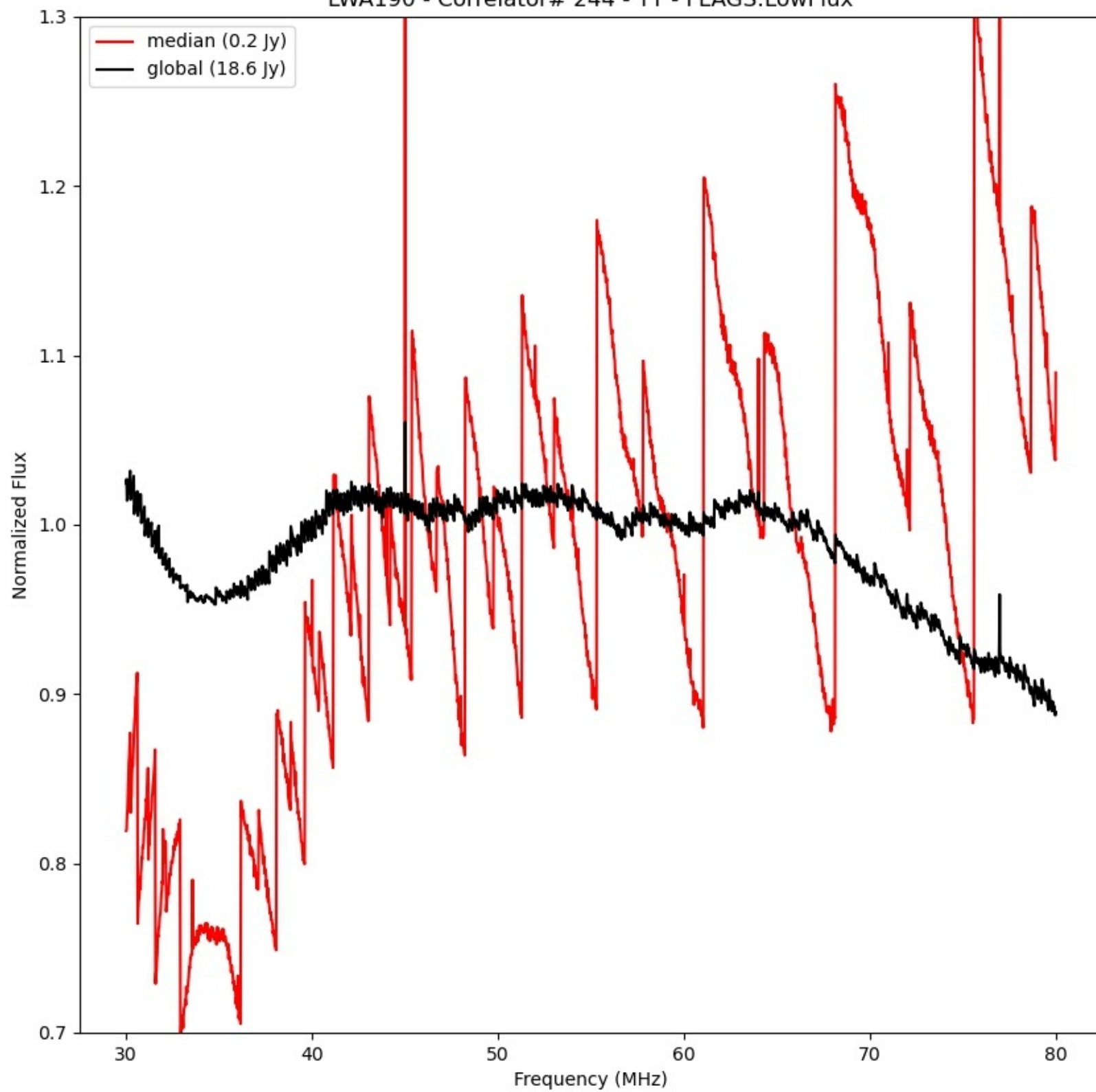
LWA190 - Correlator# 244 - YY - FLAGS:LowFlux
