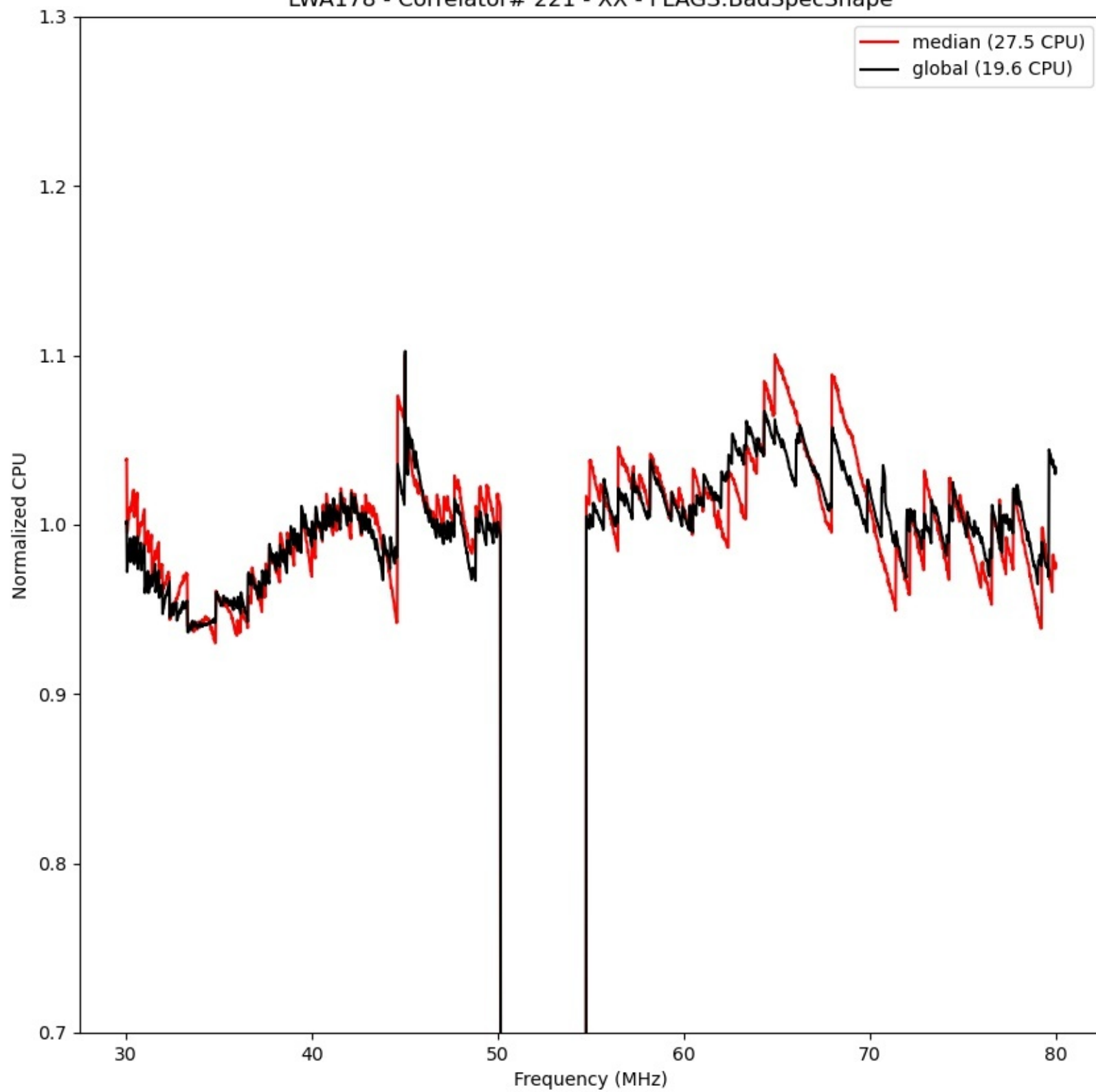
LWA178 - Correlator# 221 - XX - FLAGS:BadSpecShape
