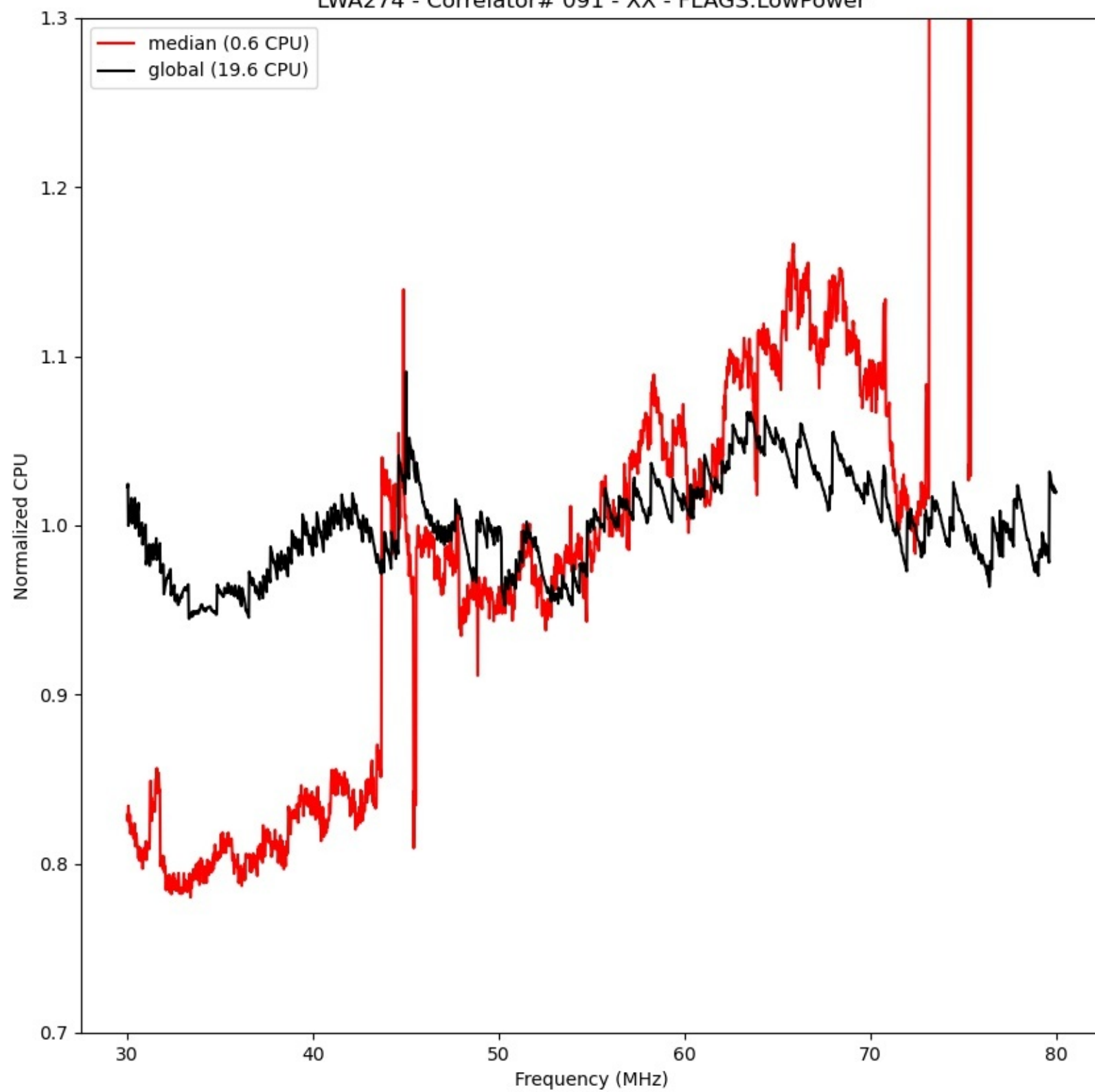
LWA274 - Correlator# 091 - XX - FLAGS:LowPower
