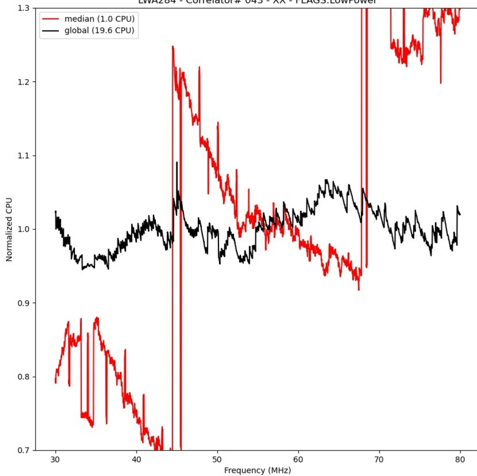
LWA284 - Correlator# 043 - XX - FLAGS:LowPower
