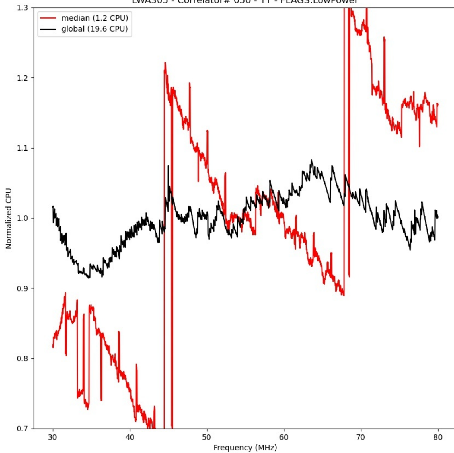
LWA305 - Correlator# 050 - YY - FLAGS:LowPower
