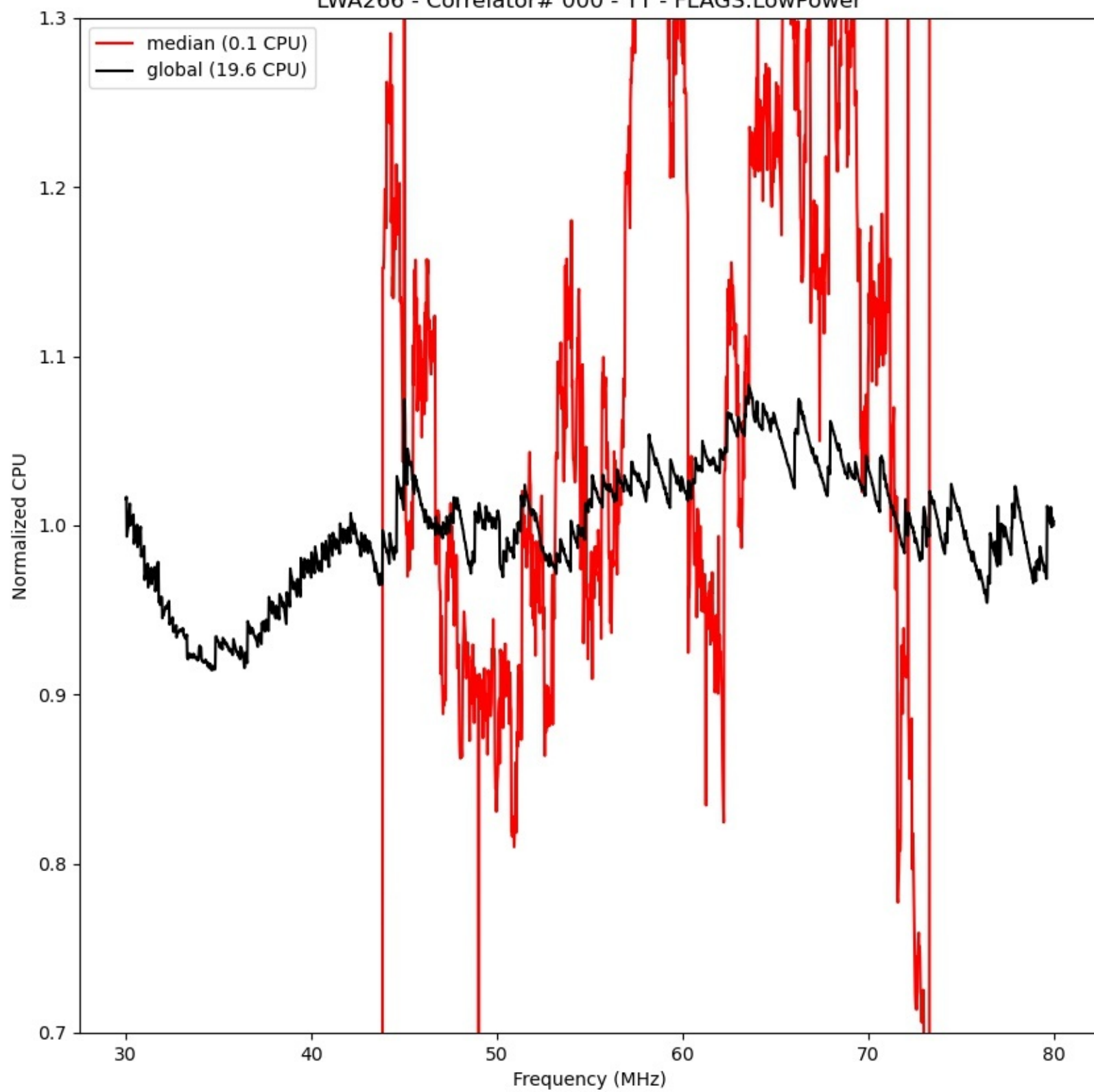
LWA266 - Correlator# 000 - YY - FLAGS:LowPower
