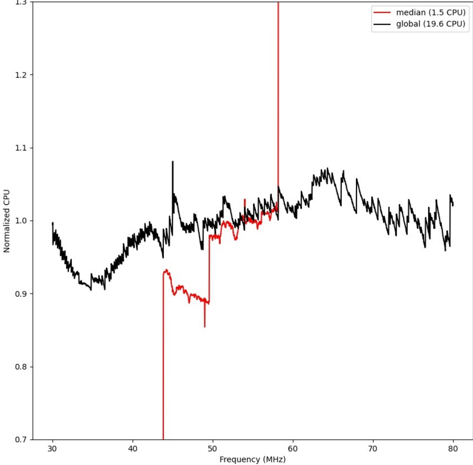
LWA255 - Correlator# 033 - YY - FLAGS:LowPower
