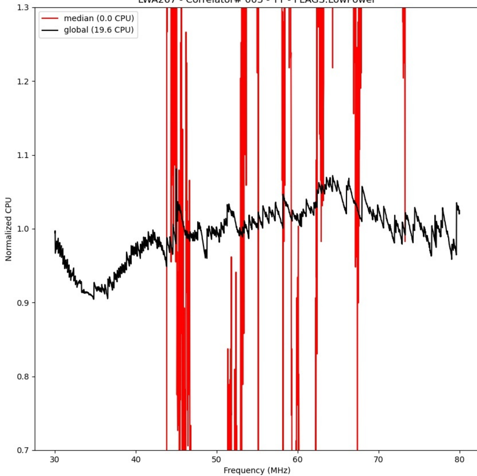
LWA267 - Correlator# 003 - YY - FLAGS:LowPower
