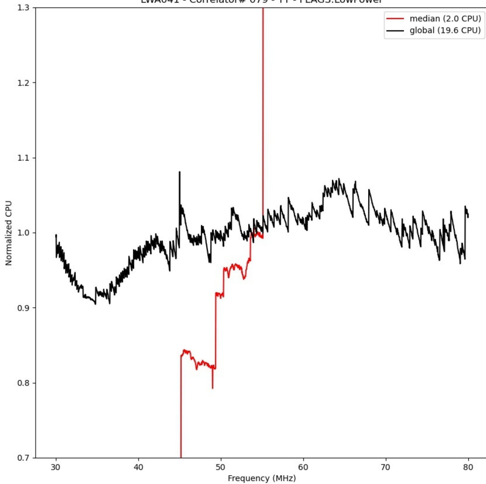
LWA041 - Correlator# 079 - YY - FLAGS:LowPower
