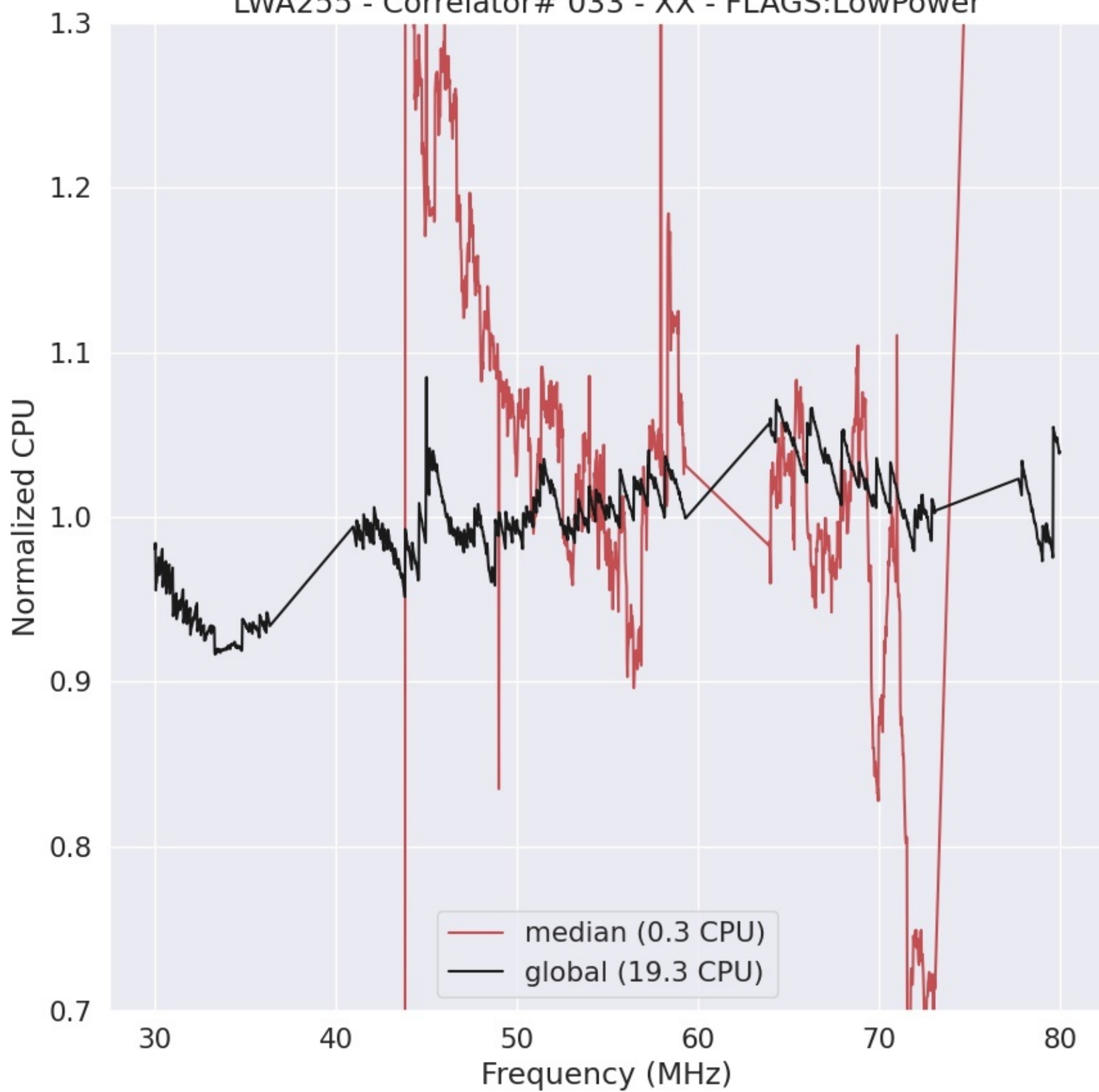
LWA255 - Correlator# 033 - XX - FLAGS:LowPower
