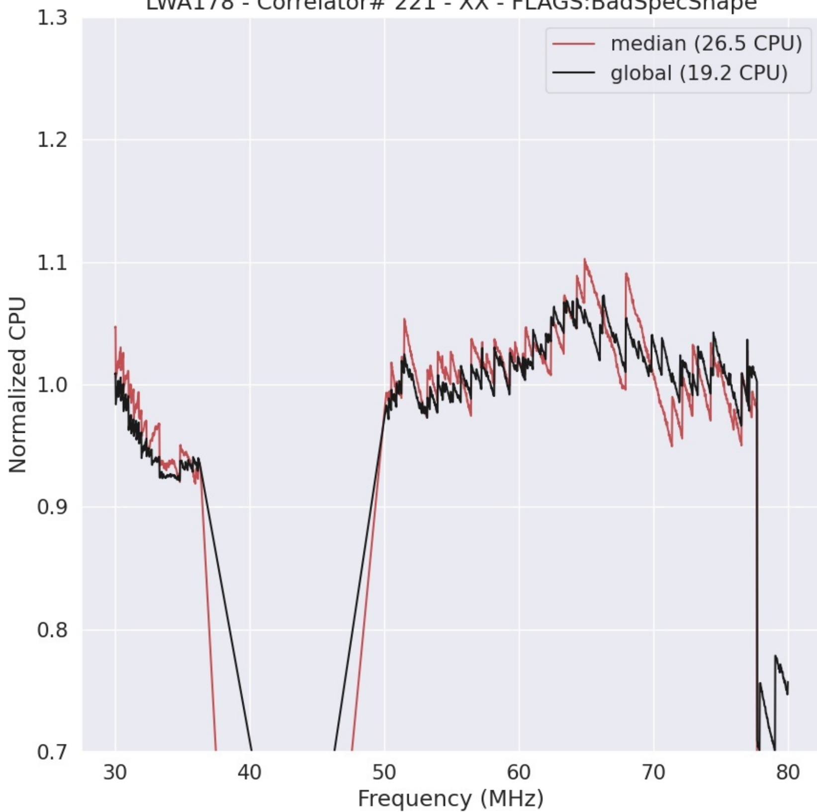
LWA178 - Correlator# 221 - XX - FLAGS:BadSpecShape
