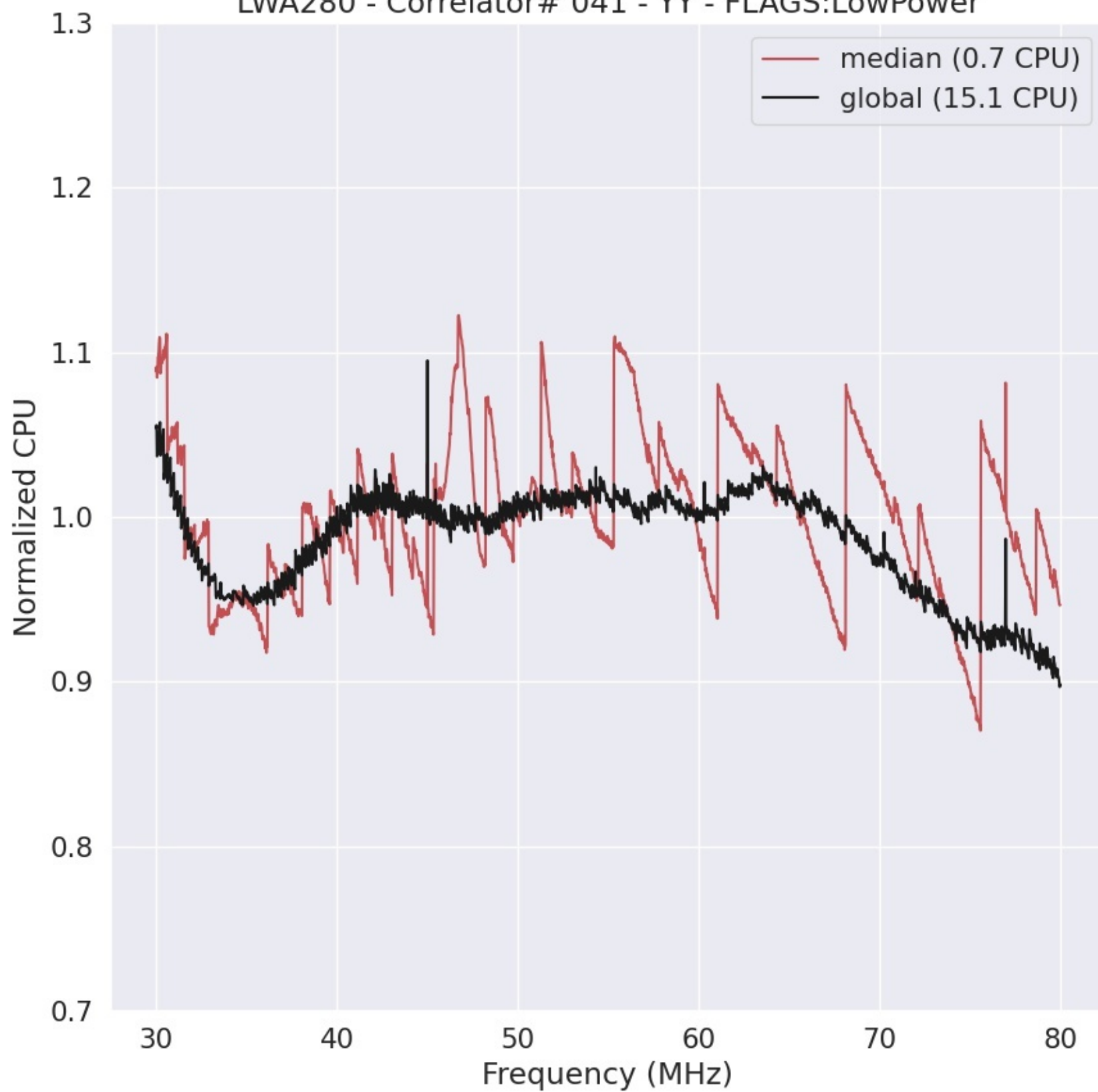
LWA280 - Correlator# 041 - YY - FLAGS:LowPower
