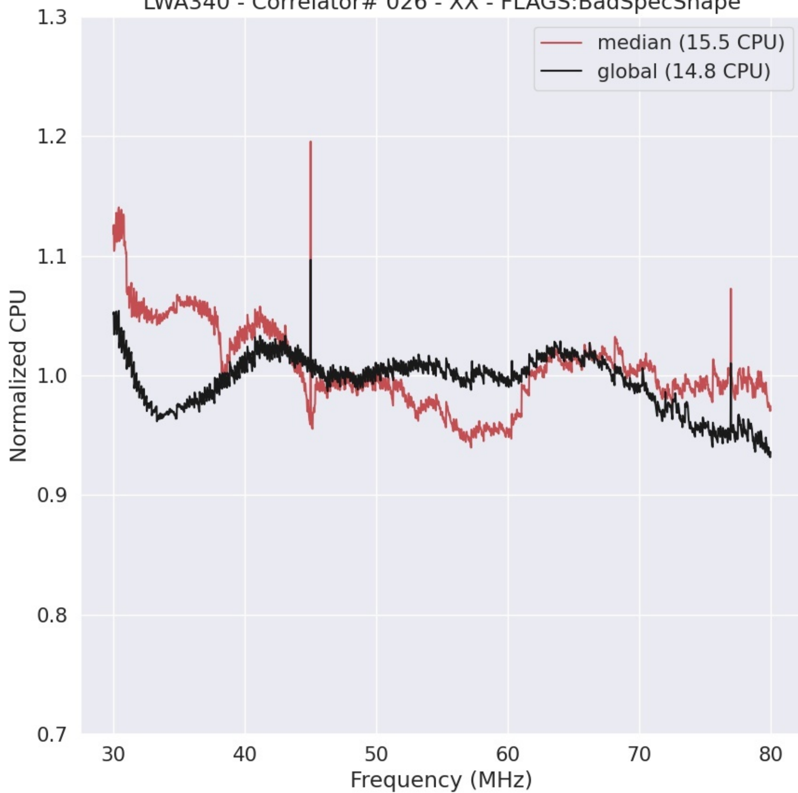
LWA340 - Correlator# 026 - XX - FLAGS:BadSpecShape
