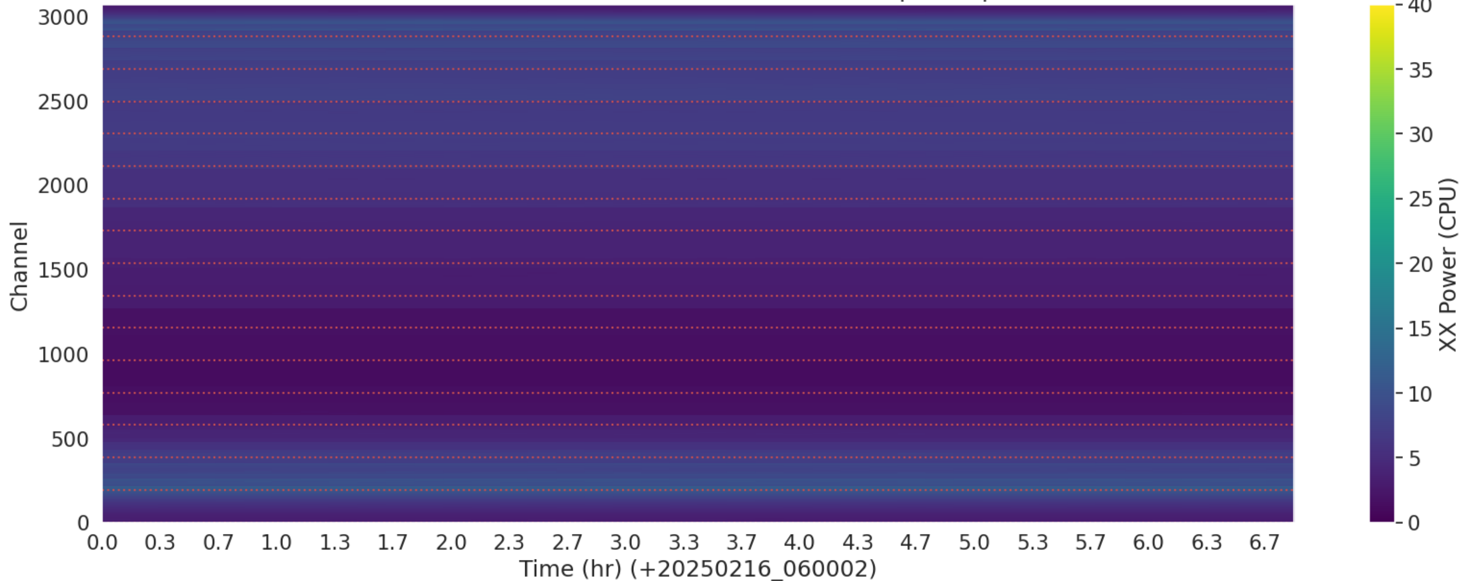
LWA321 - Correlator# 020 - XX - FLAGS: BadSpecShape
