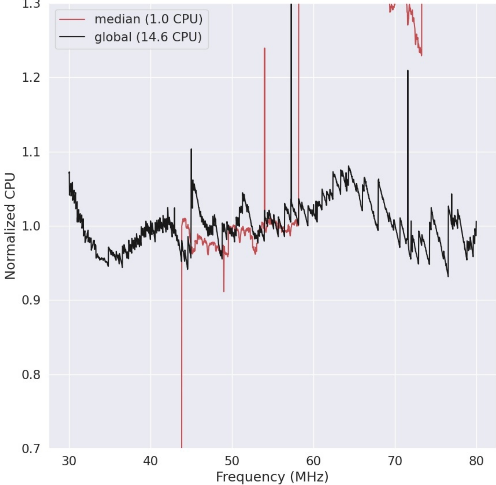
LWA347 - Correlator# 255 - XX - FLAGS:LowPower
