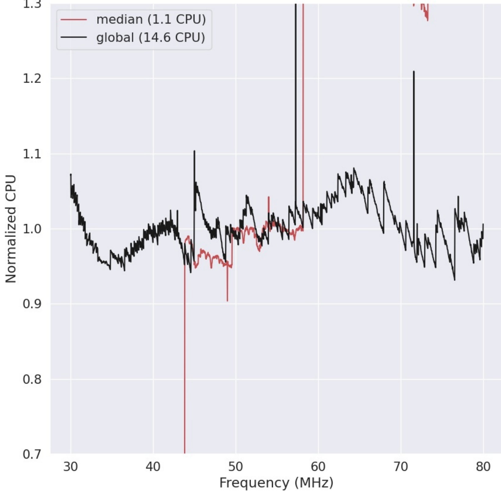
LWA311 - Correlator# 016 - XX - FLAGS:LowPower
