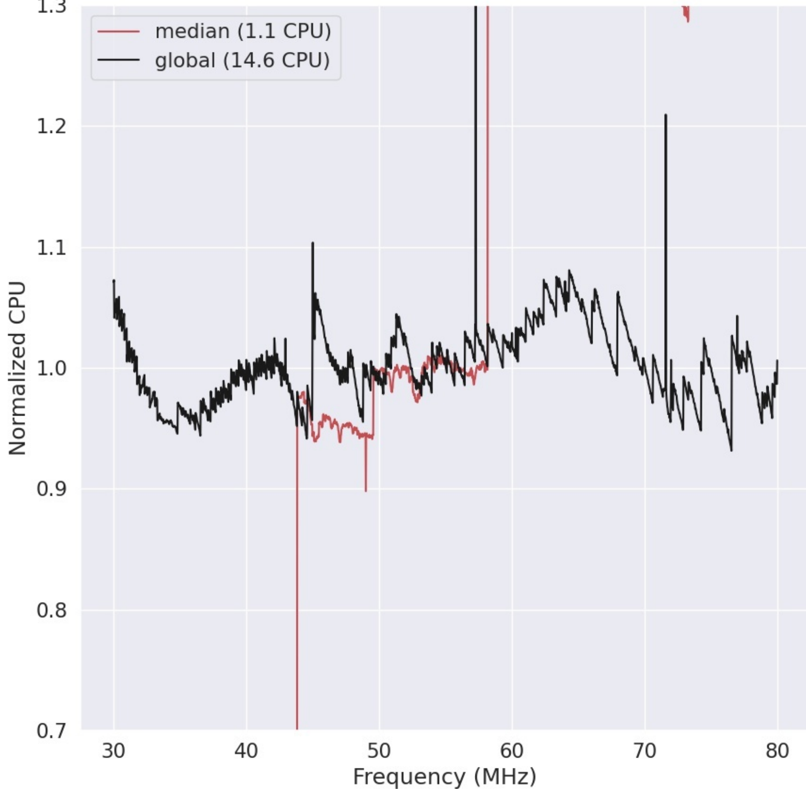
LWA341 - Correlator# 029 - XX - FLAGS:LowPower
