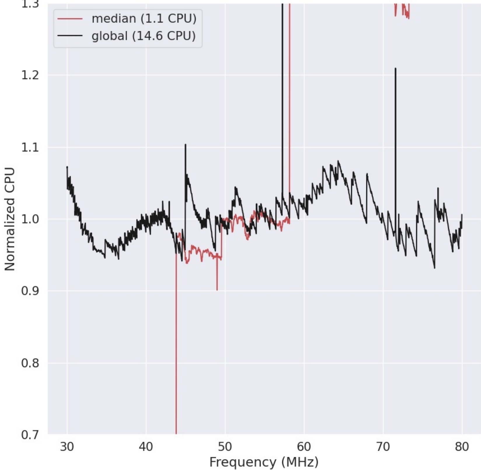
LWA319 - Correlator# 190 - XX - FLAGS:LowPower
