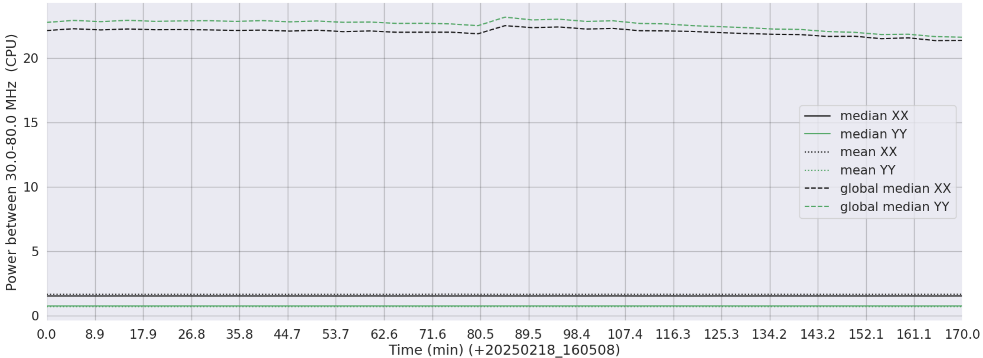
LWA352 - Correlator# 028 - XX FLAGS:LowPower - YY FLAGS:LowPower
