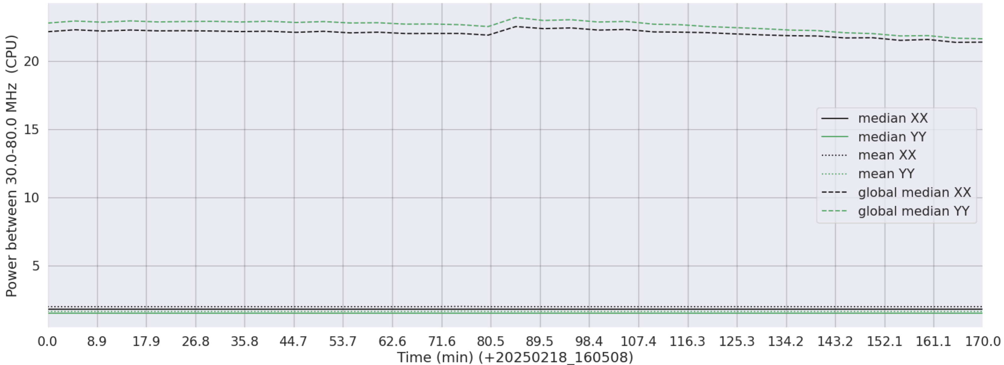
LWA287 - Correlator# 223 - XX FLAGS:LowPower - YY FLAGS:LowPower
