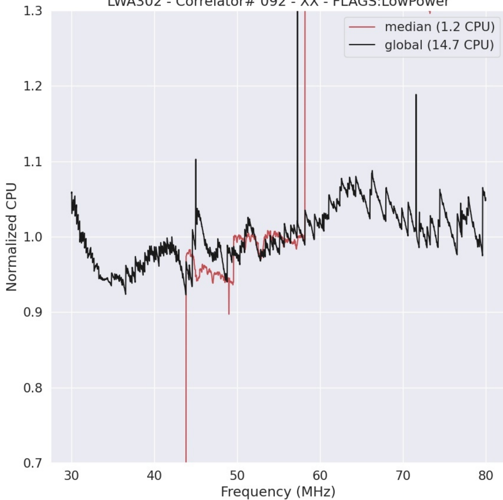
LWA302 - Correlator# 092 - XX - FLAGS:LowPower
