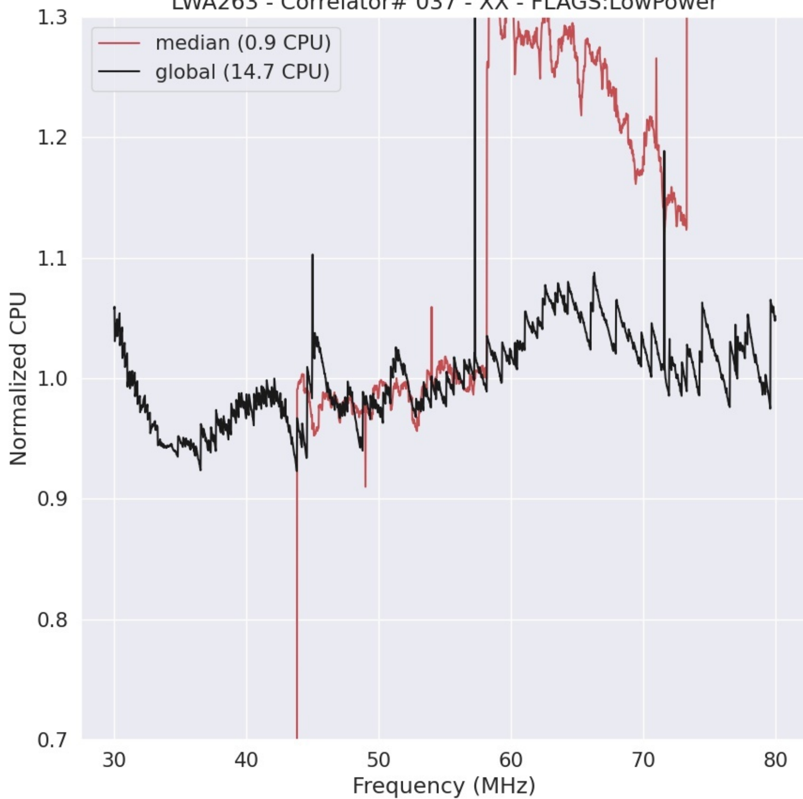
LWA263 - Correlator# 037 - XX - FLAGS:LowPower
