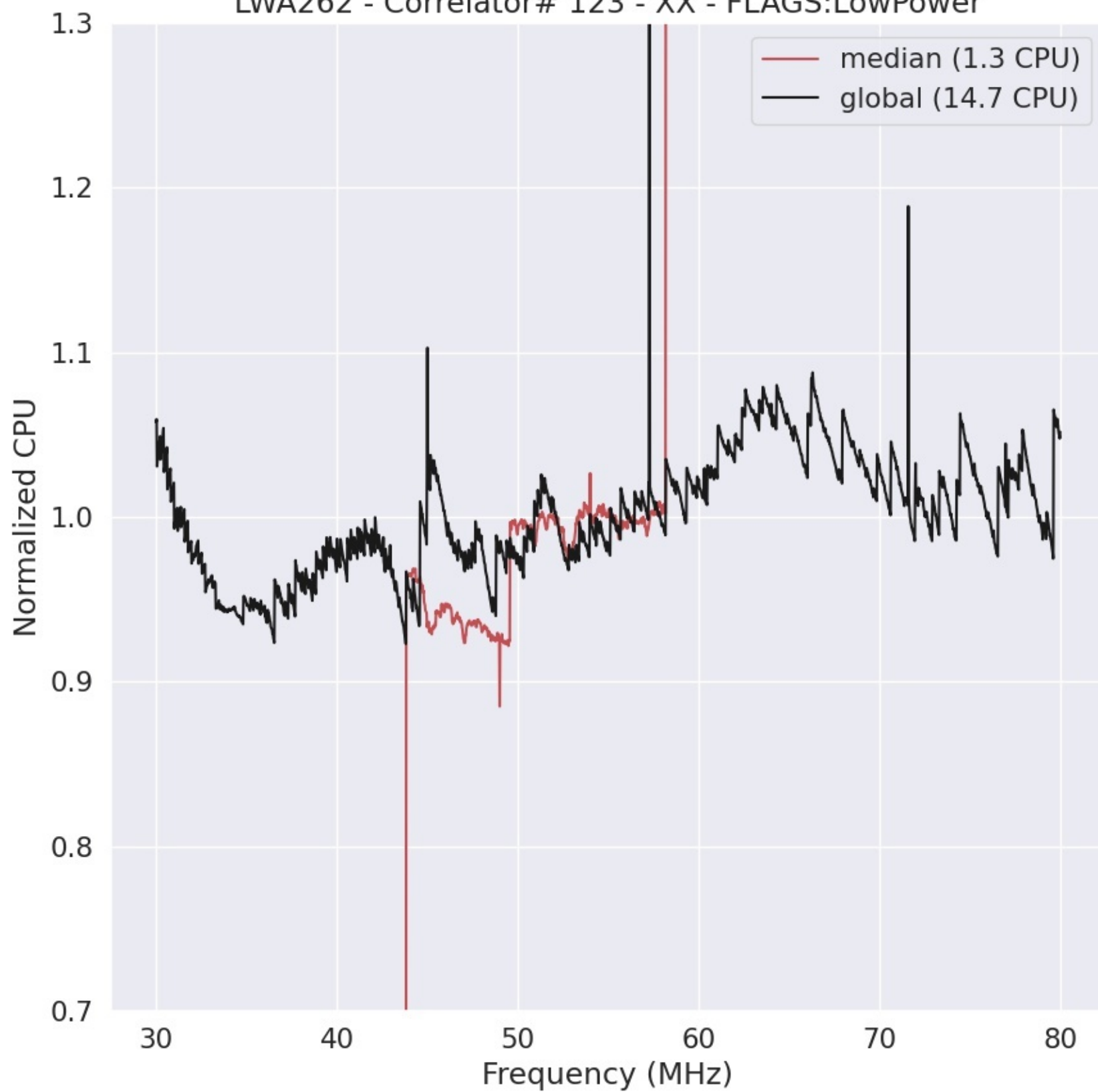
LWA262 - Correlator# 123 - XX - FLAGS:LowPower
