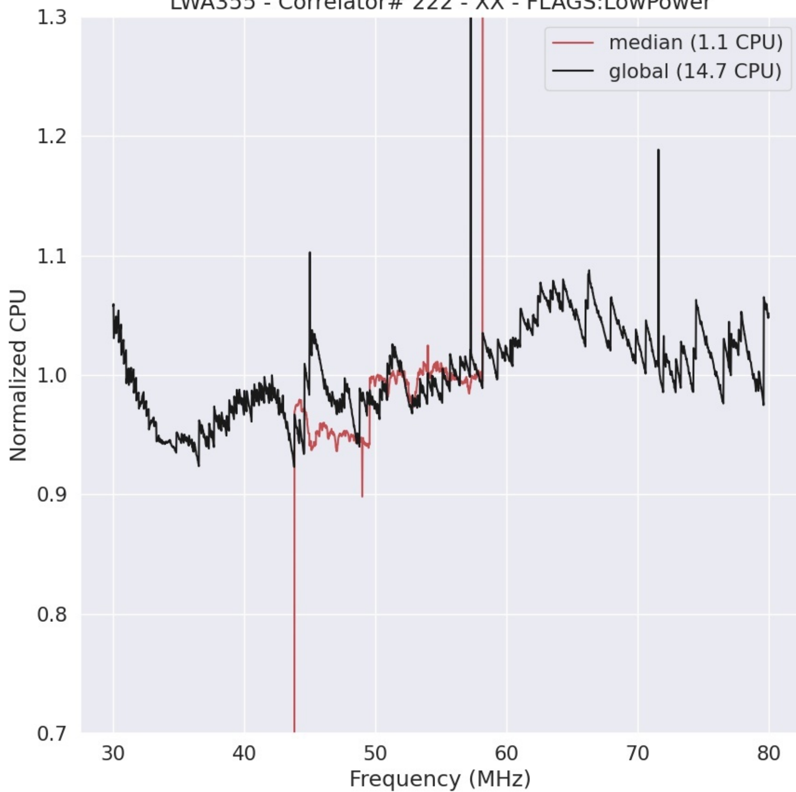
LWA355 - Correlator# 222 - XX - FLAGS:LowPower
