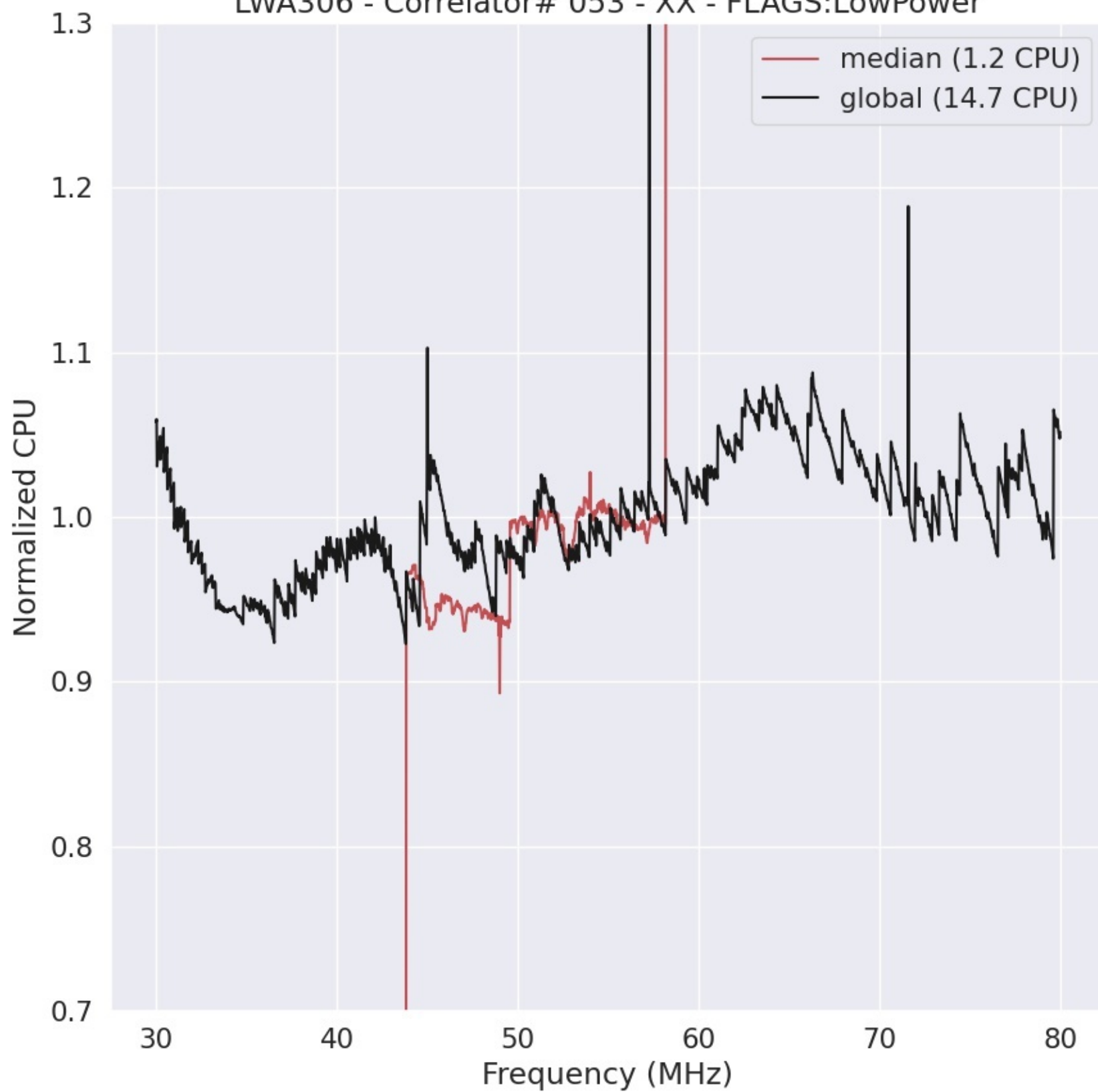
LWA306 - Correlator# 053 - XX - FLAGS:LowPower
