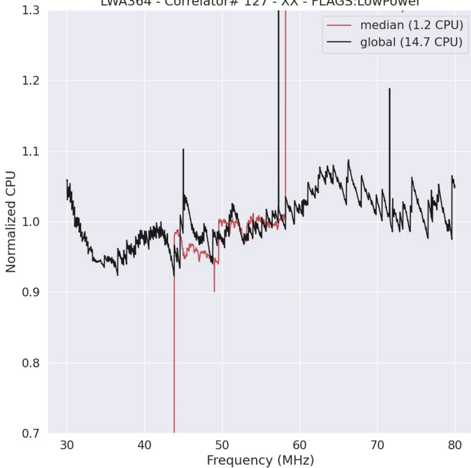
LWA364 - Correlator# 127 - XX - FLAGS:LowPower
