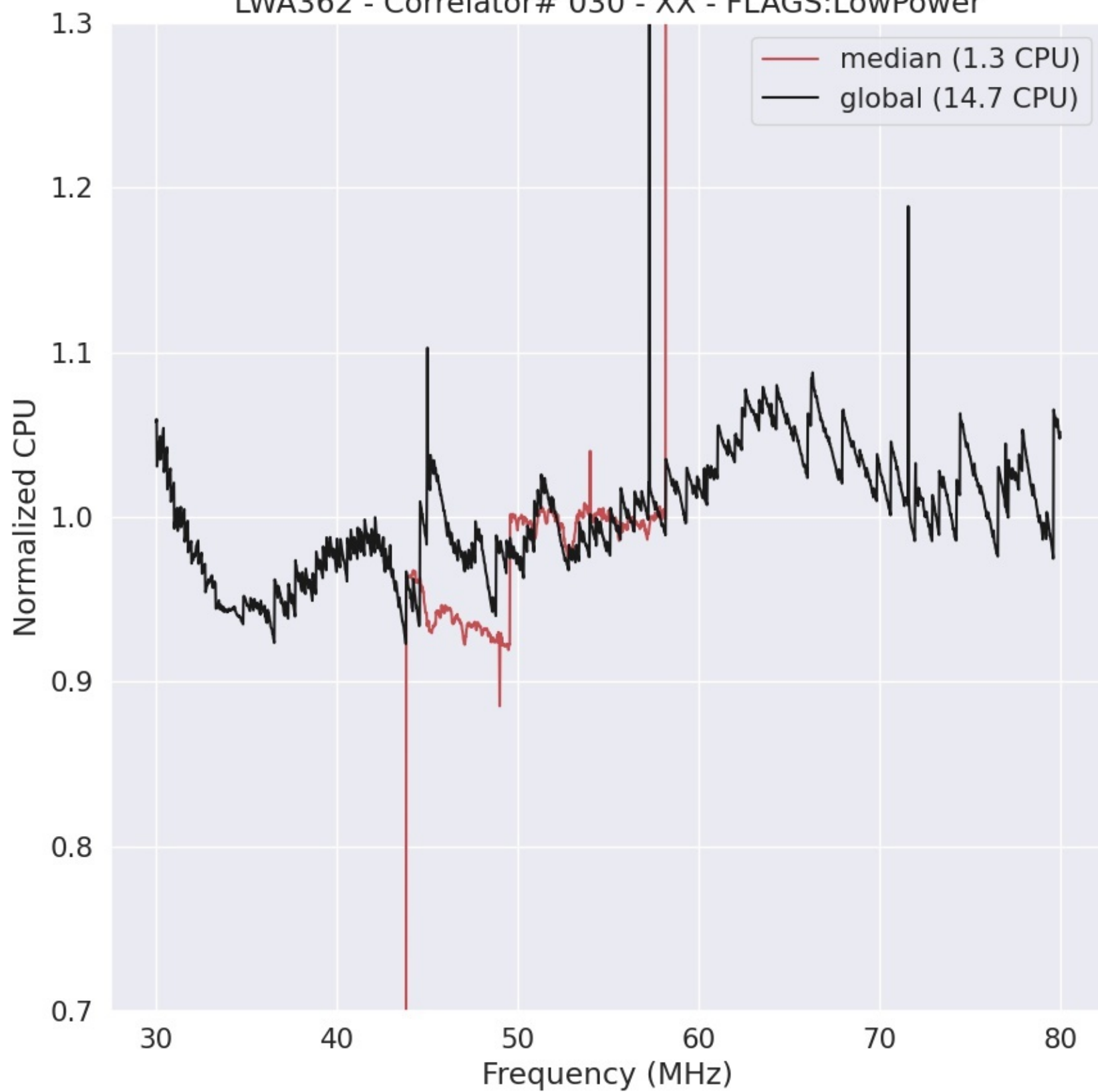
LWA362 - Correlator# 030 - XX - FLAGS:LowPower
