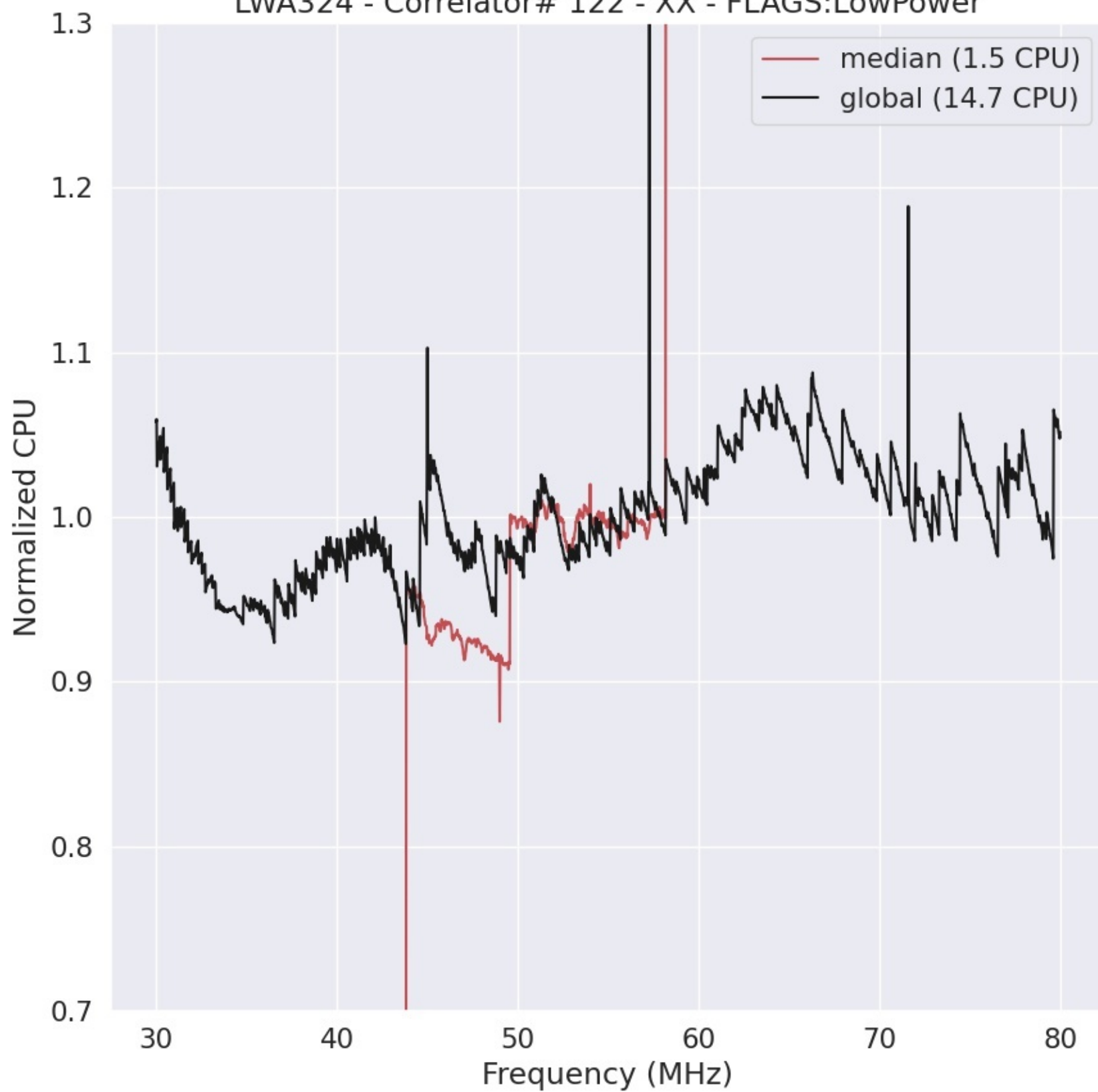
LWA324 - Correlator# 122 - XX - FLAGS:LowPower
