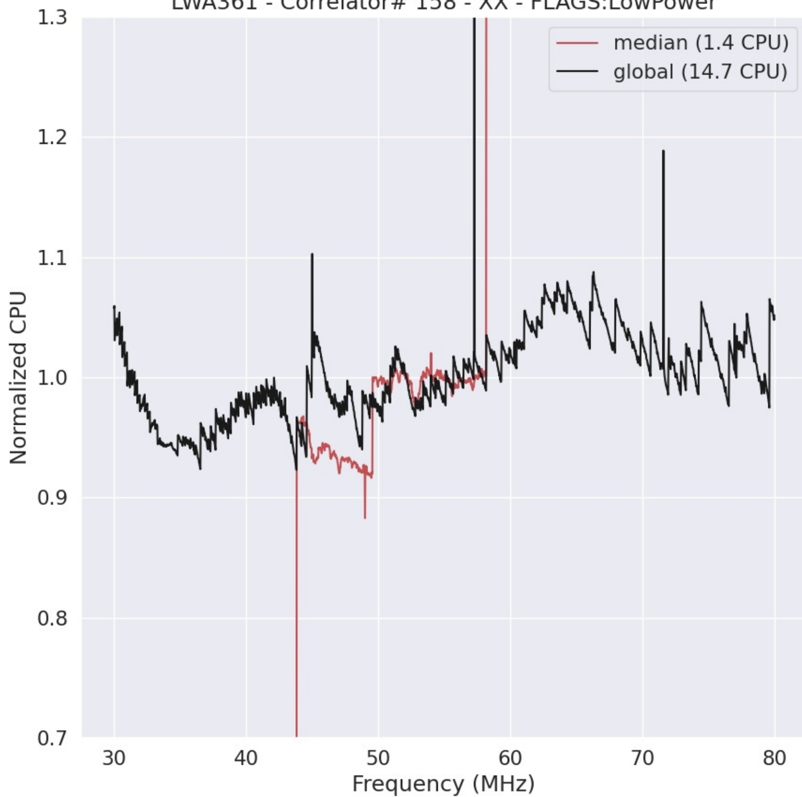
LWA361 - Correlator# 158 - XX - FLAGS:LowPower
