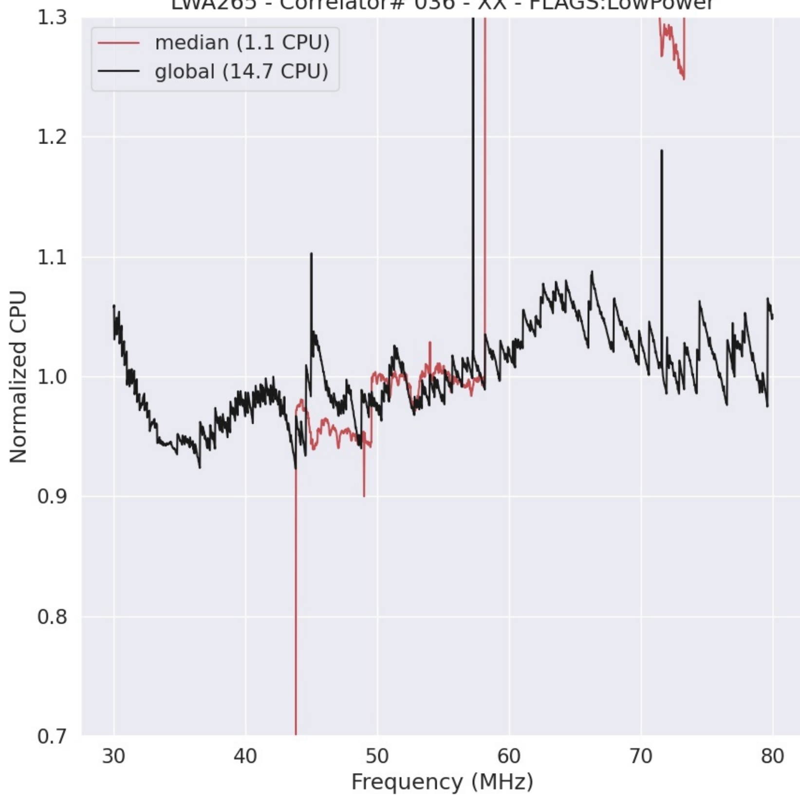
LWA265 - Correlator# 036 - XX - FLAGS:LowPower
