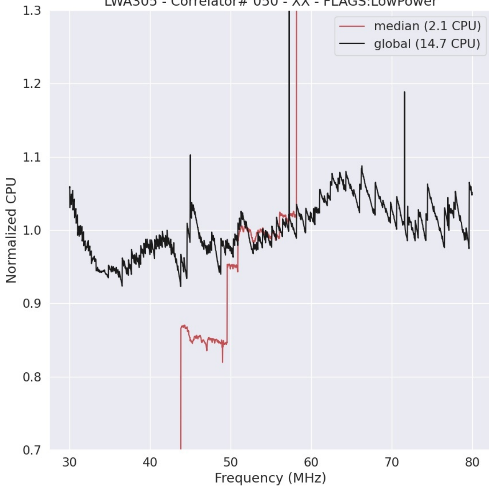
LWA305 - Correlator# 050 - XX - FLAGS:LowPower
