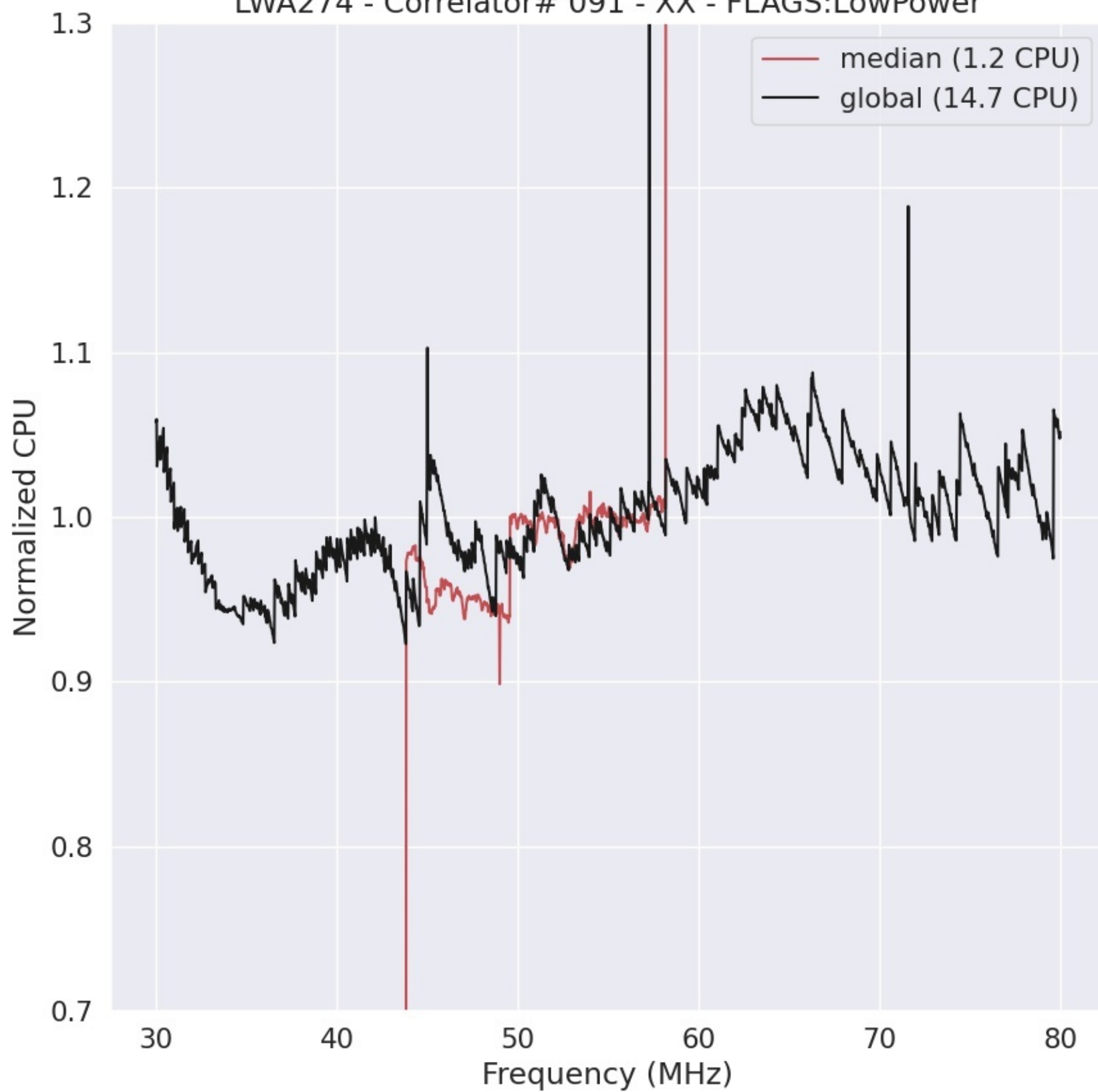
LWA274 - Correlator# 091 - XX - FLAGS:LowPower
