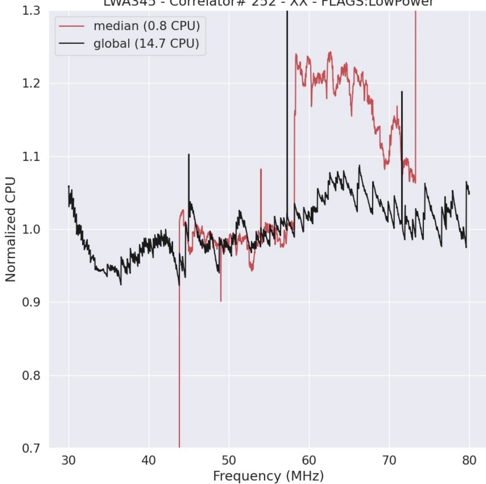
LWA345 - Correlator# 252 - XX - FLAGS:LowPower
