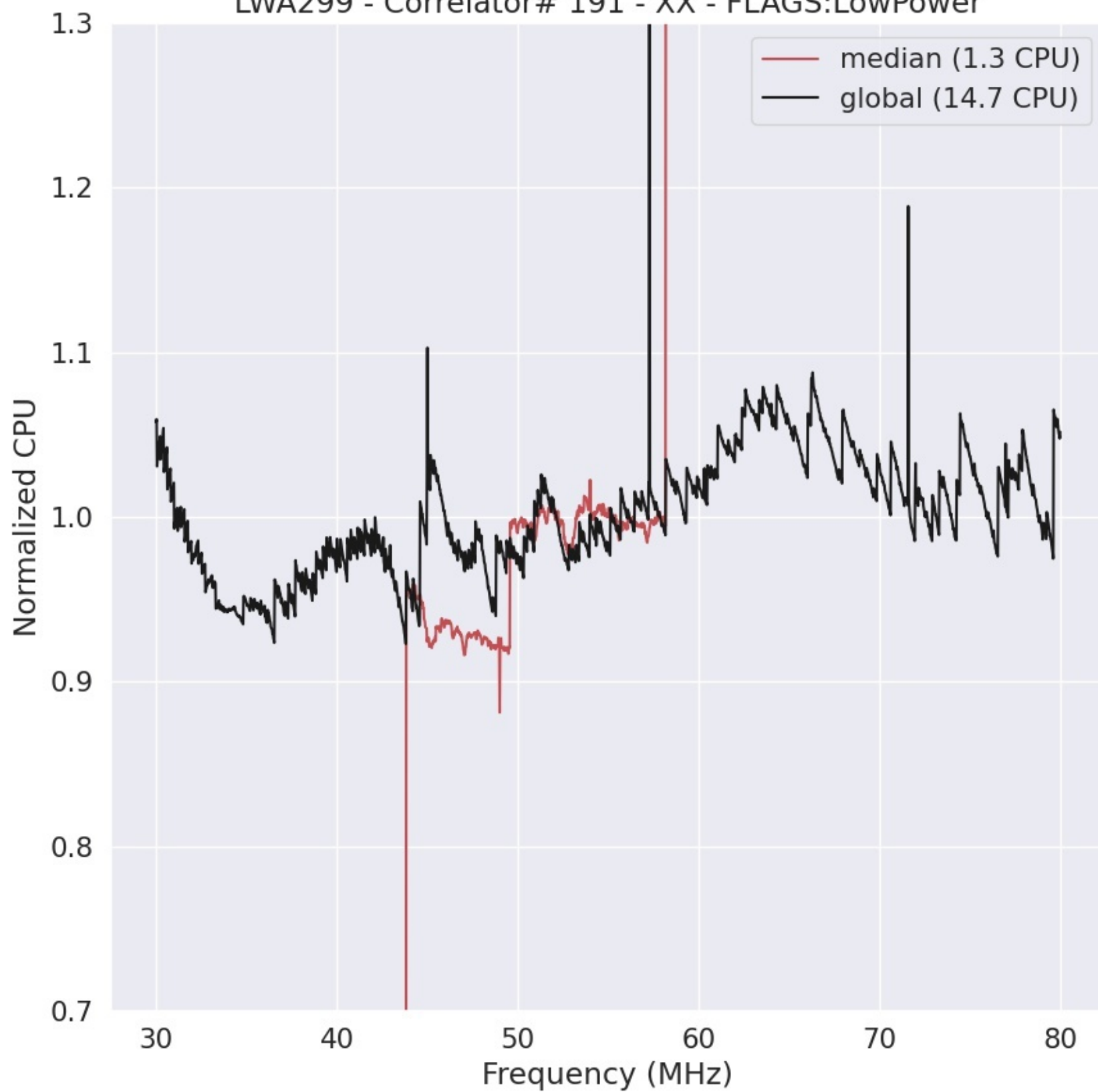
LWA299 - Correlator# 191 - XX - FLAGS:LowPower
