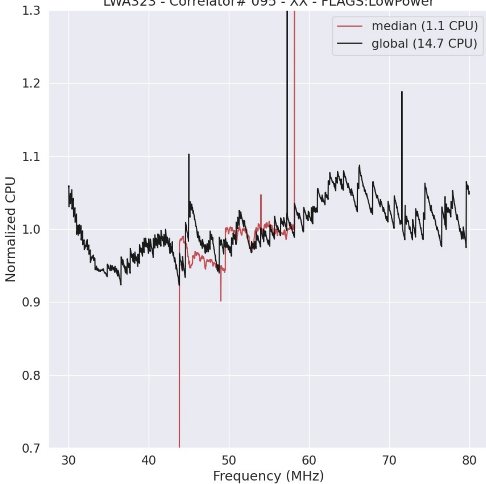
LWA323 - Correlator# 095 - XX - FLAGS:LowPower
