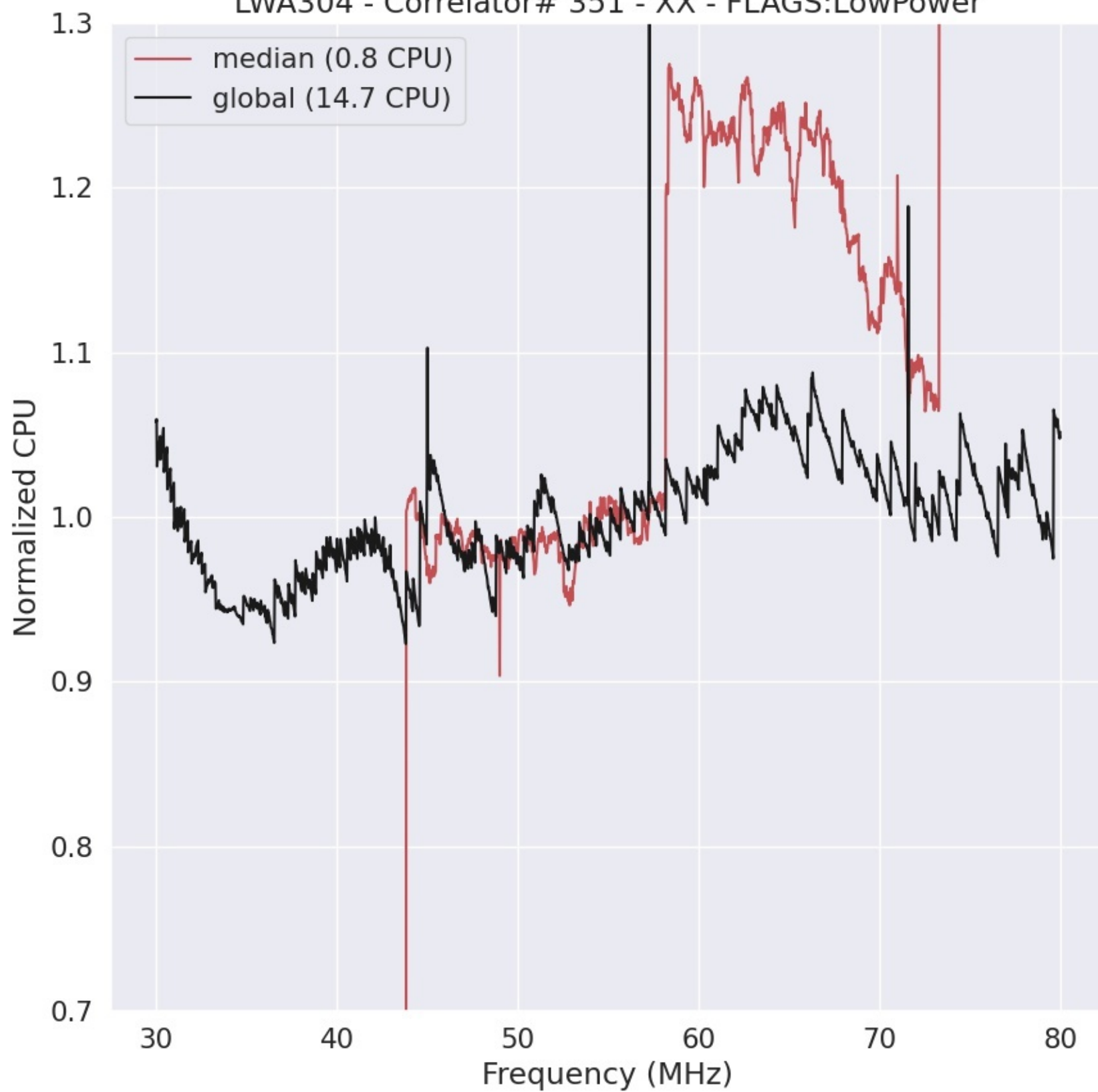
LWA304 - Correlator# 351 - XX - FLAGS:LowPower
