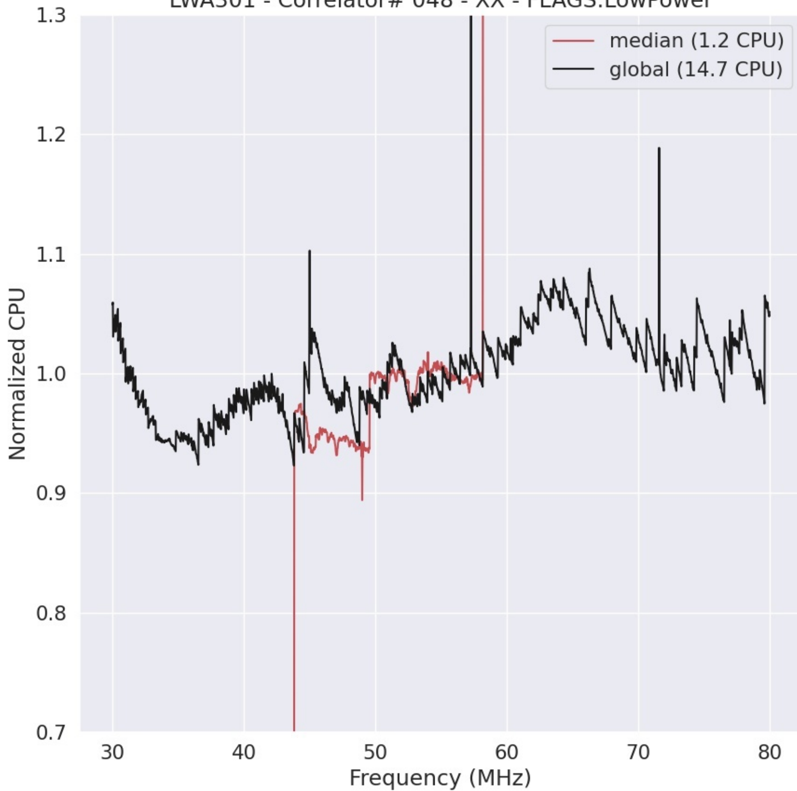
LWA301 - Correlator# 048 - XX - FLAGS:LowPower
