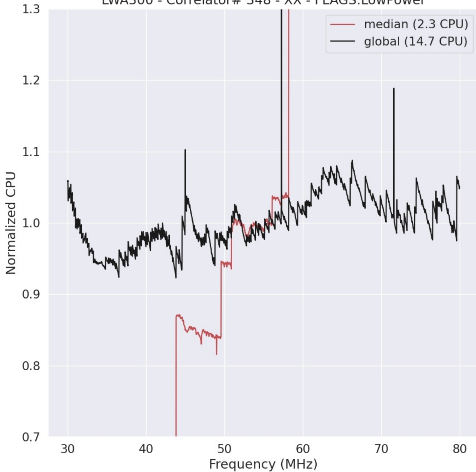
LWA300 - Correlator# 348 - XX - FLAGS:LowPower
