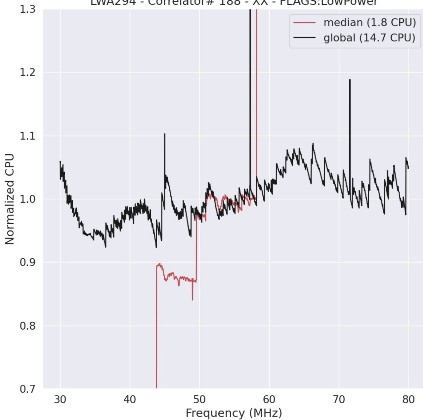
LWA294 - Correlator# 188 - XX - FLAGS:LowPower
