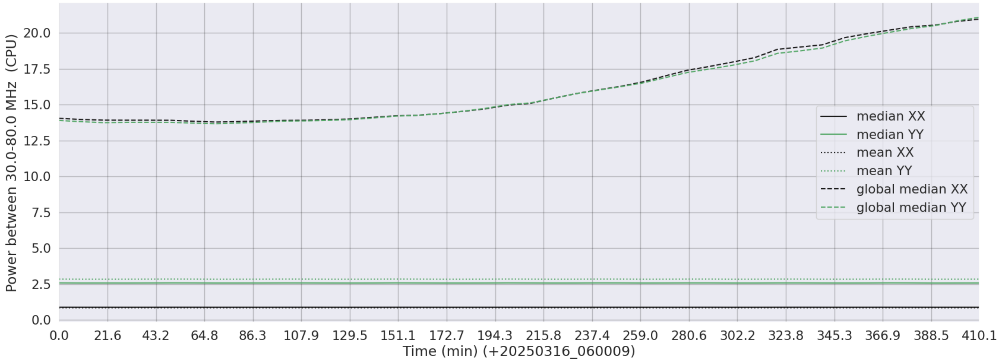
LWA308 - Correlator# 015 - XX FLAGS:LowPower - YY FLAGS:LowPower
