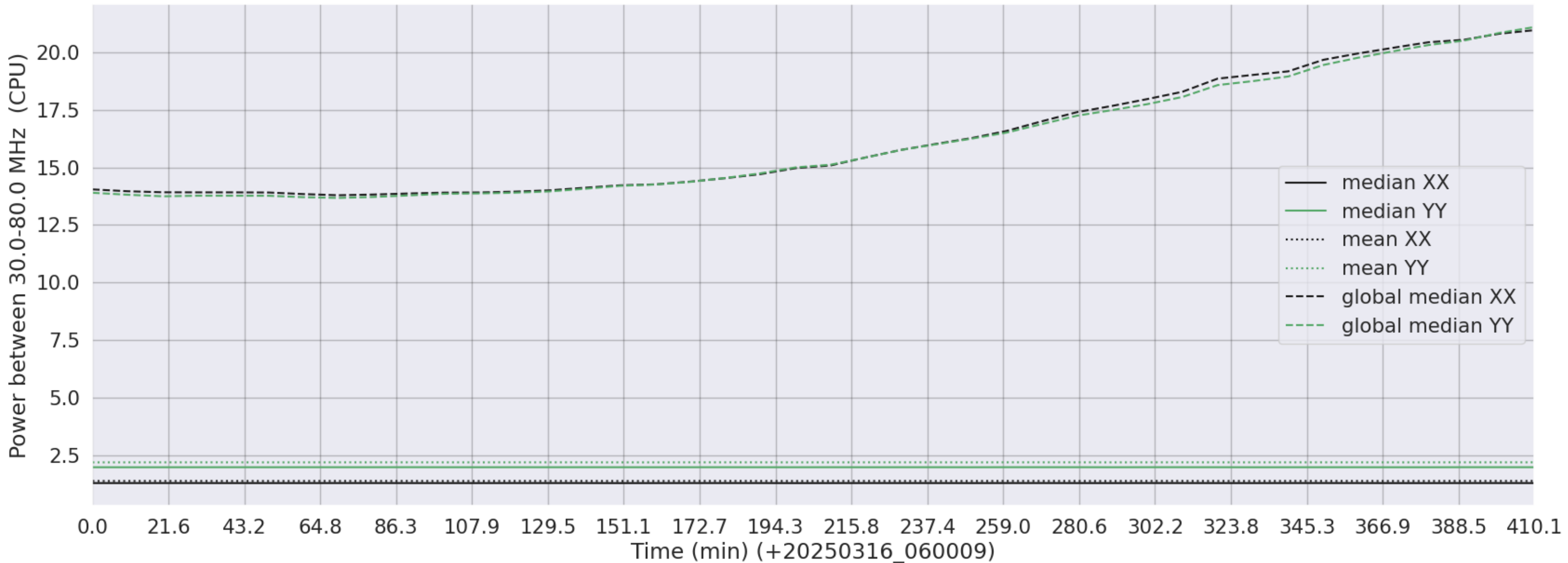
LWA259 - Correlator# 001 - XX FLAGS:LowPower - YY FLAGS:LowPower
