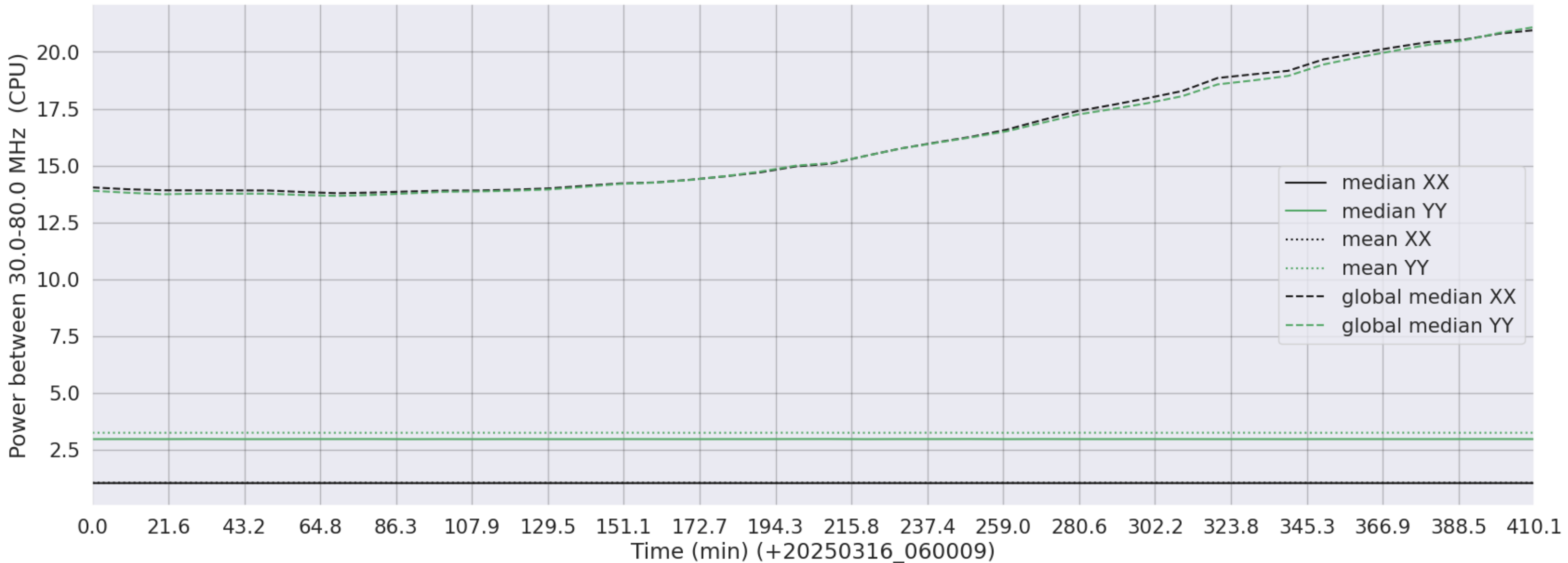
LWA344 - Correlator# 061 - XX FLAGS:LowPower - YY FLAGS:LowPower
