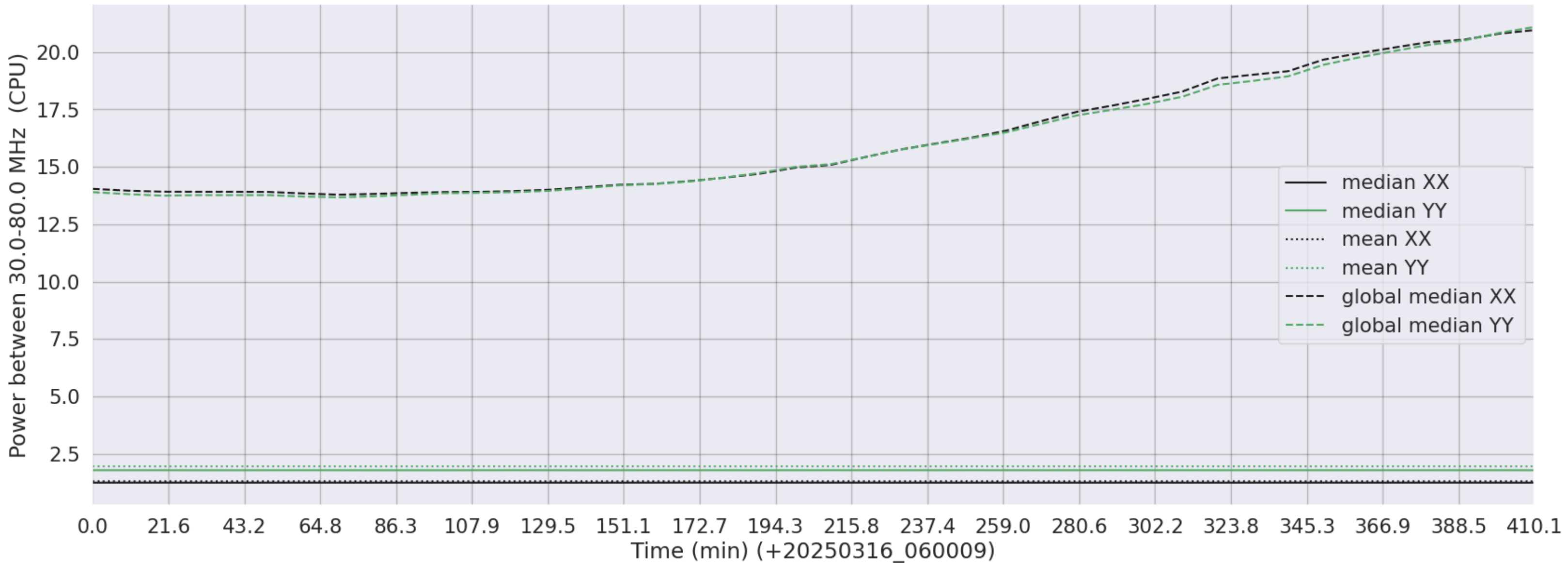
LWA343 - Correlator# 058 - XX FLAGS:LowPower - YY FLAGS:LowPower
