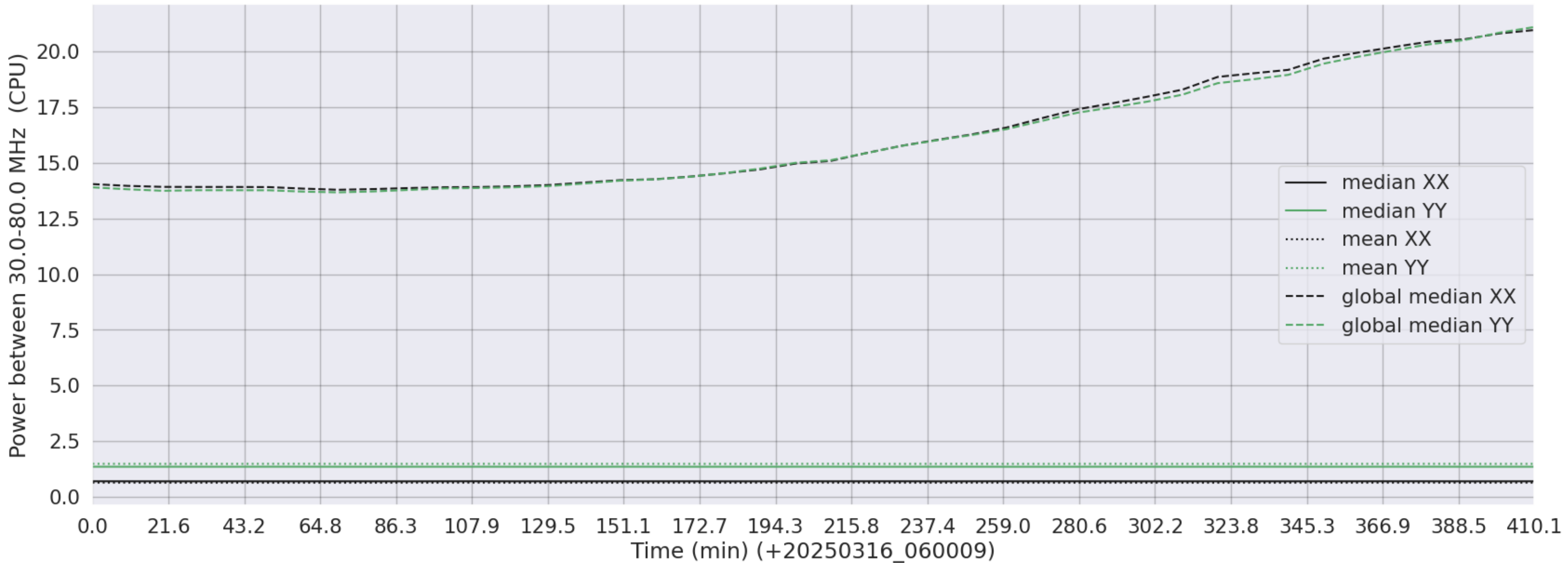
LWA322 - Correlator# 251 - XX FLAGS:LowPower - YY FLAGS:LowPower
