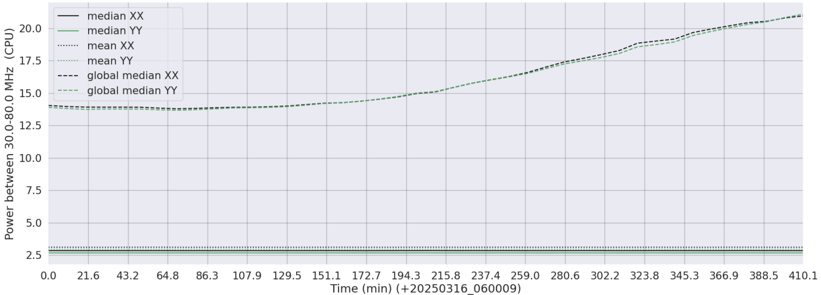
LWA338 - Correlator# 024 - XX FLAGS:LowPower - YY FLAGS:LowPower
