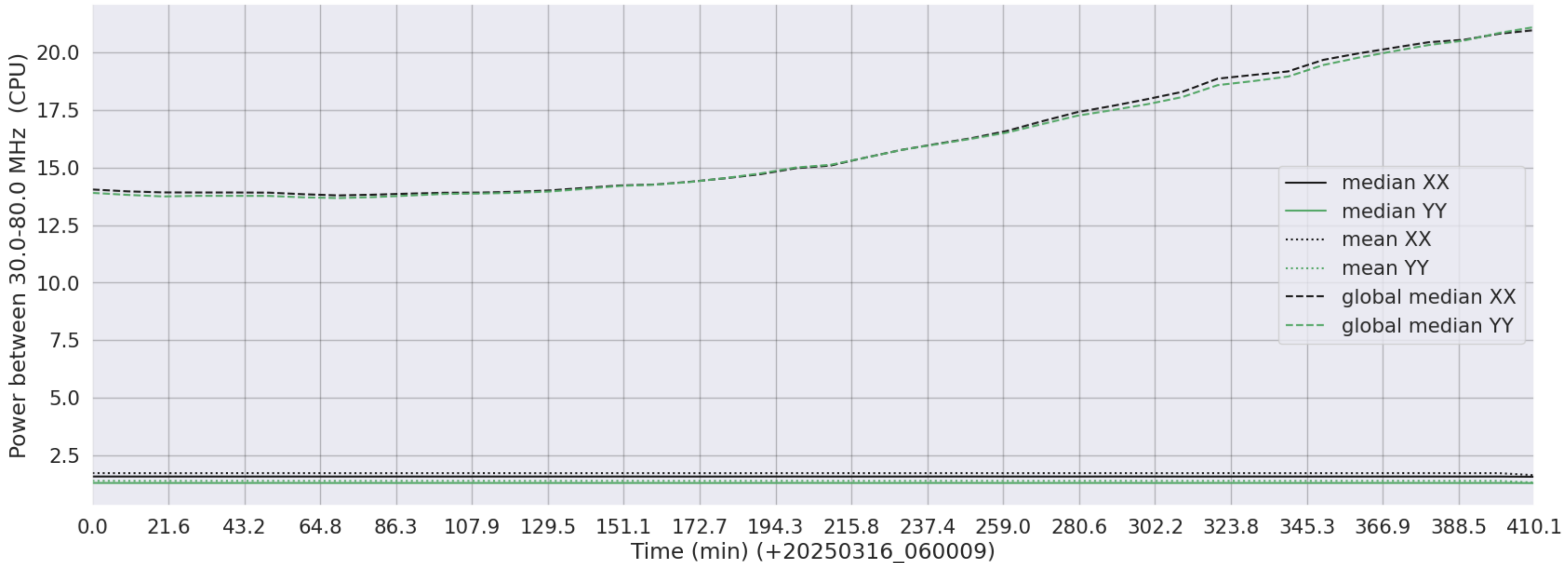
LWA270 - Correlator# 039 - XX FLAGS:LowPower - YY FLAGS:LowPower
