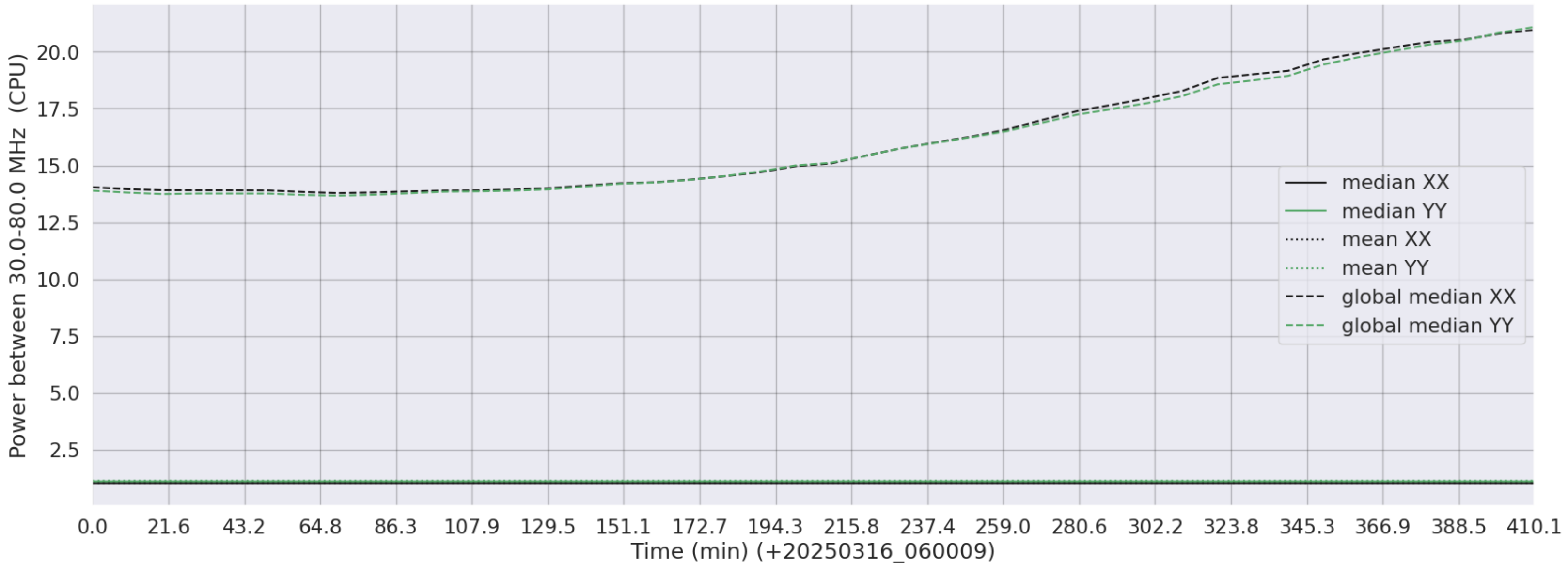
LWA278 - Correlator# 008 - XX FLAGS:LowPower - YY FLAGS:LowPower
