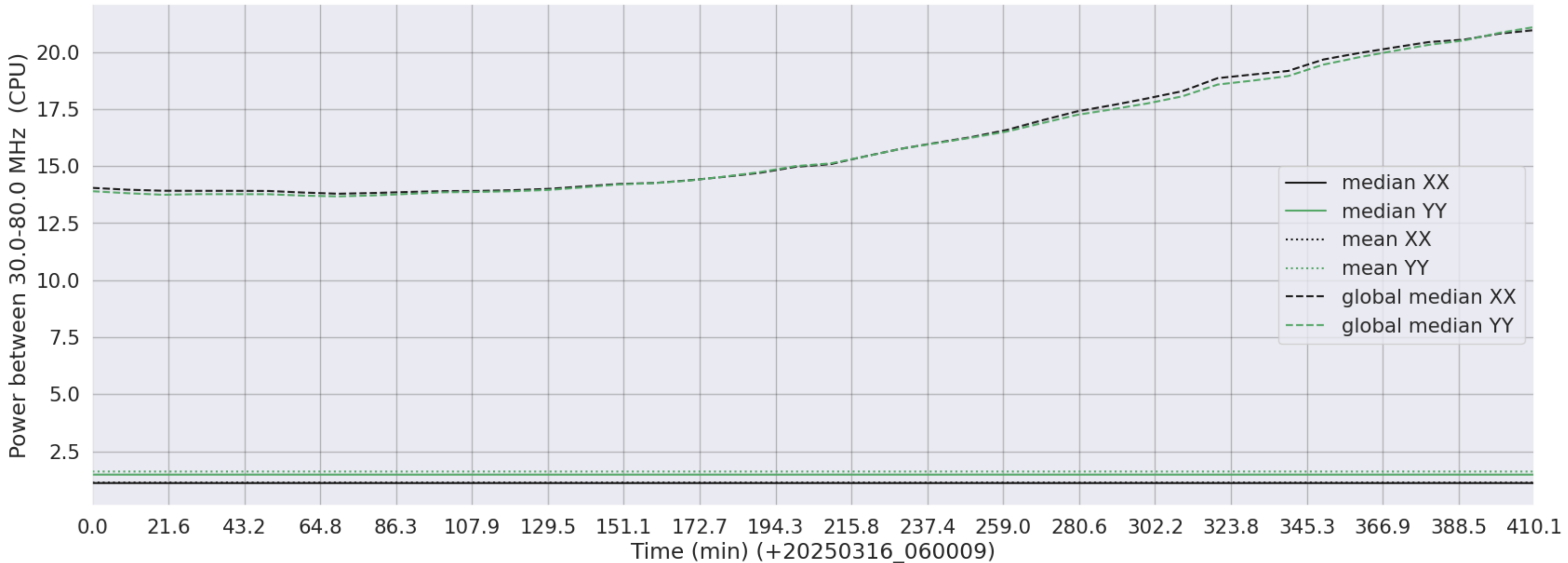
LWA268 - Correlator# 002 - XX FLAGS:LowPower - YY FLAGS:LowPower
