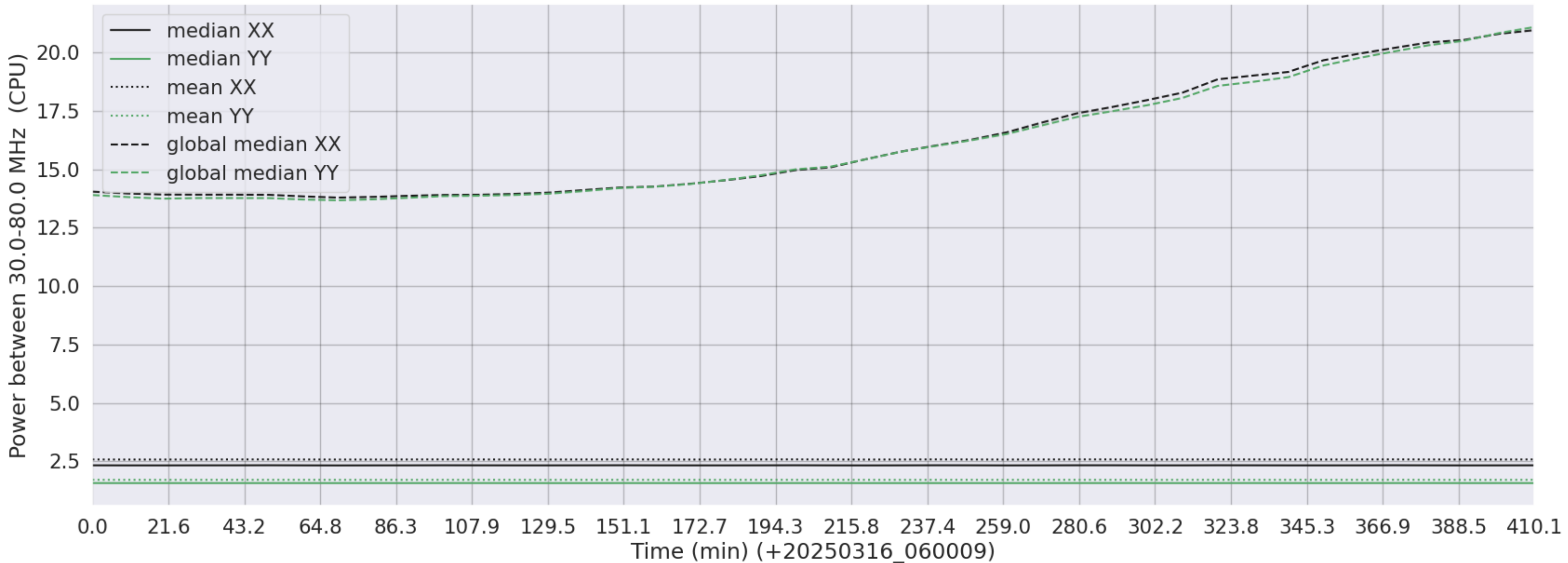
LWA330 - Correlator# 022 - XX FLAGS:LowPower - YY FLAGS:LowPower
