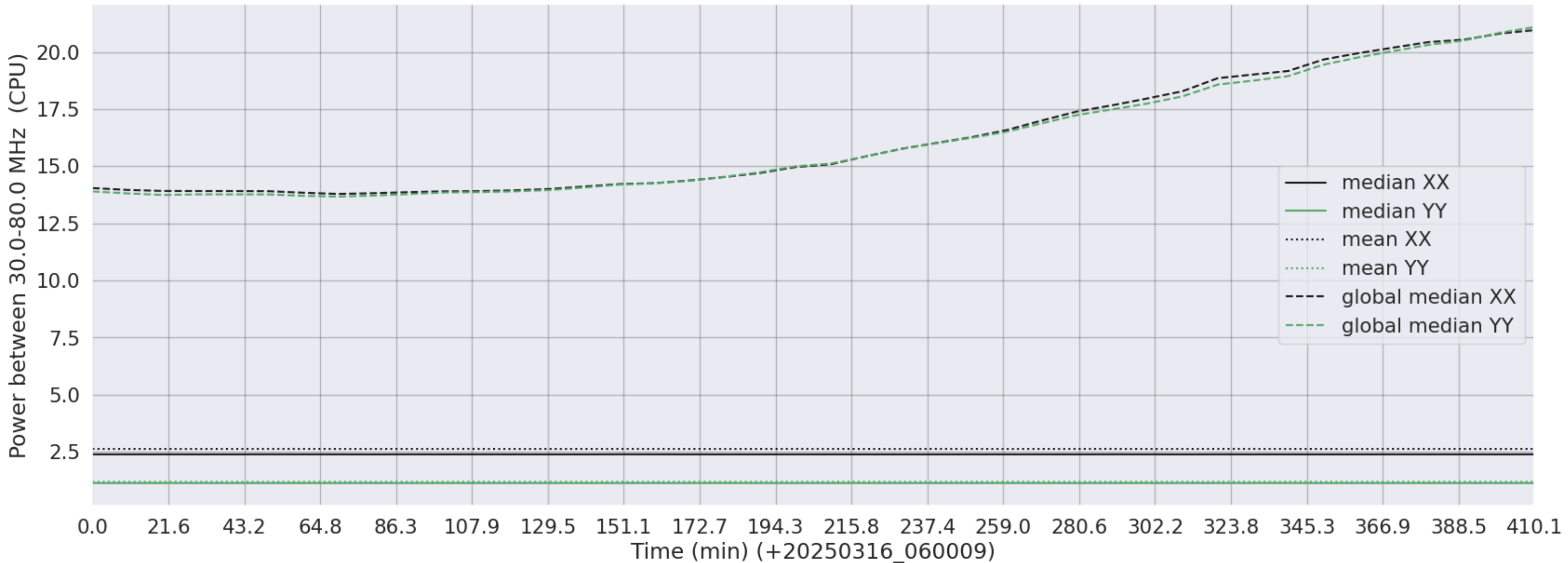
LWA288 - Correlator# 042 - XX FLAGS:LowPower - YY FLAGS:LowPower
