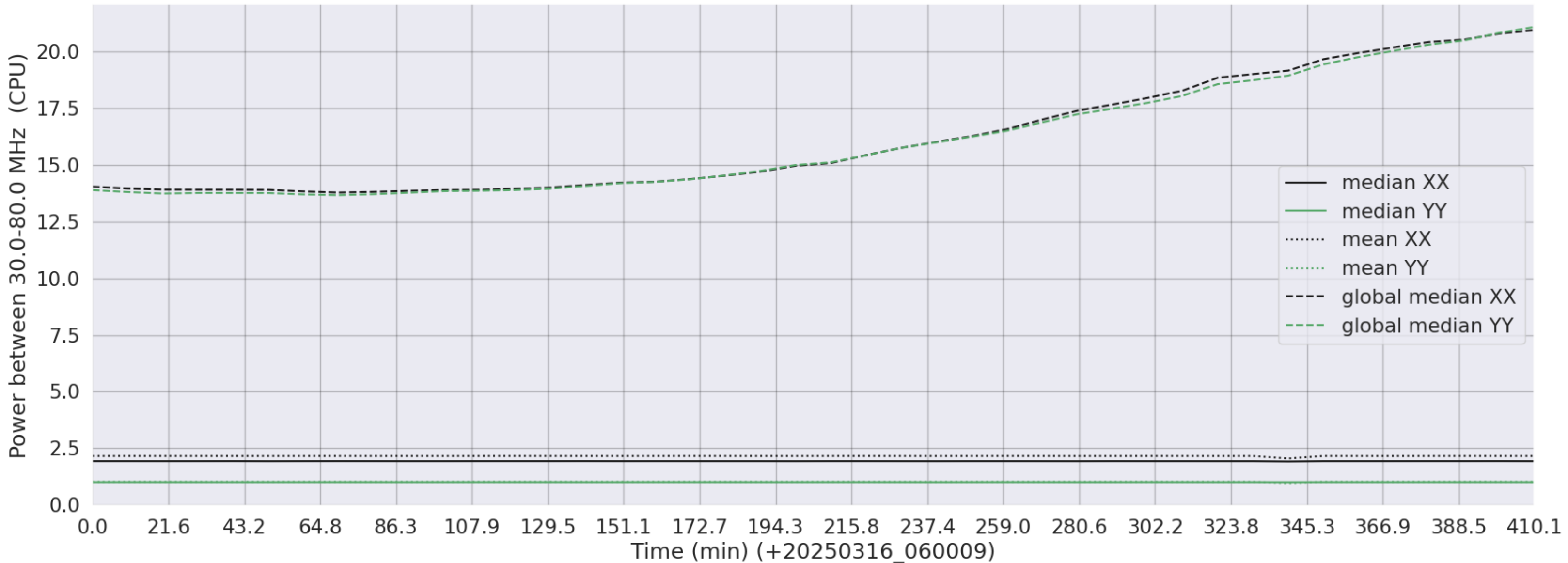
LWA331 - Correlator# 125 - XX FLAGS:LowPower - YY FLAGS:LowPower
