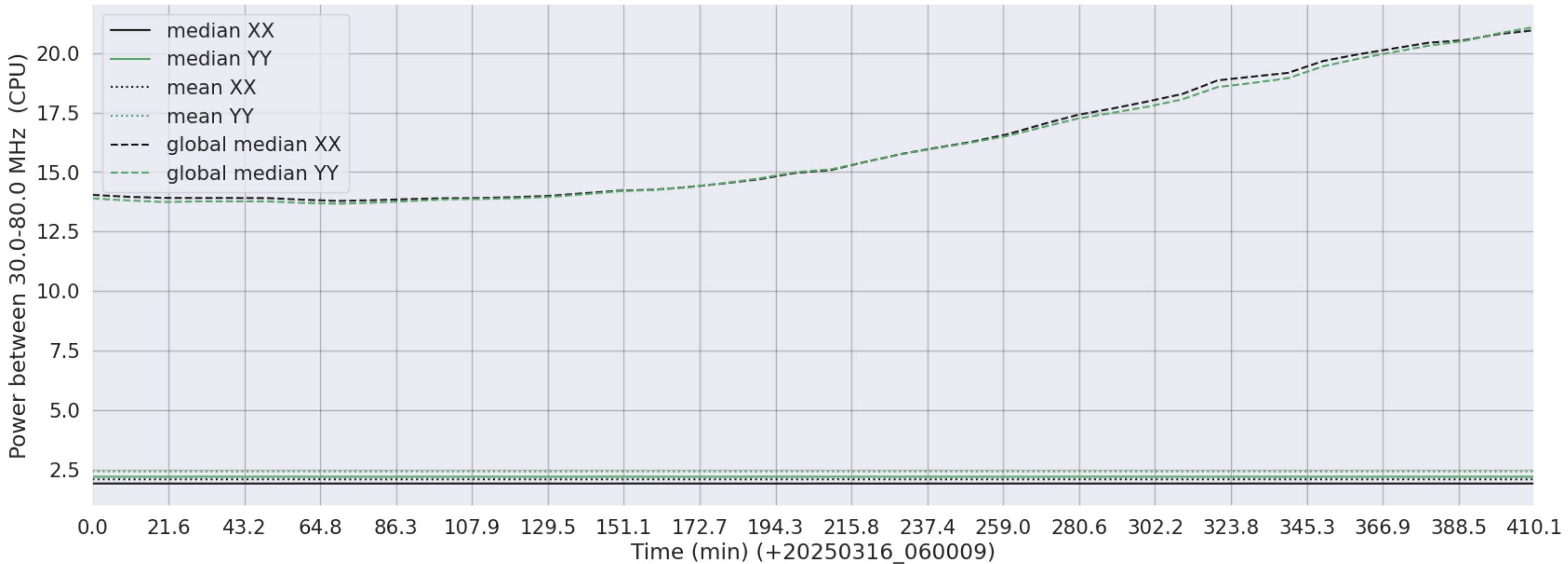
LWA279 - Correlator# 220 - XX FLAGS:LowPower - YY FLAGS:LowPower
