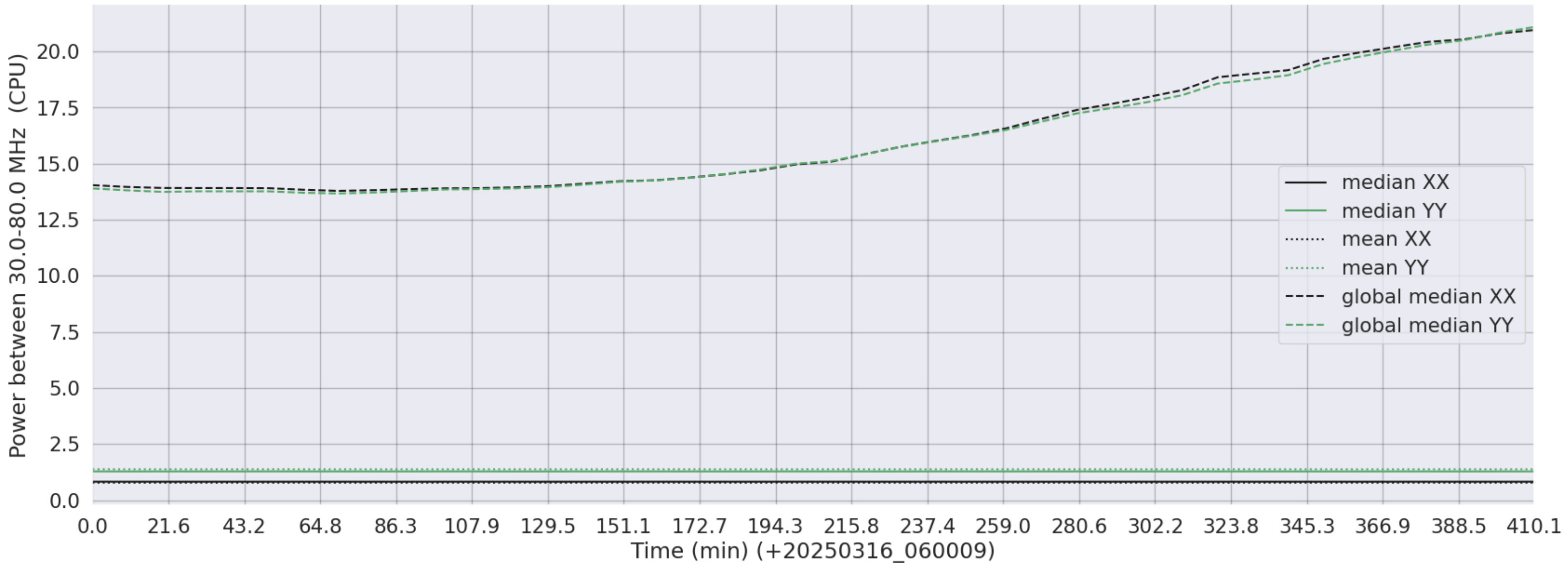
LWA267 - Correlator# 003 - XX FLAGS:LowPower - YY FLAGS:LowPower
