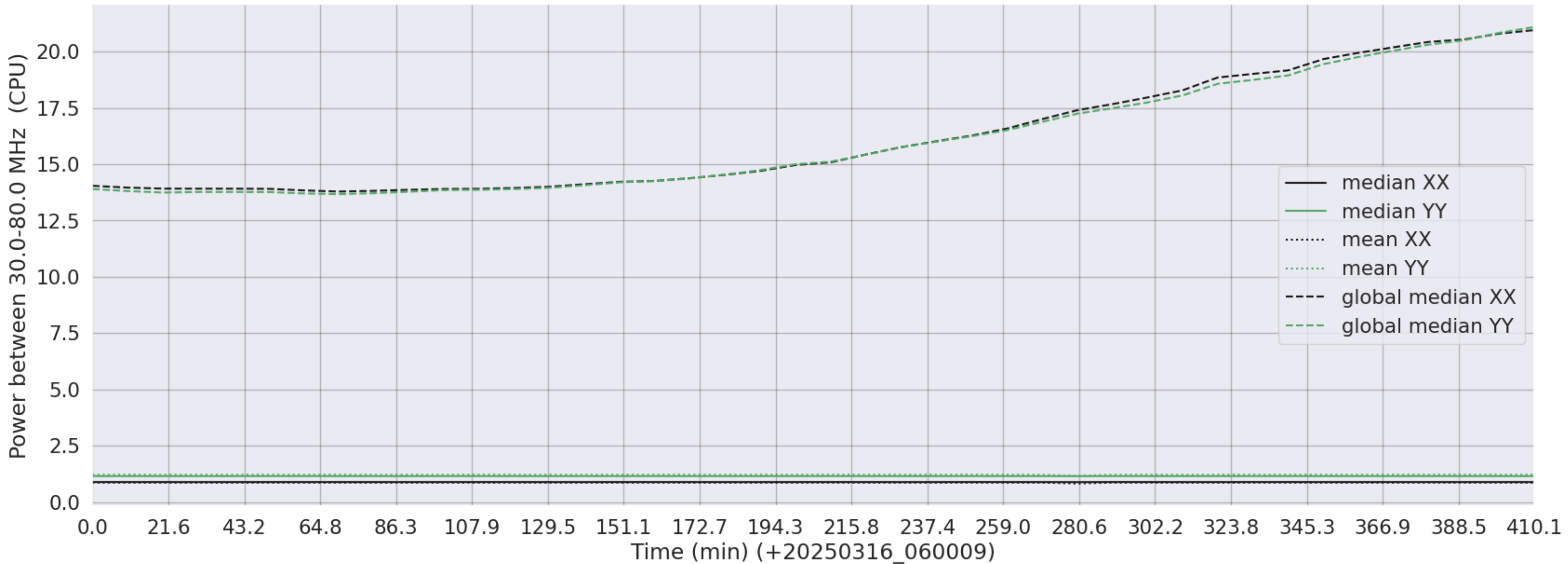
LWA325 - Correlator# 154 - XX FLAGS:LowPower - YY FLAGS:LowPower
