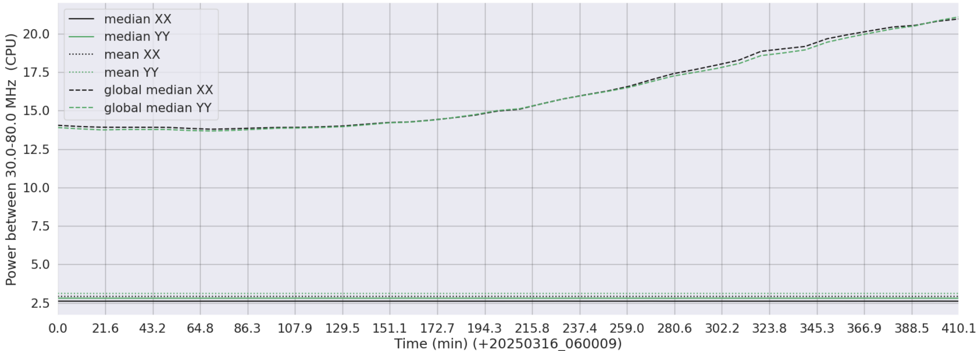
LWA275 - Correlator# 090 - XX FLAGS:LowPower - YY FLAGS:LowPower
