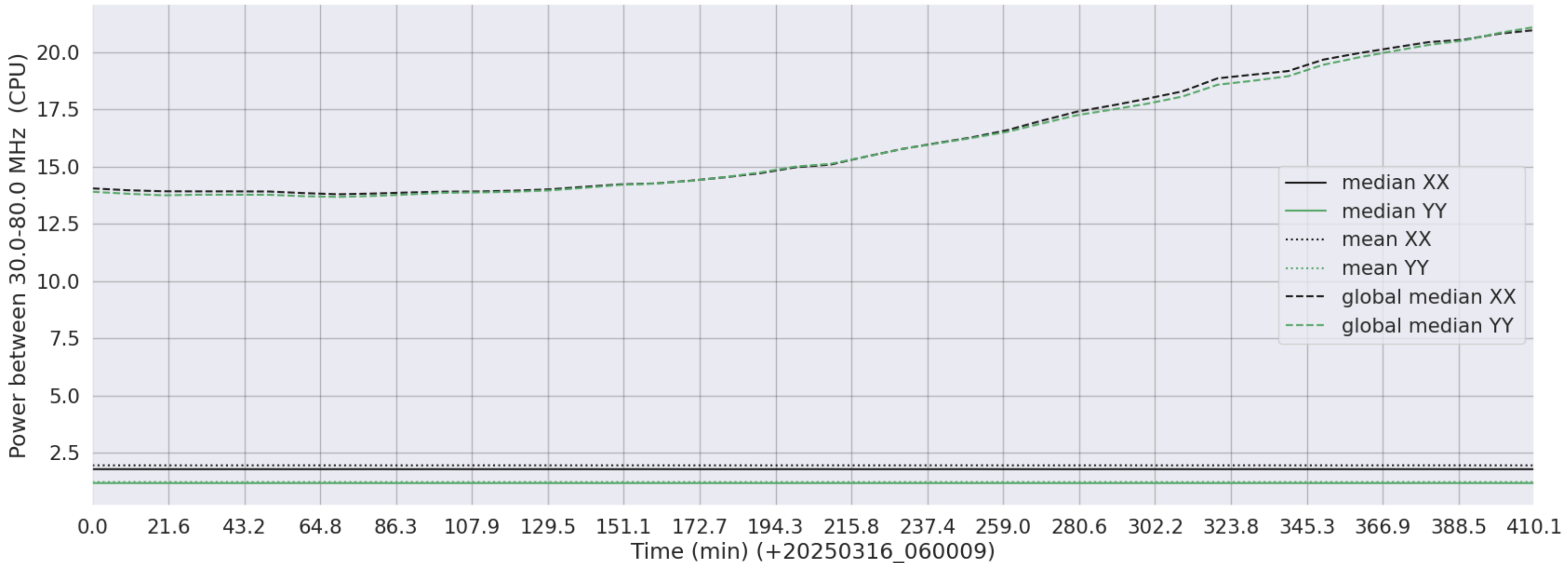
LWA351 - Correlator# 060 - XX FLAGS:LowPower - YY FLAGS:LowPower
