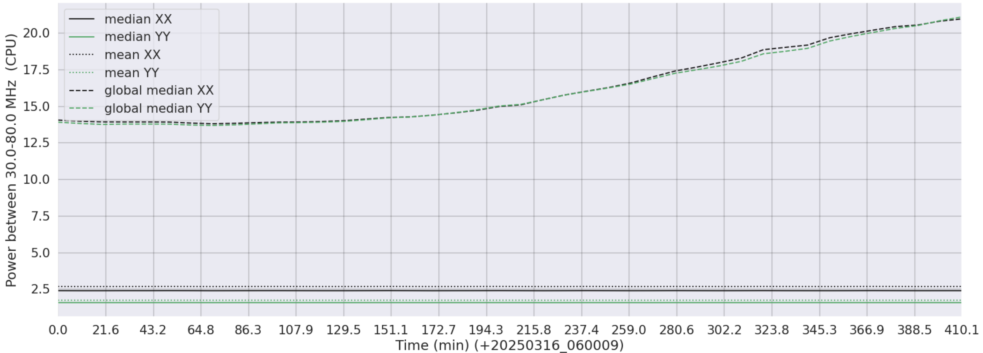
LWA333 - Correlator# 253 - XX FLAGS:LowPower - YY FLAGS:LowPower
