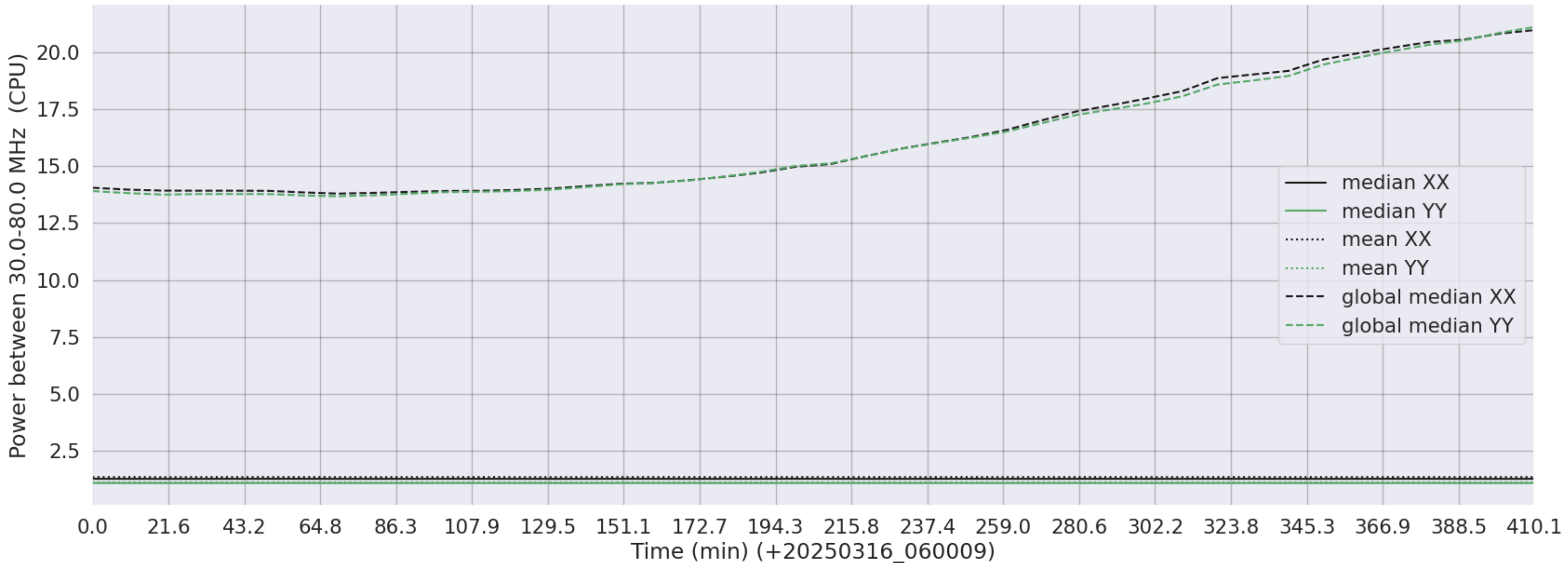
LWA309 - Correlator# 014 - XX FLAGS:LowPower - YY FLAGS:LowPower
