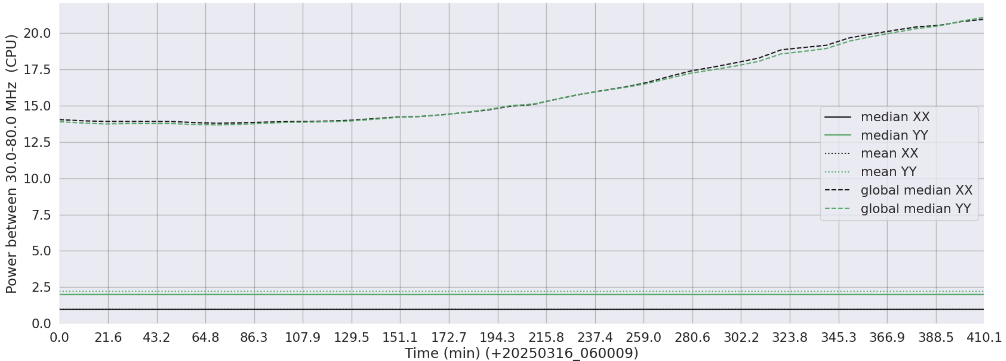
LWA257 - Correlator# 032 - XX FLAGS:LowPower - YY FLAGS:LowPower
