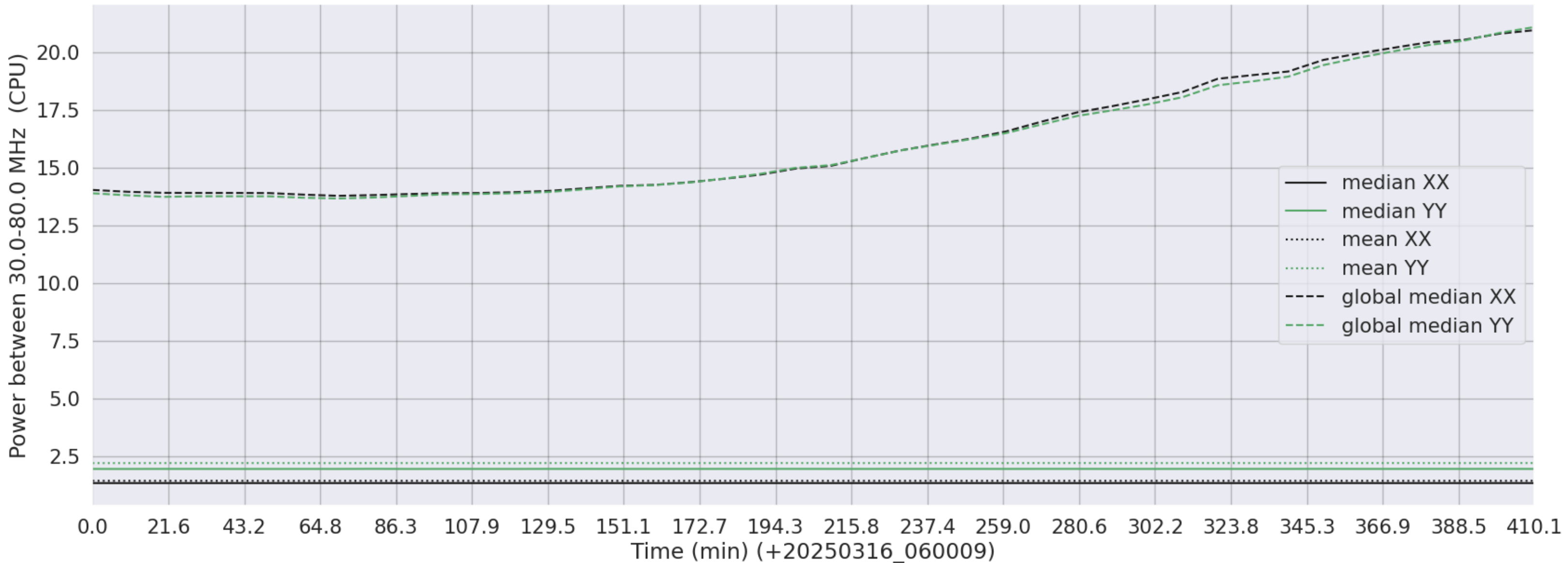
LWA266 - Correlator# 000 - XX FLAGS:LowPower - YY FLAGS:LowPower
