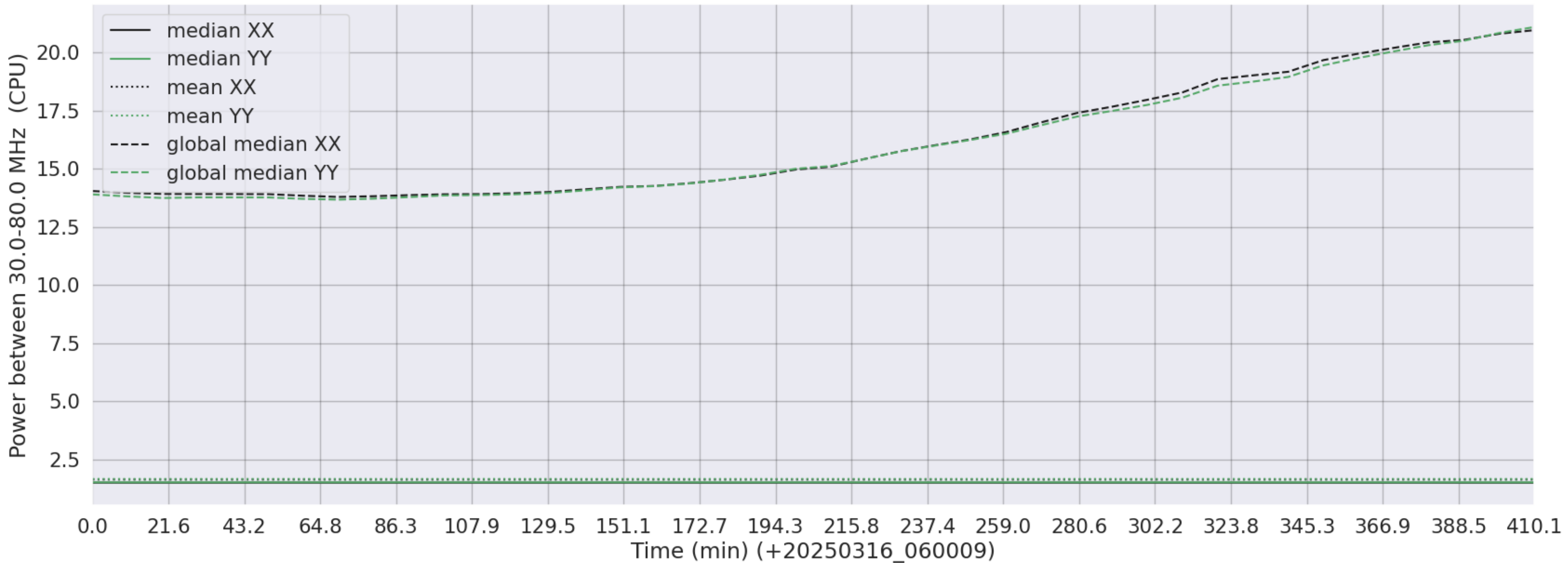
LWA298 - Correlator# 049 - XX FLAGS:LowPower - YY FLAGS:LowPower
