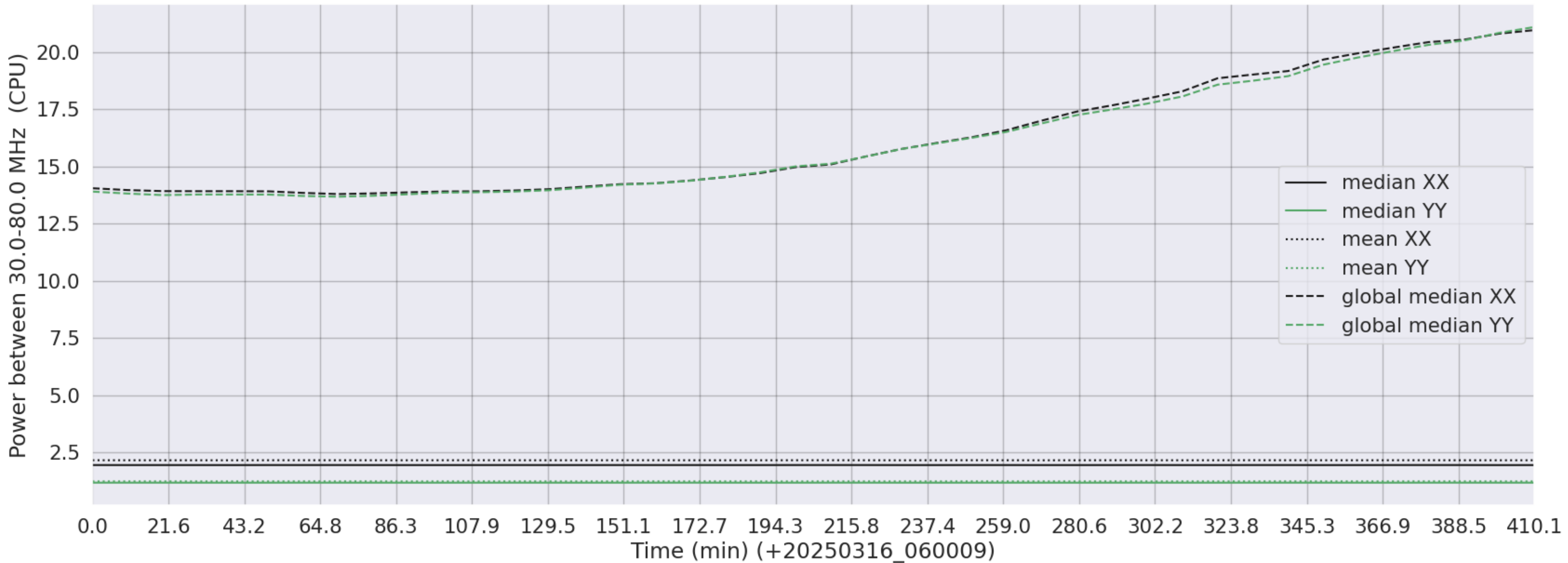
LWA329 - Correlator# 287 - XX FLAGS:LowPower - YY FLAGS:LowPower
