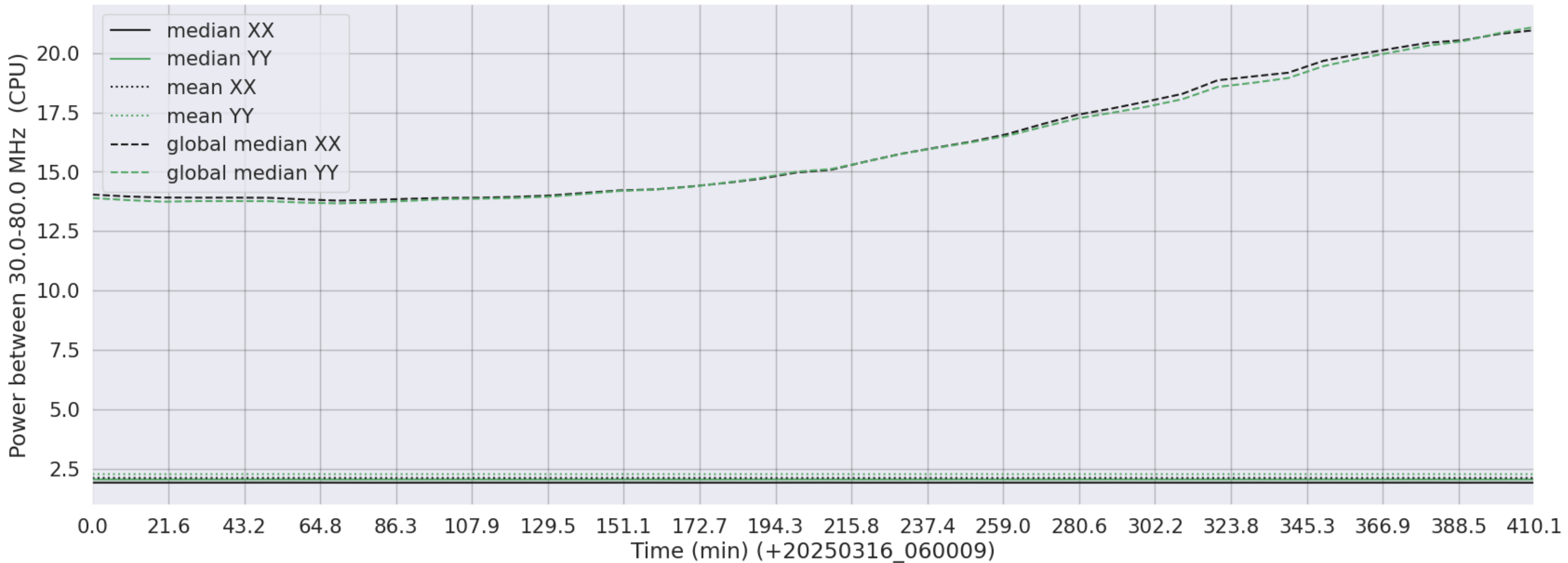
LWA312 - Correlator# 019 - XX FLAGS:LowPower - YY FLAGS:LowPower
