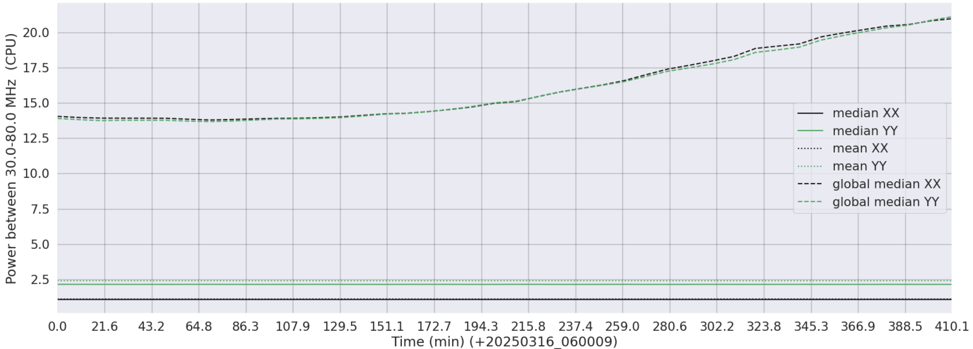
LWA311 - Correlator# 016 - XX FLAGS:LowPower - YY FLAGS:LowPower
