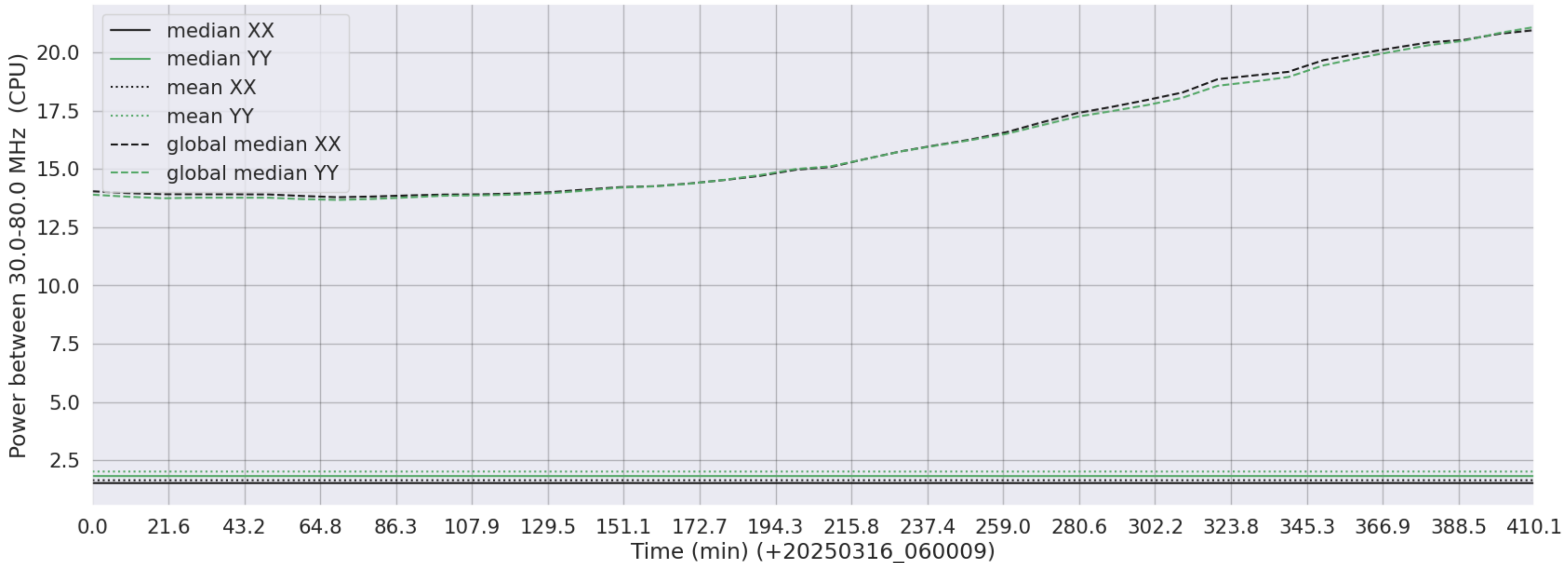
LWA327 - Correlator# 023 - XX FLAGS:LowPower - YY FLAGS:LowPower
