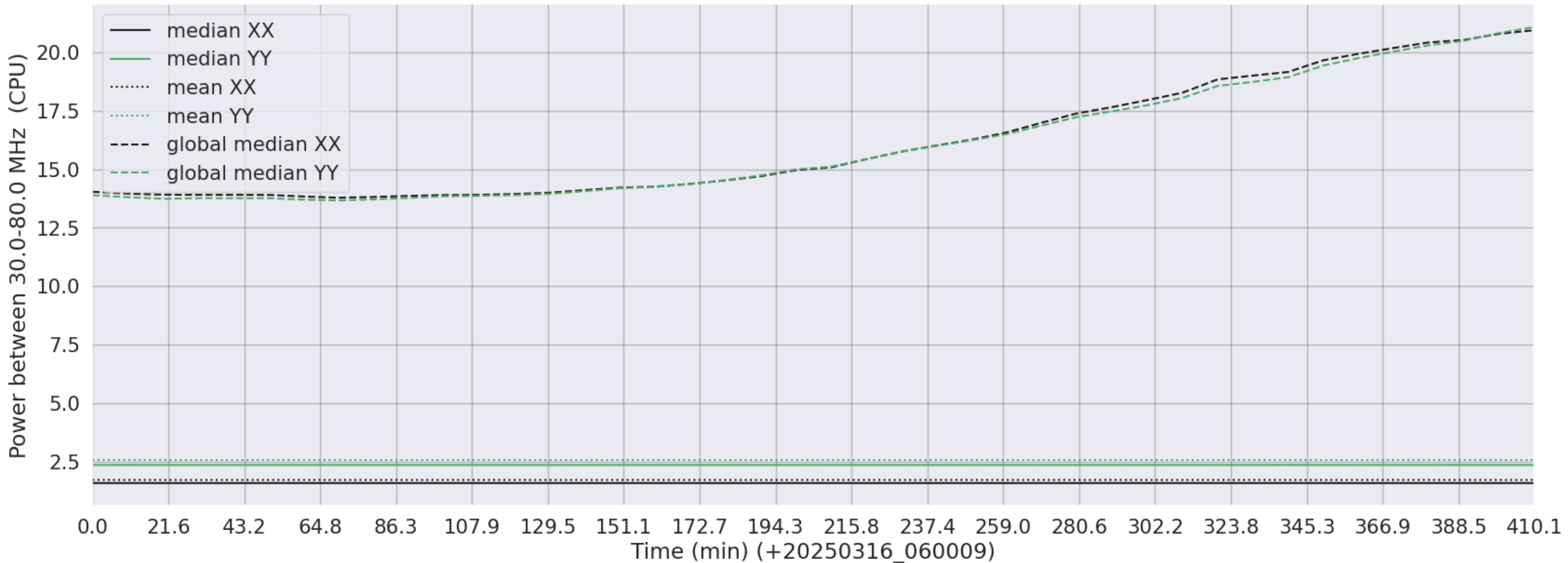
LWA337 - Correlator# 059 - XX FLAGS:LowPower - YY FLAGS:LowPower
