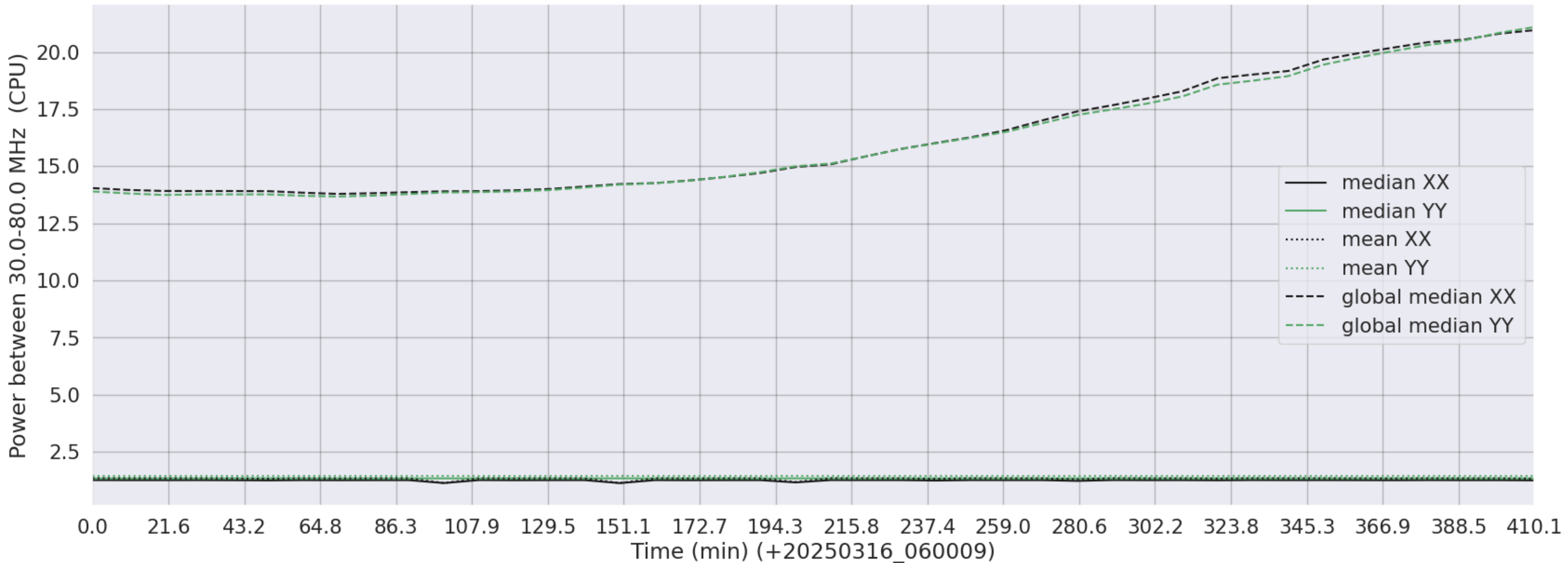
LWA349 - Correlator# 282 - XX FLAGS:LowPower - YY FLAGS:LowPower
