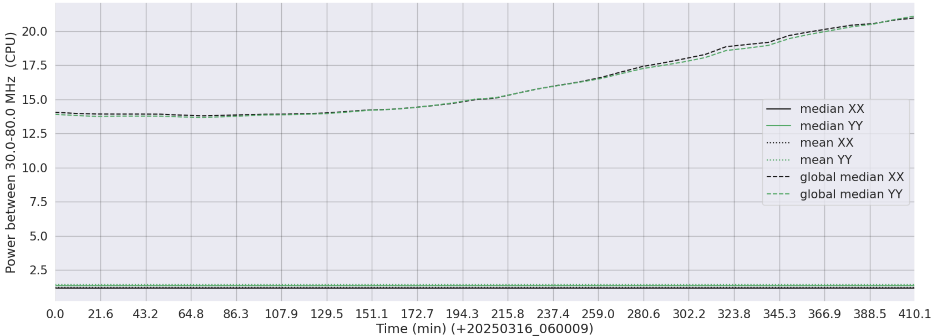
LWA272 - Correlator# 038 - XX FLAGS:LowPower - YY FLAGS:LowPower
