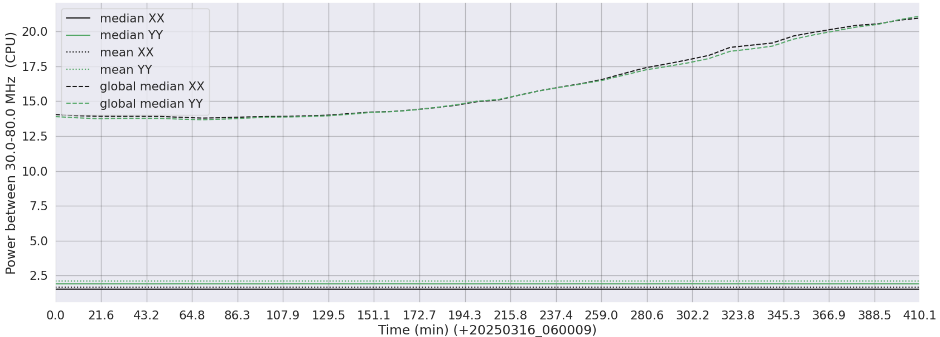
LWA291 - Correlator# 045 - XX FLAGS:LowPower - YY FLAGS:LowPower
