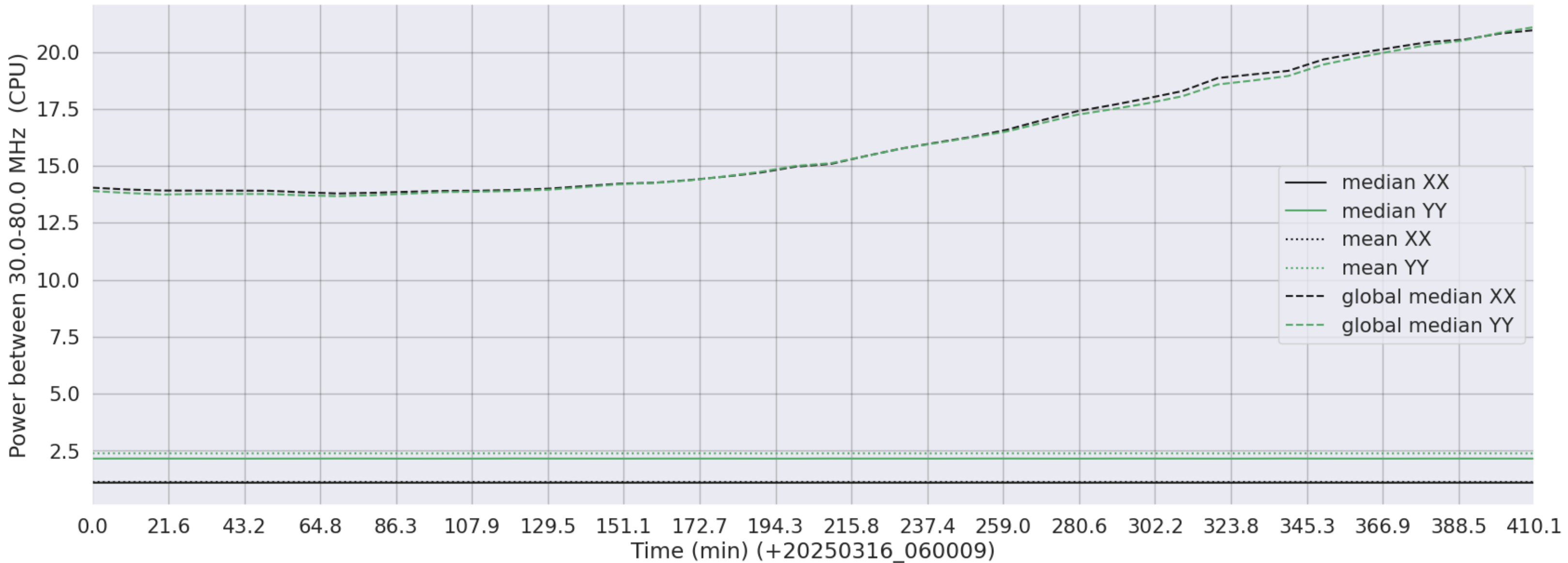
LWA319 - Correlator# 190 - XX FLAGS:LowPower - YY FLAGS:LowPower
