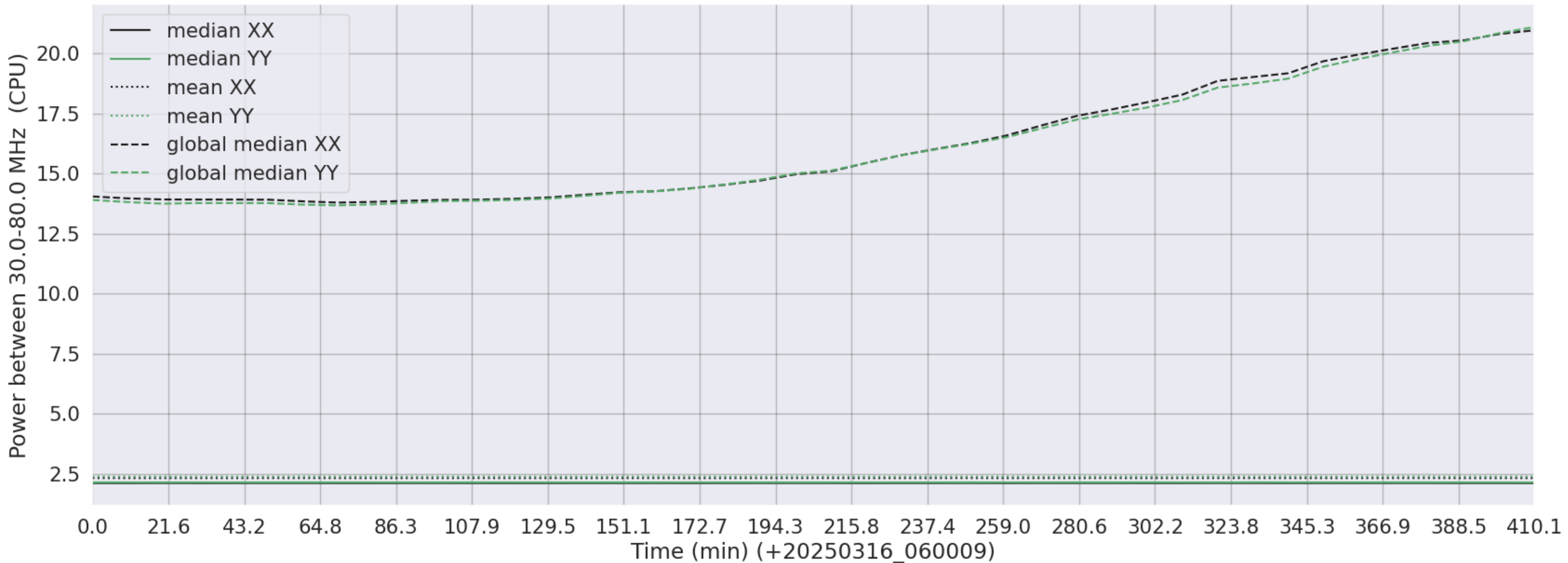
LWA276 - Correlator# 006 - XX FLAGS:LowPower - YY FLAGS:LowPower
