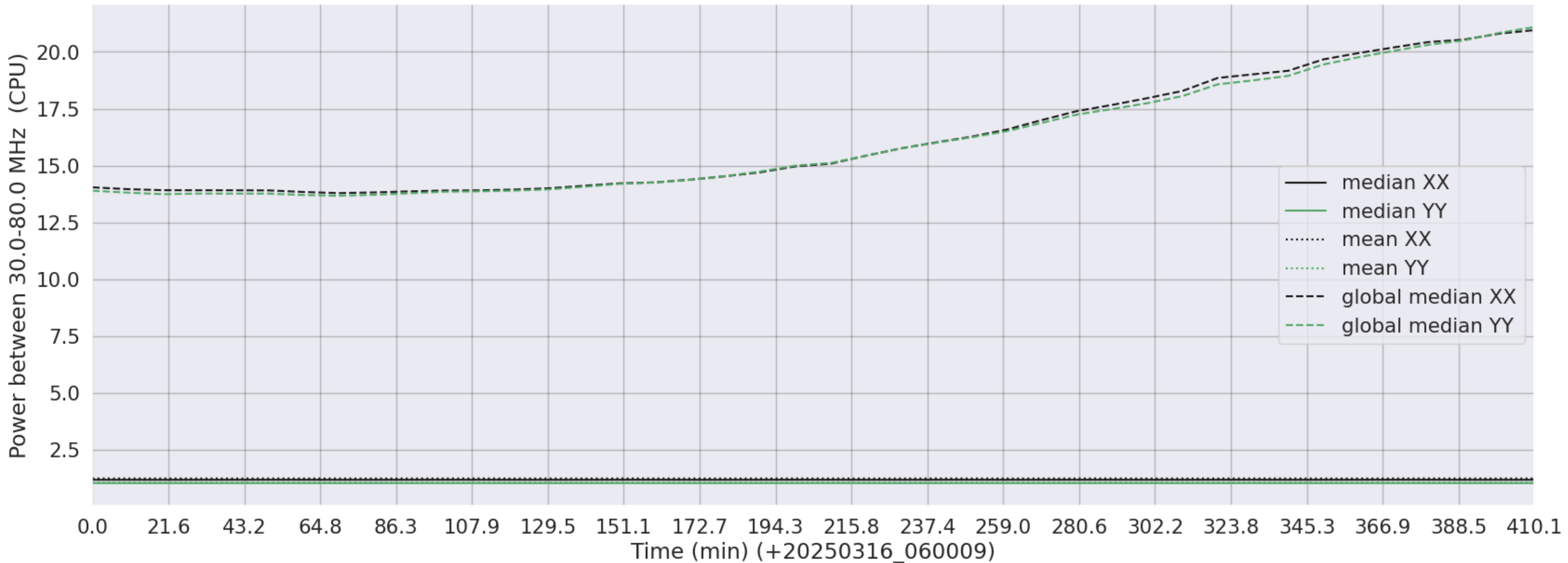
LWA353 - Correlator# 031 - XX FLAGS:LowPower - YY FLAGS:LowPower
