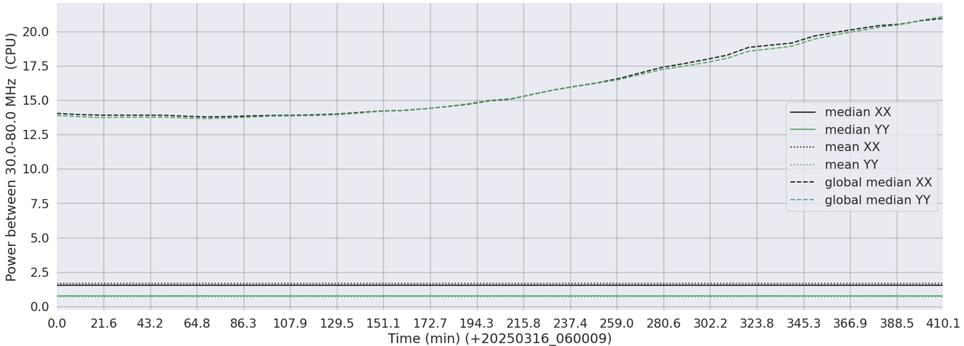
LWA352 - Correlator# 028 - XX FLAGS:LowPower - YY FLAGS:LowPower
