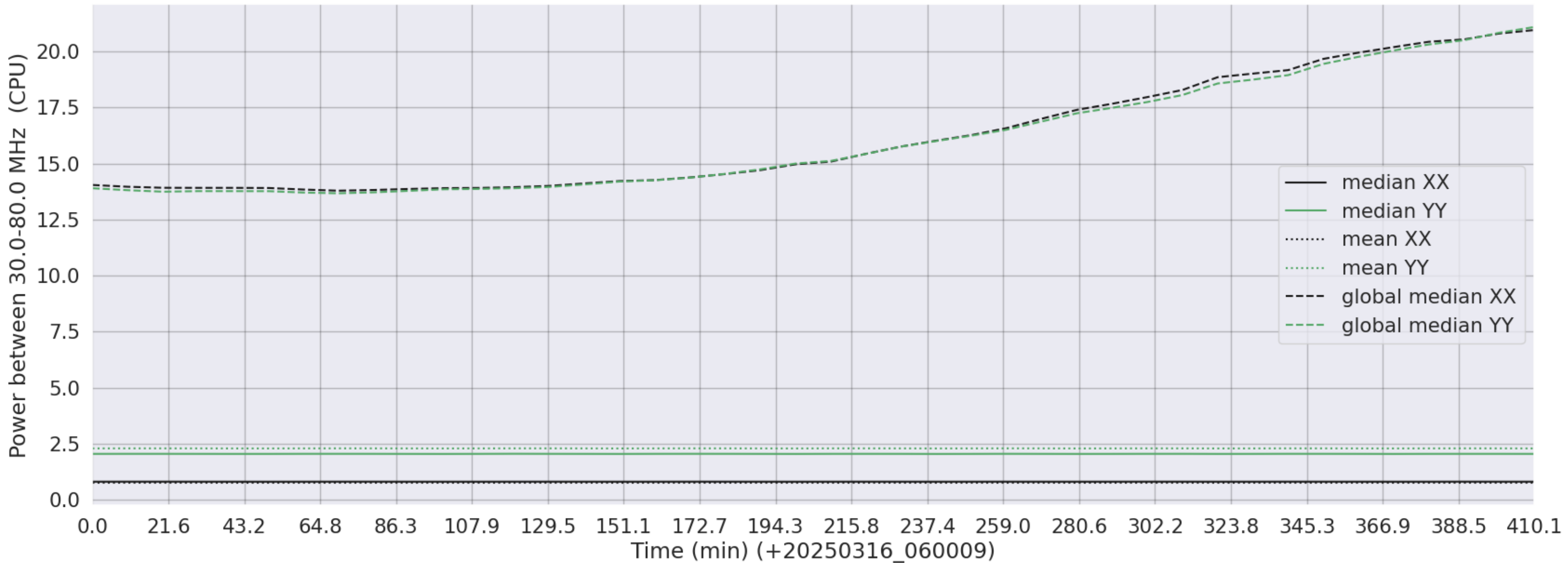
LWA348 - Correlator# 124 - XX FLAGS:LowPower - YY FLAGS:LowPower
