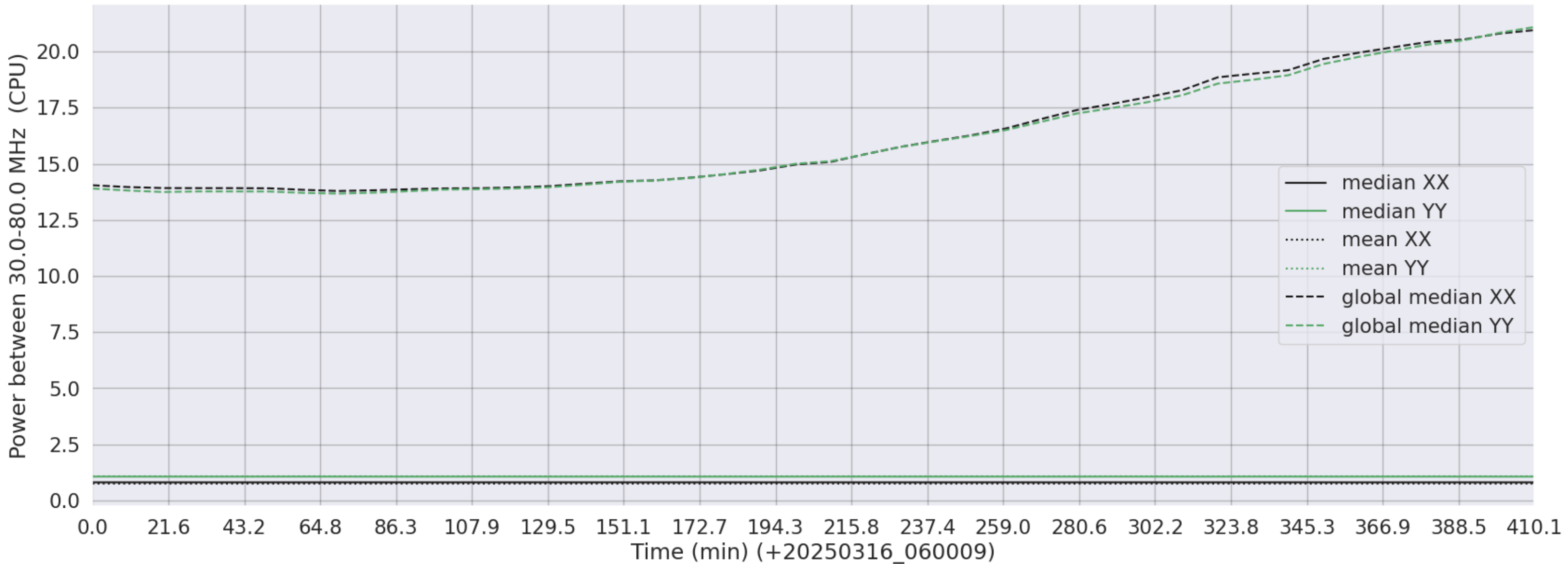
LWA314 - Correlator# 021 - XX FLAGS:LowPower - YY FLAGS:LowPower
