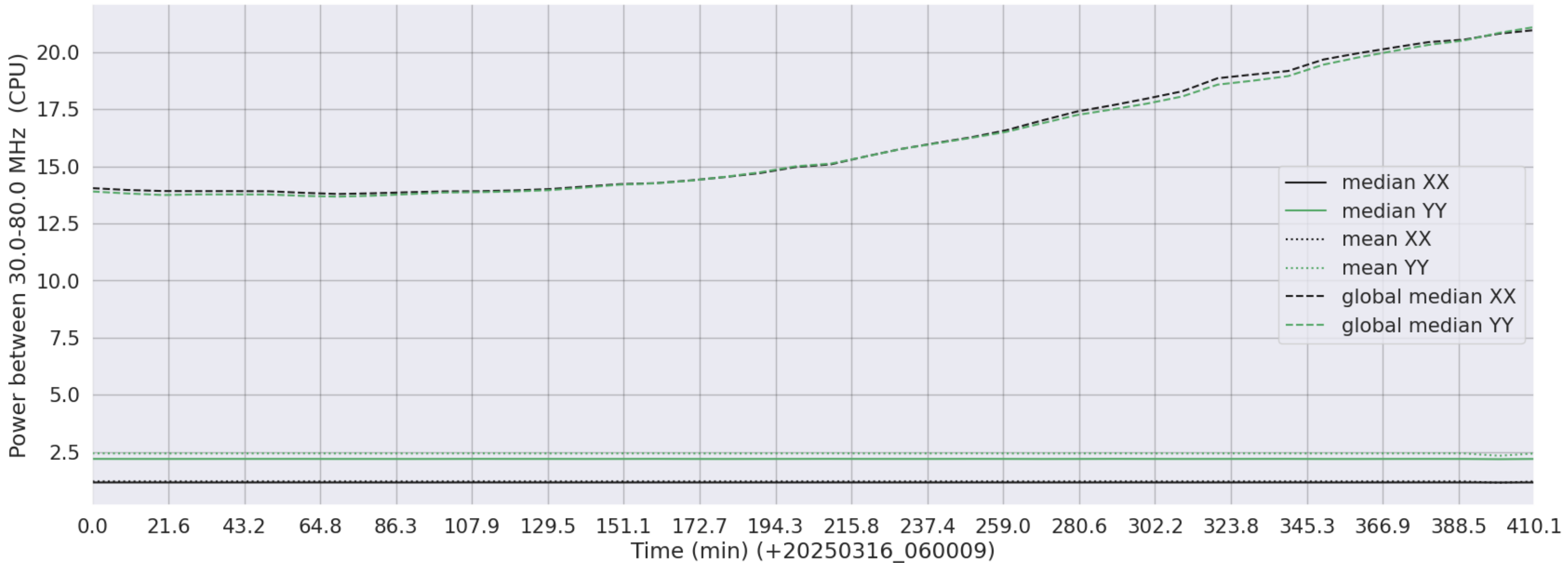
LWA271 - Correlator# 004 - XX FLAGS:LowPower - YY FLAGS:LowPower
