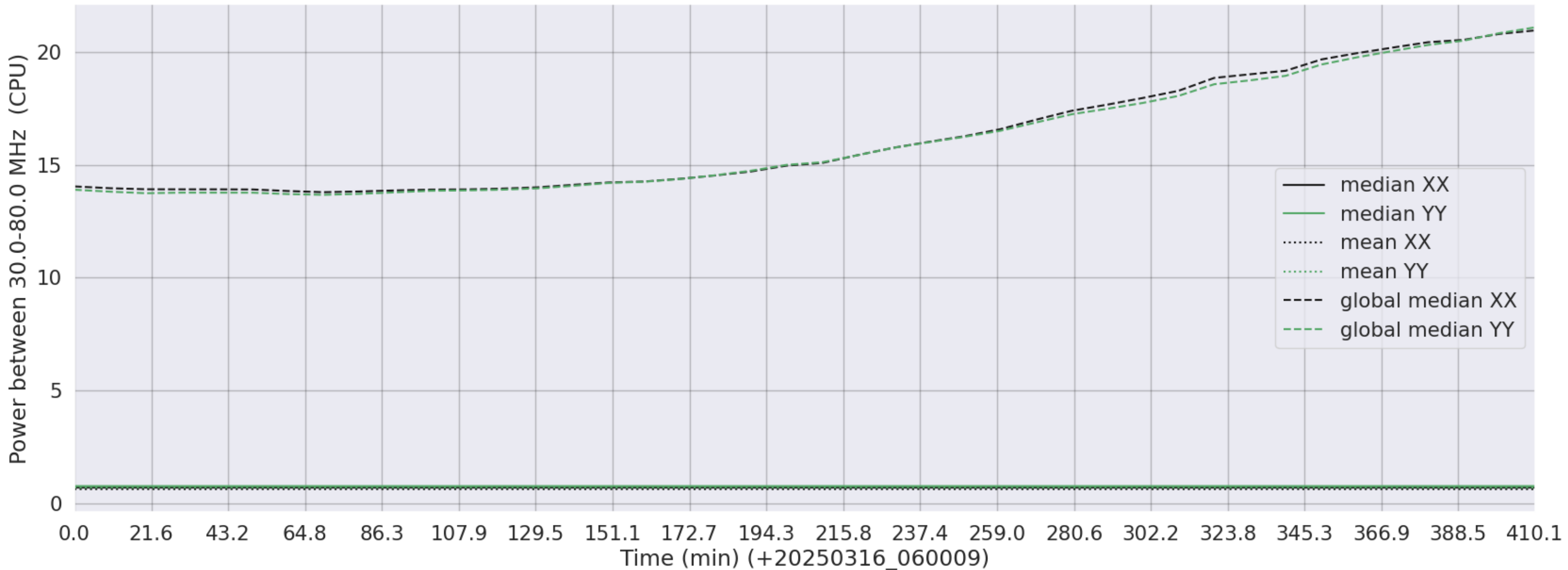
LWA281 - Correlator# 011 - XX FLAGS:LowPower - YY FLAGS:LowPower
