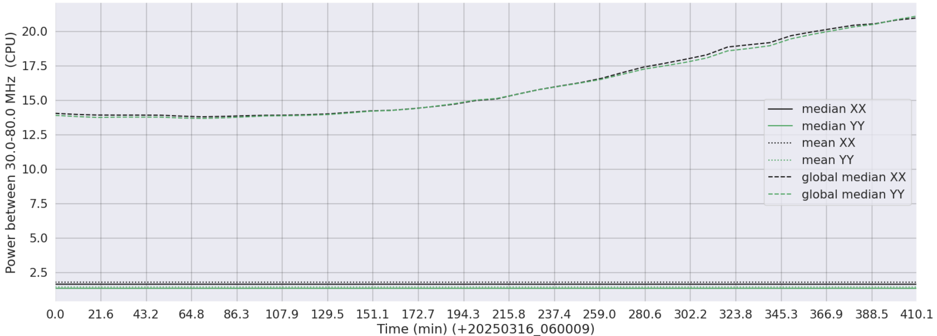
LWA340 - Correlator# 026 - XX FLAGS:LowPower - YY FLAGS:LowPower
