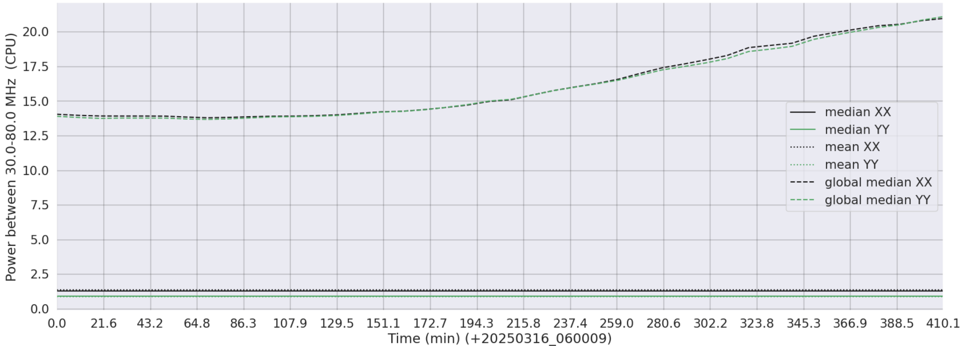
LWA273 - Correlator# 007 - XX FLAGS:LowPower - YY FLAGS:LowPower
