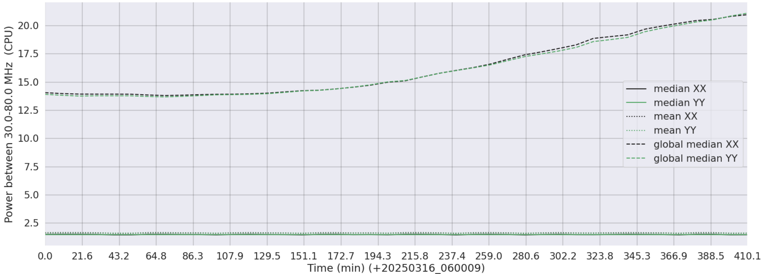
LWA334 - Correlator# 156 - XX FLAGS:LowPower - YY FLAGS:LowPower
