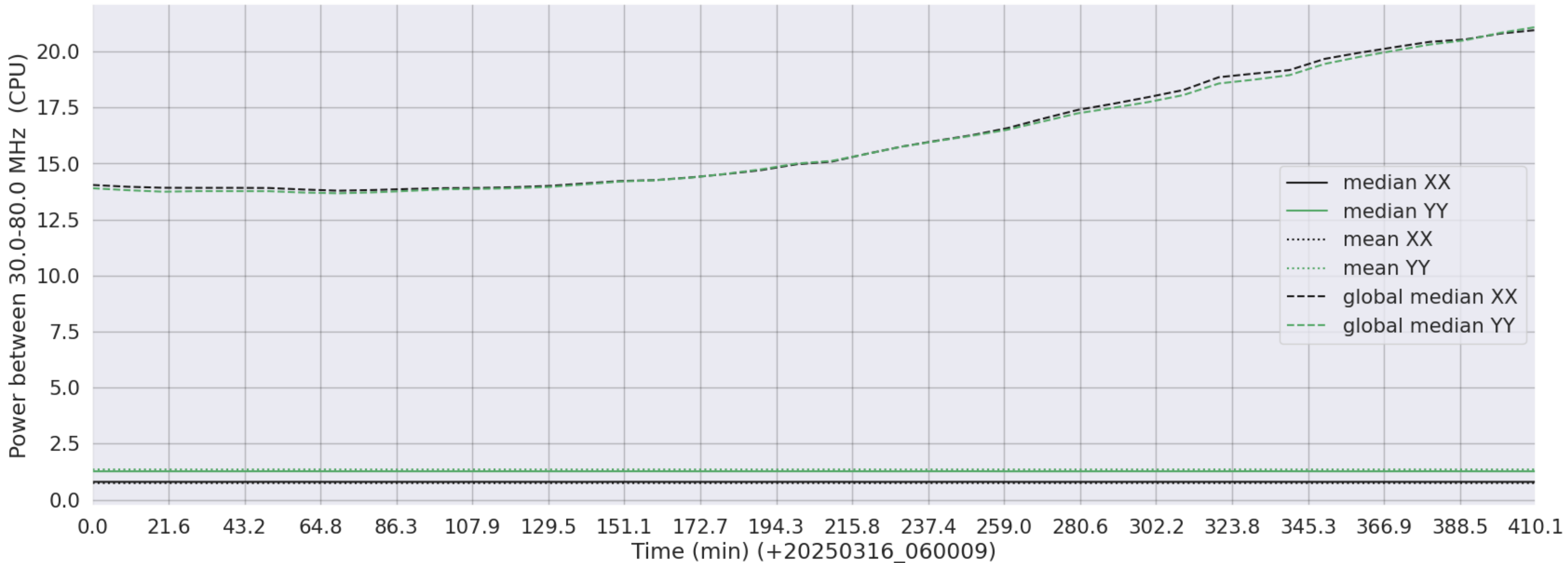
LWA261 - Correlator# 346 - XX FLAGS:LowPower - YY FLAGS:LowPower
