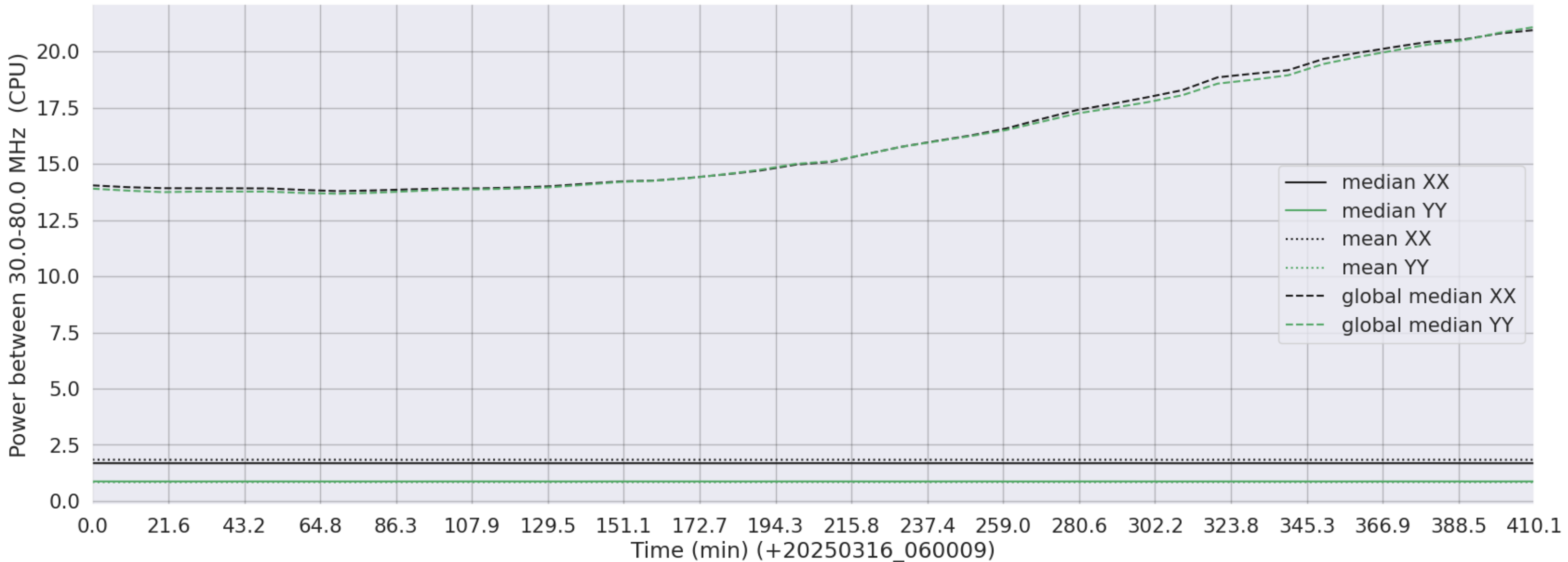
LWA285 - Correlator# 013 - XX FLAGS:LowPower - YY FLAGS:LowPower
