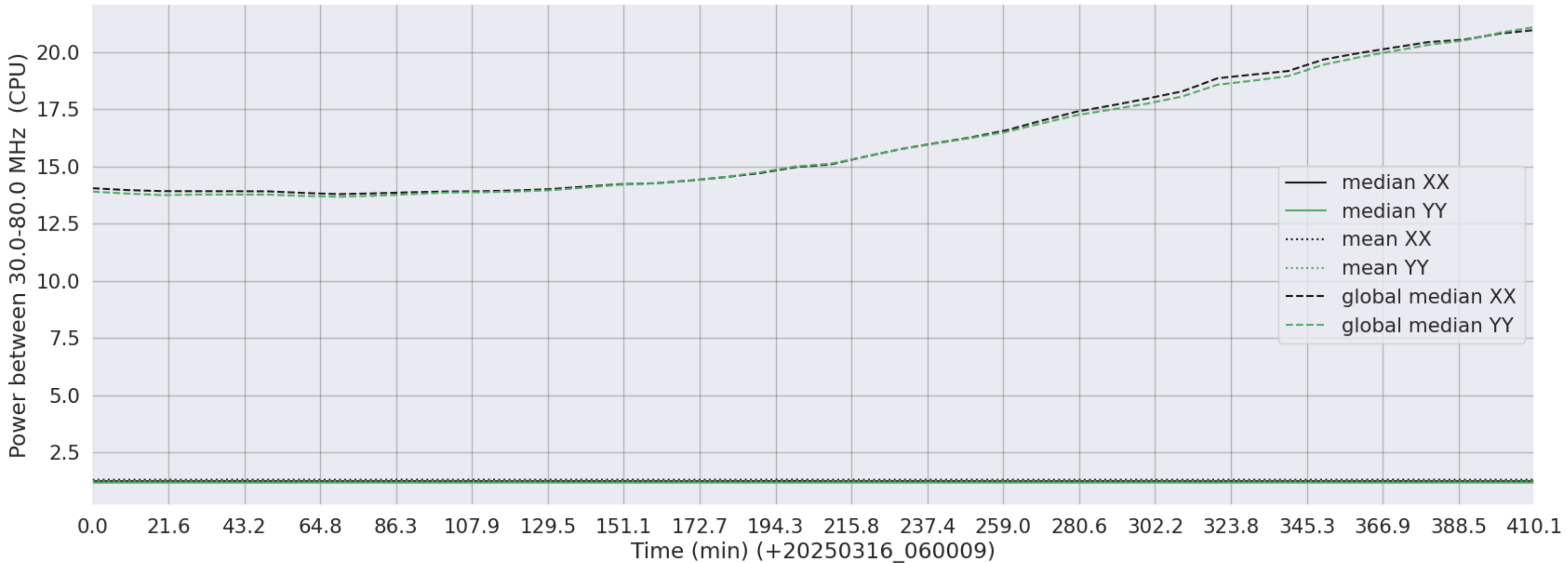
LWA336 - Correlator# 056 - XX FLAGS:LowPower - YY FLAGS:LowPower
