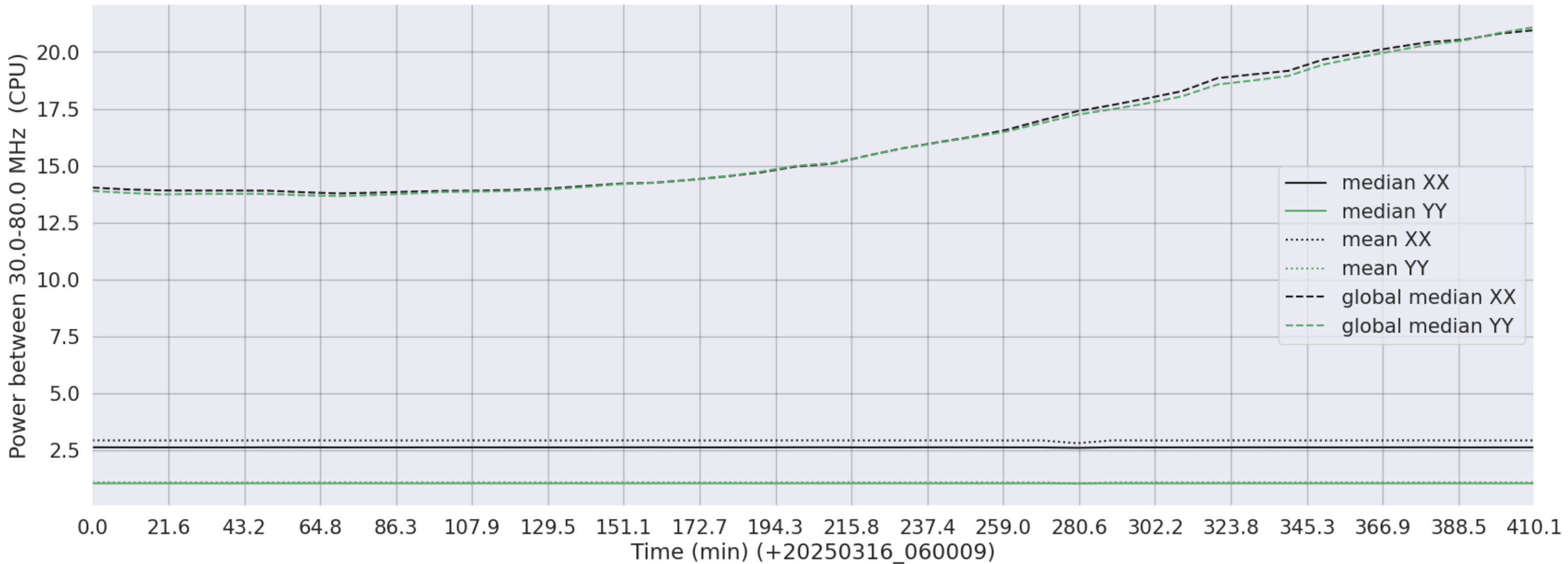
LWA316 - Correlator# 155 - XX FLAGS:LowPower - YY FLAGS:LowPower
