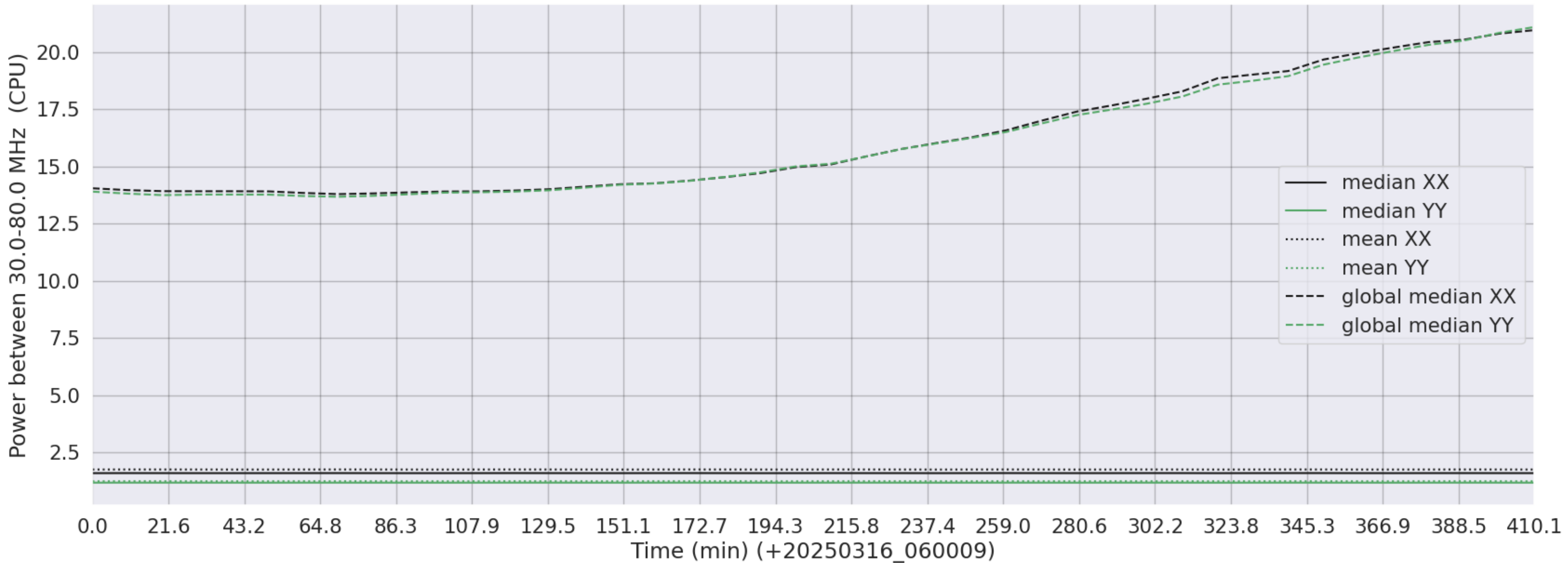
LWA310 - Correlator# 017 - XX FLAGS:LowPower - YY FLAGS:LowPower
