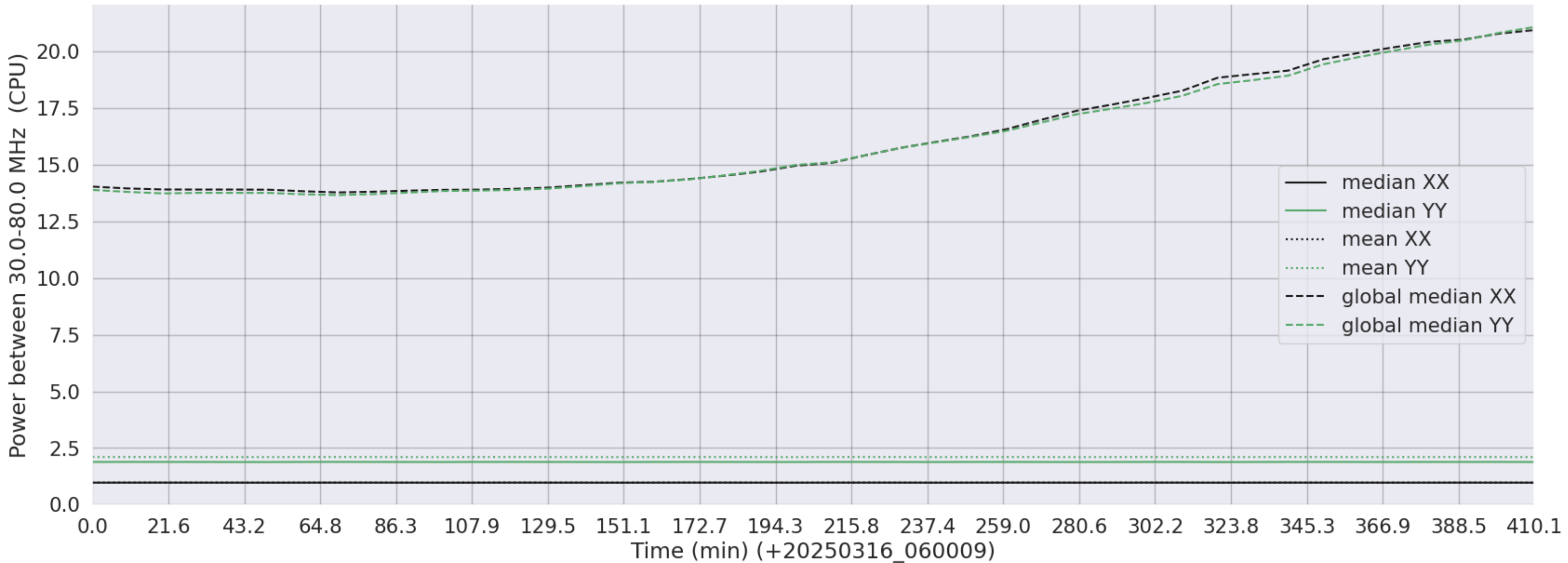
LWA332 - Correlator# 025 - XX FLAGS:LowPower - YY FLAGS:LowPower
