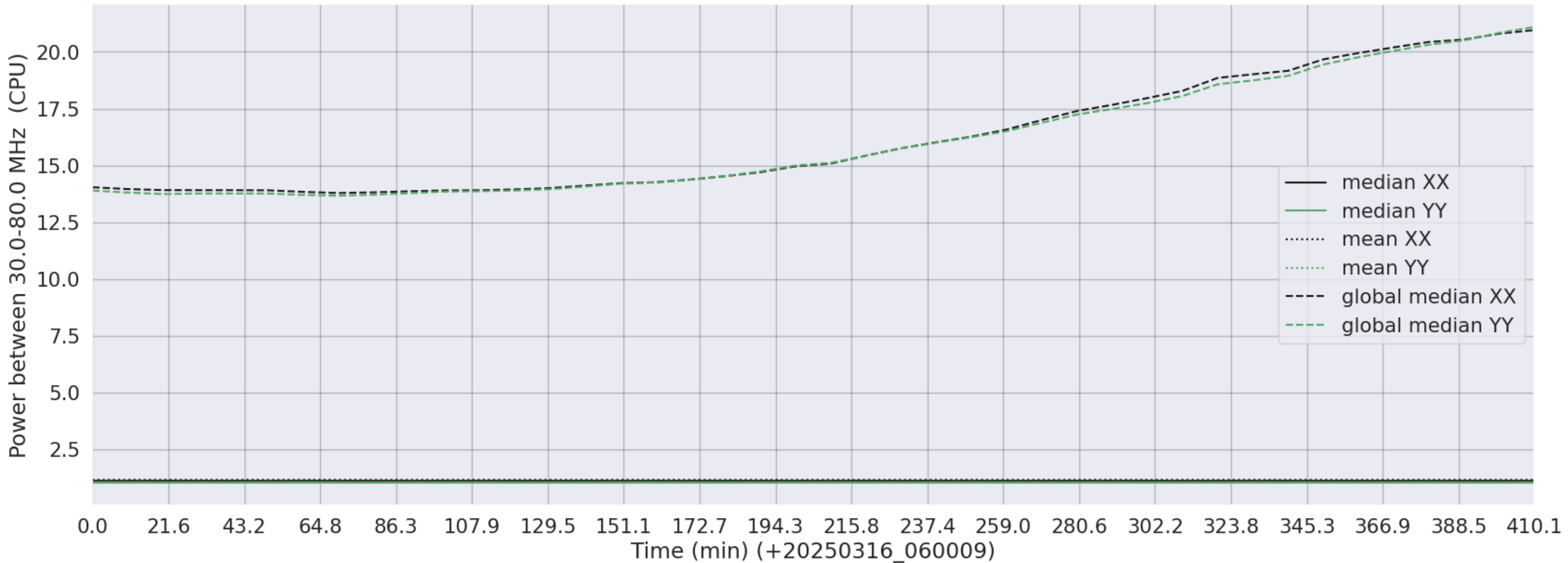
LWA341 - Correlator# 029 - XX FLAGS:LowPower - YY FLAGS:LowPower
