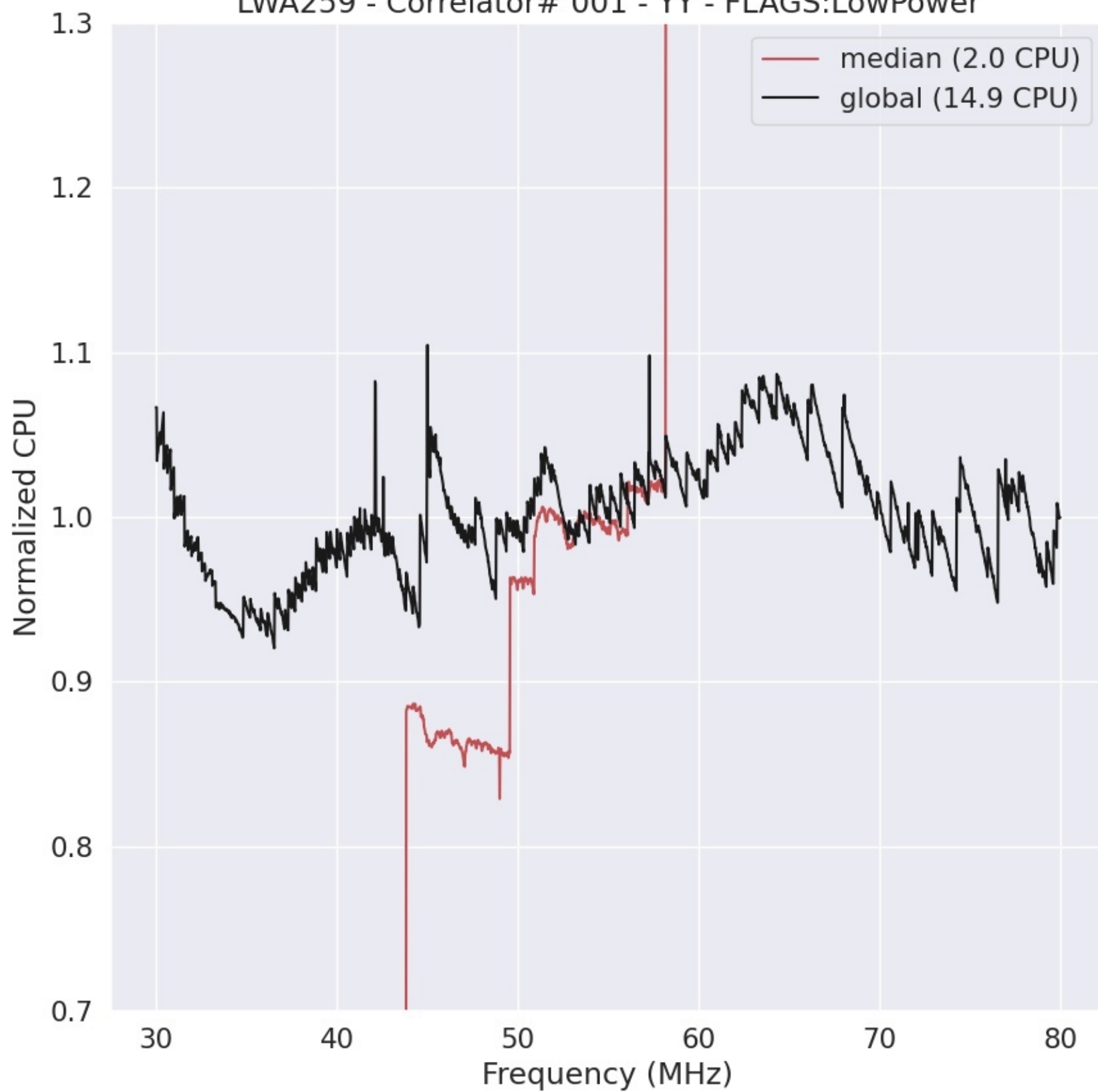
LWA259 - Correlator# 001 - YY - FLAGS:LowPower
