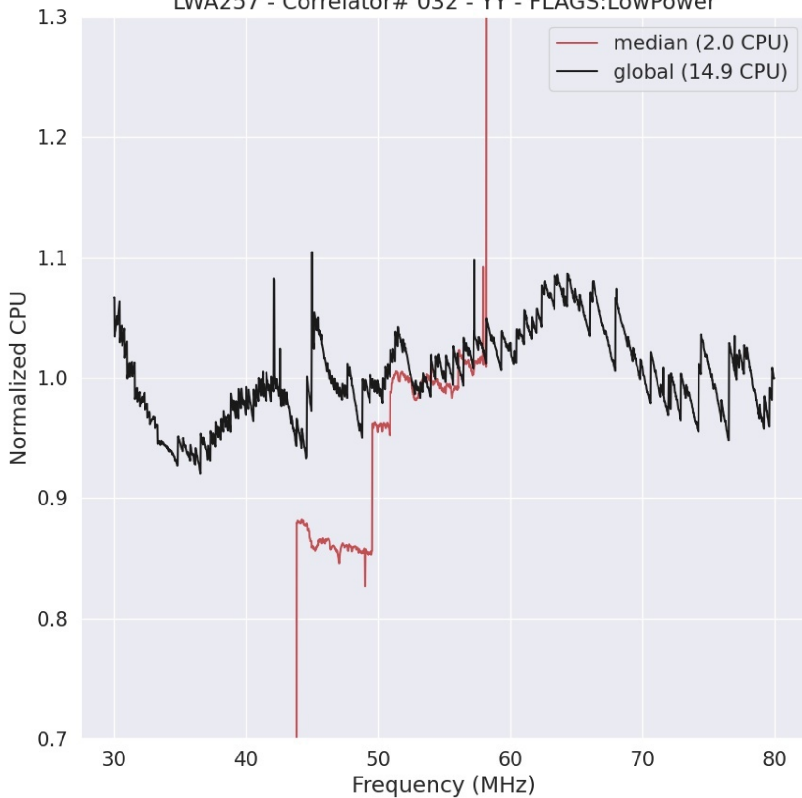
LWA257 - Correlator# 032 - YY - FLAGS:LowPower
