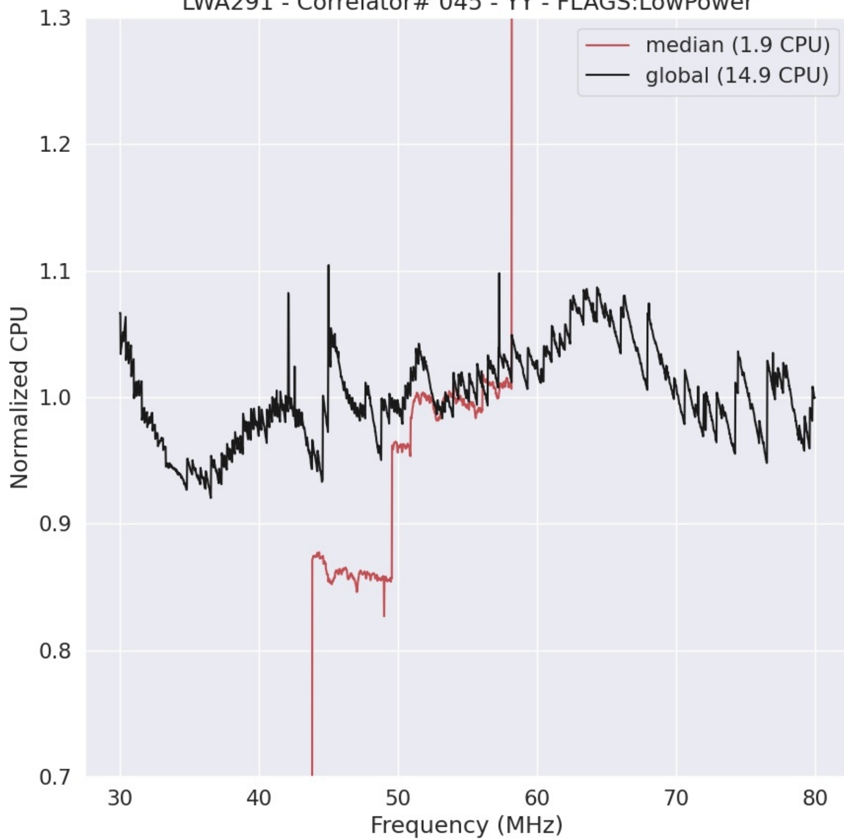
LWA291 - Correlator# 045 - YY - FLAGS:LowPower
