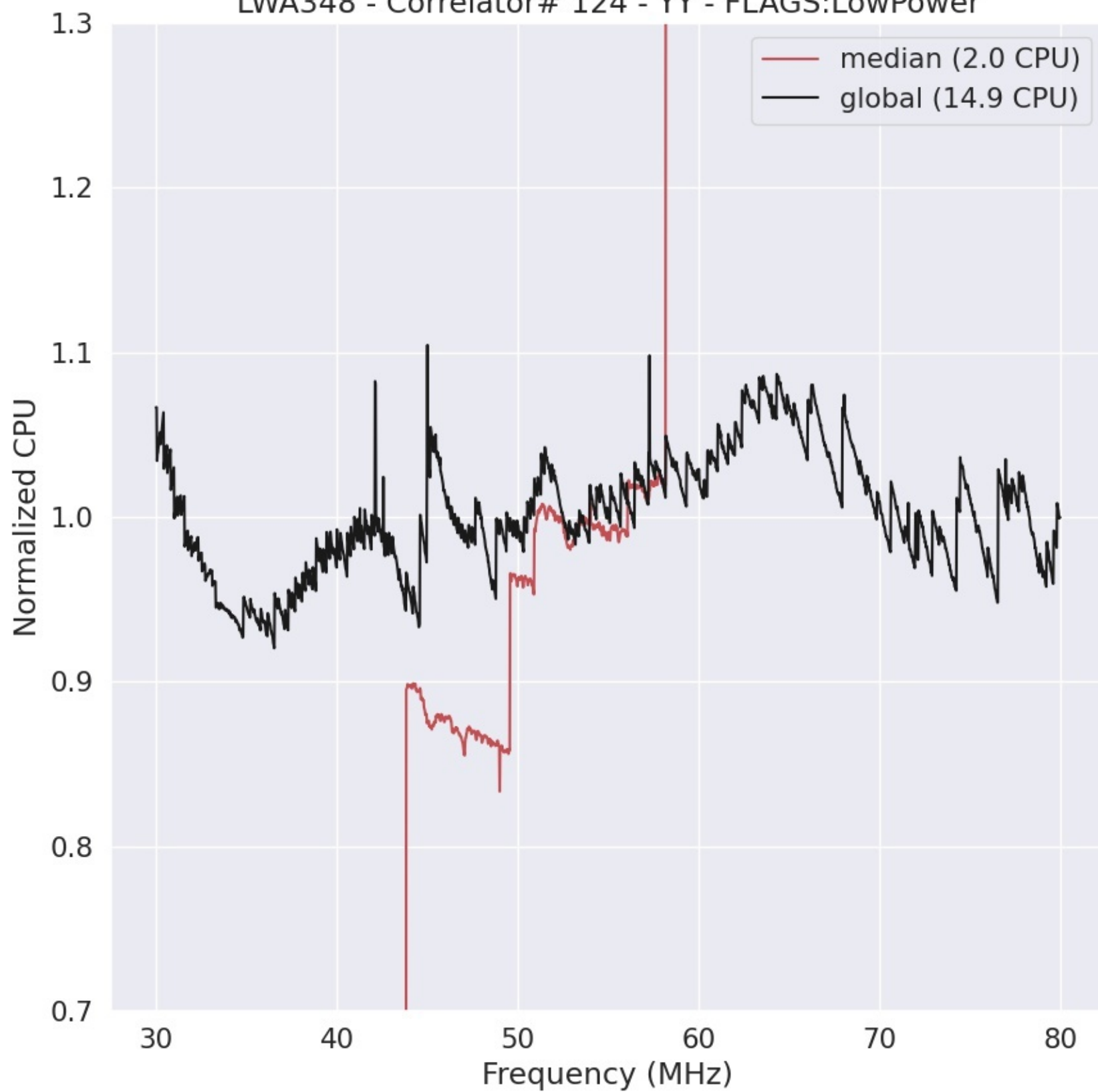
LWA348 - Correlator# 124 - YY - FLAGS:LowPower
