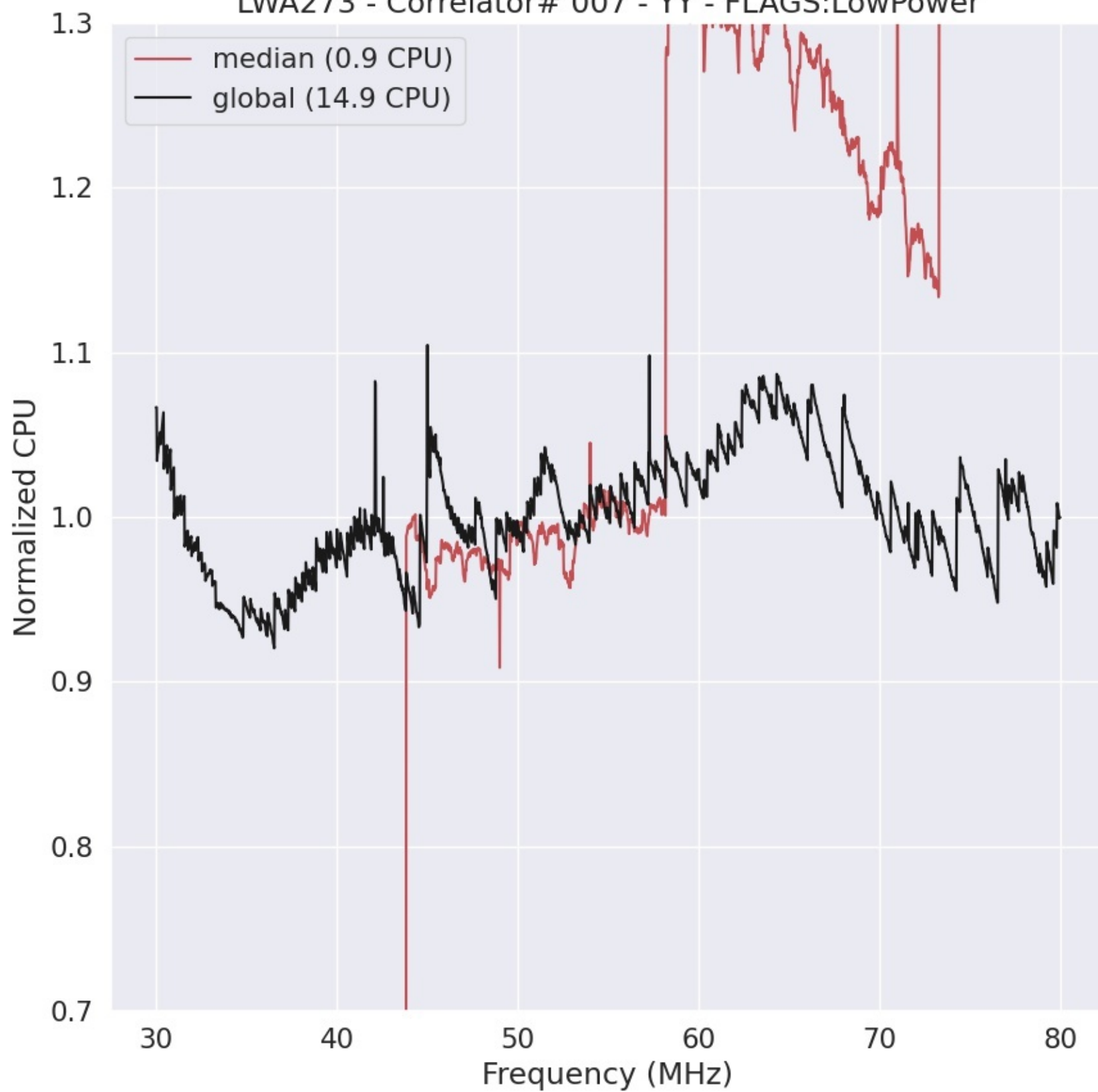
LWA273 - Correlator# 007 - YY - FLAGS:LowPower
