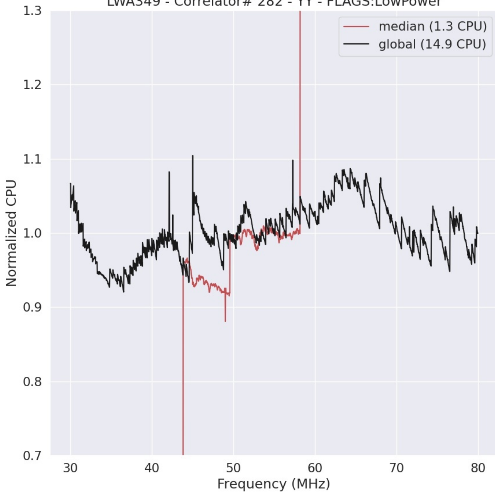
LWA349 - Correlator# 282 - YY - FLAGS:LowPower
