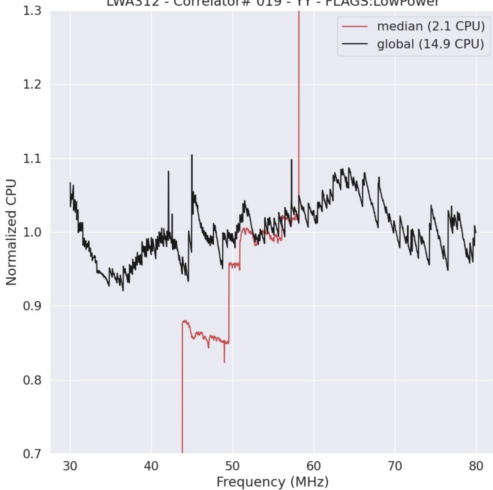
LWA312 - Correlator# 019 - YY - FLAGS:LowPower
