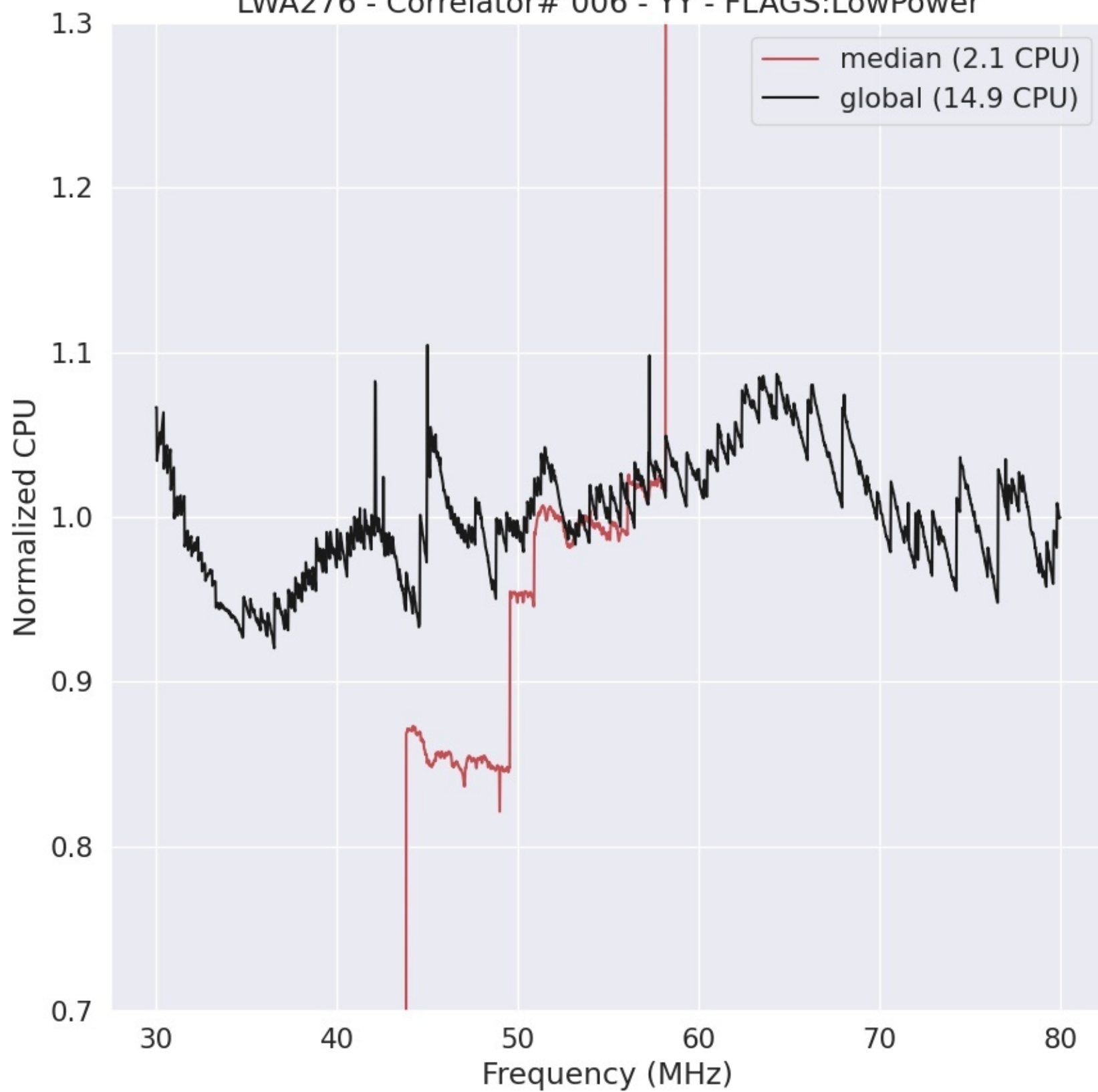
LWA276 - Correlator# 006 - YY - FLAGS:LowPower
