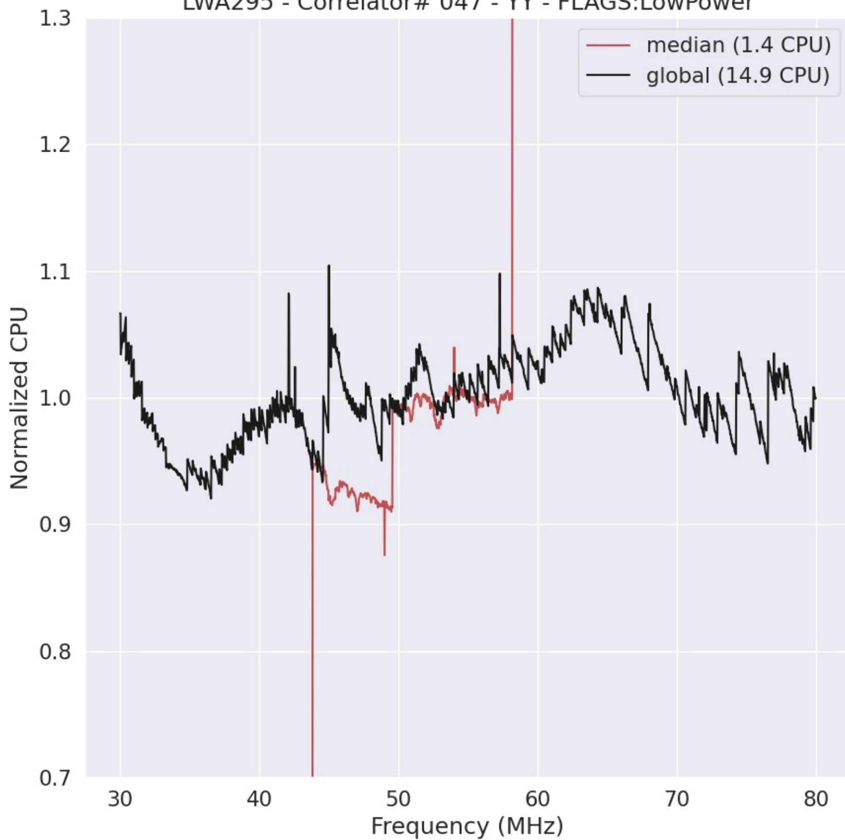
LWA295 - Correlator# 047 - YY - FLAGS:LowPower
