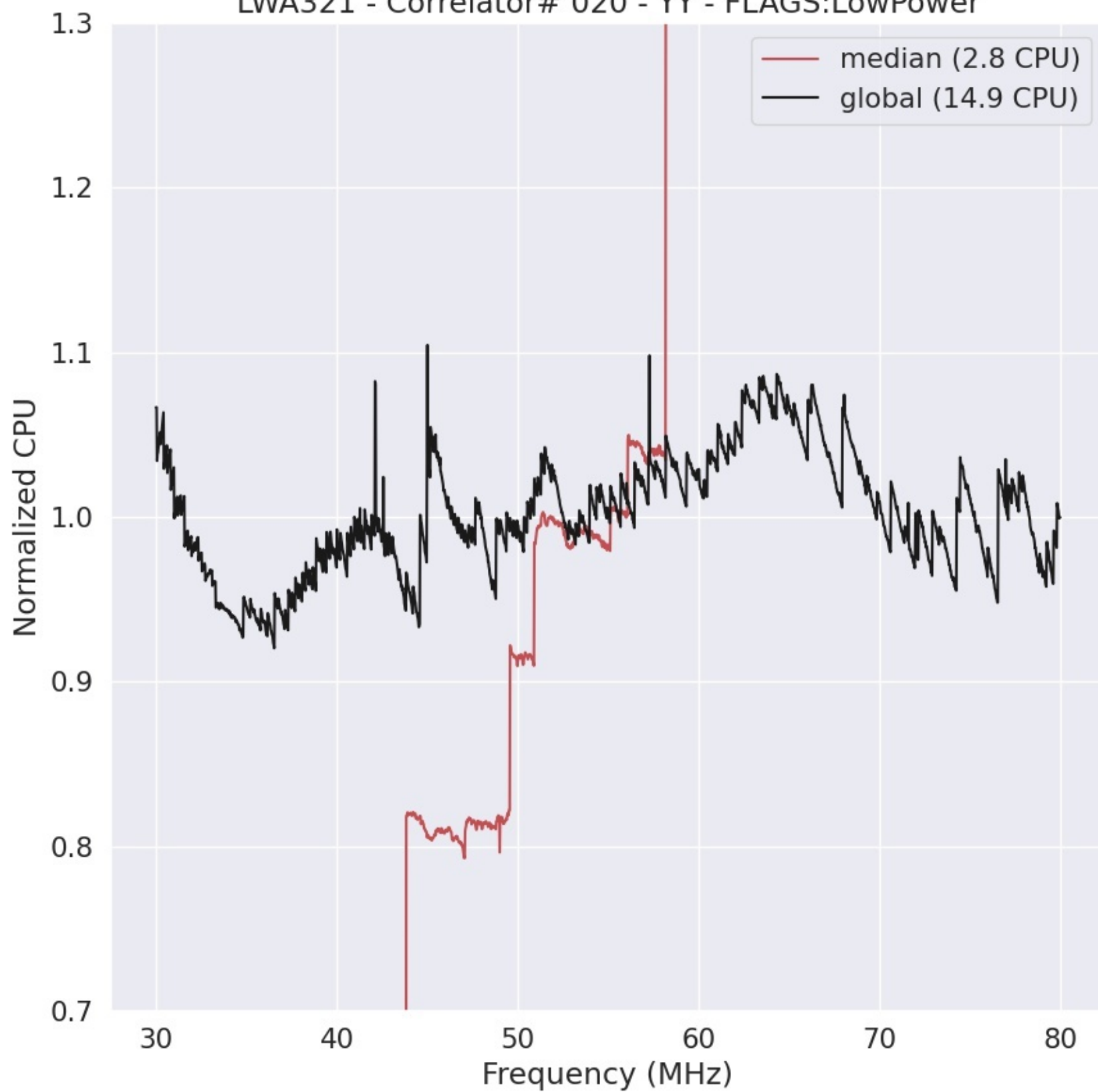
LWA321 - Correlator# 020 - YY - FLAGS:LowPower
