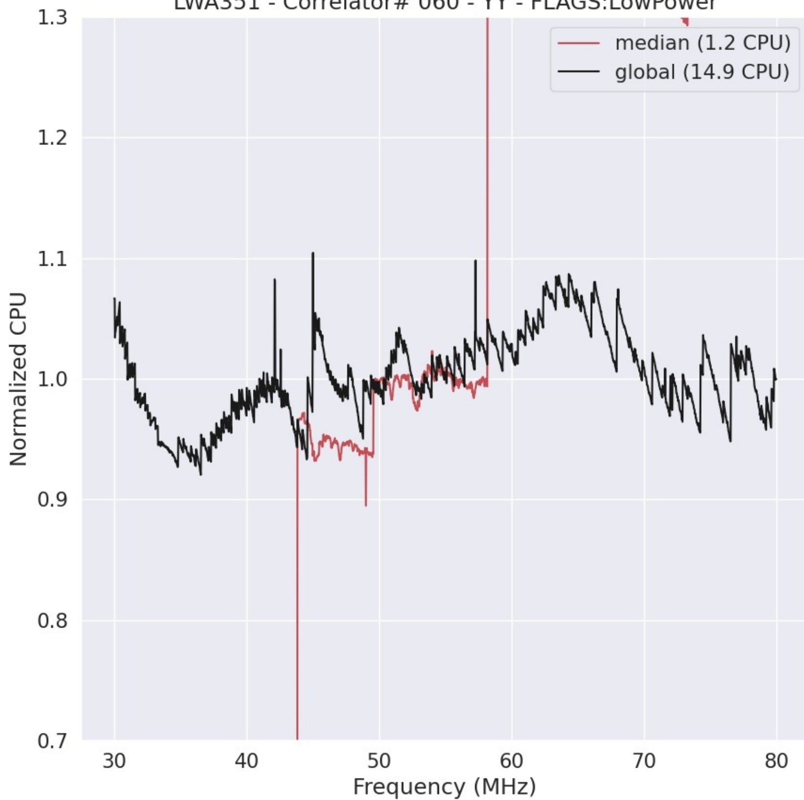
LWA351 - Correlator# 060 - YY - FLAGS:LowPower
