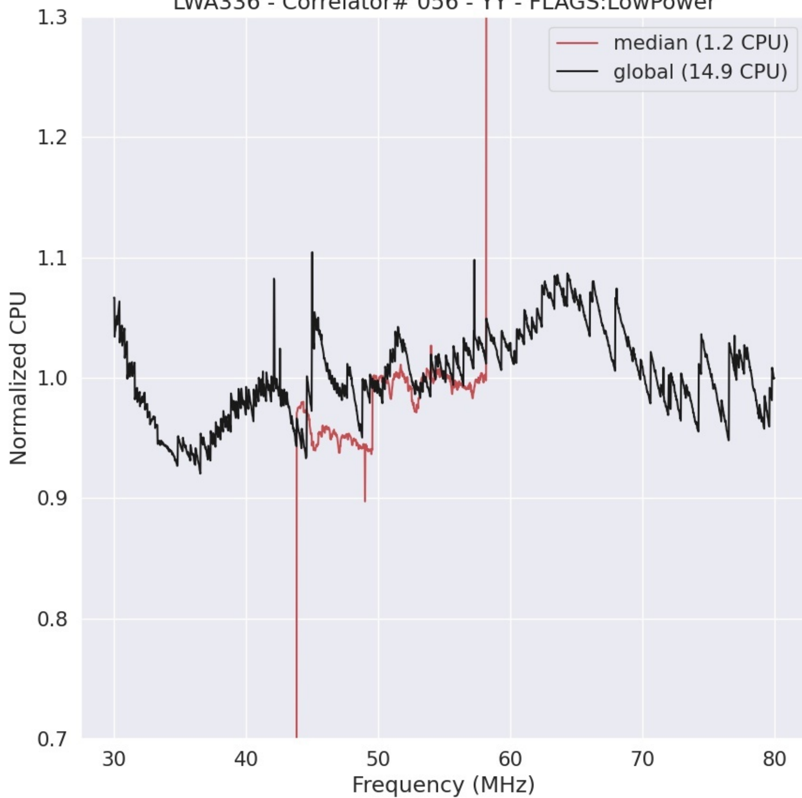
LWA336 - Correlator# 056 - YY - FLAGS:LowPower
