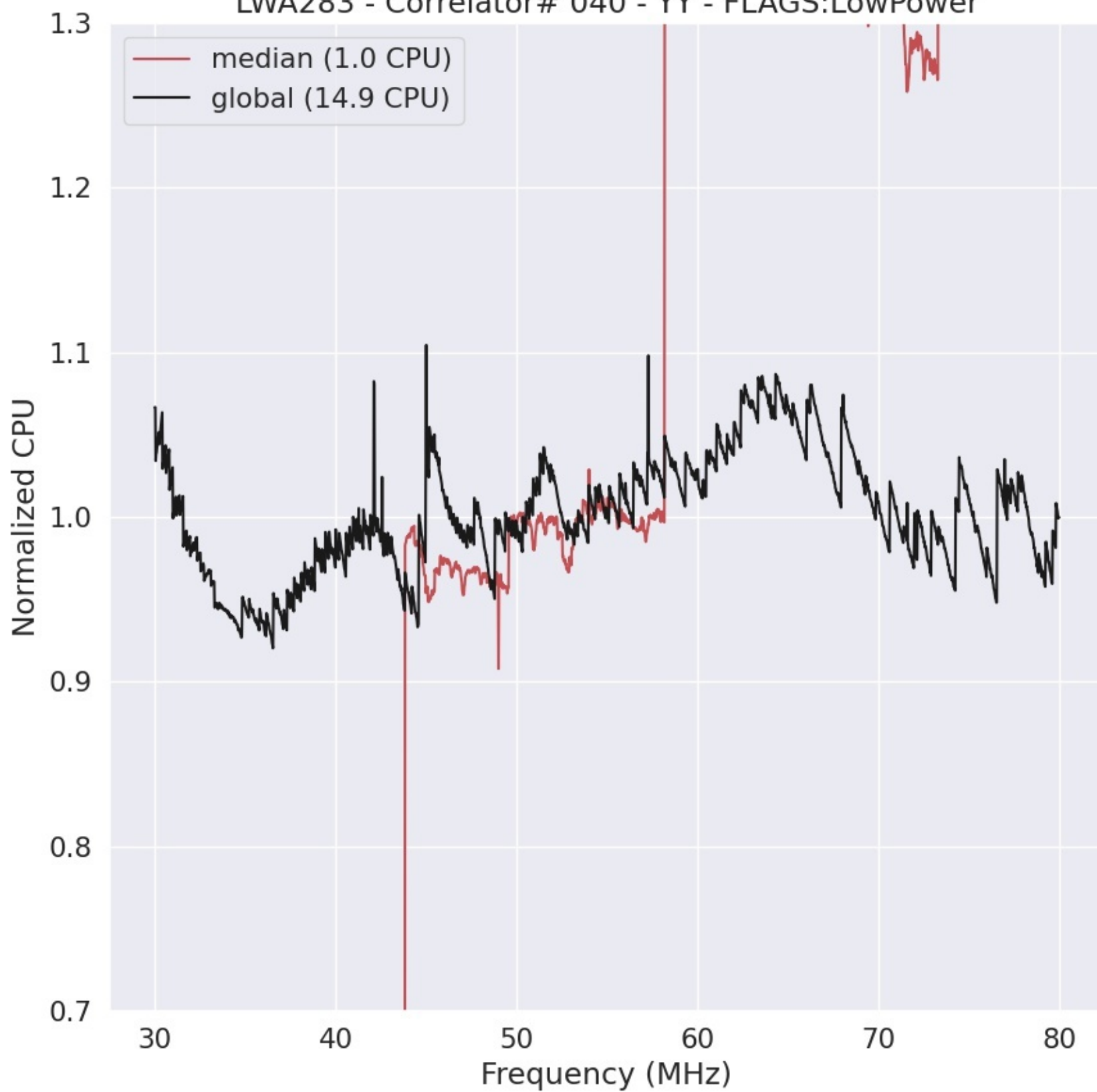
LWA283 - Correlator# 040 - YY - FLAGS:LowPower
