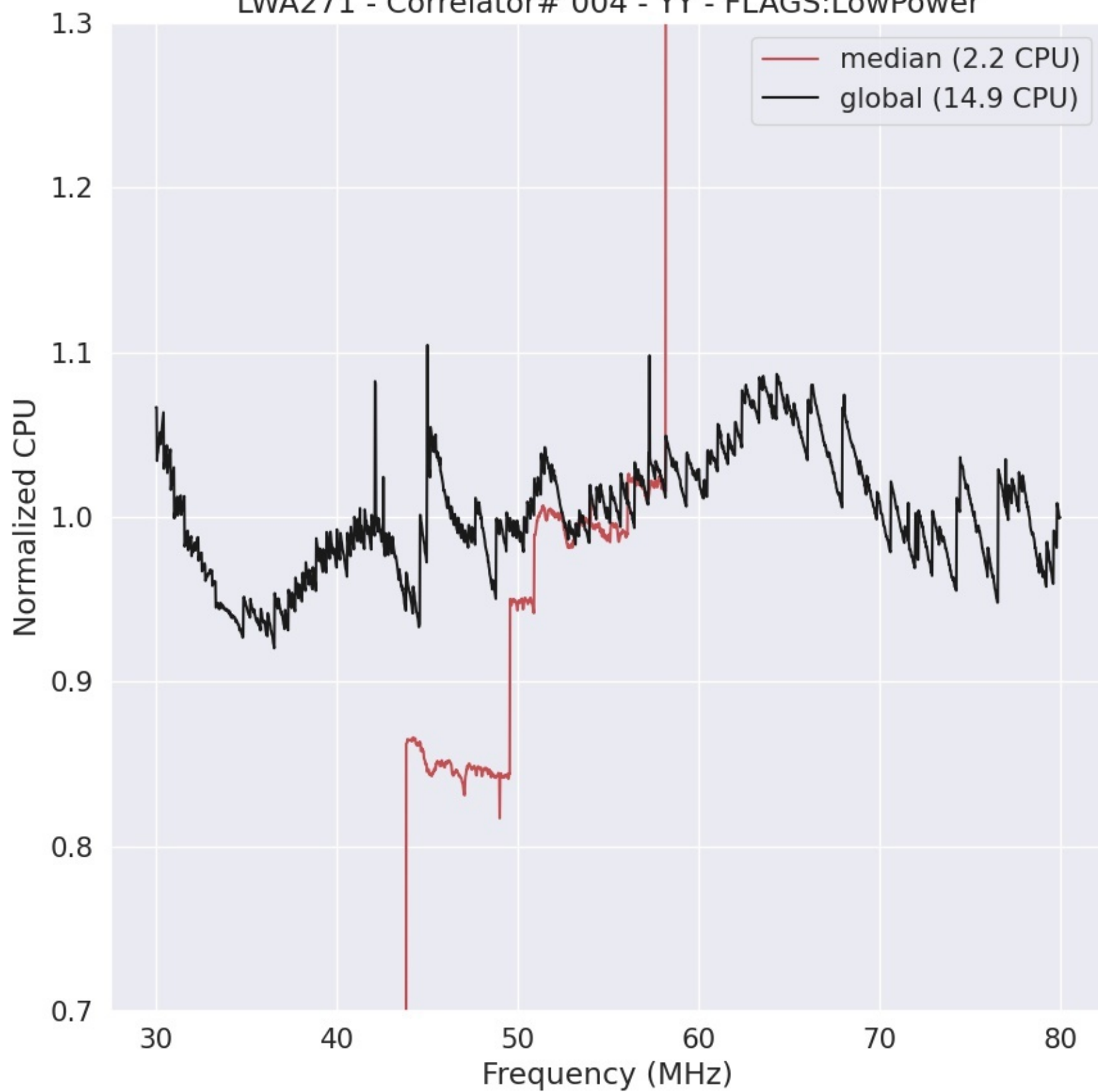
LWA271 - Correlator# 004 - YY - FLAGS:LowPower
