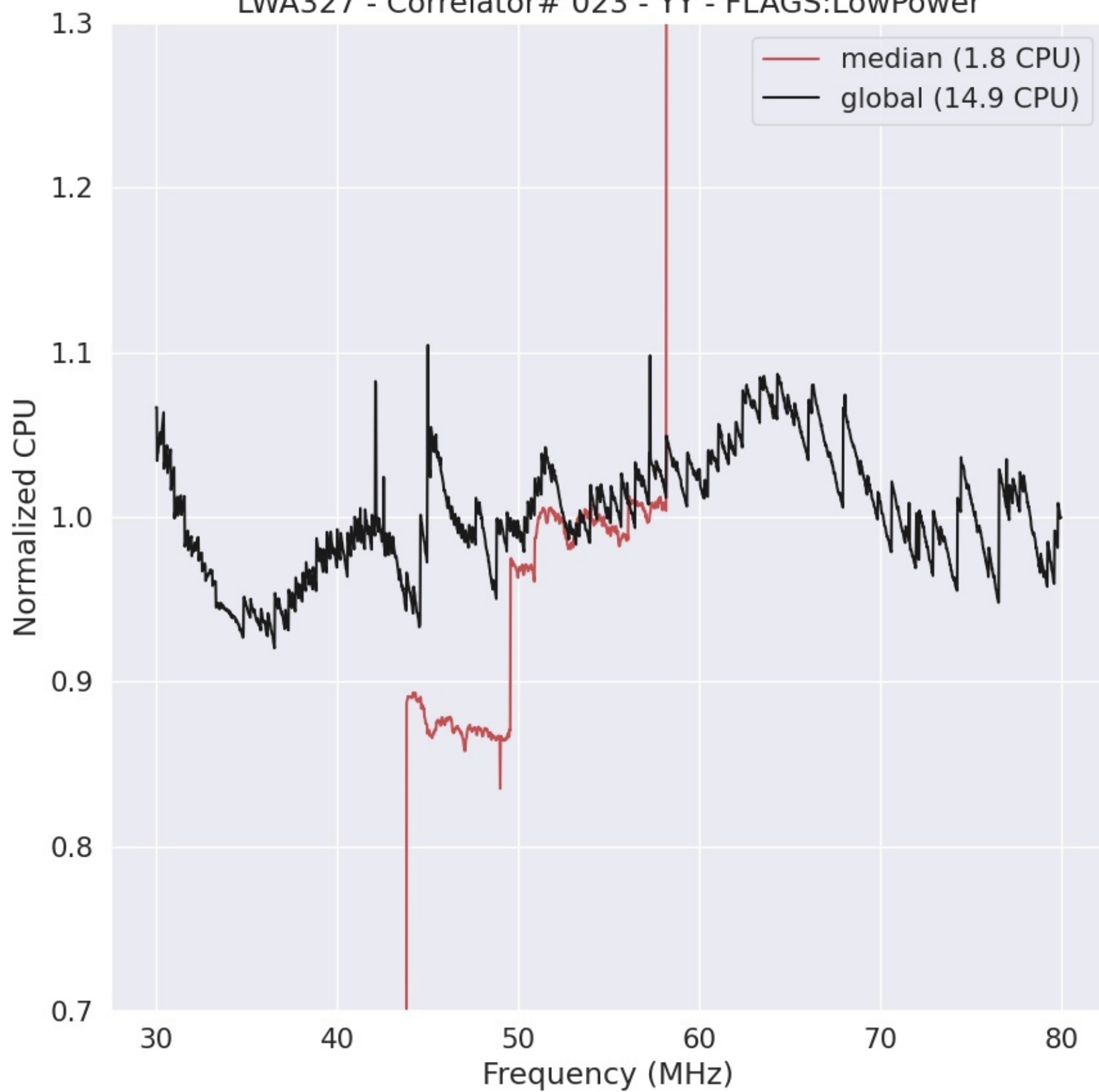
LWA327 - Correlator# 023 - YY - FLAGS:LowPower
