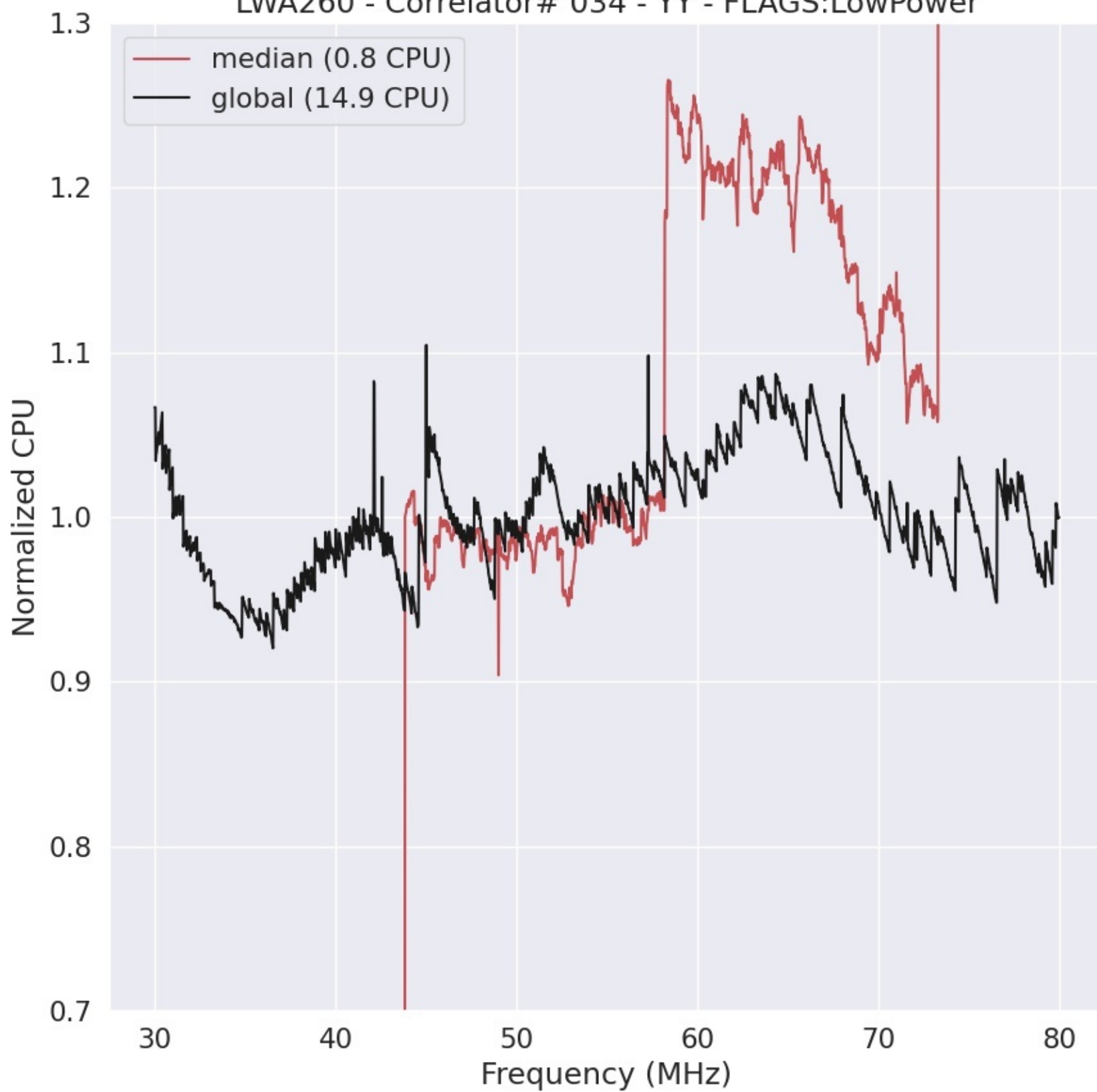
LWA260 - Correlator# 034 - YY - FLAGS:LowPower
