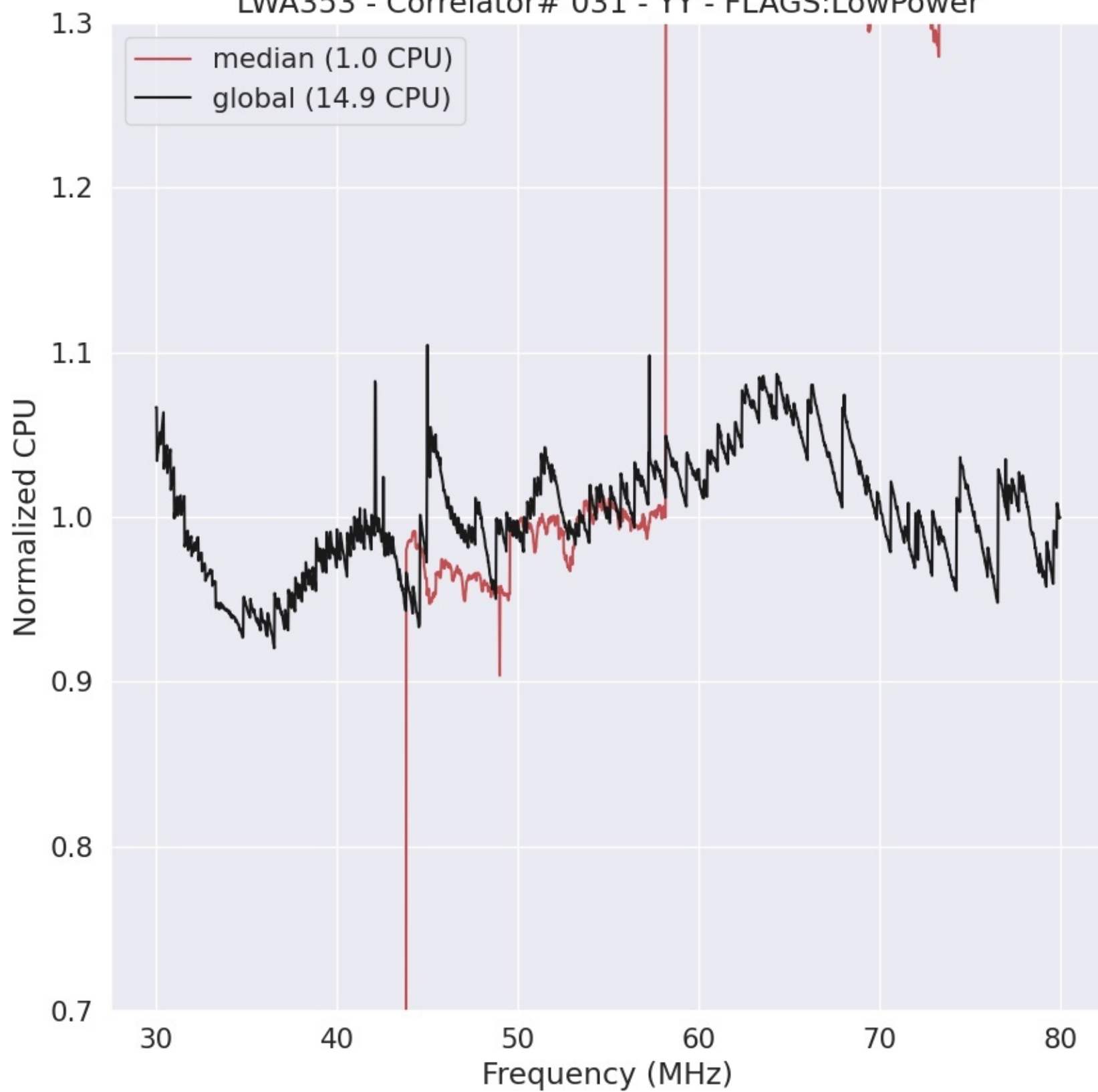
LWA353 - Correlator# 031 - YY - FLAGS:LowPower
