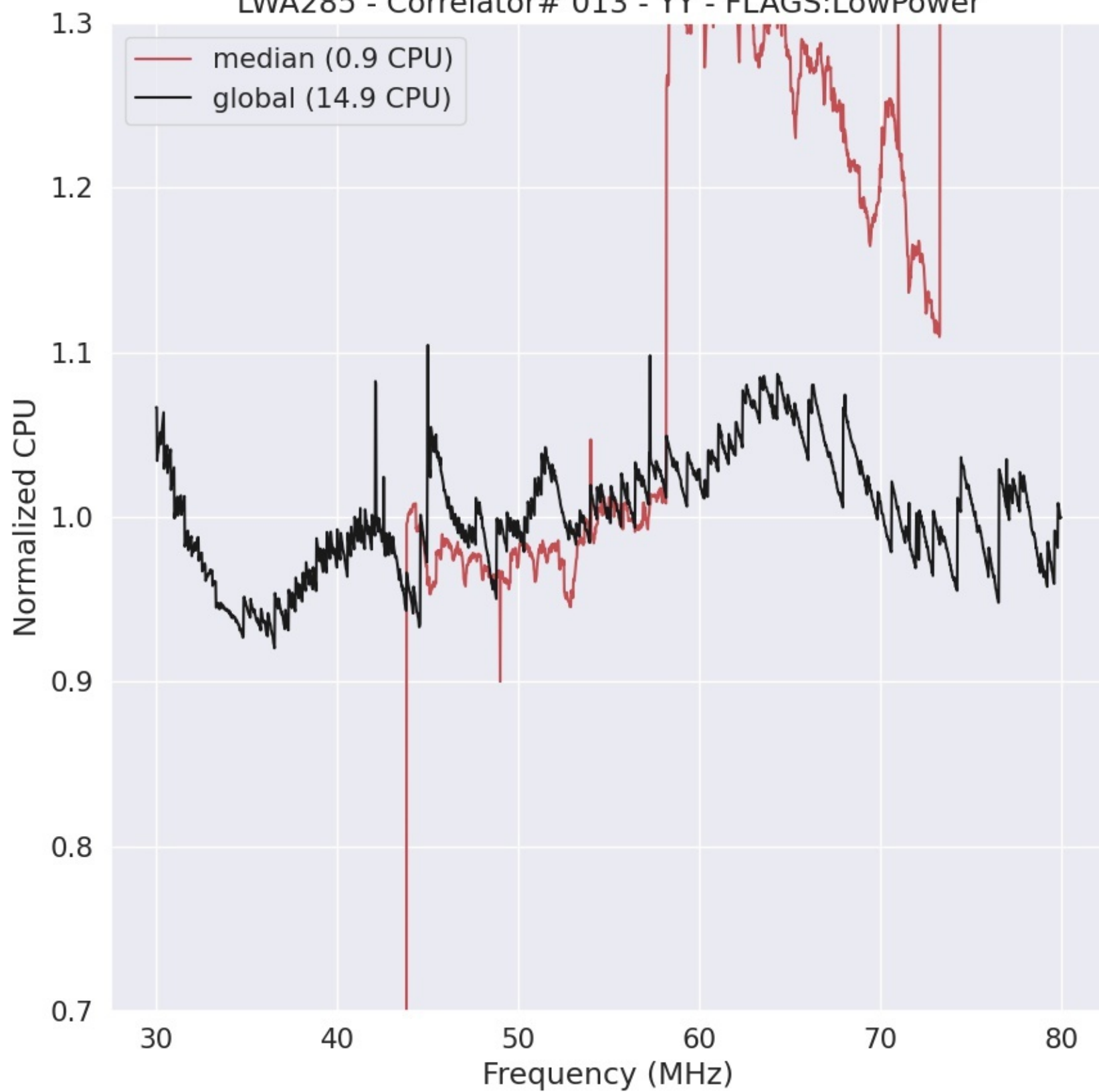
LWA285 - Correlator# 013 - YY - FLAGS:LowPower
