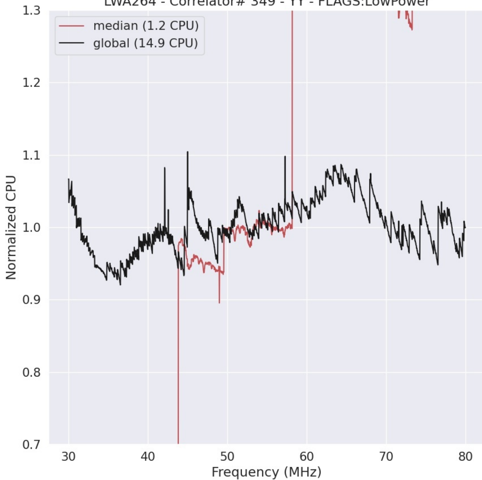
LWA264 - Correlator# 349 - YY - FLAGS:LowPower
