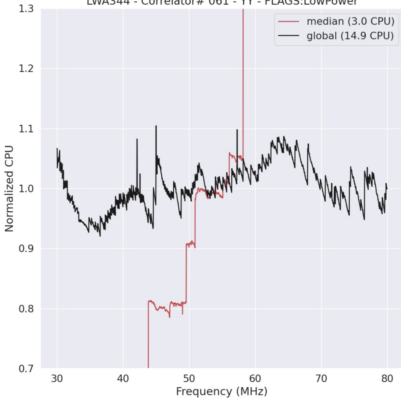
LWA344 - Correlator# 061 - YY - FLAGS:LowPower
