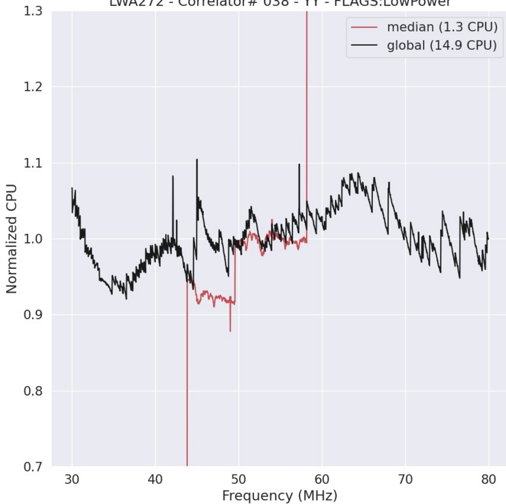
LWA272 - Correlator# 038 - YY - FLAGS:LowPower
