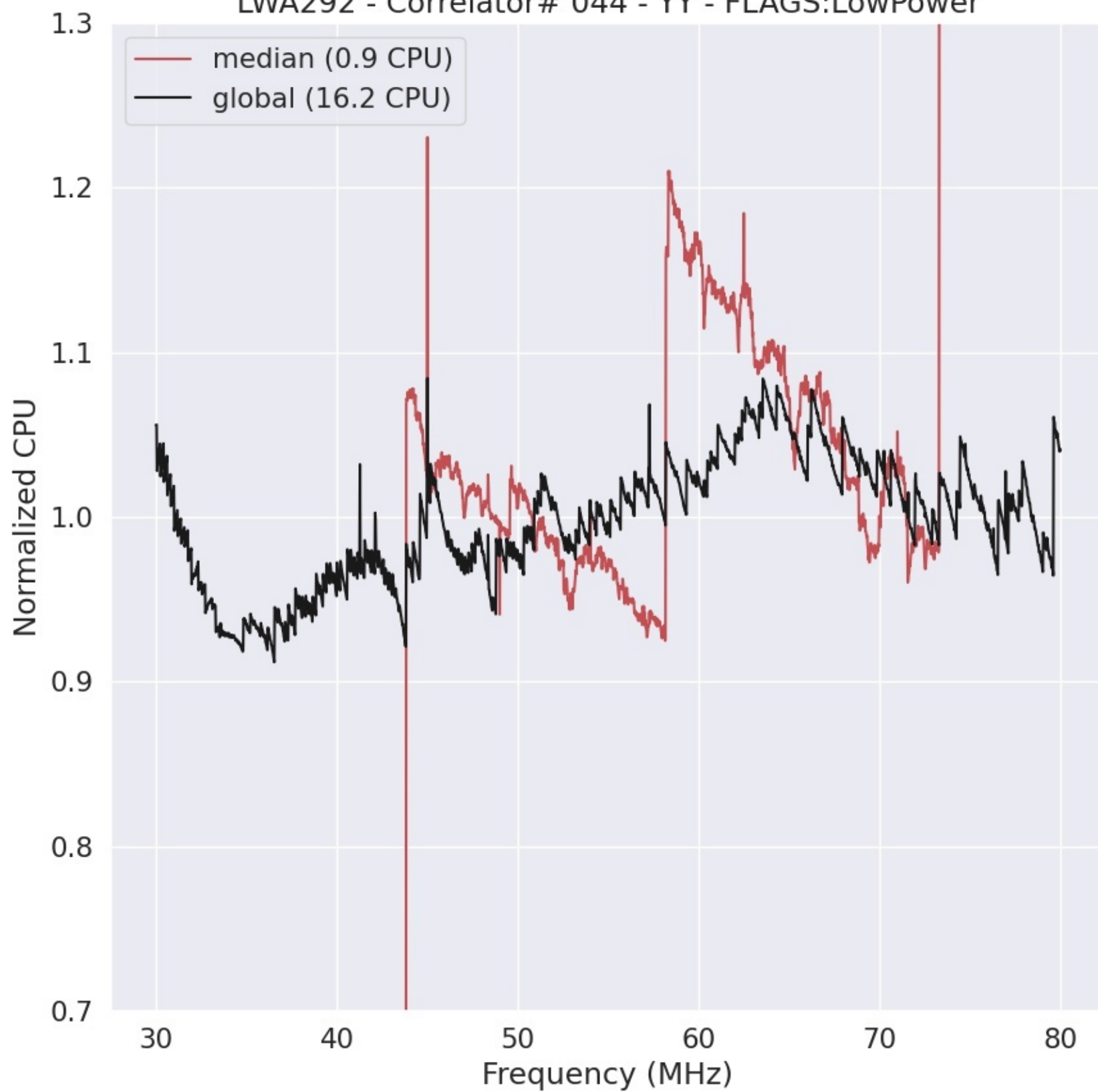
LWA292 - Correlator# 044 - YY - FLAGS:LowPower
