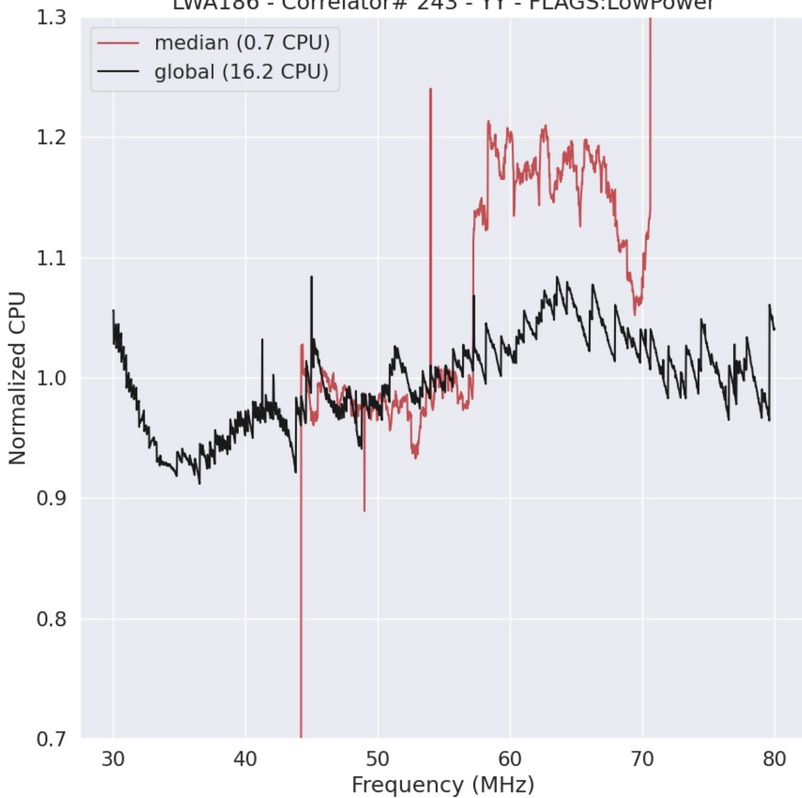
LWA186 - Correlator# 243 - YY - FLAGS:LowPower
