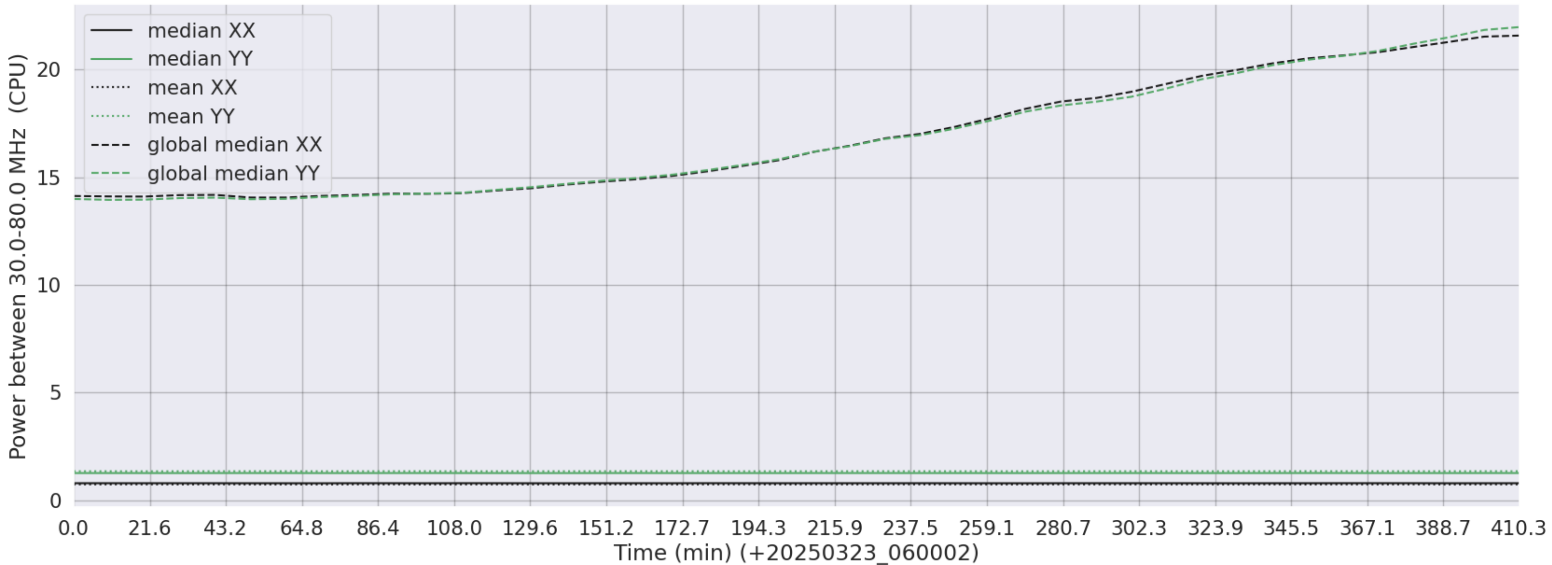
LWA261 - Correlator# 346 - XX FLAGS:LowPower - YY FLAGS:LowPower
