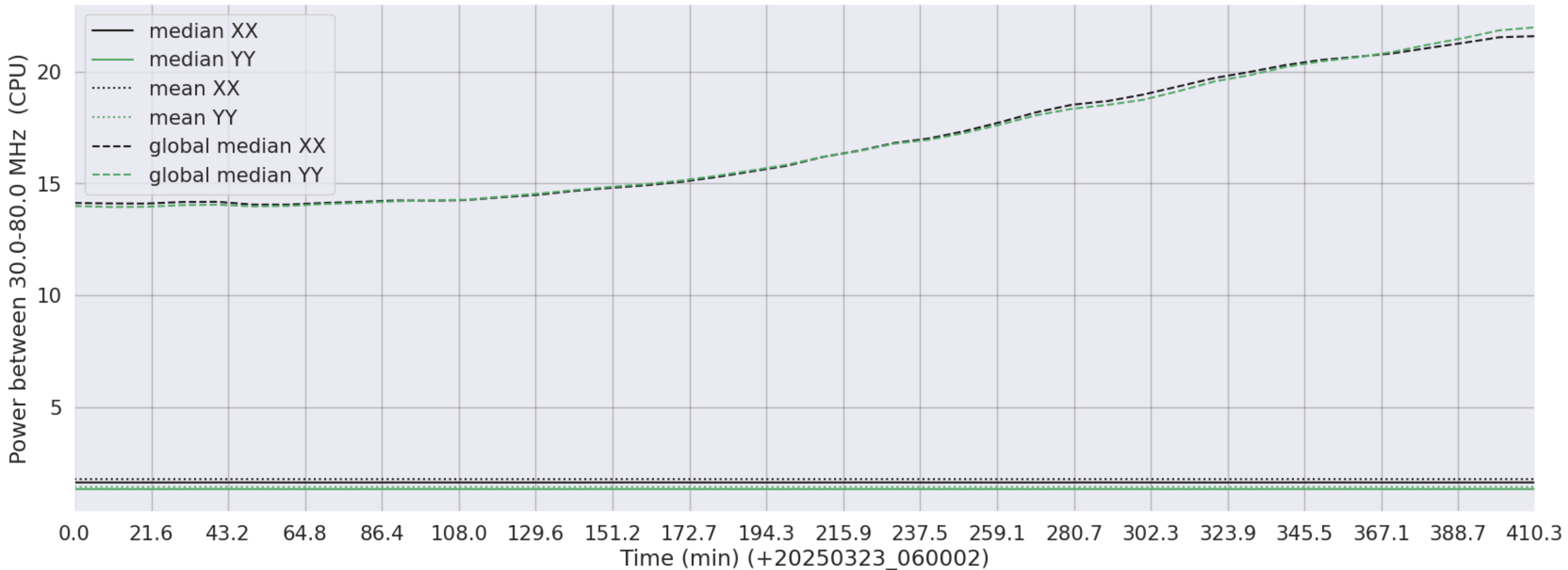
LWA340 - Correlator# 026 - XX FLAGS:LowPower - YY FLAGS:LowPower
