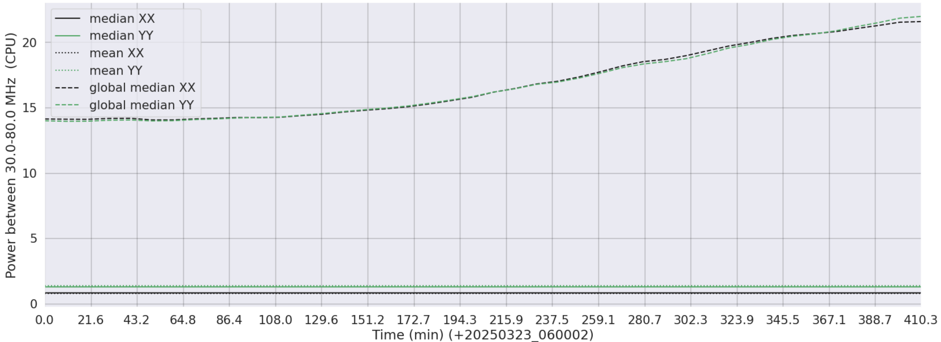
LWA267 - Correlator# 003 - XX FLAGS:LowPower - YY FLAGS:LowPower
