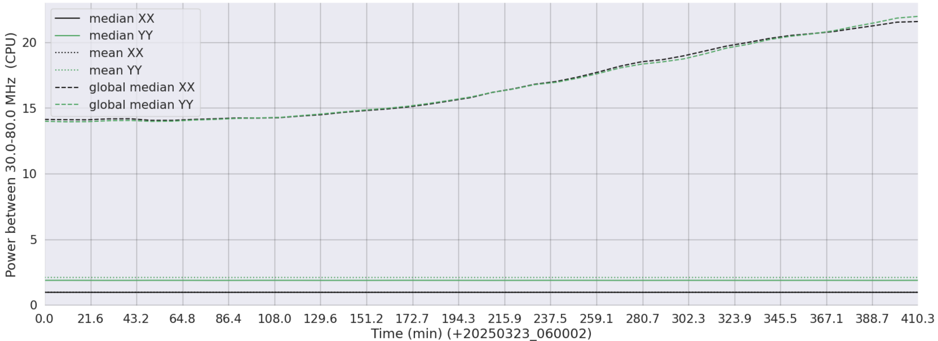
LWA332 - Correlator# 025 - XX FLAGS:LowPower - YY FLAGS:LowPower
