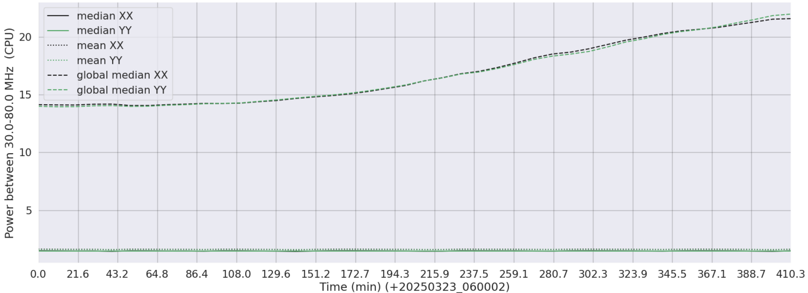
LWA334 - Correlator# 156 - XX FLAGS:LowPower - YY FLAGS:LowPower
