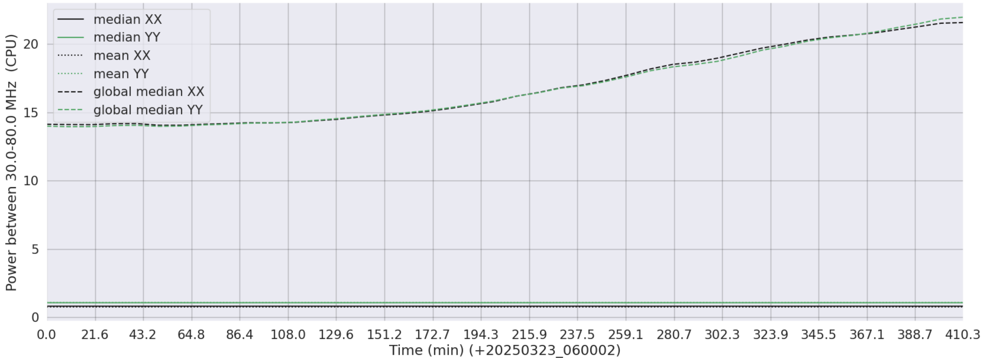
LWA314 - Correlator# 021 - XX FLAGS:LowPower - YY FLAGS:LowPower
