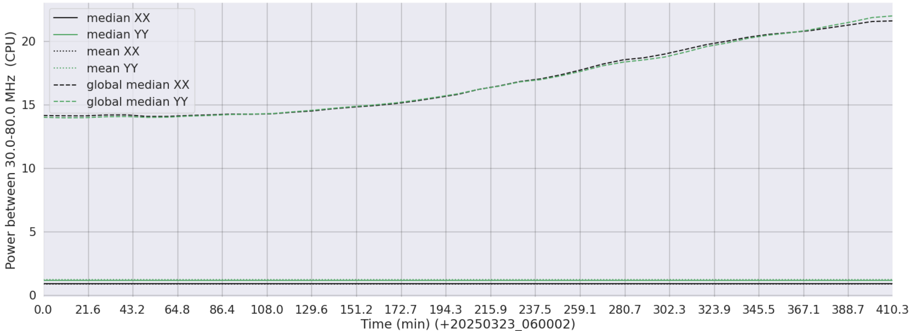
LWA325 - Correlator# 154 - XX FLAGS:LowPower - YY FLAGS:LowPower
