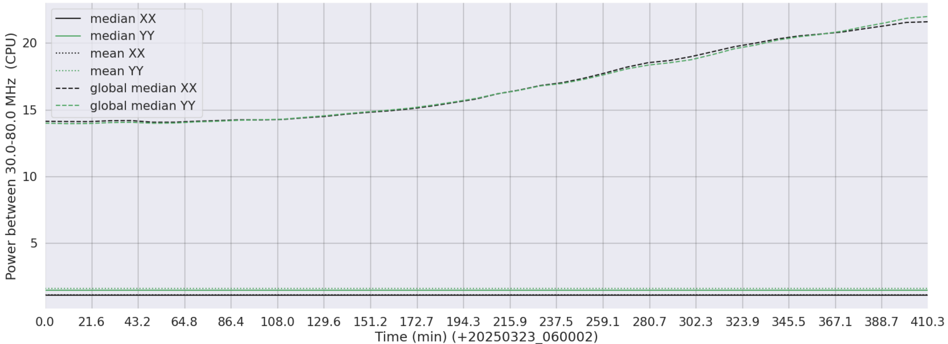
LWA268 - Correlator# 002 - XX FLAGS:LowPower - YY FLAGS:LowPower
