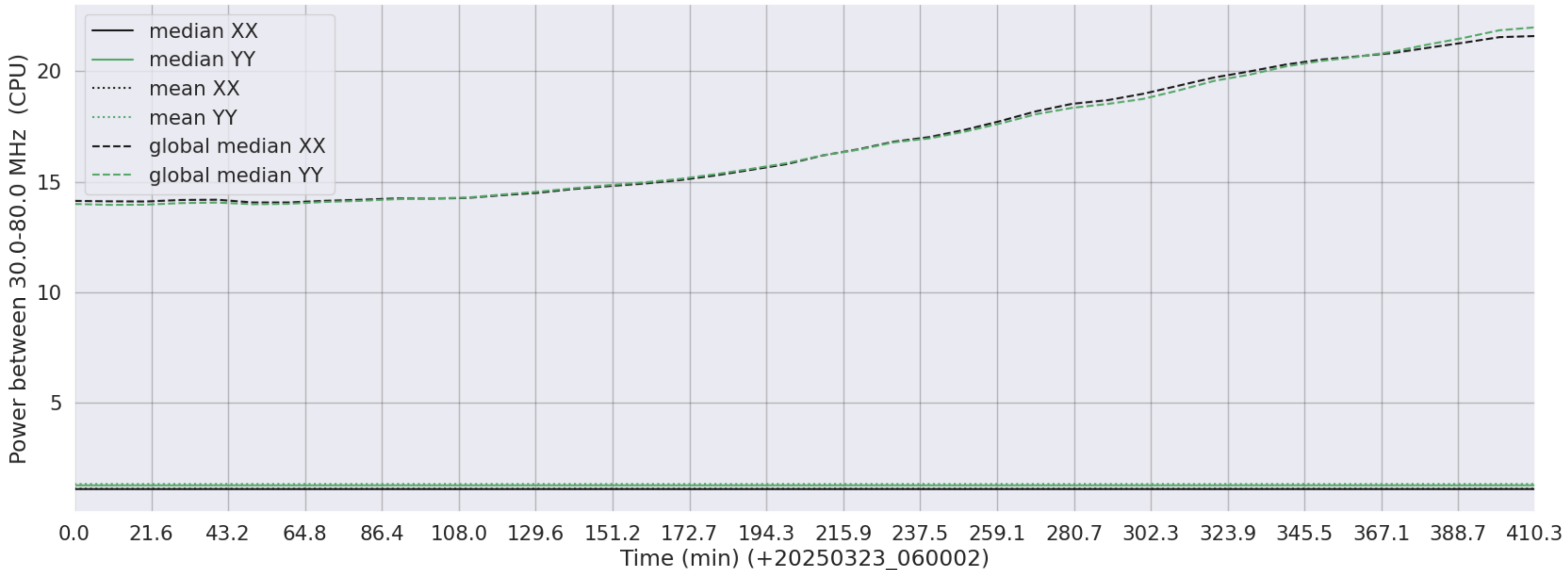
LWA282 - Correlator# 010 - XX FLAGS:LowPower - YY FLAGS:LowPower
