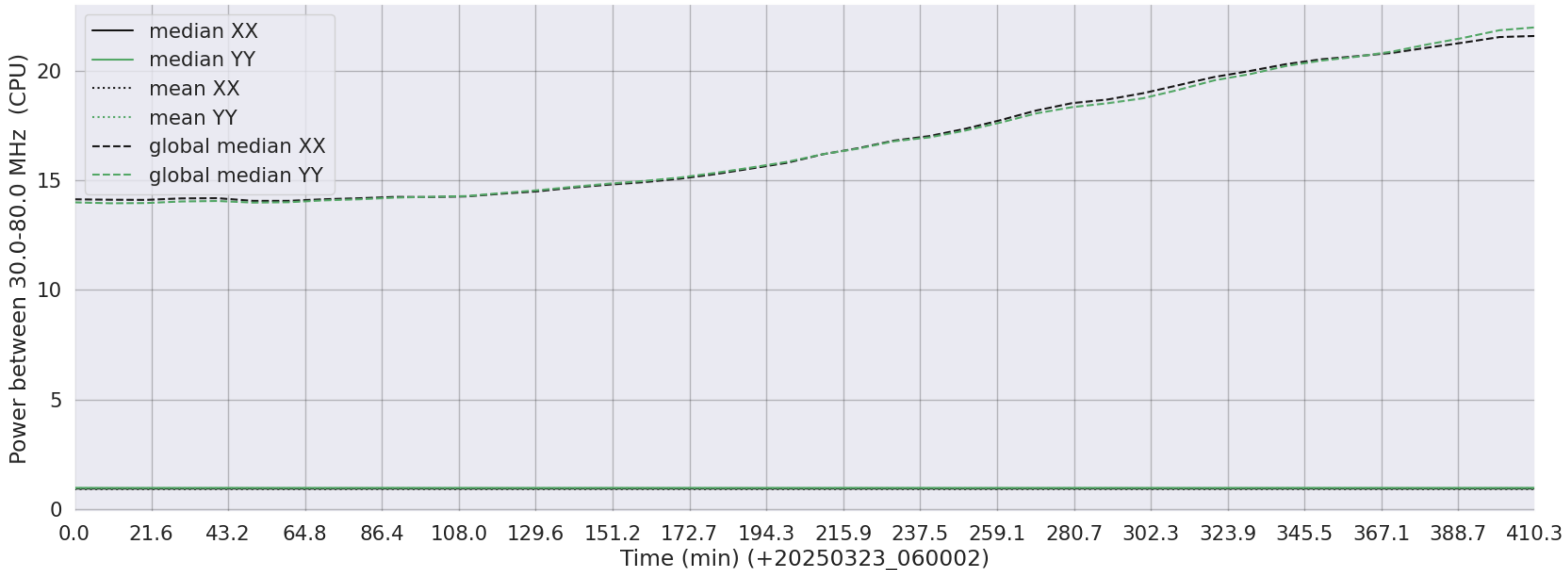
LWA307 - Correlator# 012 - XX FLAGS:LowPower - YY FLAGS:LowPower
