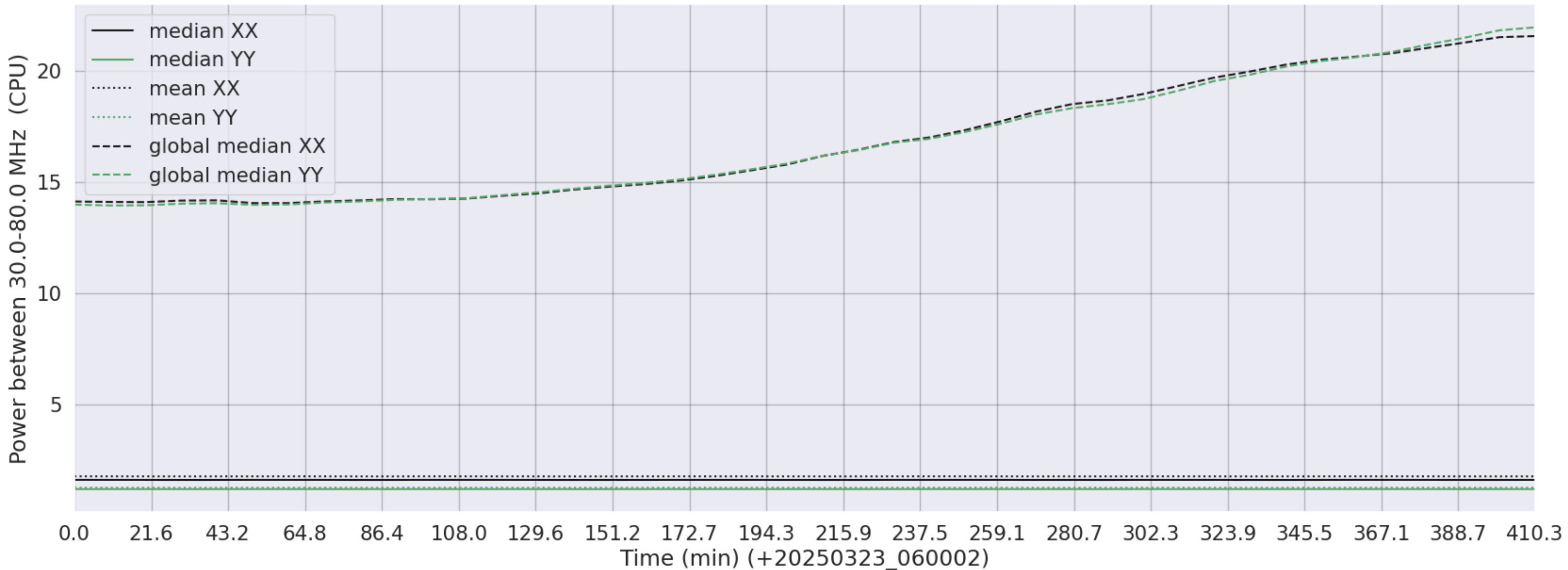
LWA310 - Correlator# 017 - XX FLAGS:LowPower - YY FLAGS:LowPower
