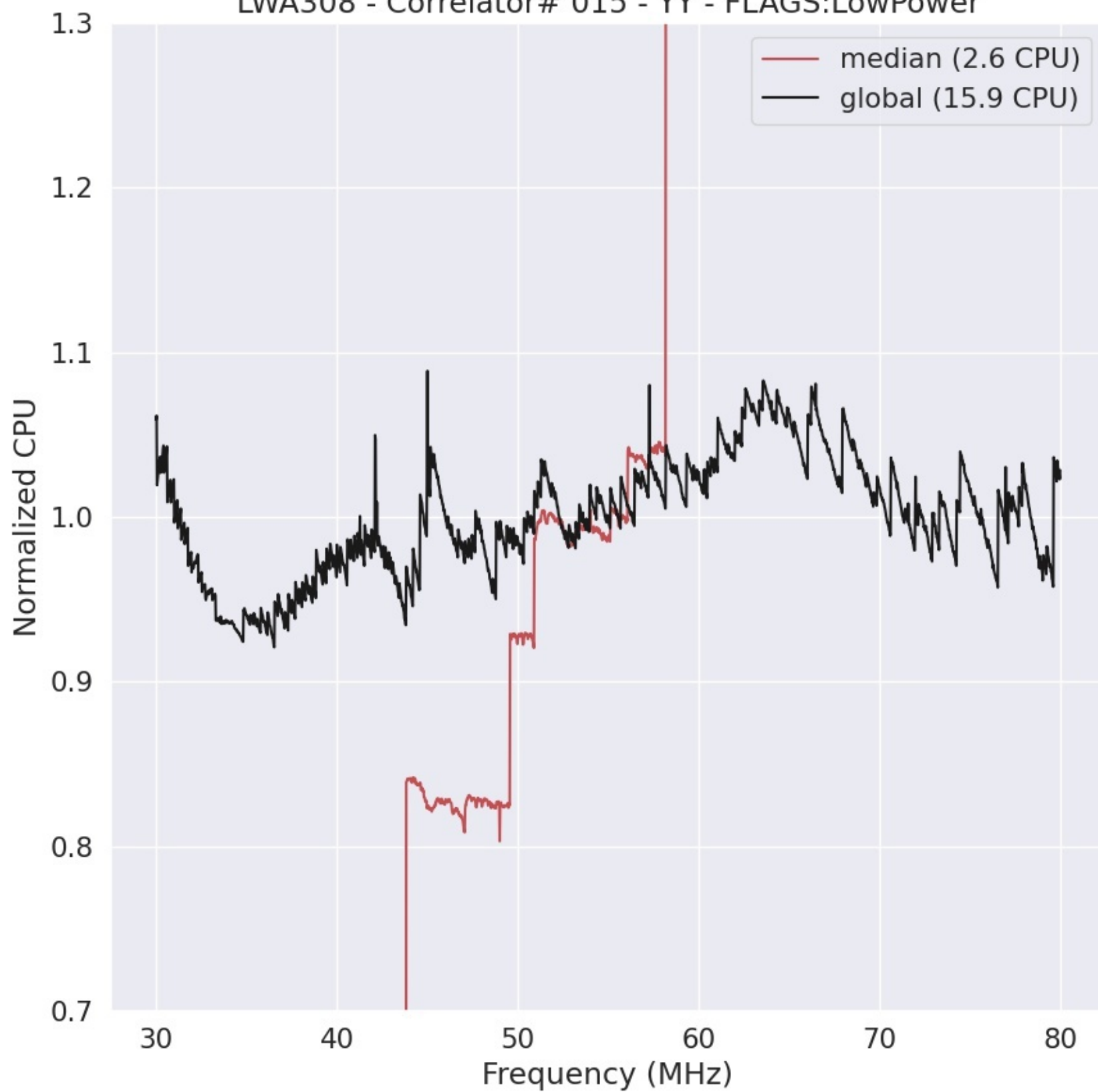
LWA308 - Correlator# 015 - YY - FLAGS:LowPower
