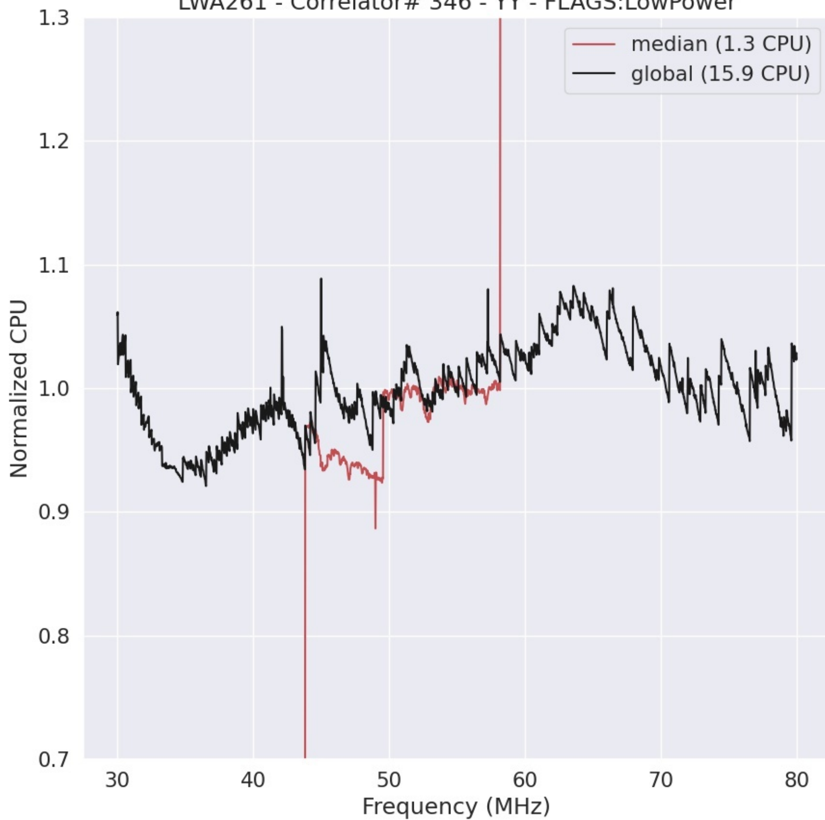
LWA261 - Correlator# 346 - YY - FLAGS:LowPower
