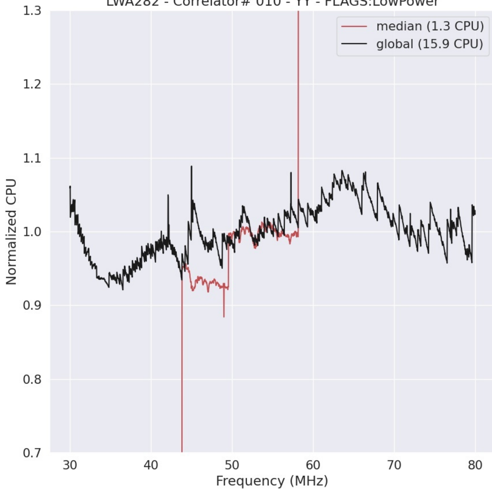
LWA282 - Correlator# 010 - YY - FLAGS:LowPower
