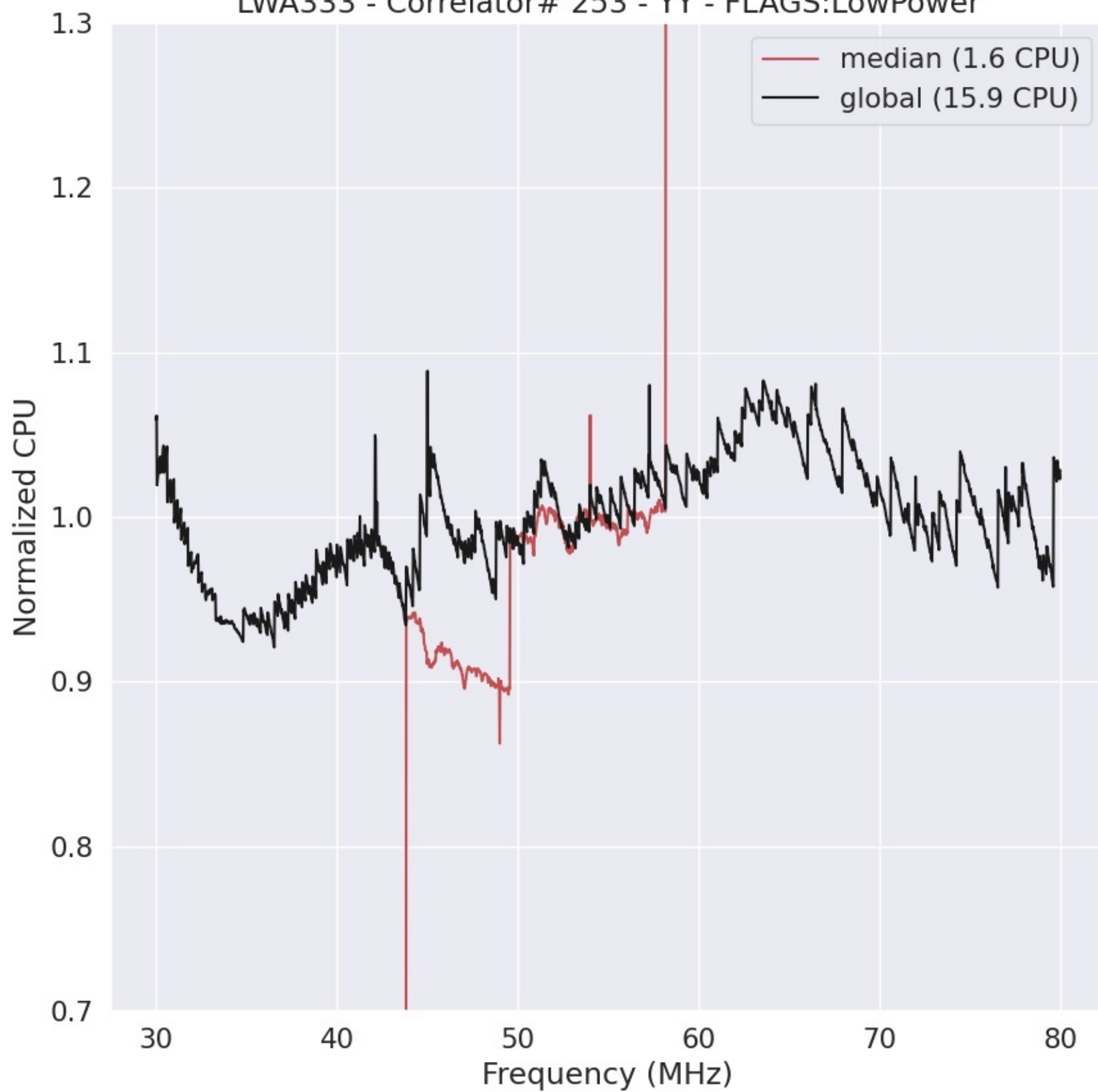
LWA333 - Correlator# 253 - YY - FLAGS:LowPower
