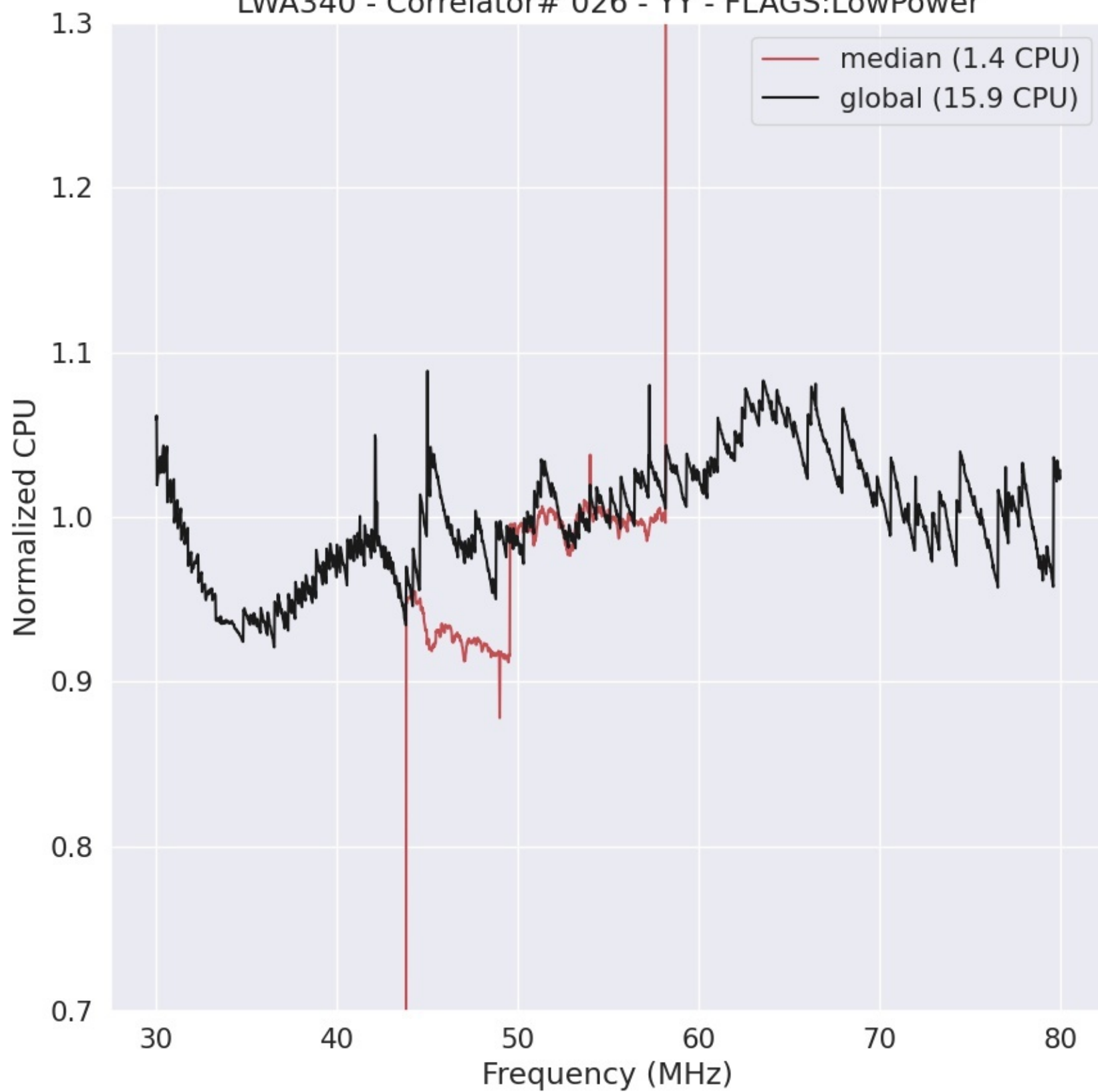
LWA340 - Correlator# 026 - YY - FLAGS:LowPower
