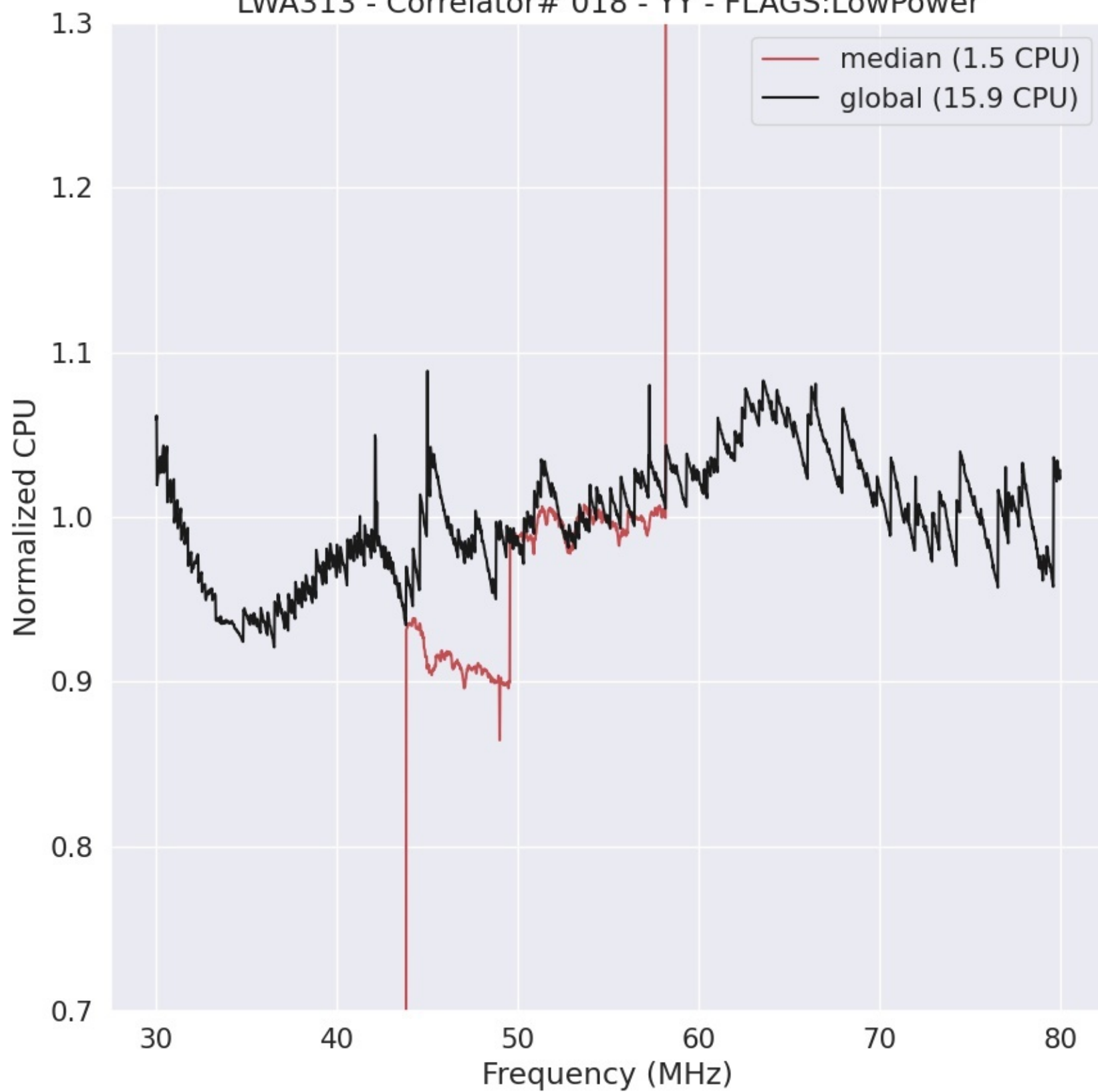
LWA313 - Correlator# 018 - YY - FLAGS:LowPower
