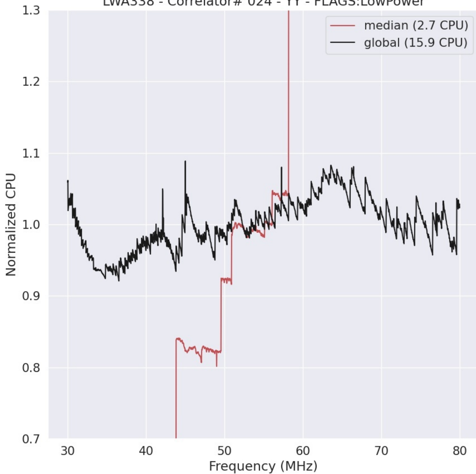
LWA338 - Correlator# 024 - YY - FLAGS:LowPower
