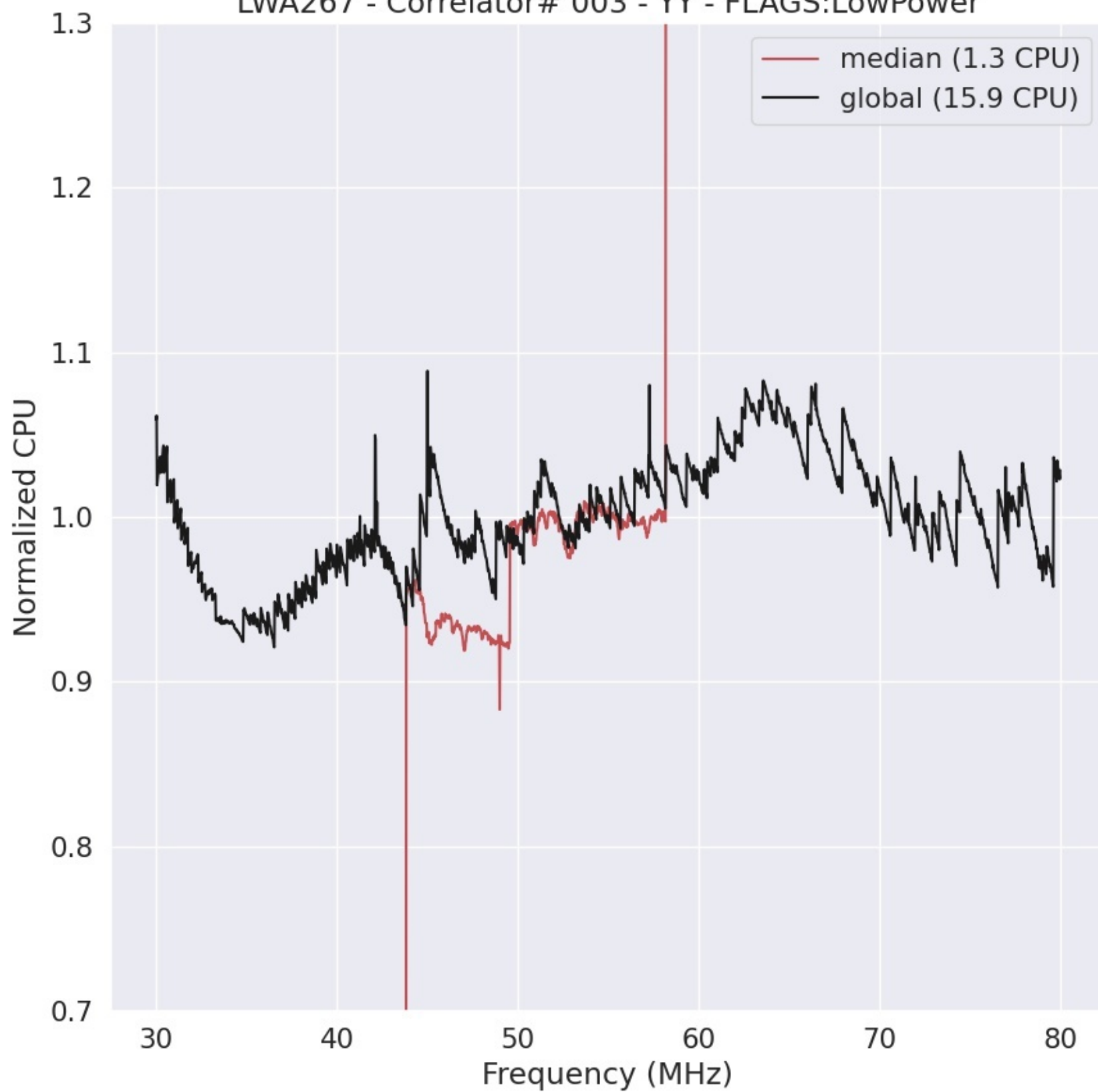
LWA267 - Correlator# 003 - YY - FLAGS:LowPower
