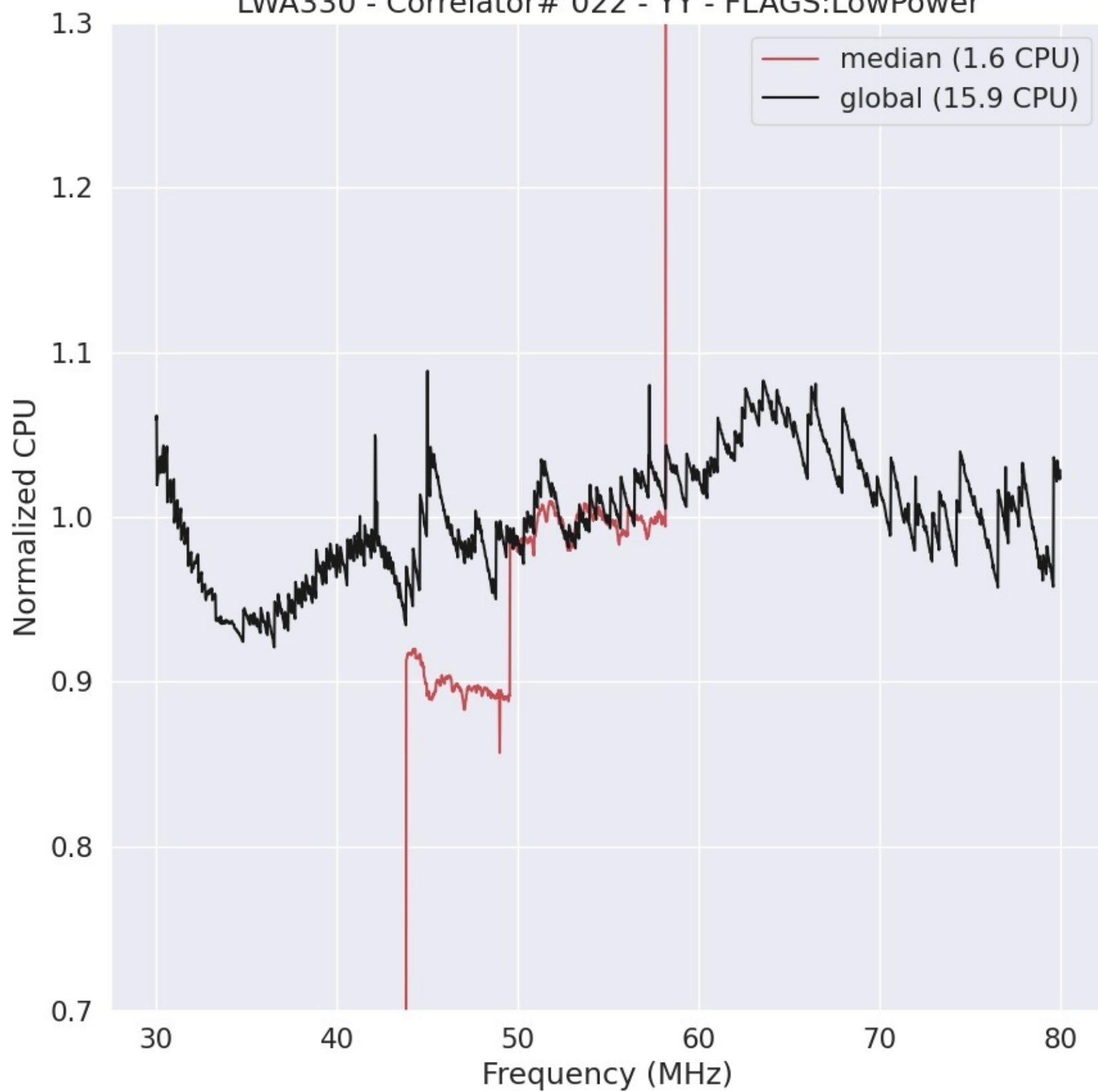
LWA330 - Correlator# 022 - YY - FLAGS:LowPower
