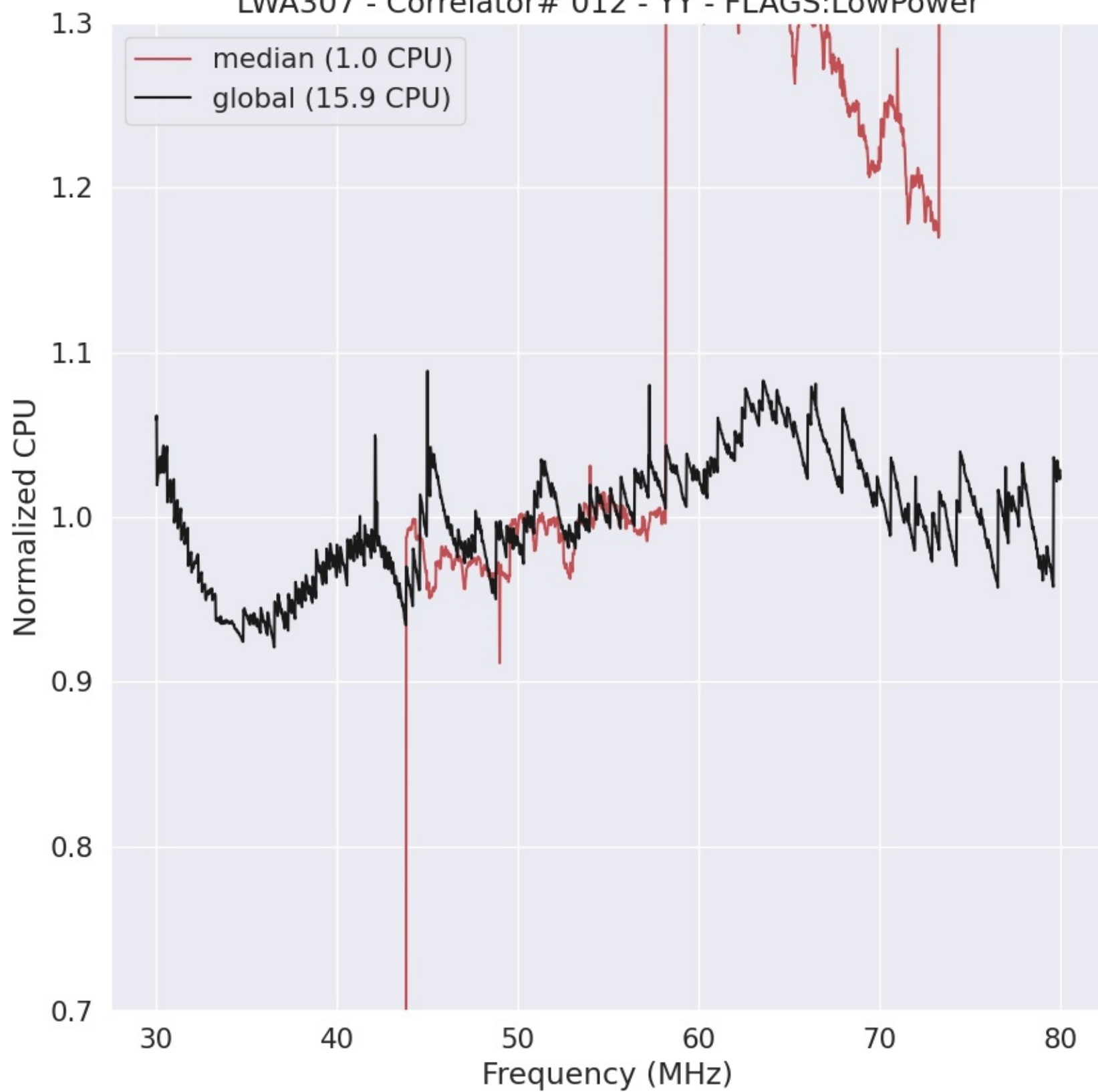
LWA307 - Correlator# 012 - YY - FLAGS:LowPower
