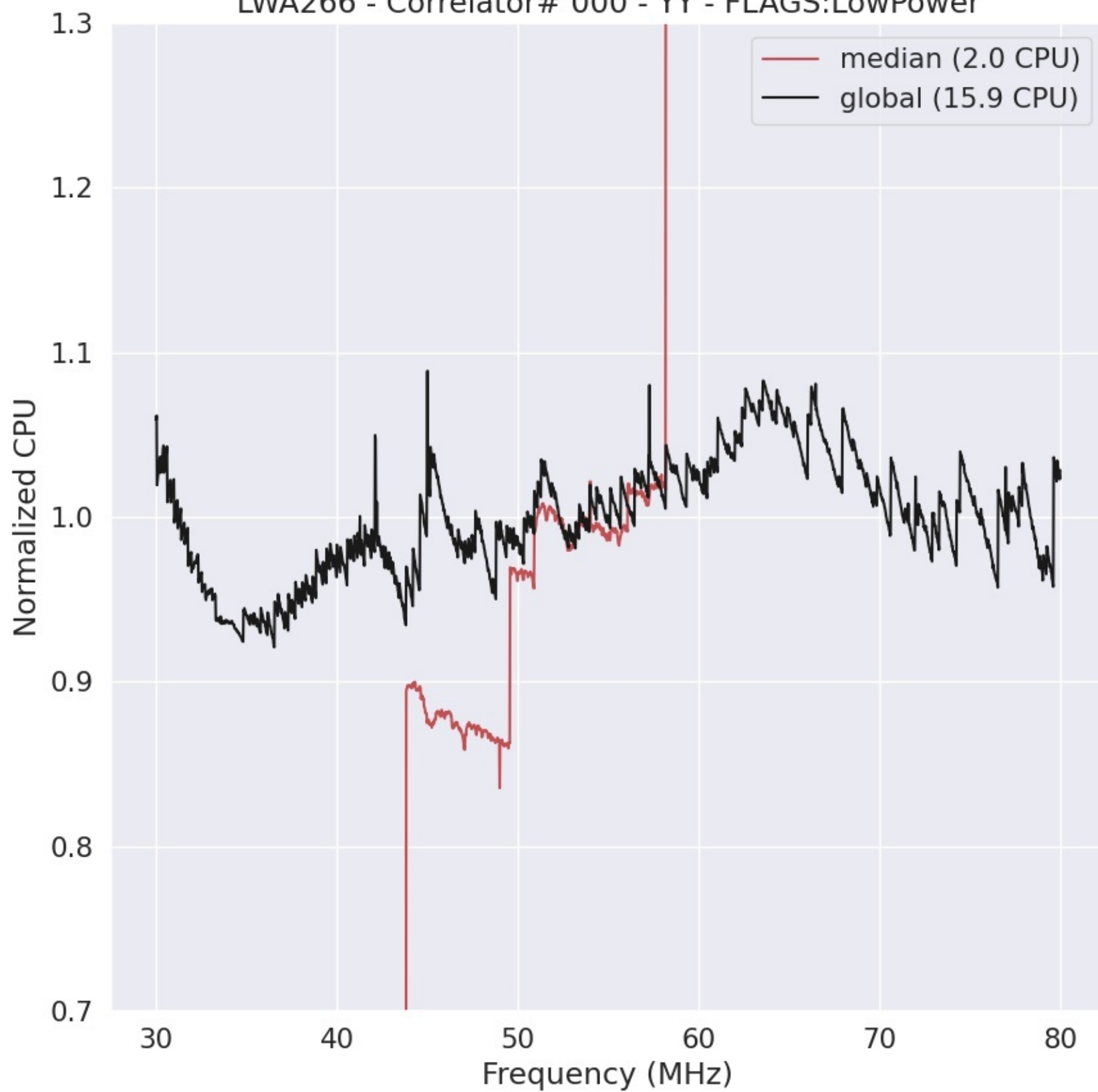
LWA266 - Correlator# 000 - YY - FLAGS:LowPower
