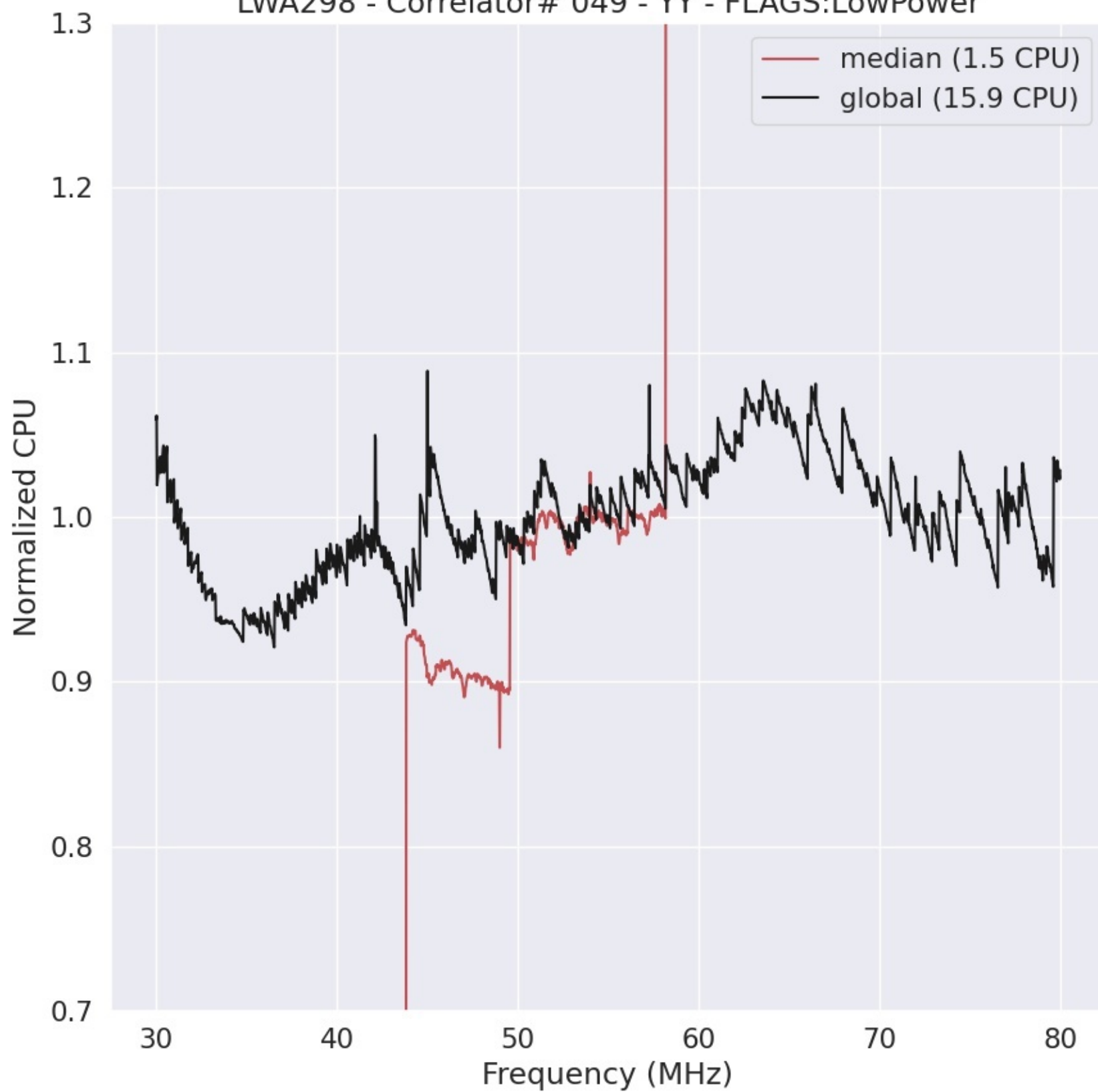
LWA298 - Correlator# 049 - YY - FLAGS:LowPower
