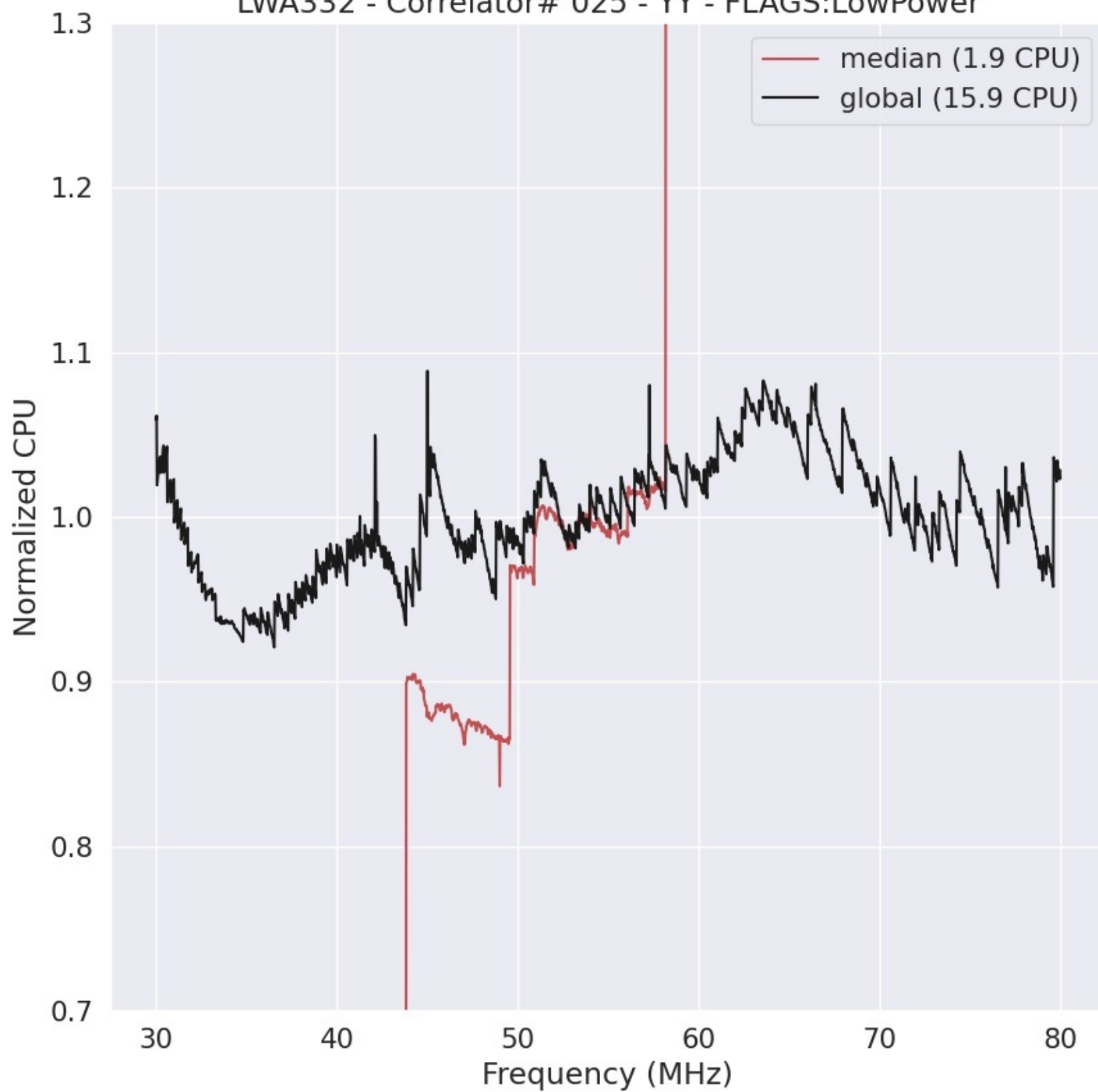
LWA332 - Correlator# 025 - YY - FLAGS:LowPower
