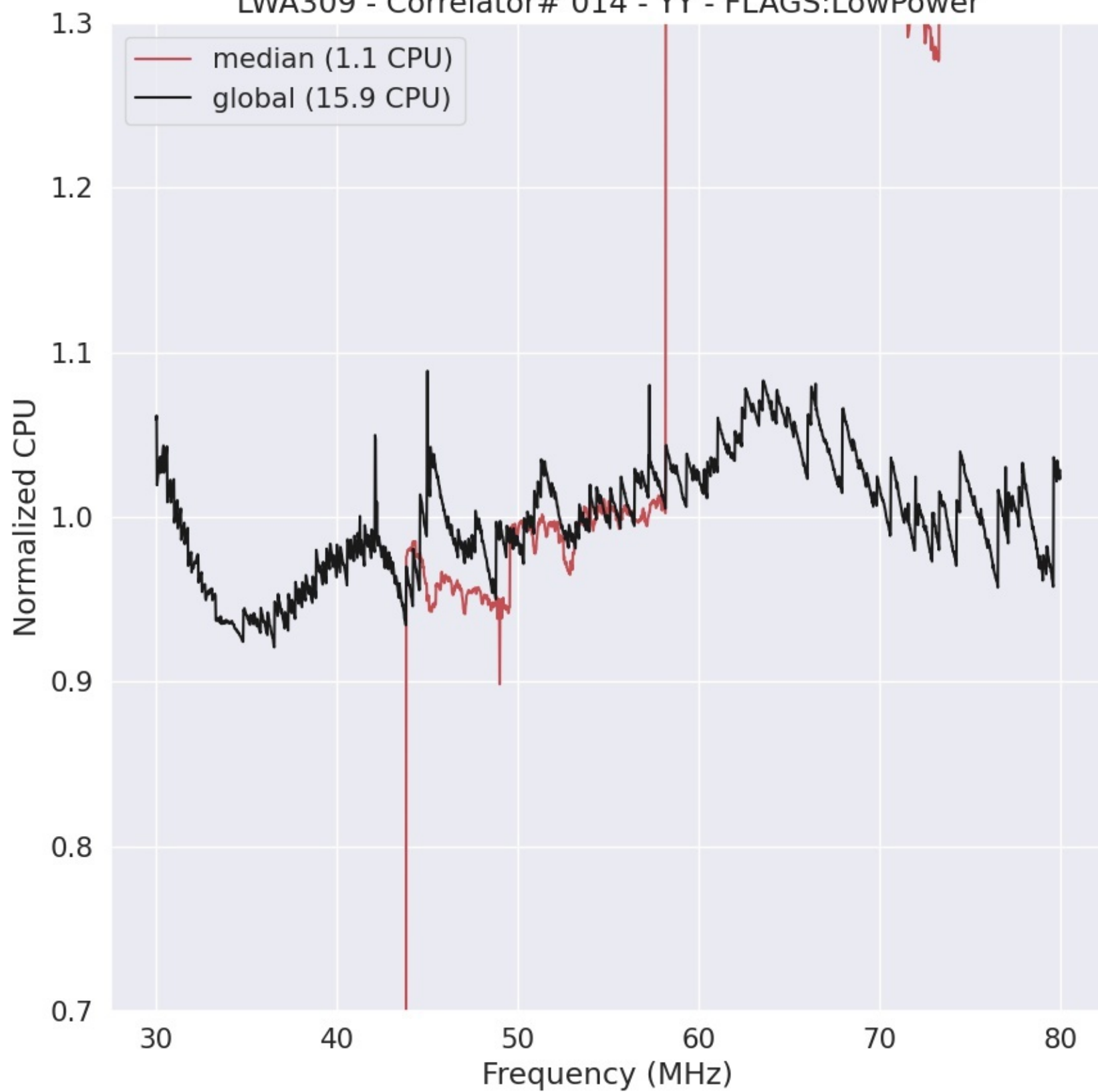
LWA309 - Correlator# 014 - YY - FLAGS:LowPower
