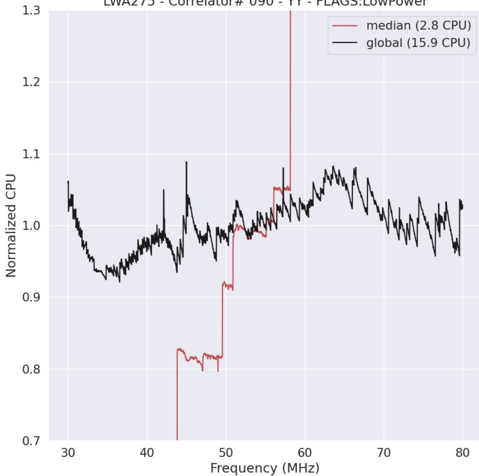
LWA275 - Correlator# 090 - YY - FLAGS:LowPower
