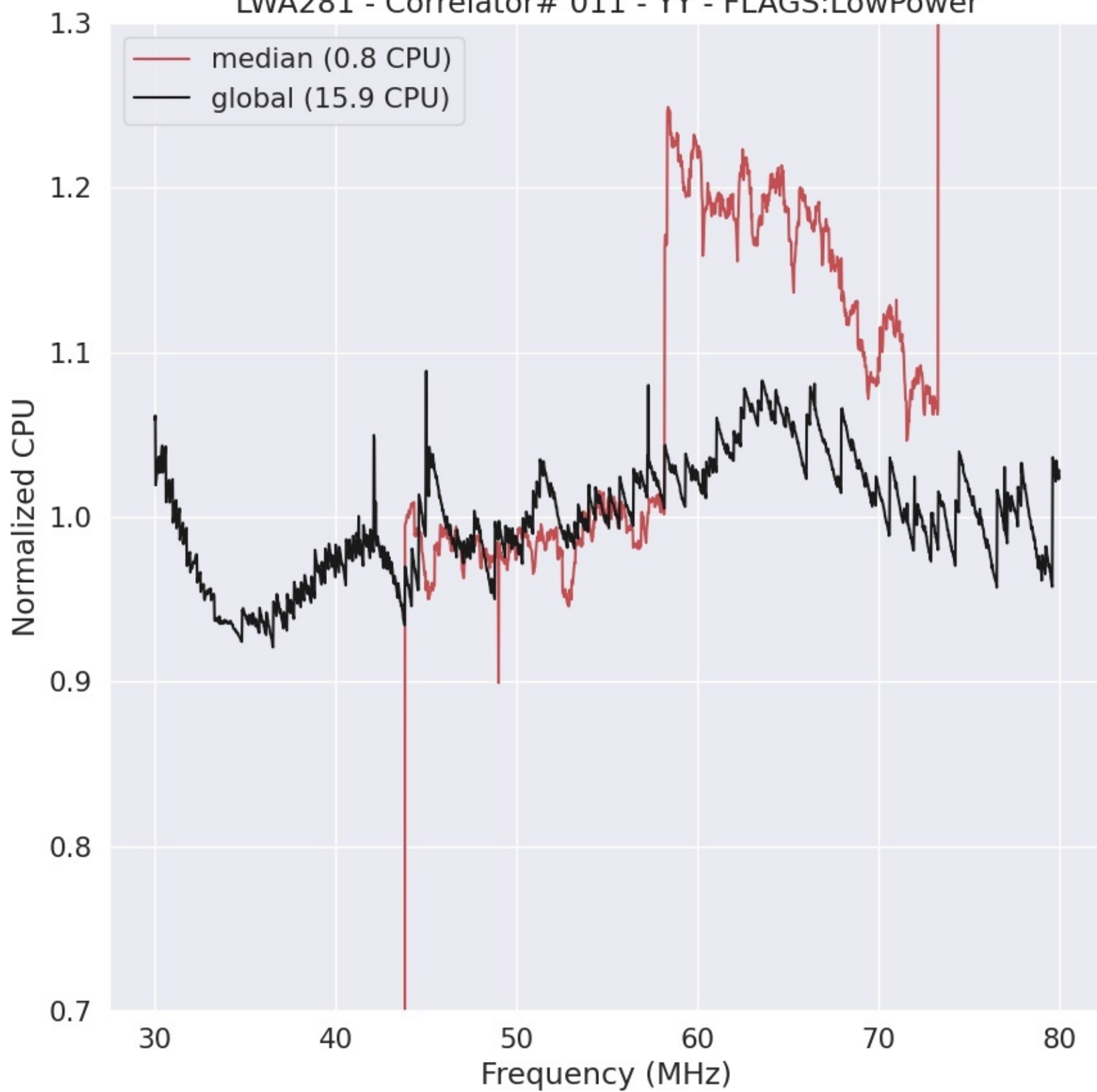
LWA281 - Correlator# 011 - YY - FLAGS:LowPower
