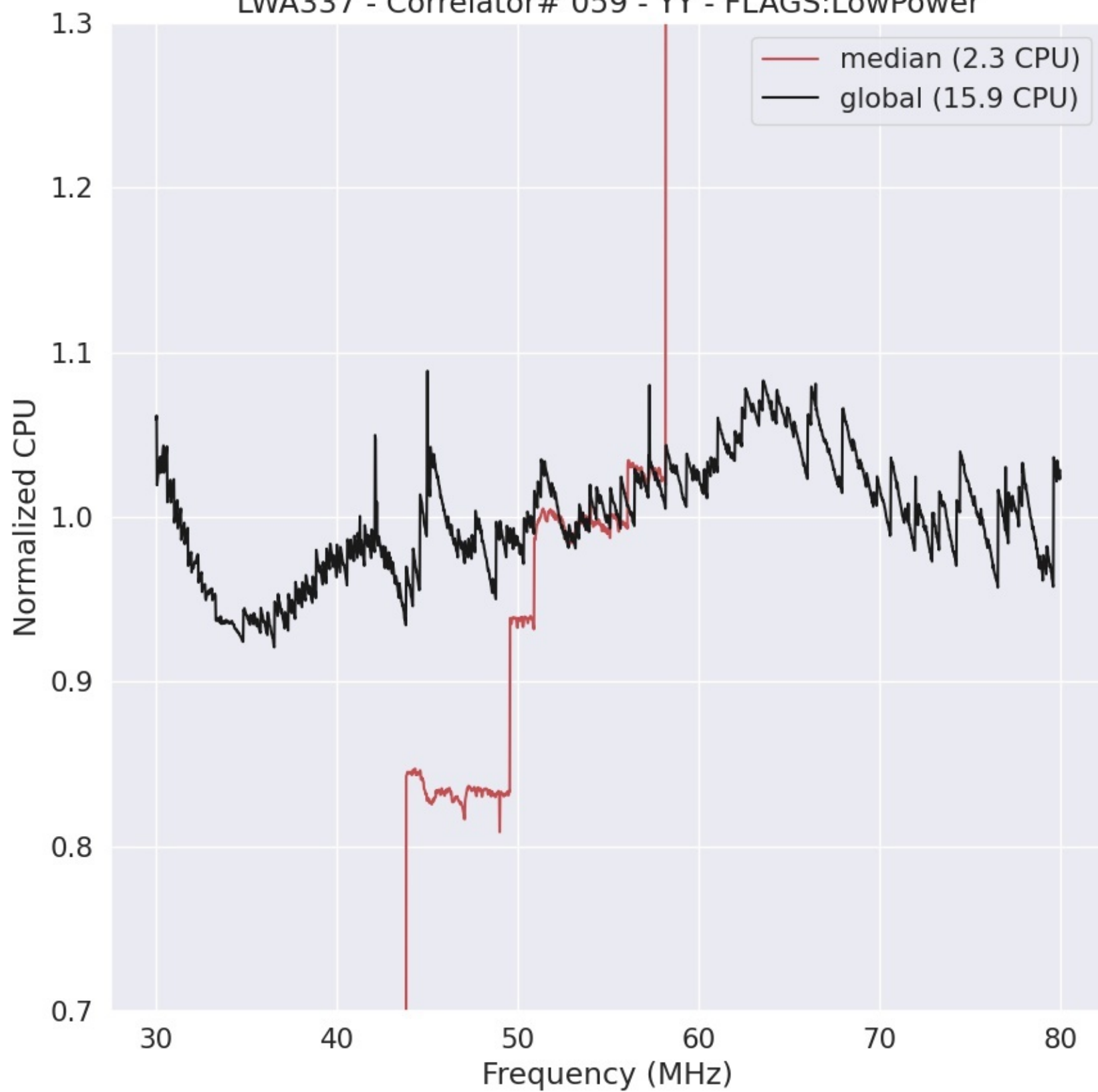
LWA337 - Correlator# 059 - YY - FLAGS:LowPower
