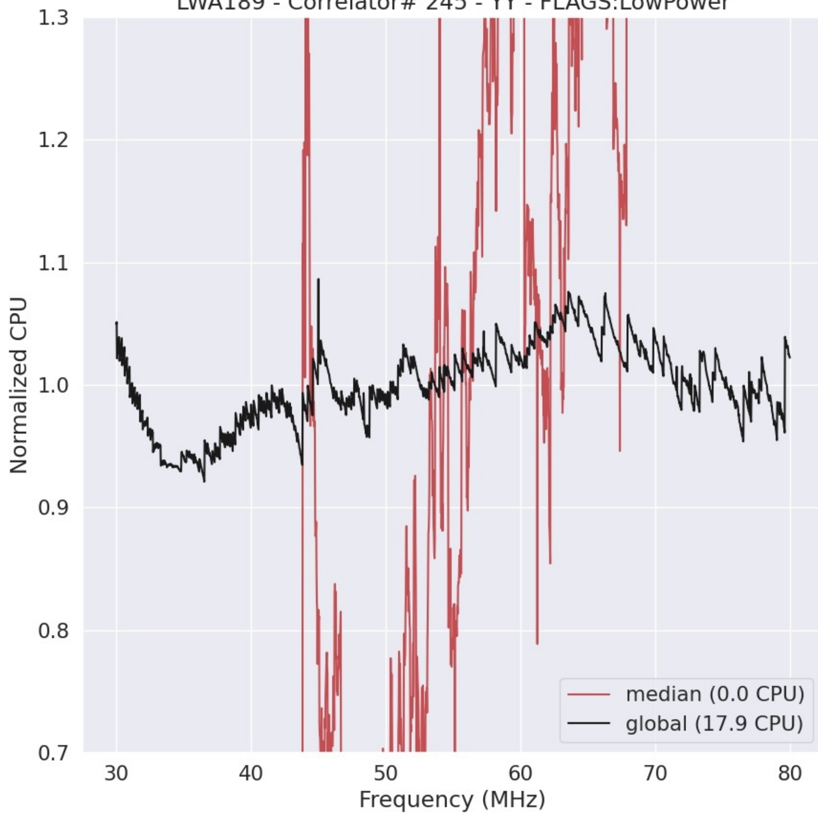
LWA189 - Correlator# 245 - YY - FLAGS:LowPower
