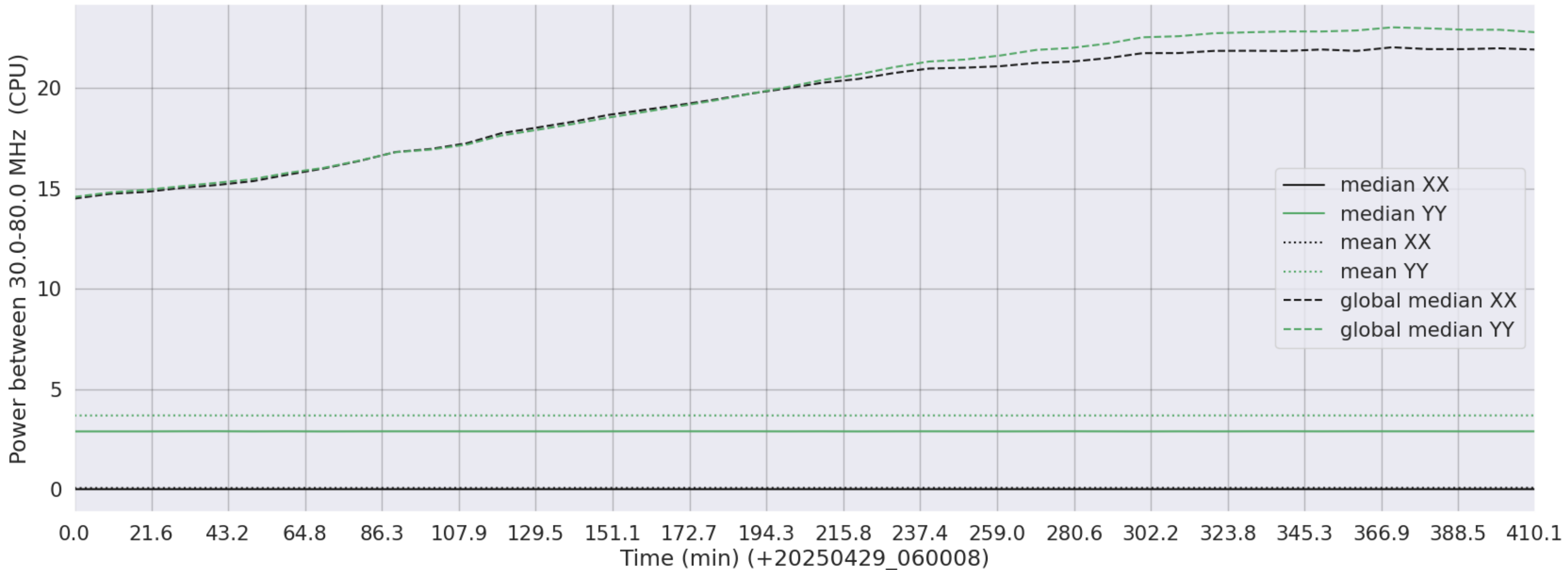
LWA209 - Correlator# 301 - XX FLAGS:LowPower - YY FLAGS:LowPower
